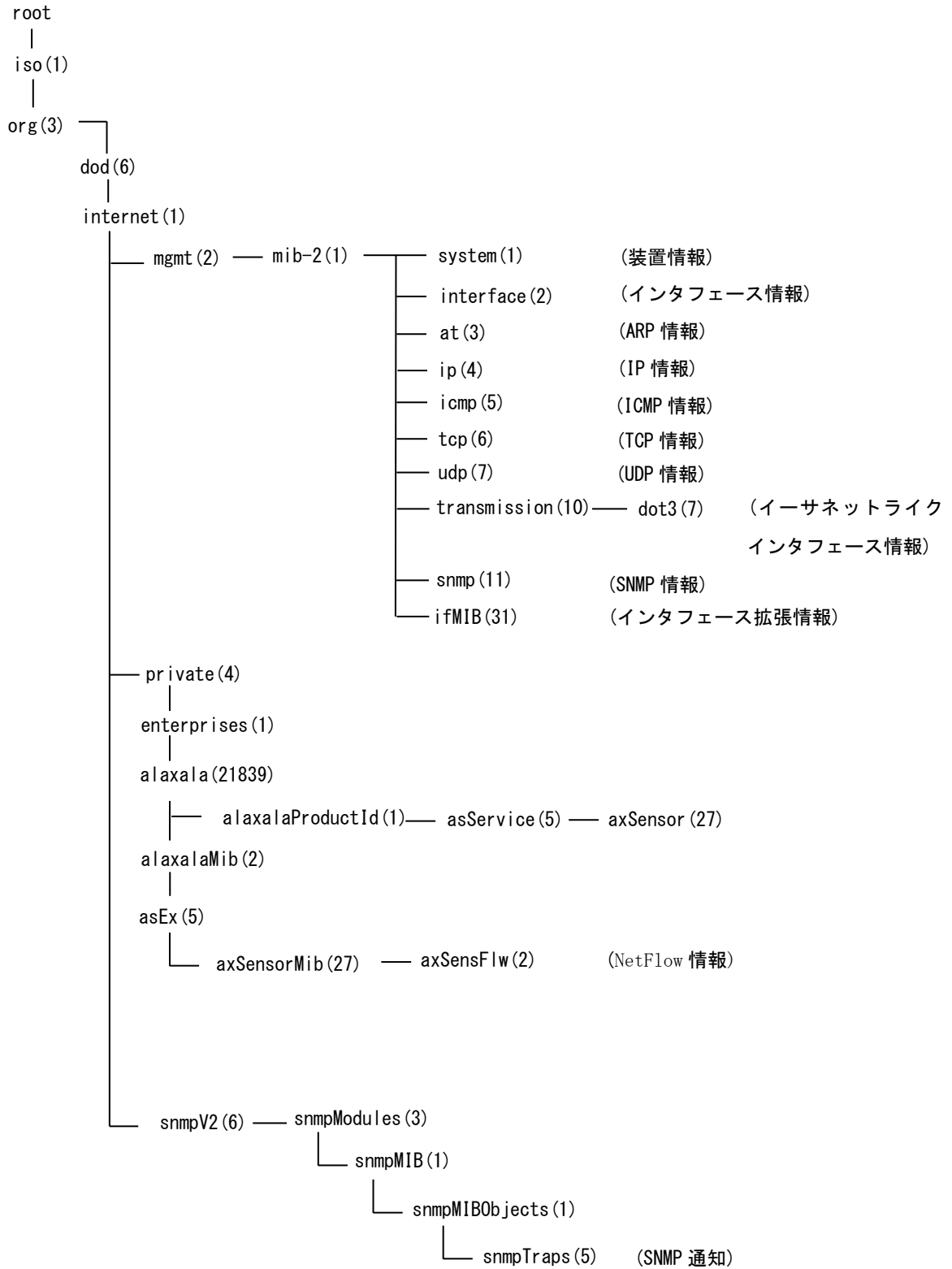
図 1.1-1 MIB 体系図
