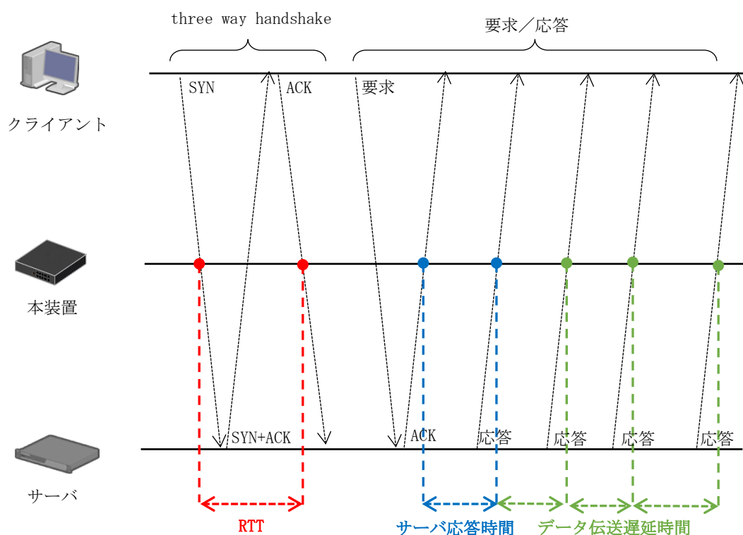
図 6.1-7 TCP通信の測定方法
