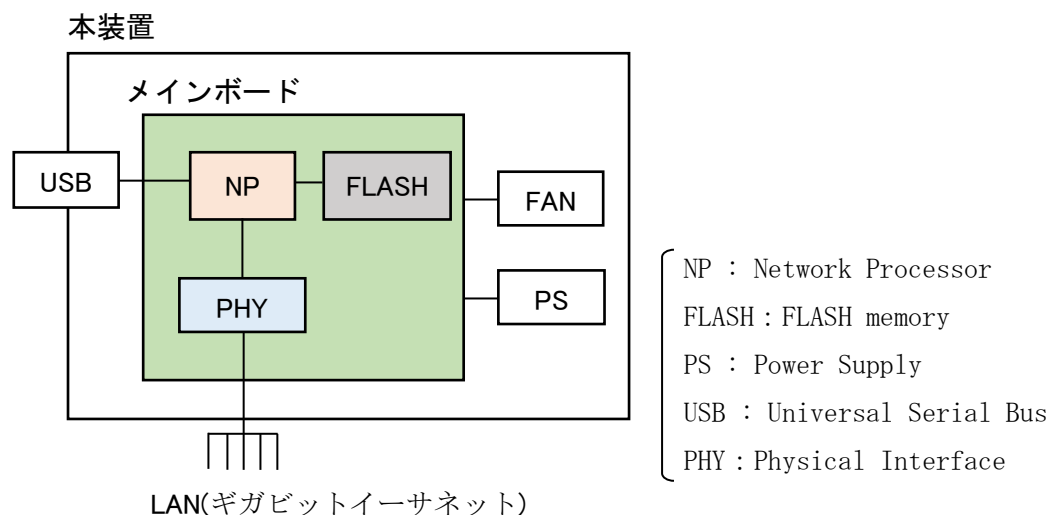
図 1.3-3 ハードウェア構成 (AX-Sensor-08T モデル)
