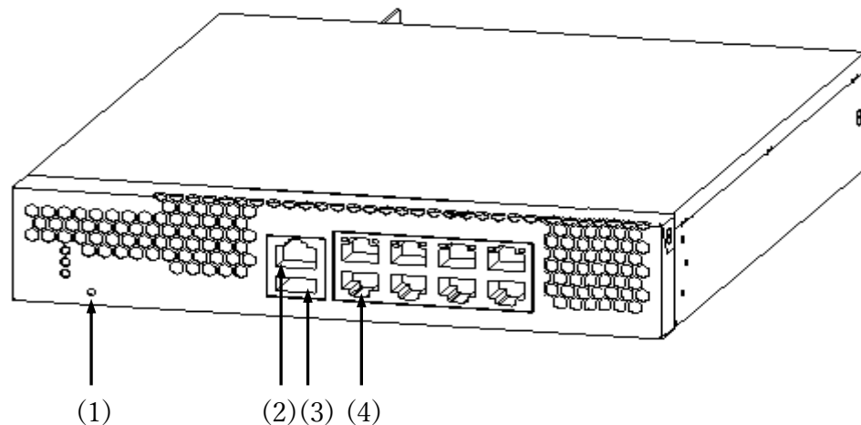
図 1.3-1 AX-Sensor-08T モデル
