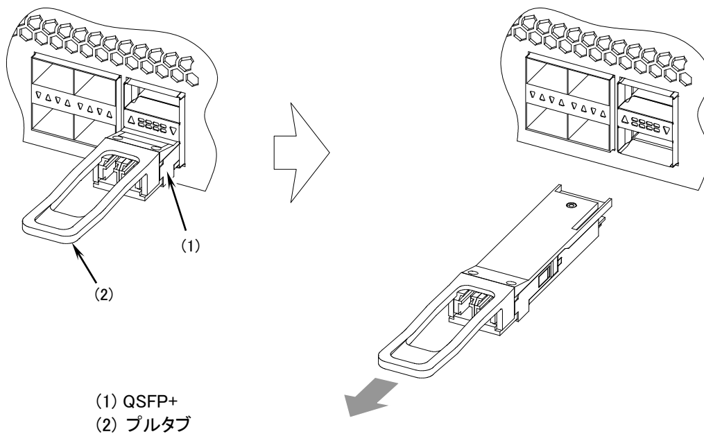
図2-8 QSFP+の取り外し（プルタブタイプの場合）
