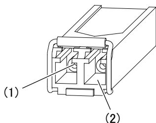
図 A-1 光コネクタとフェルール端面
