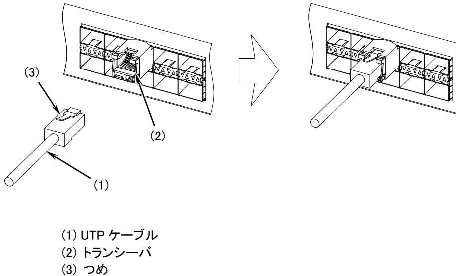
図2-11 UTP ケーブルの取り付け
