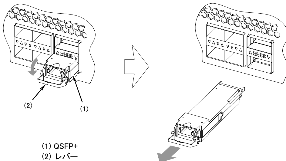
図2-7 QSFP+の取り外し（レバータイプの場合）
