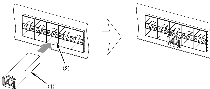
図2-2 SFP の取り付け（下側のポート）
