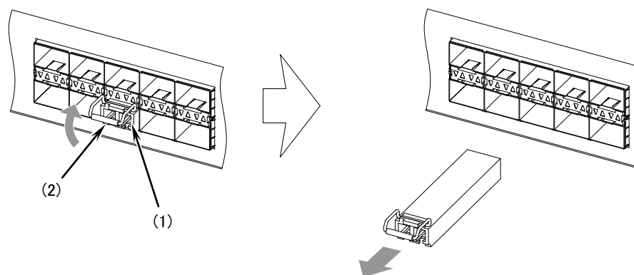
図2-4 SFP の取り外し（下側のポート）
