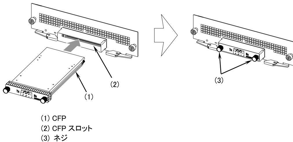
図2-9 CFP の取り付け
