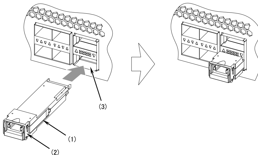
図2-5 QSFP+の取り付け（レバータイプの場合）
