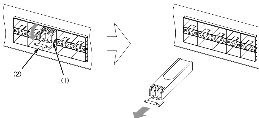
図2-3 SFP の取り外し（上側のポート）
