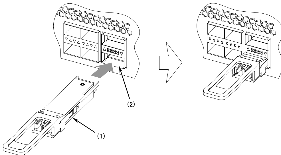
図2-6 QSFP+の取り付け（プルタブタイプの場合）
