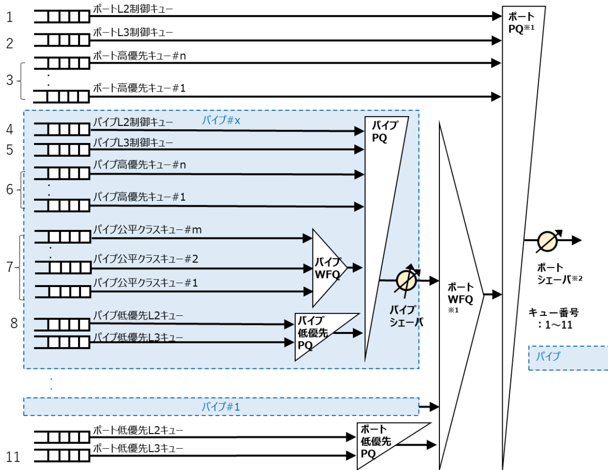
図 3-7 upstream に対するシェーパポートポロジ
