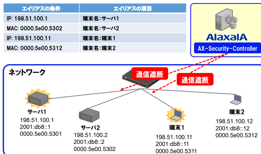
図 1-14 エイリアス未登録端末通信遮断有効時に端末が通信遮断されるケース
