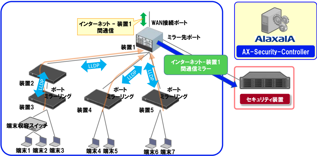
図 1-4 前提とするネットワーク構成例
