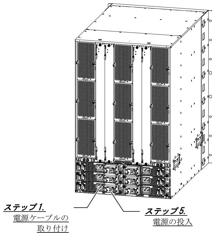
図2-10 AX8632S（背面）概略図
