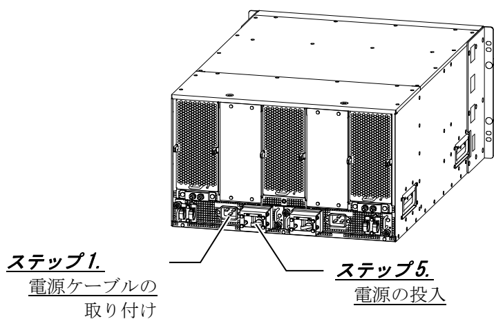
図2-2 AX8608S（背面）概略図
