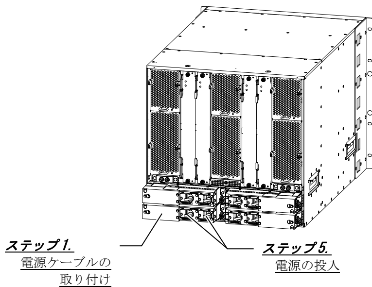
図2-8 AX8616S（背面）概略図
