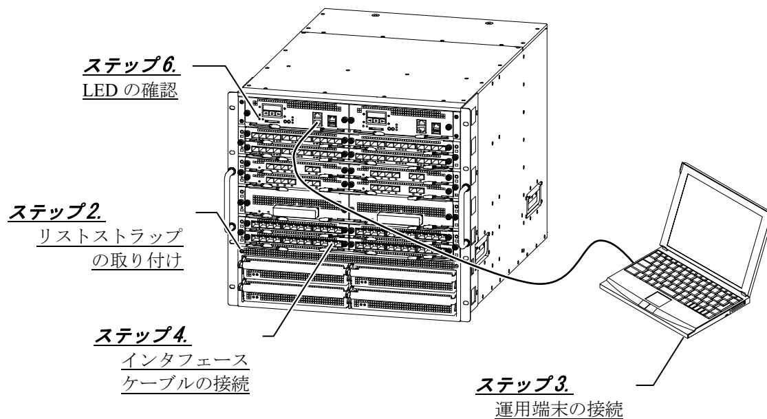
図2-7 AX8616S（正面）概略図
