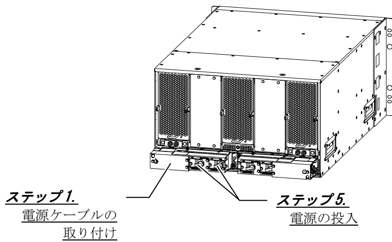
図2-4 AX8608S（背面）概略図
