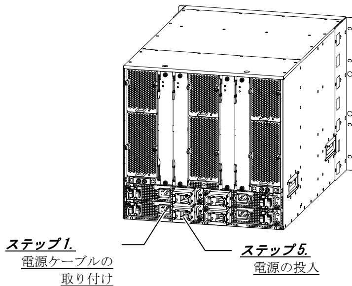
図2-6 AX8616S（背面）概略図
