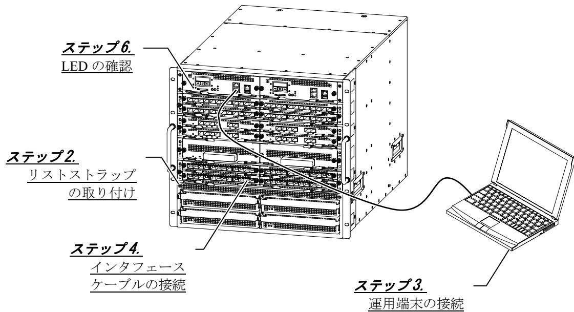
図2-5 AX8616S（正面）概略図
