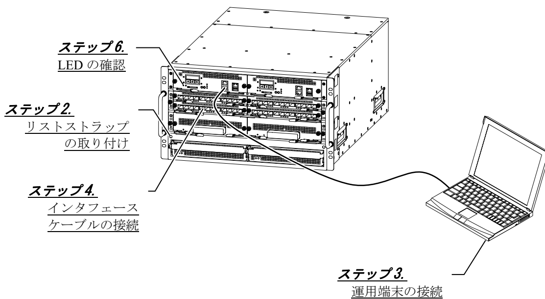
図2-1 AX8608S（正面）概略図
