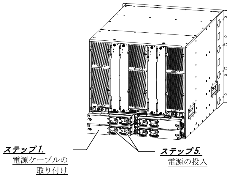
図2-8 AX8616S（背面）概略図
