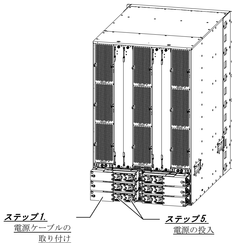
図2-12 AX8632R（背面）概略図
