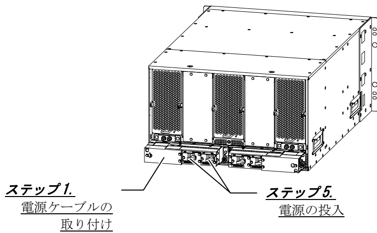
図2-4 AX8608R（背面）概略図
