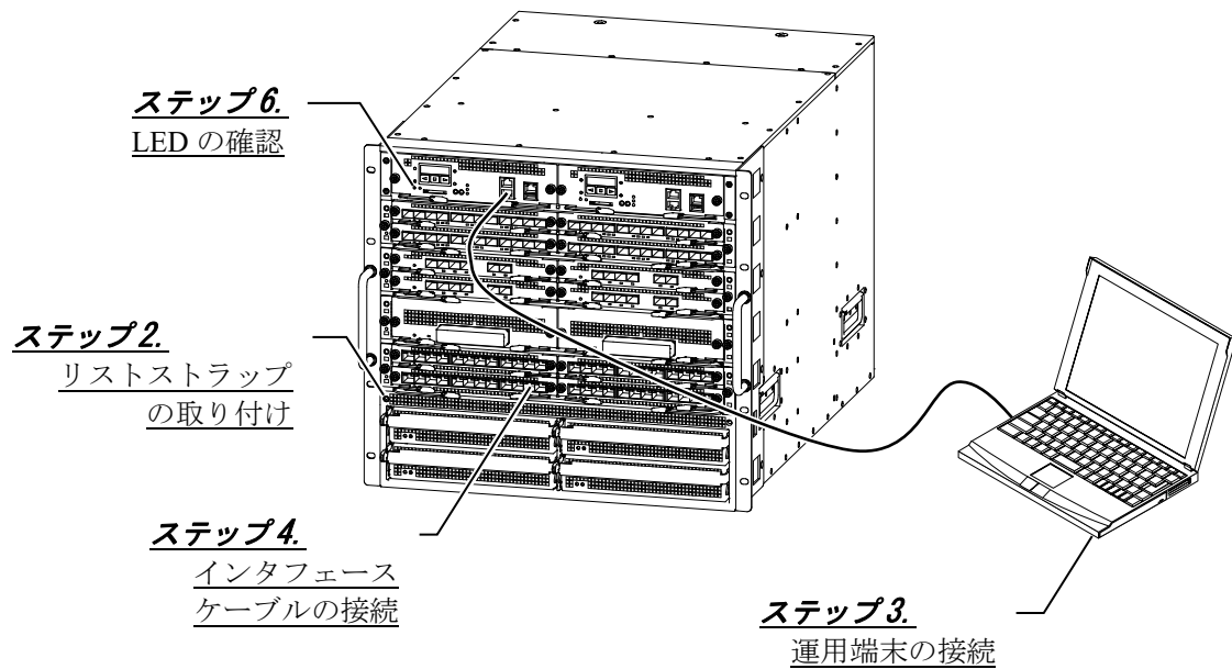
図2-7 AX8616R（正面）概略図
