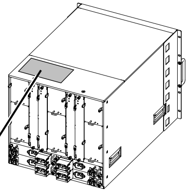
装置（背面側）
