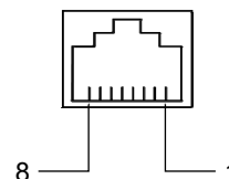
本装置側 RJ-45 のピン配置
