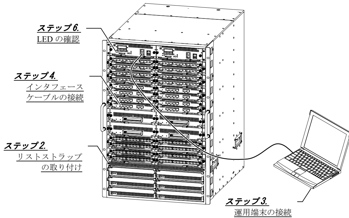
図2-12 AX8632R（背面）概略図
