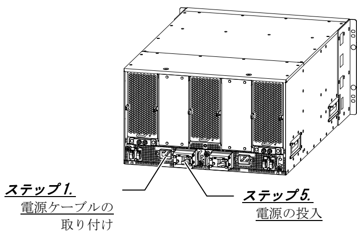
図2-2 AX8608R（背面）概略図
