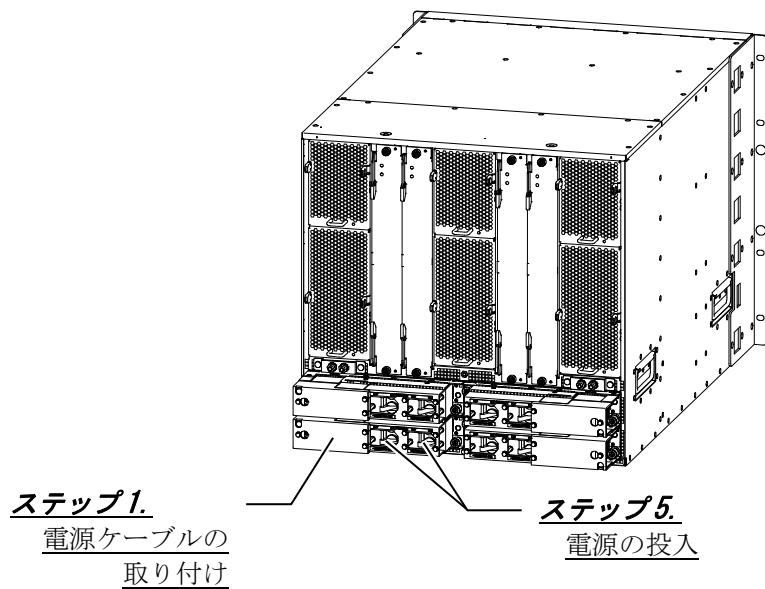
図2-8 AX8616R（背面）概略図
