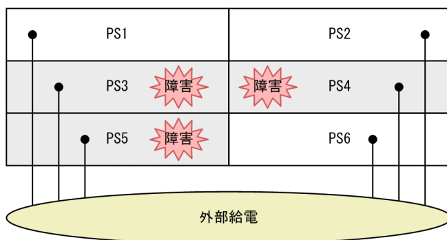
図 14-6 AX8600S の電源ユニット冗長の構成例
