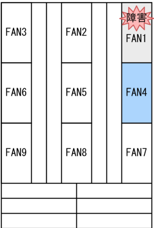
図 12-45 ファンユニット故障時の動作例（AX8632S で FAN1 のファンユニットが故障した場合）
