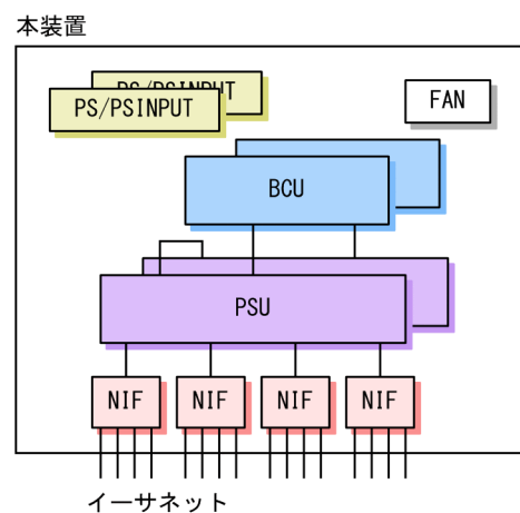
図 2-7 AX8616S および AX8632S のハードウェアの構成
