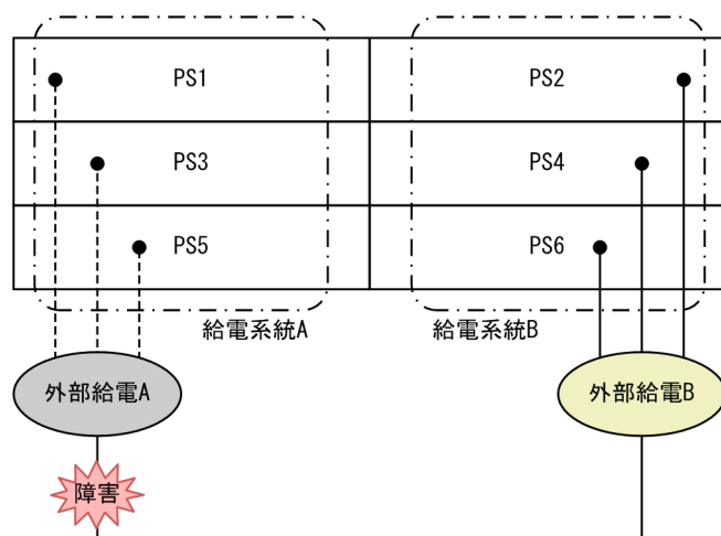
図 14-8 AX8600S の給電系統冗長の構成例
