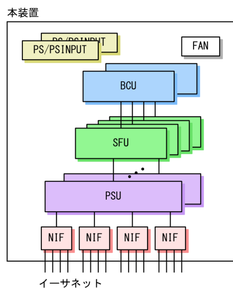
図 2-7 AX8616S および AX8632S のハードウェアの構成
