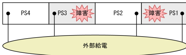
図 14-7 AX8300S の電源ユニット冗長の構成例
