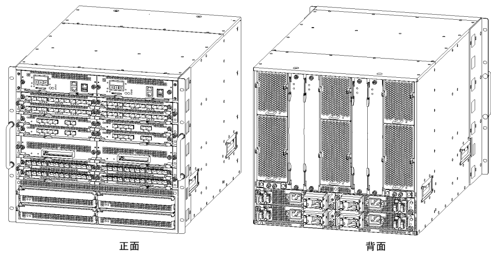
図 2-2 AX8616S モデル
