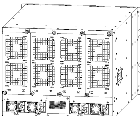
背面
