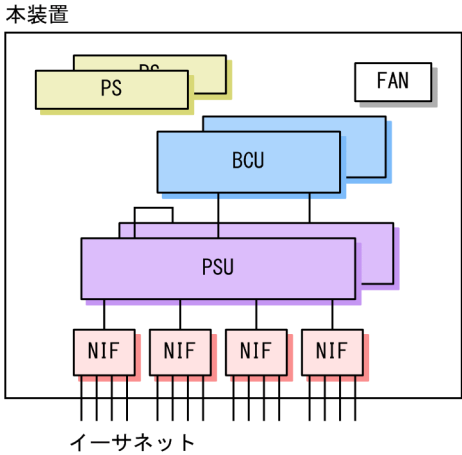
図 2-8 AX8308S のハードウェアの構成
