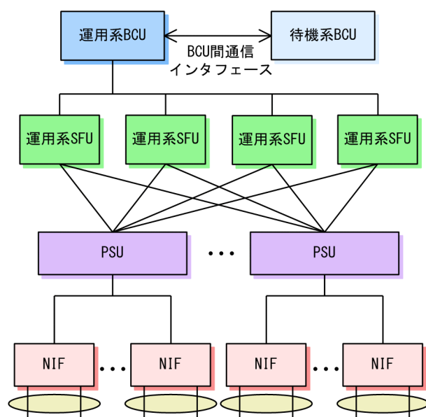
図 14-2 BCU-SFU-PSU-NIF 間の冗長構成でのインタフェース
