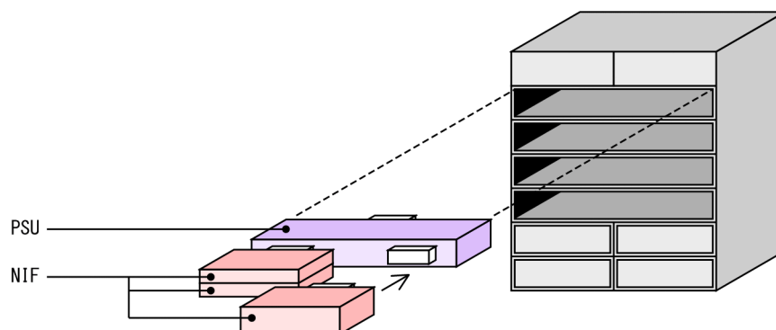
図 3-1 PSU と NIF の搭載イメージ
