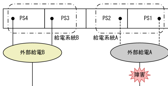
図 14-9 AX8300S の給電系統冗長の構成例
