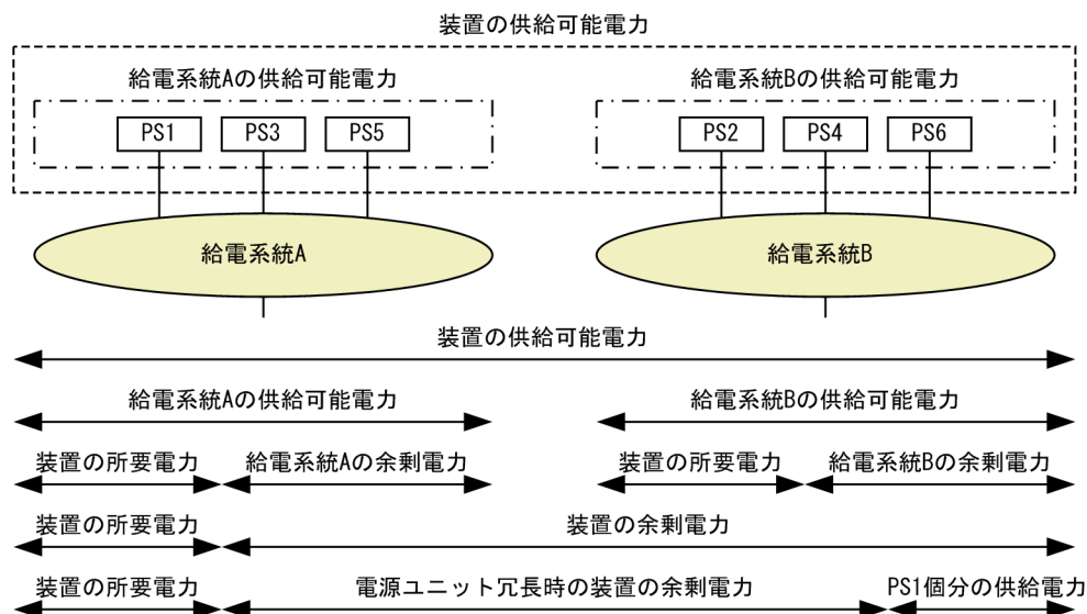
図 14-10 供給電力の管理 (PS を 6 個搭載した例)
