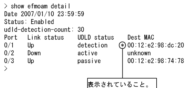
図 6-107 IEEE802.3ah/OAM の運用状態表示
