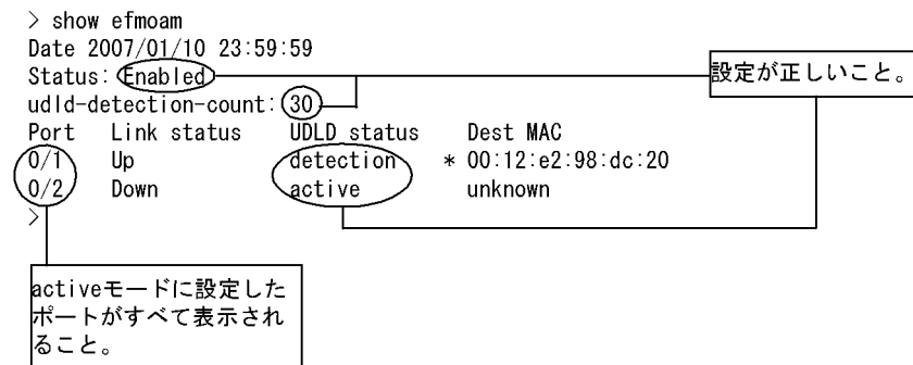
図 6-106 IEEE802.3ah/OAM の設定状態表示
