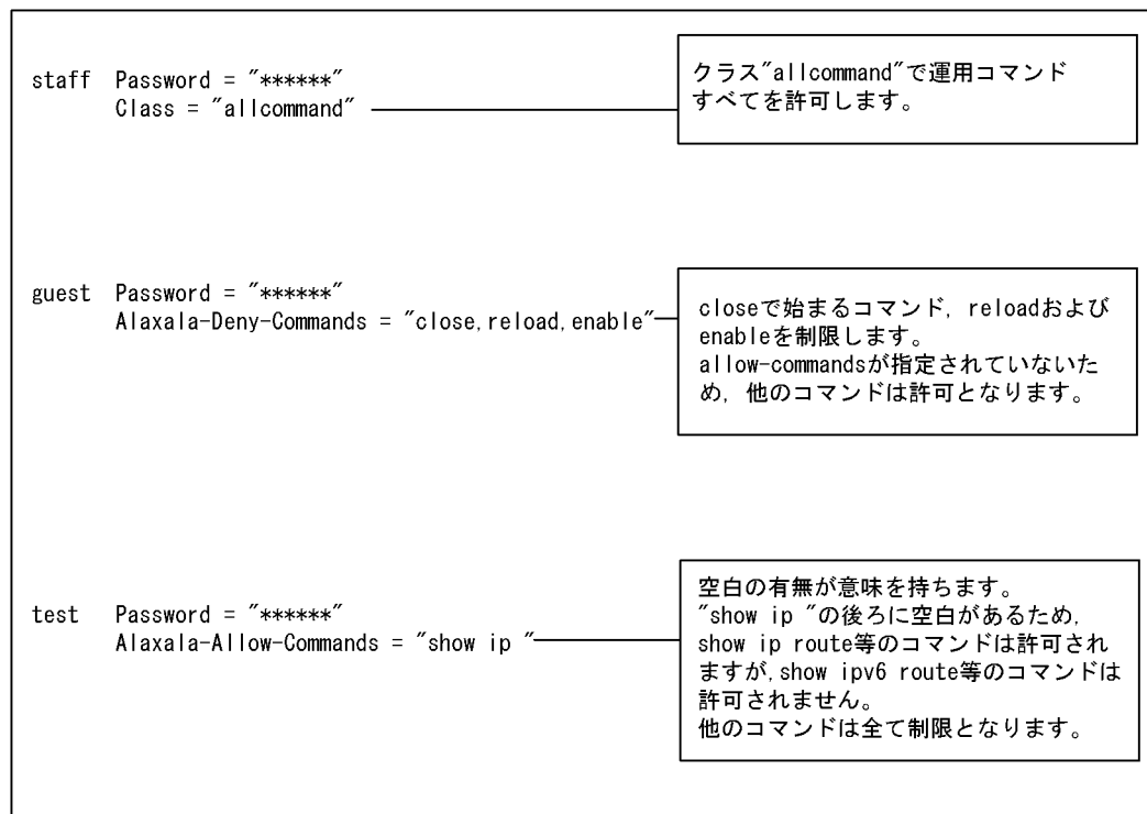
図 5-9 RADIUS サーバ設定例
