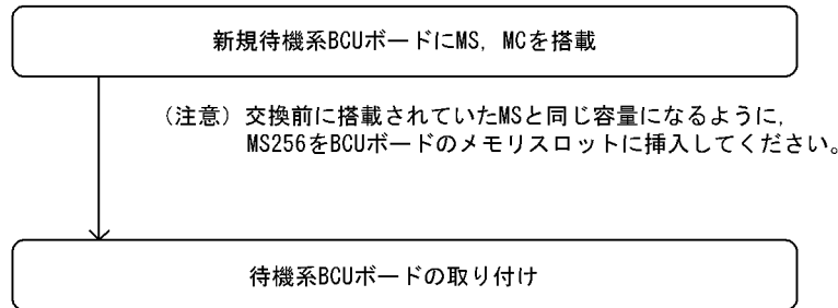
図 9-25 待機系 BCU 取り付け手順
