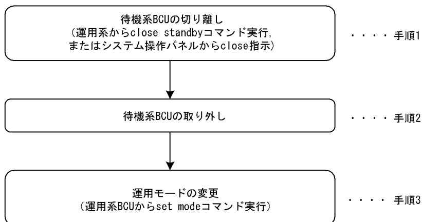
図 9-38 待機系 BCU 取り外し手順
