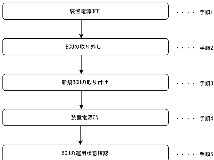
図 9-32 待機系 BCU 交換手順
