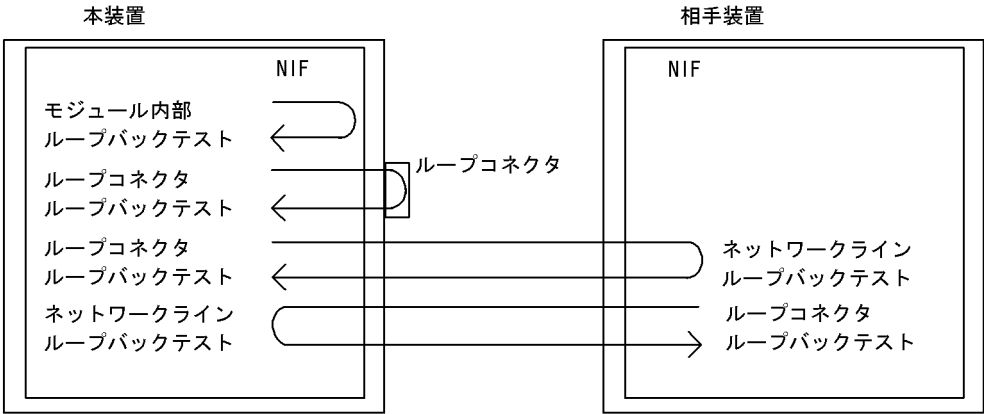
図 9-62 回線テストのテスト種別によるフレームの折り返し位置
