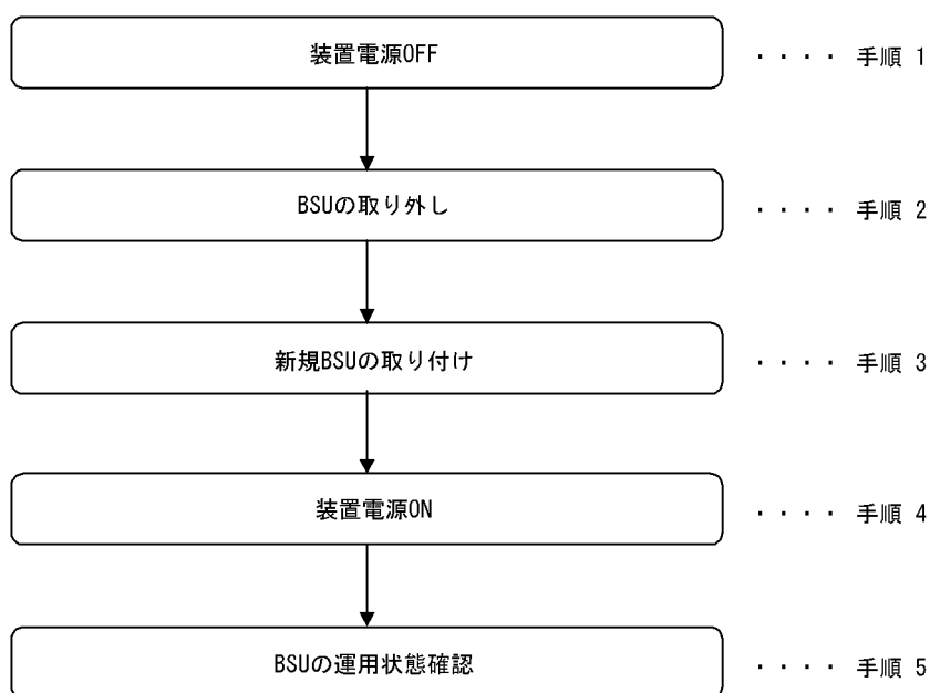
図 9-36 待機系 BCU 交換手順
