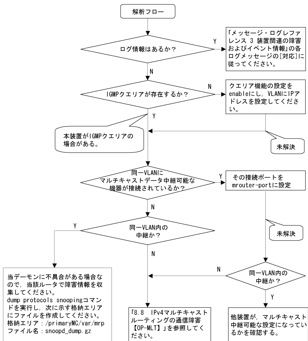
図 8-7 解析フロー
