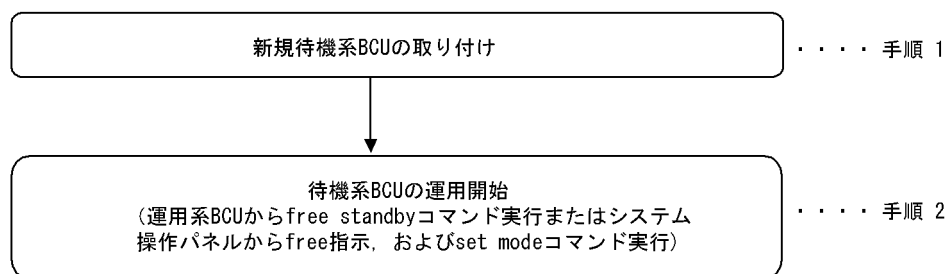
図 9-43 待機系 BCU 増設手順
