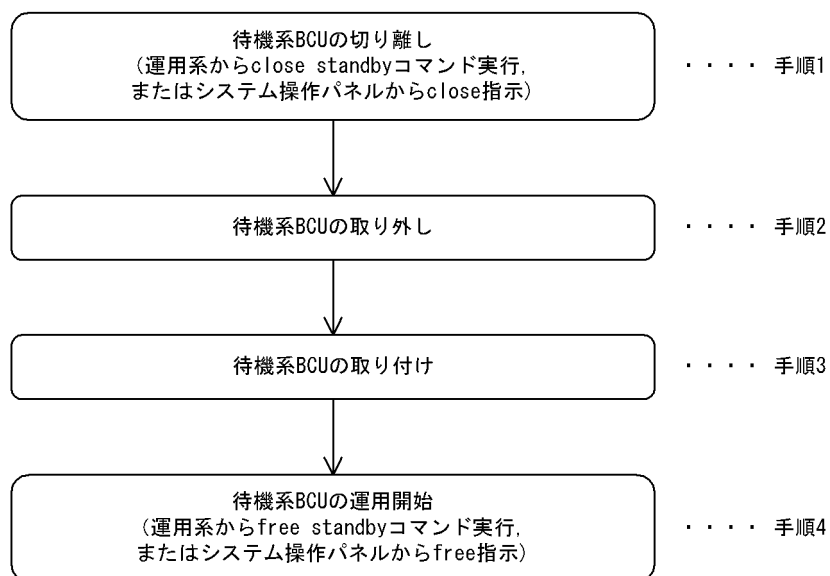
図 9-22 待機系 BCU 交換手順
