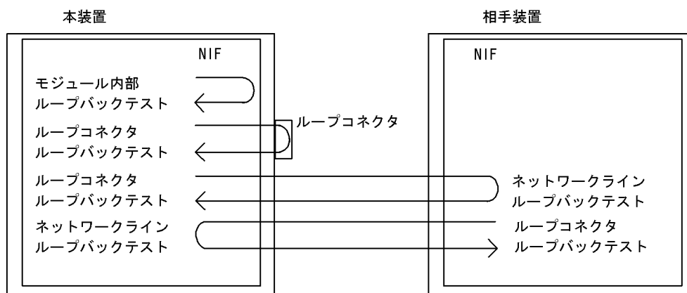
図 9-64 回線テストのテスト種別によるフレームの折り返し位置
