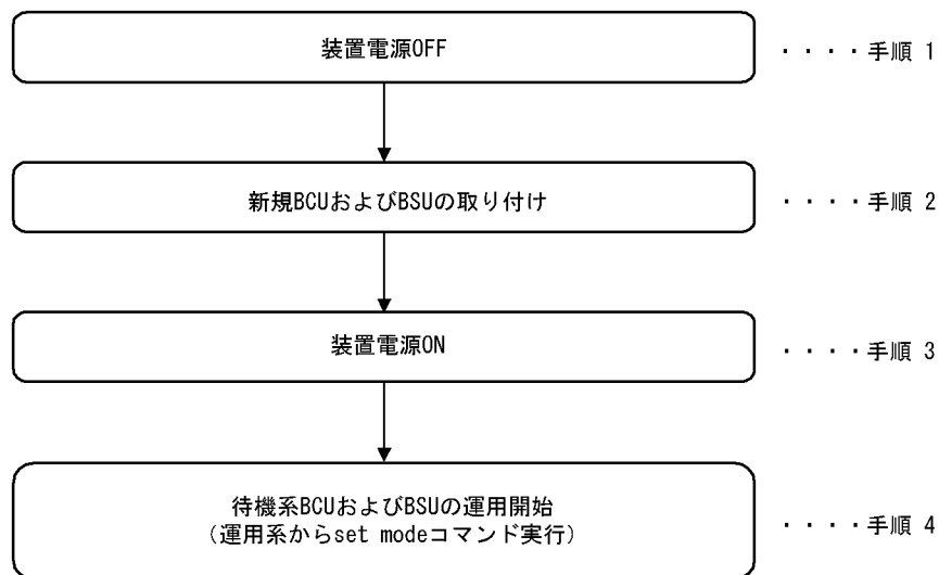
図 9-56 待機系 BCU 交換手順
