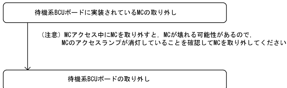
図 9-24 待機系 BCU 取り外し手順
