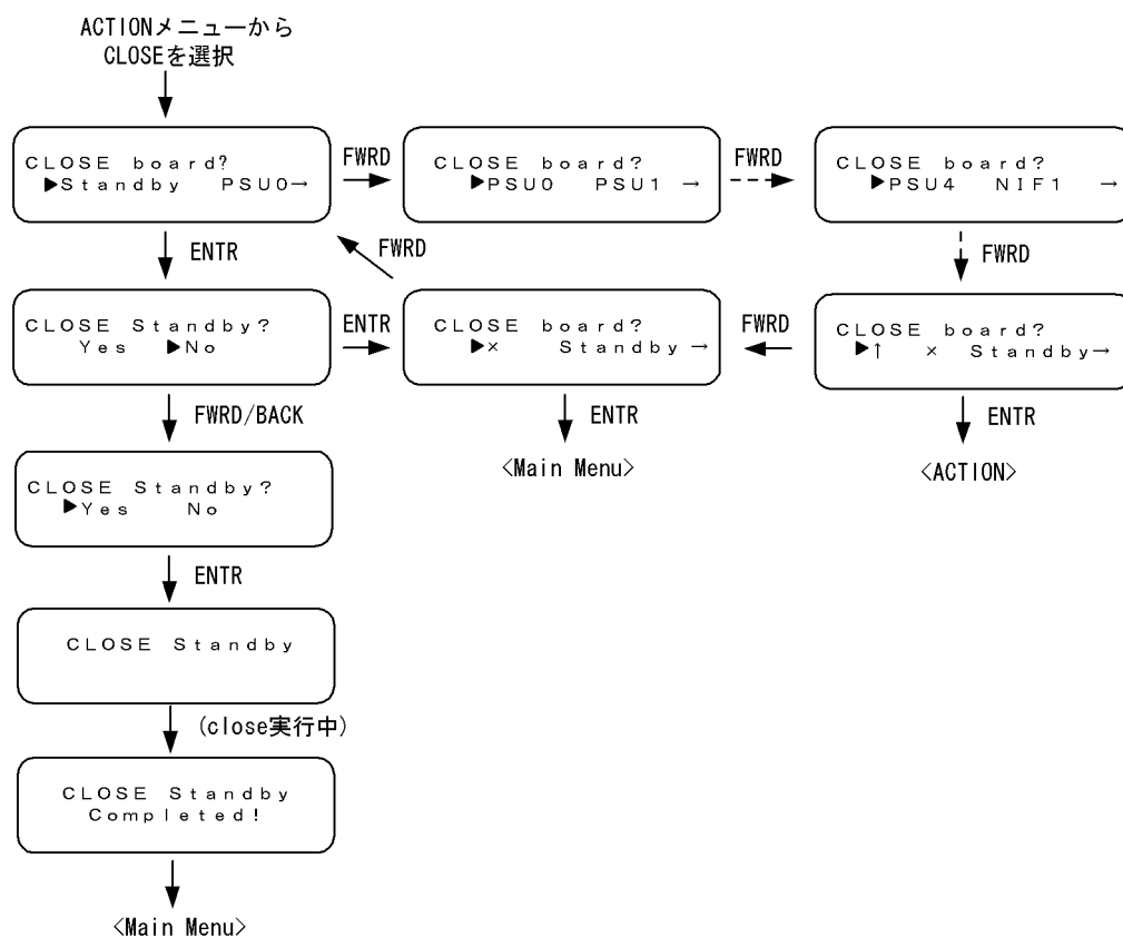
図 4-10 close の操作手順
