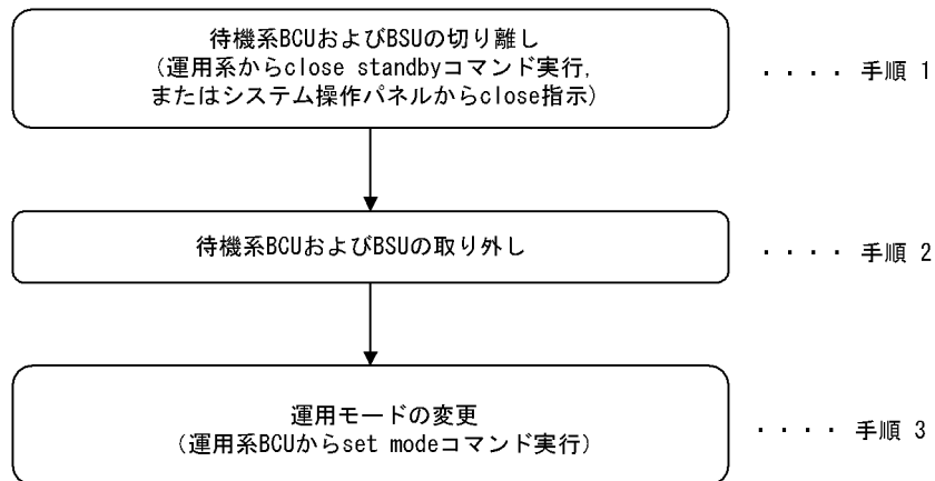
図 9-50 待機系 BCU,BSU 取り外し手順
