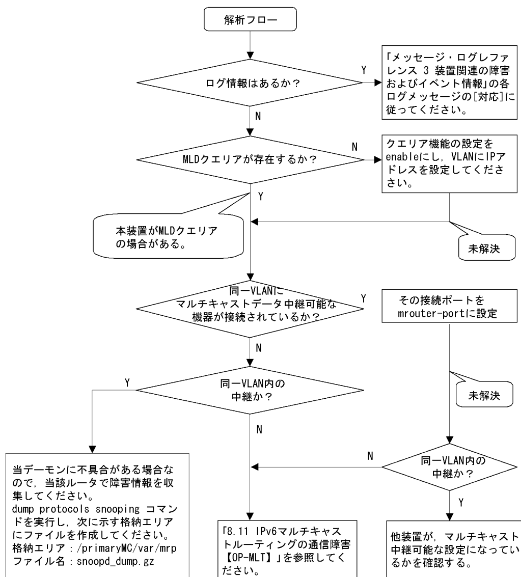
図 8-8 解析フロー
