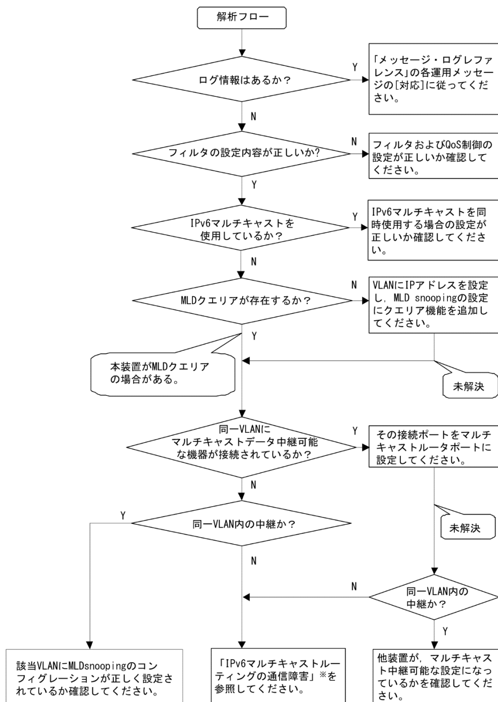
図 4-3 解析フロー
