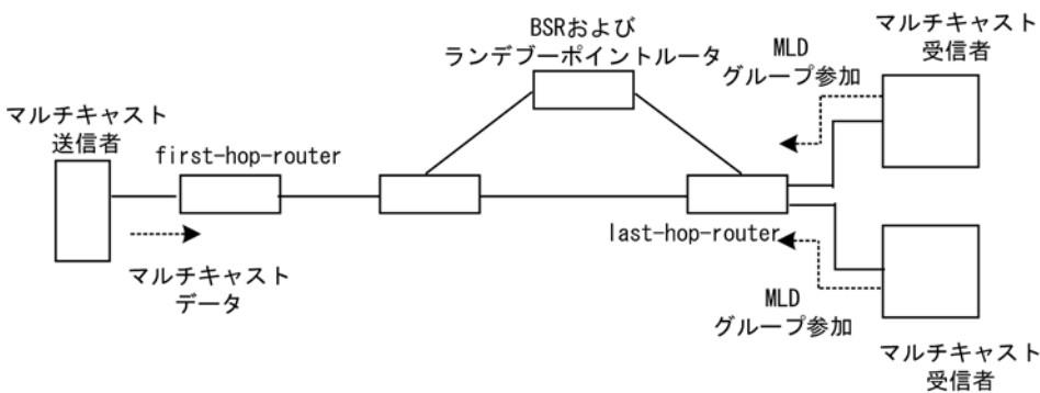
図 7-11 IPv6 PIM-SM ネットワーク例
