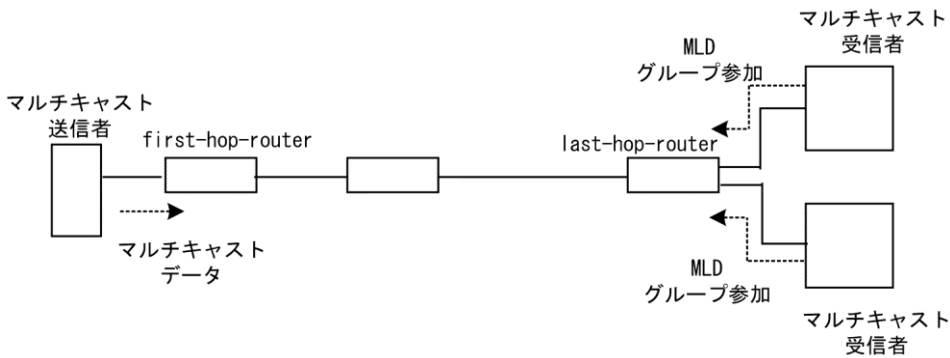
図 7-12 IPv6 PIM-SSM ネットワーク例
