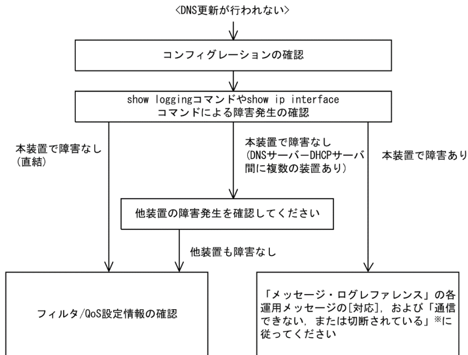
図 7-4 DNS 連携時の DHCP サーバ障害解析手順
