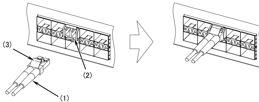
図2-11 光ファイバケーブル (LC2 芯コネクタ) の取り付け
