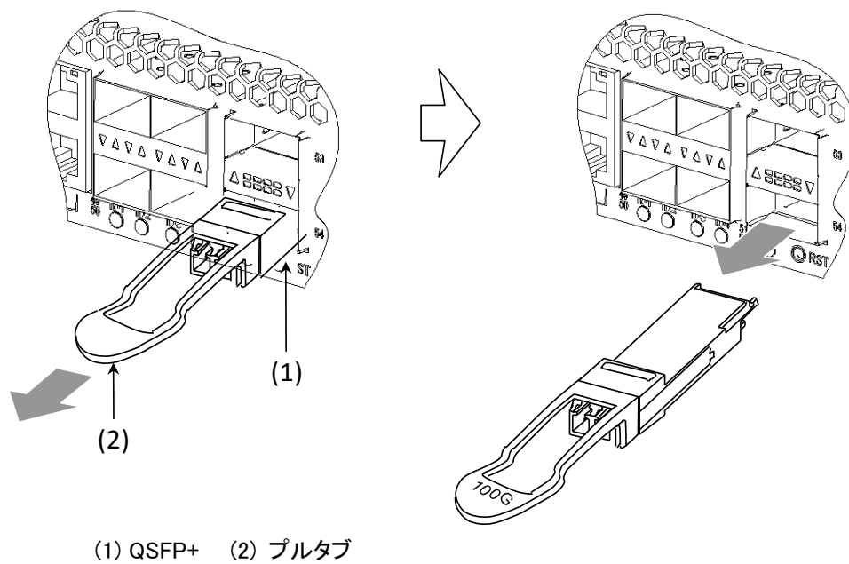
図2-7 QSFP+の取り外し（プルタブタイプの場合）
