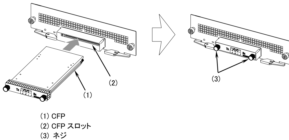
図2-8 CFP の取り付け
