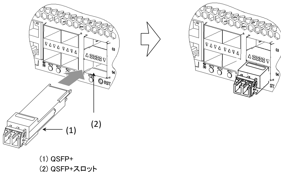
図2-5 QSFP+の取り付け
