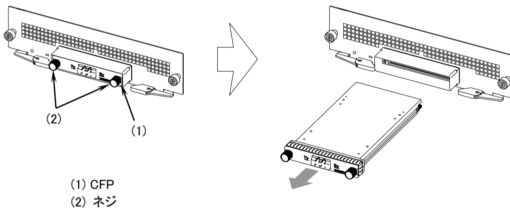
図2-9 CFP の取り外し
