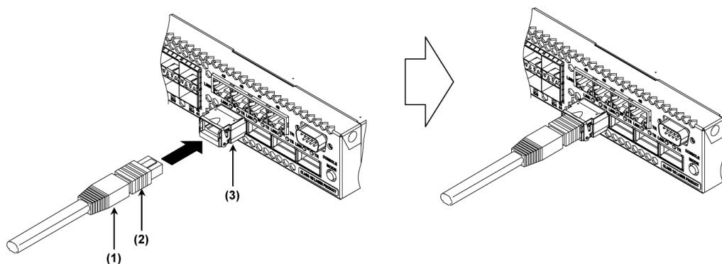
図2-13 光ファイバケーブル（MPO コネクタ）の取り付け
