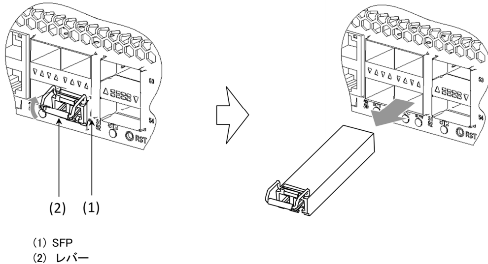
図4-13 SFP の取り外し（下側のポート）
