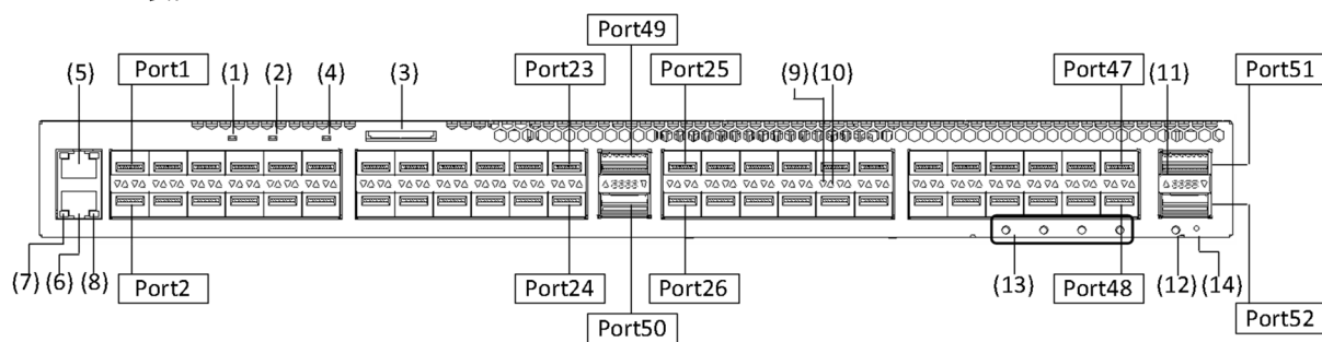
図1-24 正面パネルレイアウト
