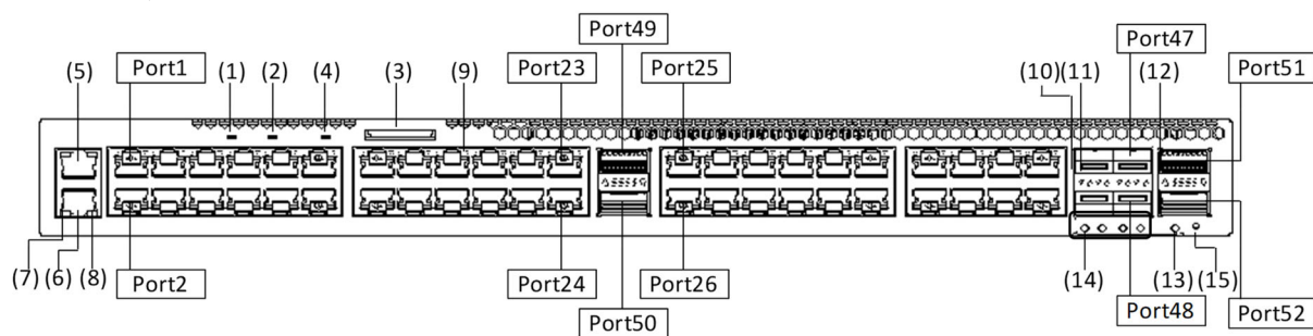
図1-18 正面パネルレイアウト
