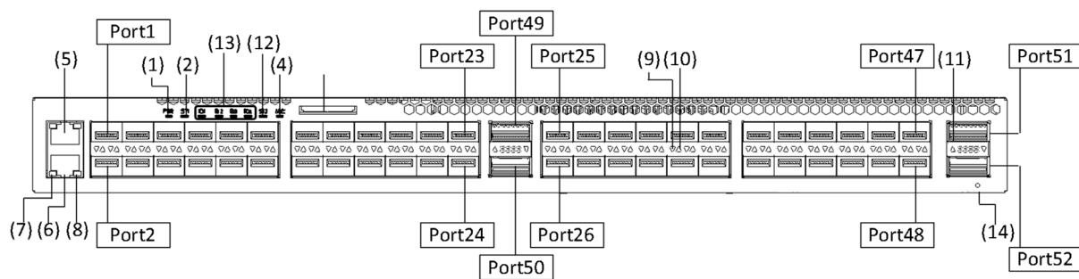
図1-21 正面パネルレイアウト
