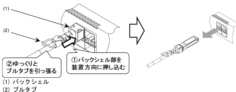
図4-24 ダイレクトアタッチケーブルの取り外し
