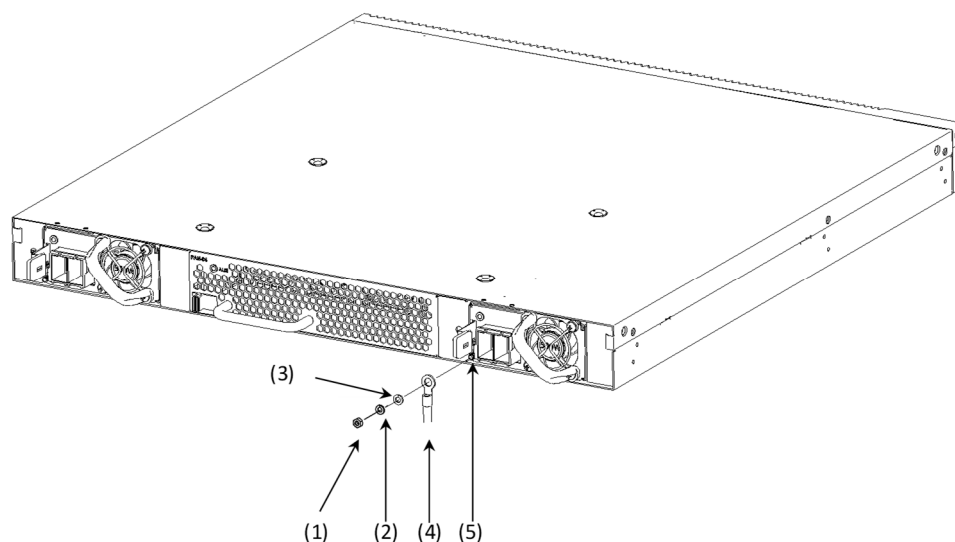
図4-6 接地用ケーブルの取り付け
