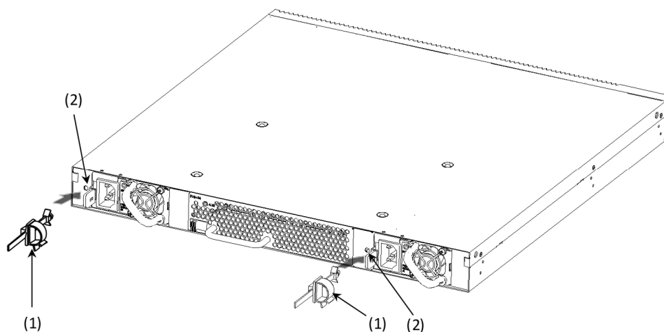
図4-2 ケーブルクランプの取り付け
