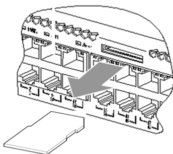
図4-17 ダミーカードの取り出し
