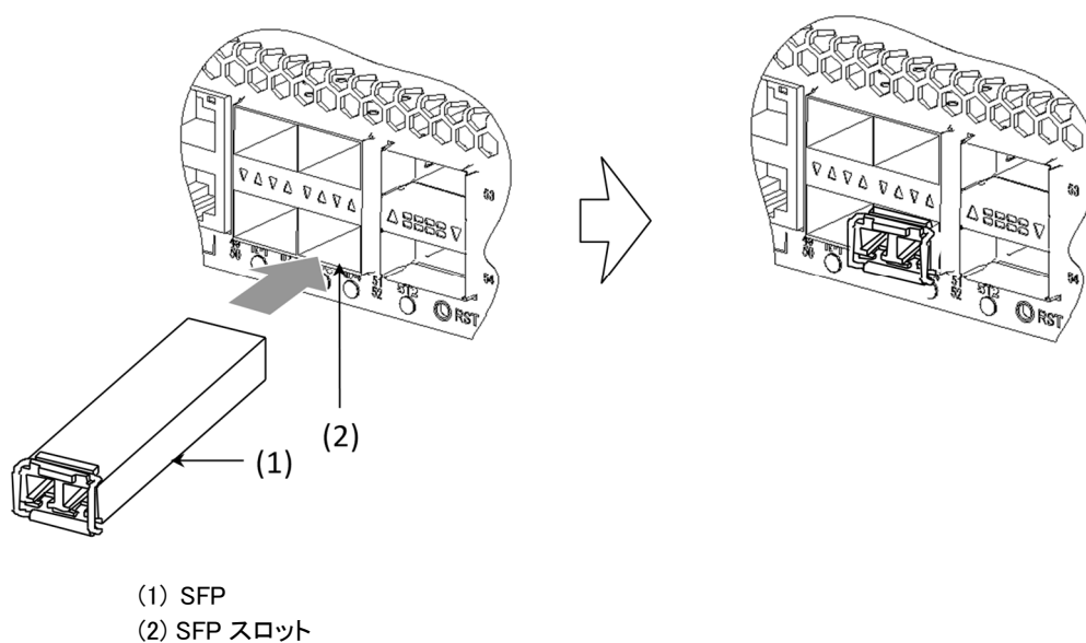
図4-12 SFP の取り付け（下側のポート）
