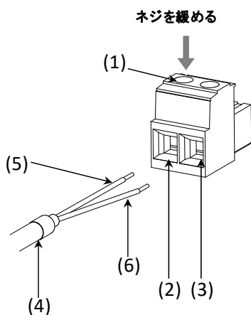
図4-7 DC 電源ケーブルの取り付け 1
