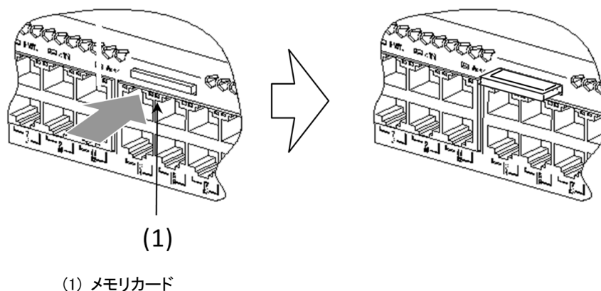
図4-13 メモ리카ードの取り外し方
