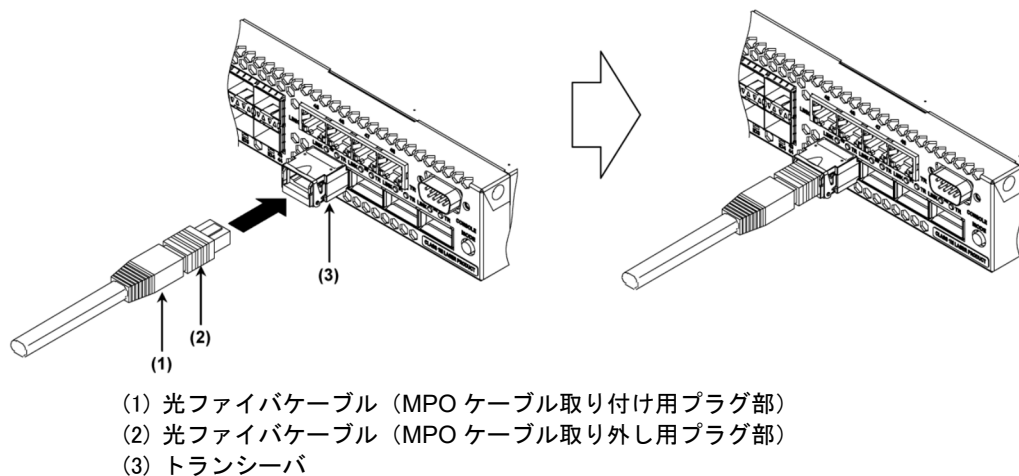
図4-22 光ファイバケーブル（MPO コネクタ）の取り付け
