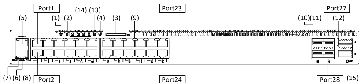
図1-3 正面パネルレイアウト
