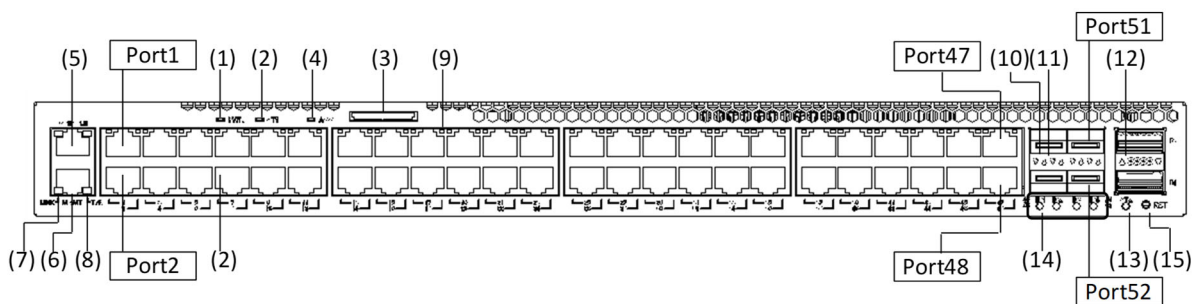
図1-9 正面パネルレイアウト
