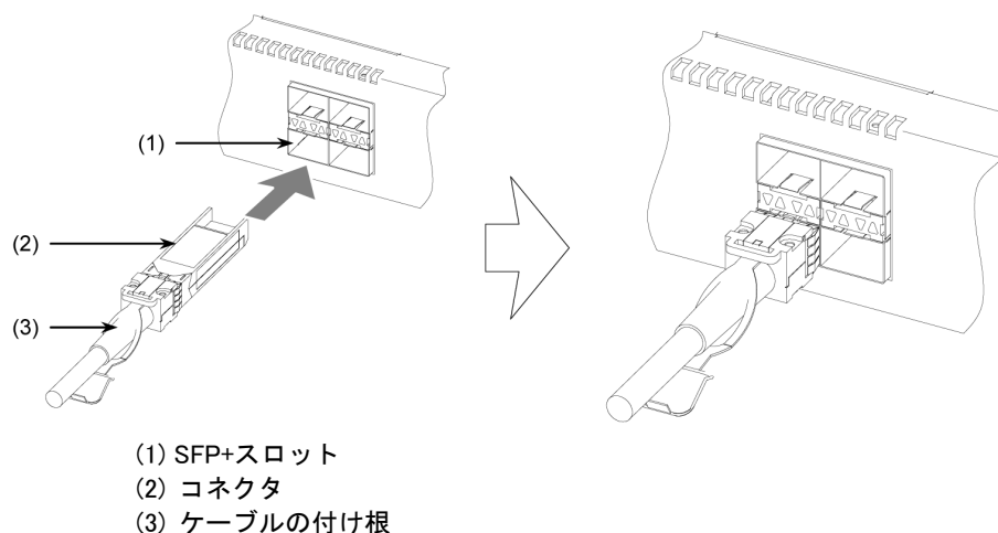
図4-23 ダイレクトアタッチケーブルの取り付け
