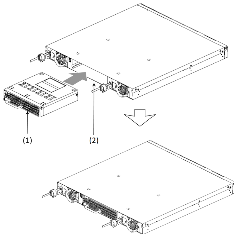
図5-5 ファンユニットの取り付け
