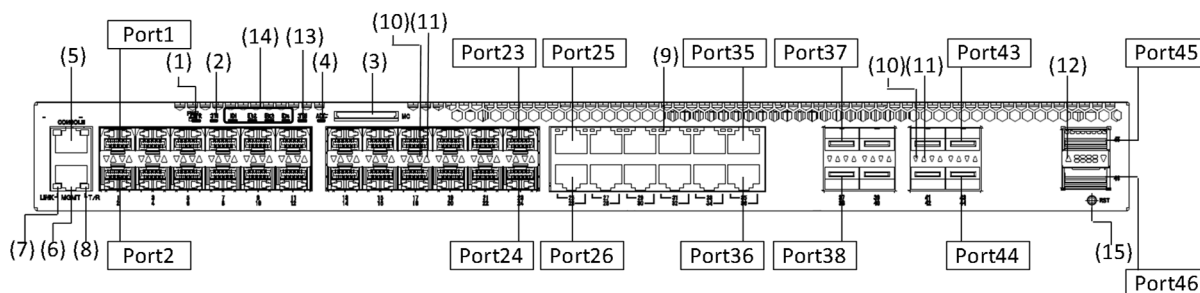
図1-12 正面パネルレイアウト
