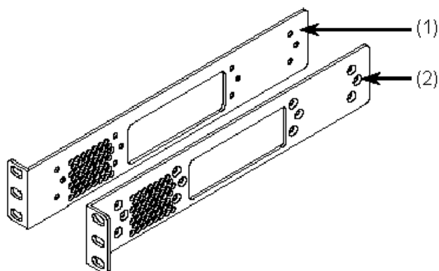
図1-25 ラック固定金具
