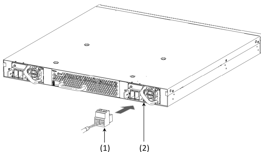
図4-9 DC 電源コネクタの取り付け
