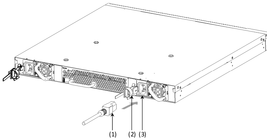
図4-3 電源ケーブルの取り付け
