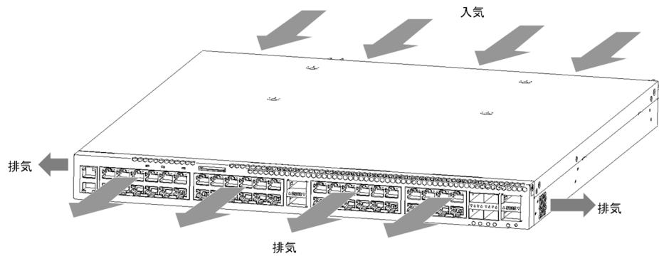
図2-10 AAX3660S-24X4QW, AX3660S-48X4QW のエアフロー（背面吸気・前面排気構成時）
