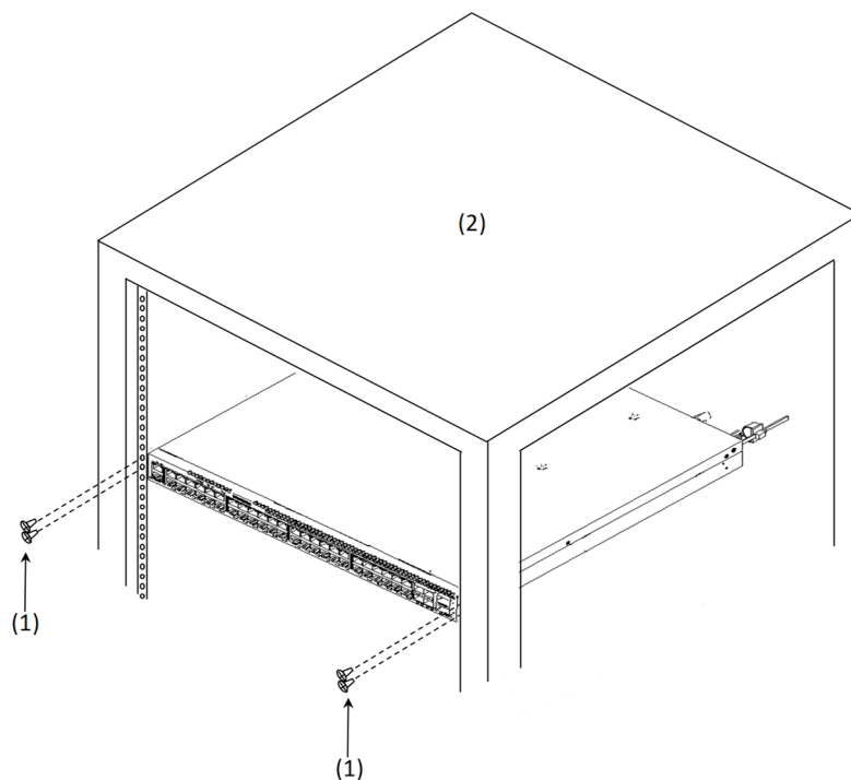
図4-1 ラックへの搭載
