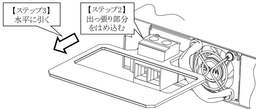
図4-11 DC 電源コネクタの取り外し
