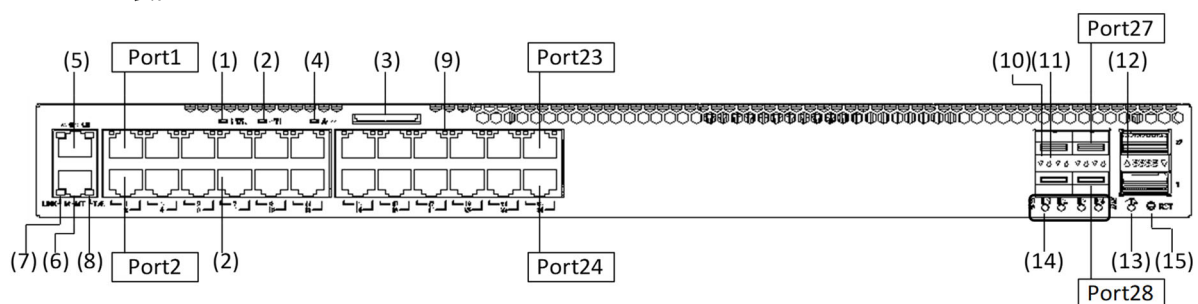
図1-6 正面パネルレイアウト
