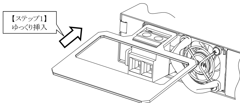
図4-10 DC 電源コネクタ引抜き工具の挿入
