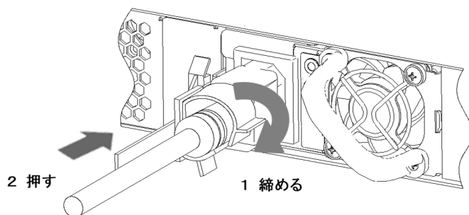
図4-4 電源ケーブルのクランプ
