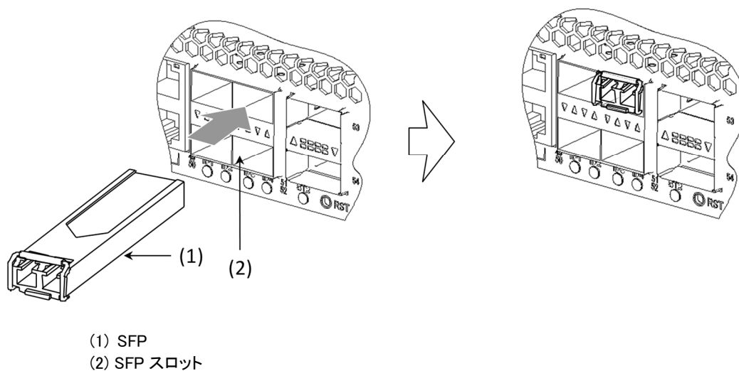
図4-18 SFP の取り付け（上側のポート）
