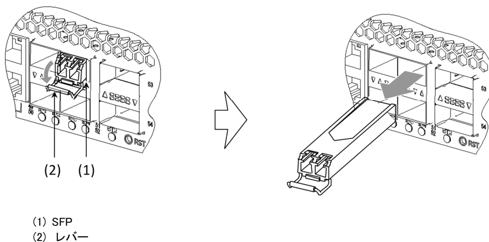
図4-12 SFP の取り外し（上側のポート）
