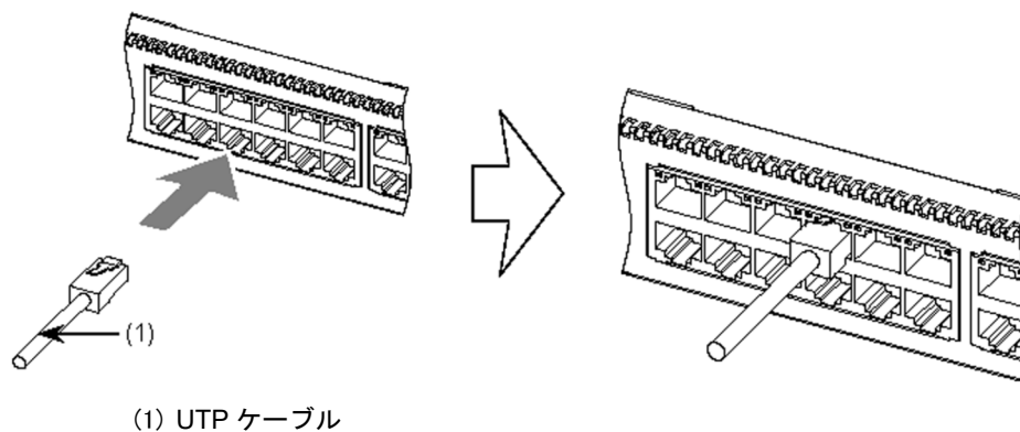
図4-19 UTP ケーブルの取り付け
