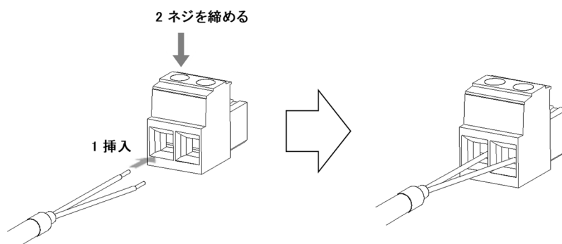
図4-8 DC 電源ケーブルの取り付け 2
