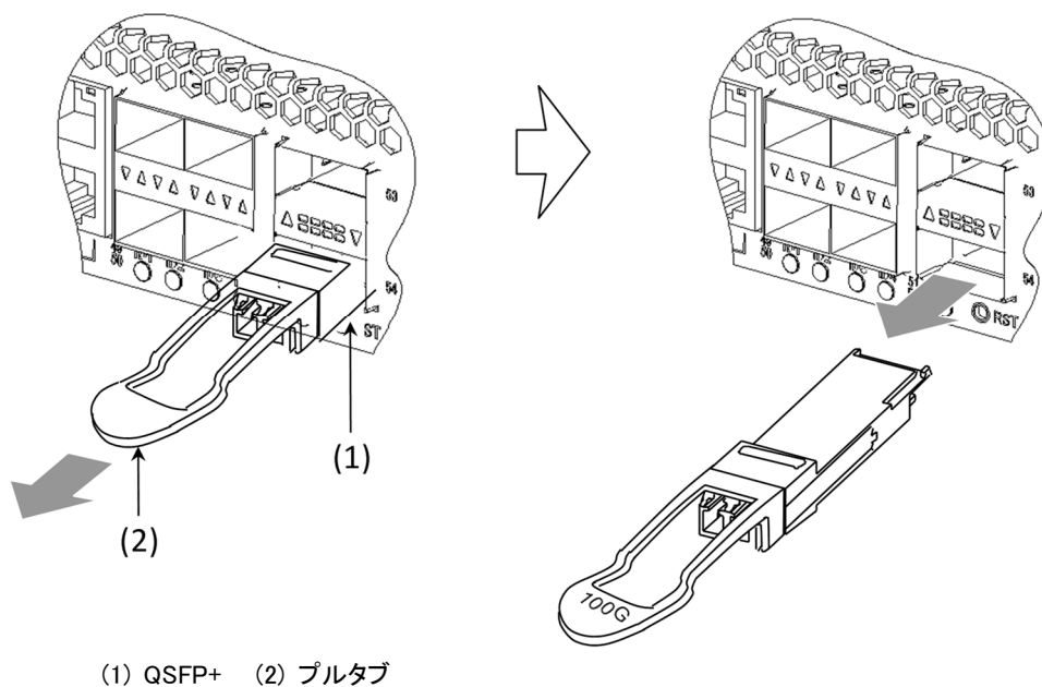
図4-16 QSFP+の取り外し（プルタブタイプの場合）
