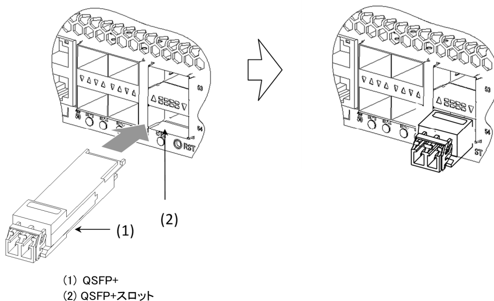
図4-14 QSFP+の取り付け
