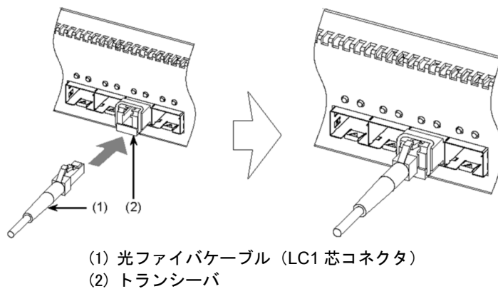
図4-21 光ファイバケーブル（LC1 芯コネクタ）の取り付け
