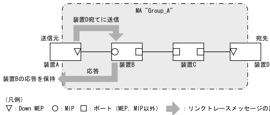
図 21-23 宛先にリンクトレースメッセージを送信
