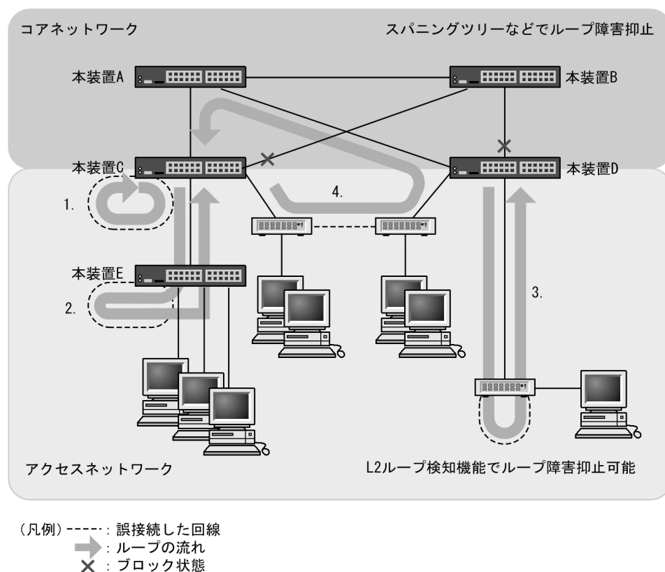
図 20-1 ループ障害の基本パターン
