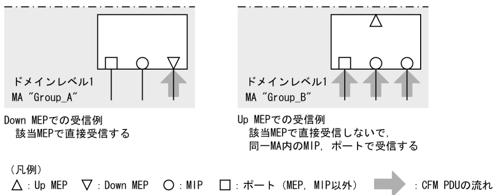
図 21-7 Down MEP, Up MEP での受信
