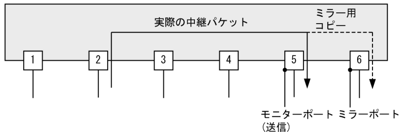
図 27-2 送信フレームのミラーリング
