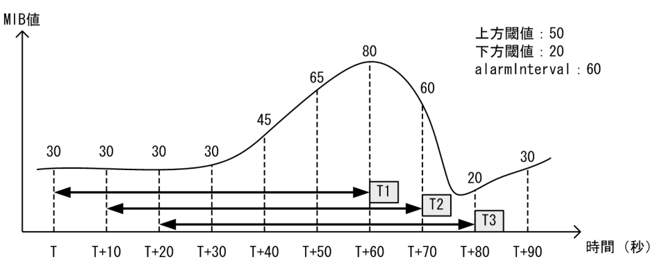
図 22-29 delta 方式による MIB 監視例
