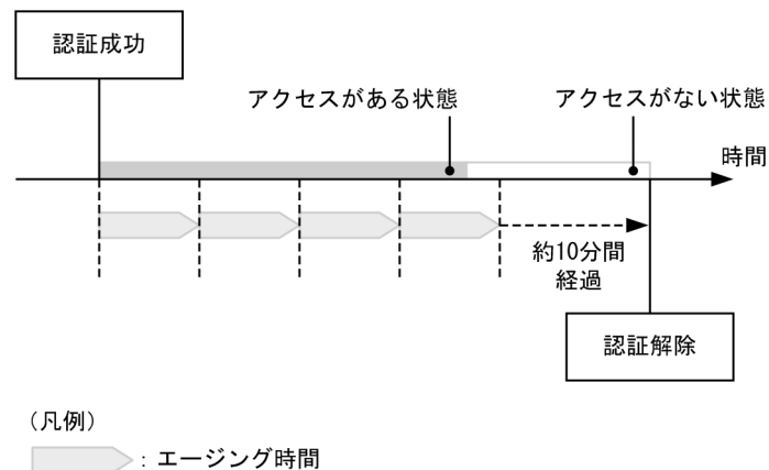
図 8-16 認証済み端末の MAC アドレステーブルエージングによるログアウト
