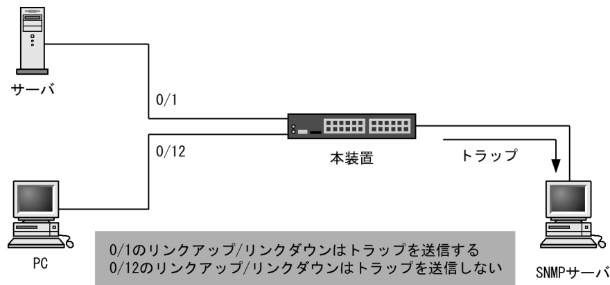
図 22-31 リンクトラップの構成図
