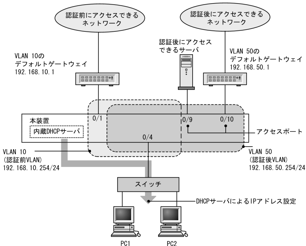
図 9-8 口一カル認証方式+内蔵 DHCP 使用時の構成例
