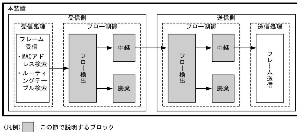
図 1-2 本装置のフィルタの機能ブロック【AX3640S】
