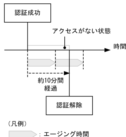
図 8-17 認証成功直後からアクセスがない場合のログアウト
