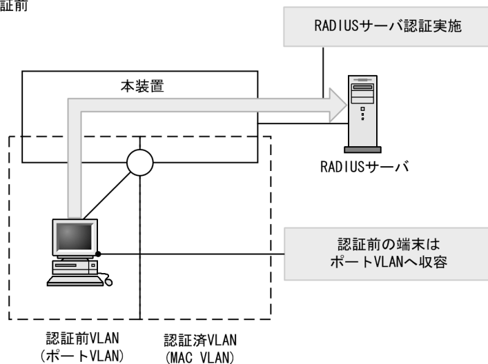
図 6-7 VLAN 単位認証（動的）の動作イメージ
