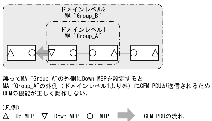
図 21-8 誤って Down MEP を設定した例
