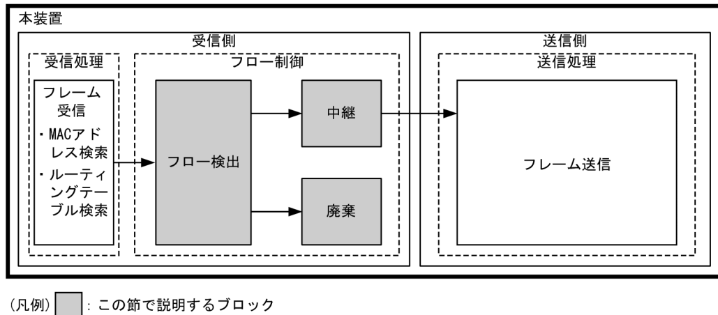
図 1-3 本装置のフィルタの機能ブロック【AX3630S】
