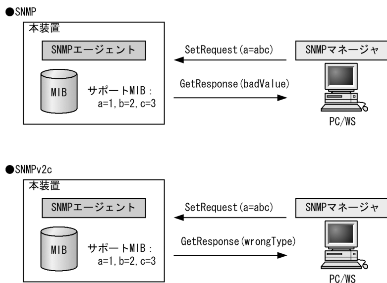
図 22-14 設定値のタイプが正しくない場合の SetRequest オペレーション例
