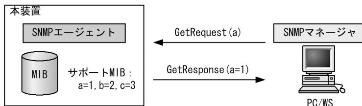
図 22-7 GetRequest オペレーション
