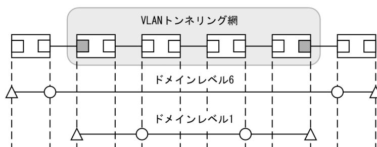
図 21-27 VLAN トネリング網内と VLAN トネリング網外で CFM を使用する例
