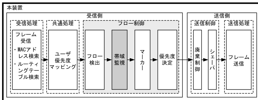
図 3-3 帯域監視の位置づけ
