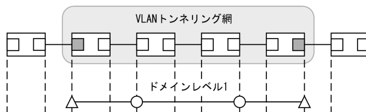
図 21-28 VLAN トネリング網内だけで CFM を使用する例
