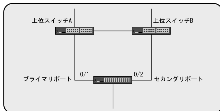
図 17-7 アップリンク・リダンダントの設定例
