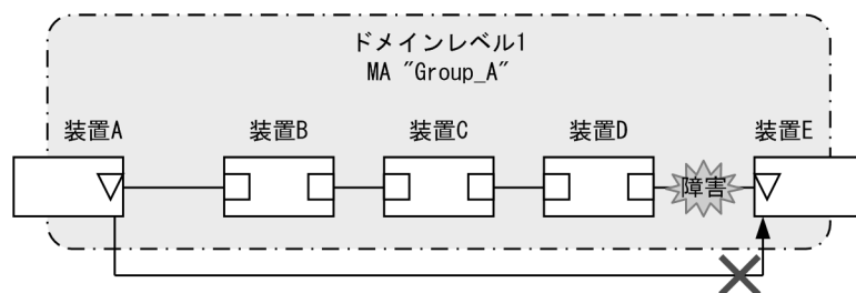
図 21-10 ドメイン内に MIP が設定されていない構成の例
