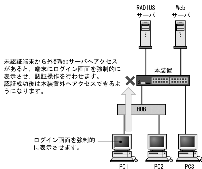
図 8-11 URL リダイレクト機能
