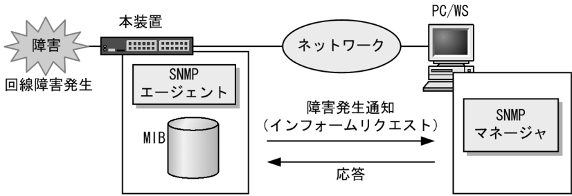
図 22-27 インフォームの例
