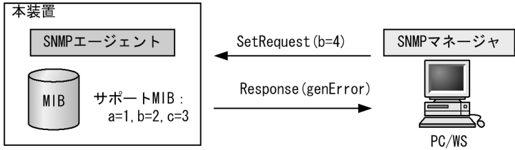
図 22-23 装置の状態によって設定できない場合の SetRequest オペレーション
