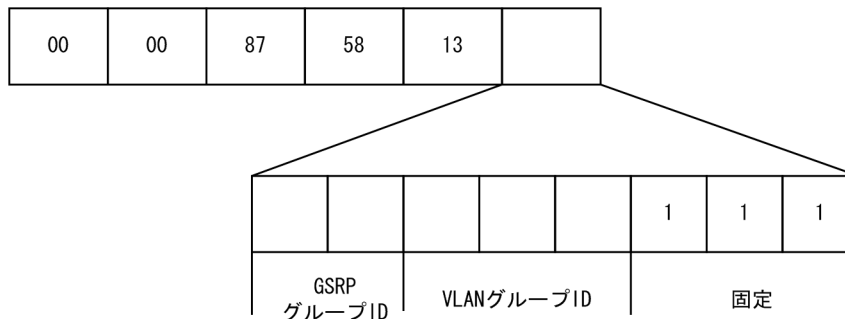
図 14-9 GSRP レイヤ 3 冗長切替機能の仮想 MAC アドレスの生成方法 (VLAN グループ ID が 8 以下)
