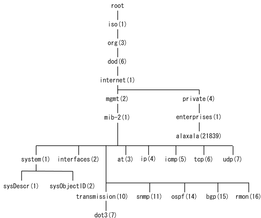
図 22-6 MIB ツリーの構造例
