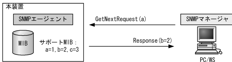
図 22-18 GetNextRequest オペレーション
