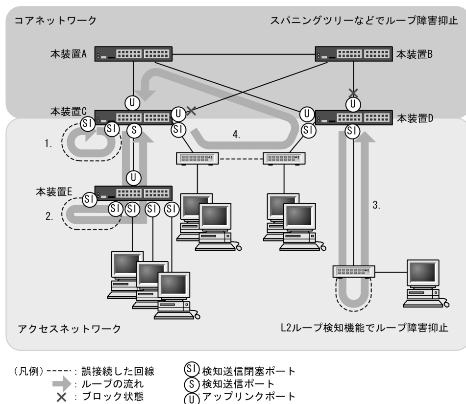
図 20-2 L2 ループ検知機能を適用したネットワーク構成
