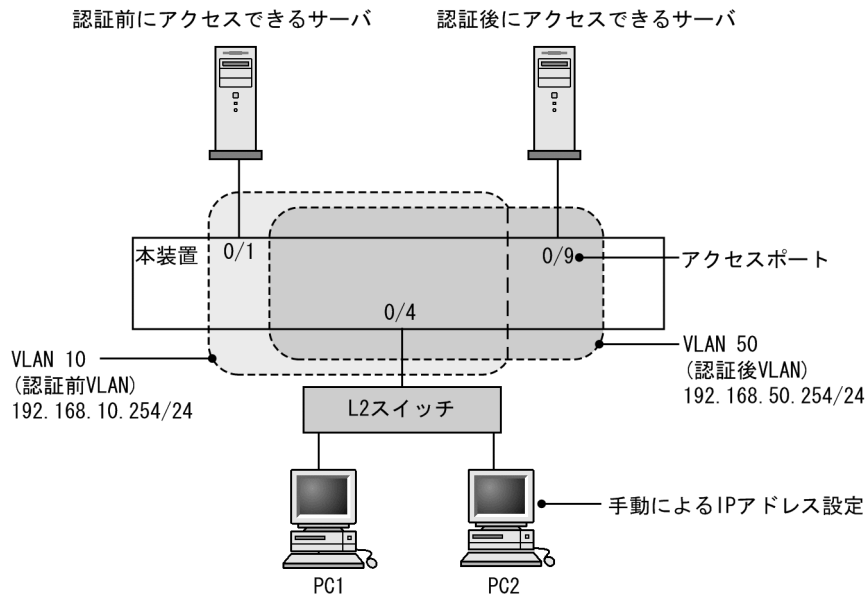
図 9-7 ローカル認証方式の構成例
