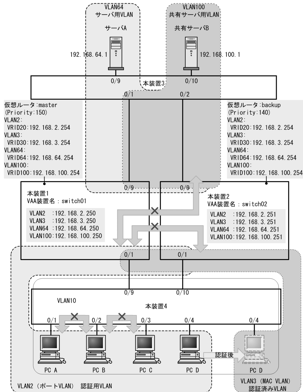
図 12-7 認証 VLAN 冗長構成
