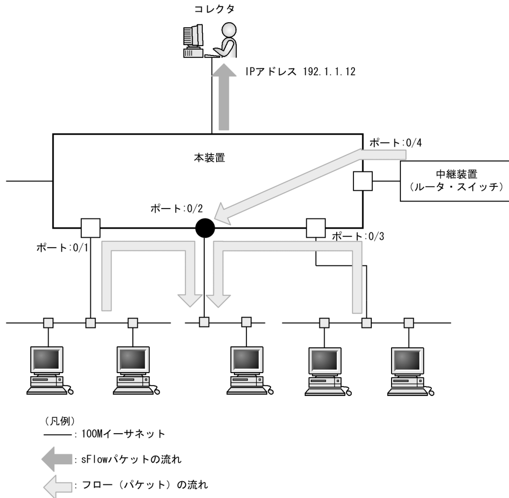
図 24-8 ポート 0/2 の送信パケットをモニタする設定例
