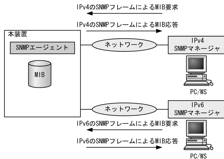
図 22-4 IPv4/IPv6 SNMP マネージャからの MIB 要求と応答の例
