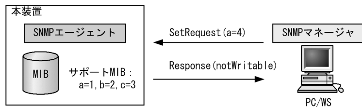
図 22-21 MIB 変数が読み出し専用の場合の SetRequest オペレーション
