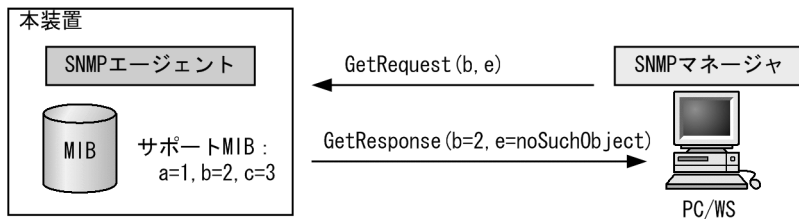
図 22-8 GetRequest オペレーション (SNMPv2C)
