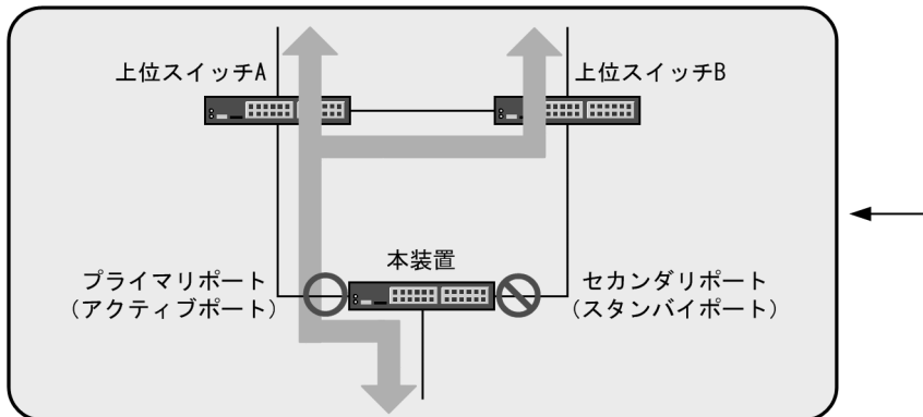
図 17-2 アップリンク・リダundantの動作概要
