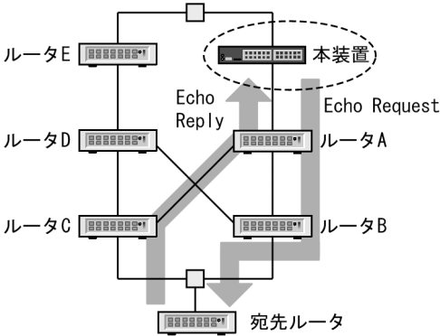
図 16-12 自装置配下ではないネットワーク上のインタフェース不一致
