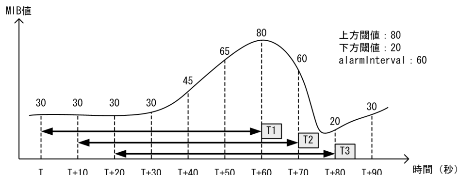
図 22-30 absolute 方式による MIB 監視例
