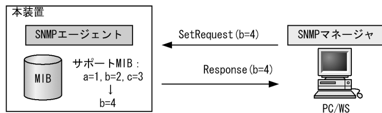
図 22-20 SetRequest オペレーション
