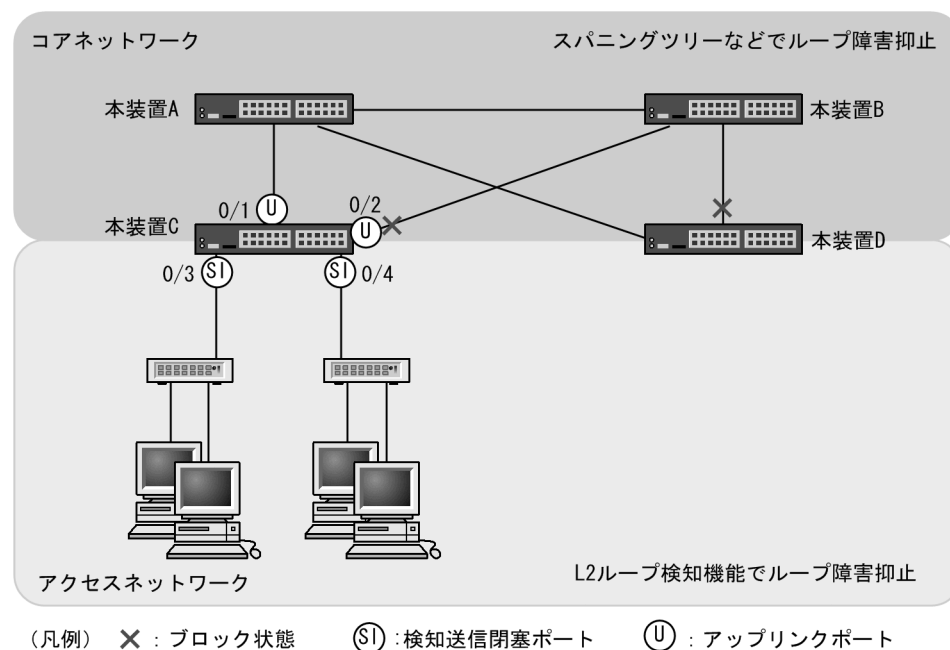
図 20-5 L2 ループ検知の設定例
