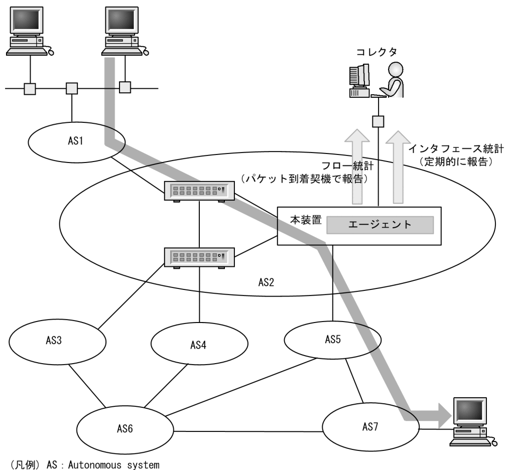
図 24-1 sFlow 統計のネットワーク構成例
