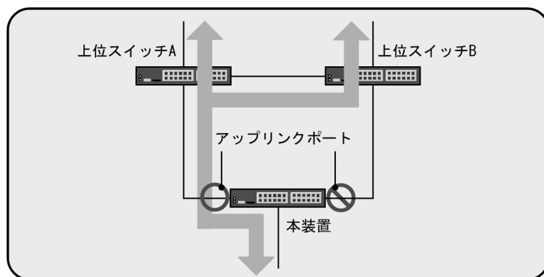
図 17-1 アップリンク・リダンダントの基本構成
