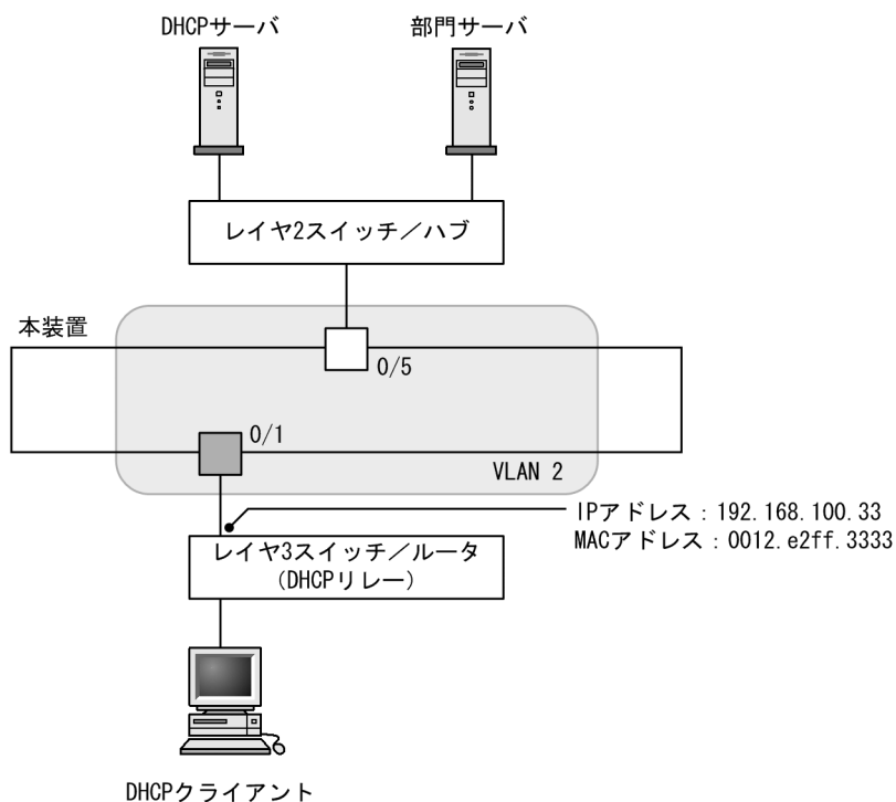
図 13-12 本装置の配下に DHCP リレーを接続した場合の構成例
