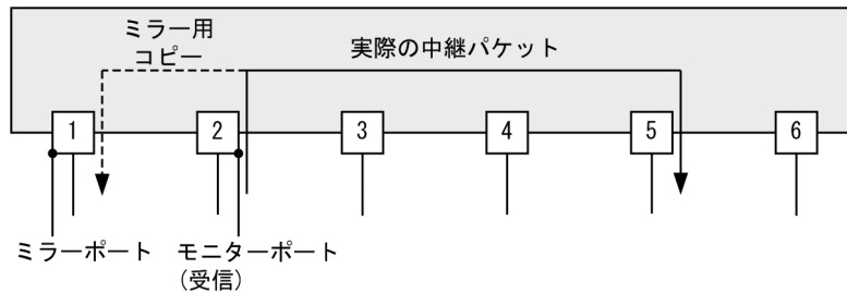
図 27-1 受信フレームのミラーリング
