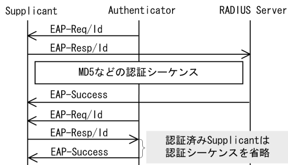
図 6-10 shortcut, disable, full, auto の EAP-Request/Identity のシーケンス
