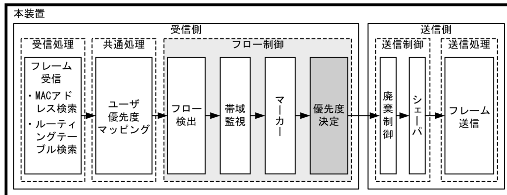
図 3-17 優先度決定の位置づけ
