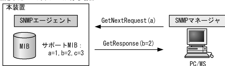
図 22-9 GetNextRequest オペレーション
