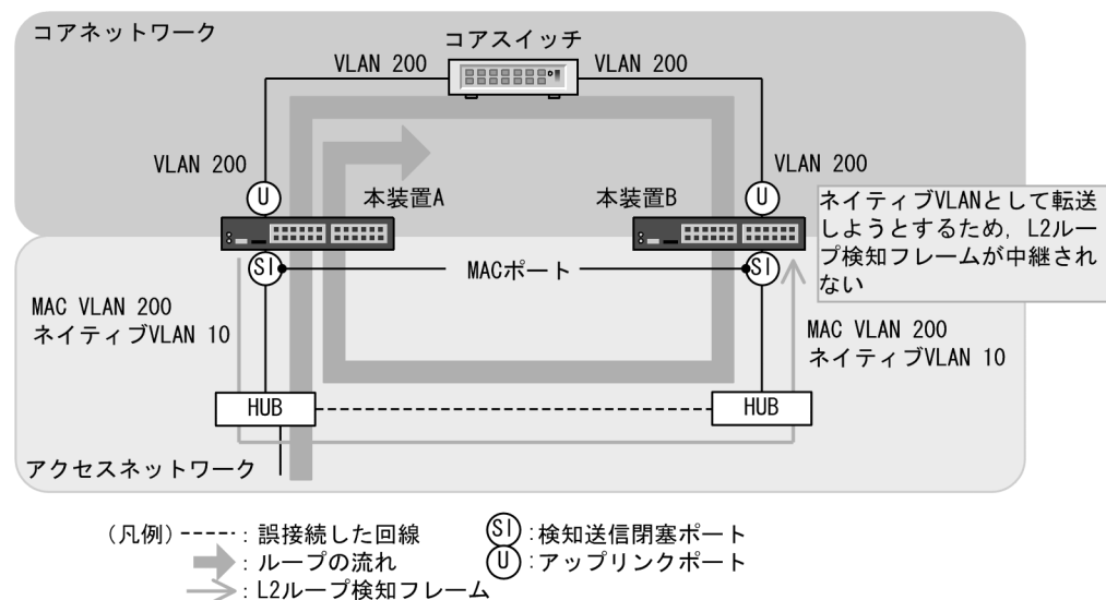
図 20-3 ループ検知の制限となる構成
