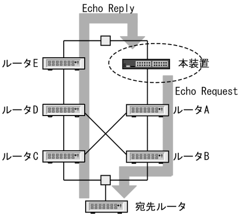
図 16-11 送受信インタフェースが一致しない場合
