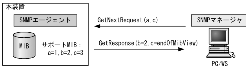
図 22-10 GetNextRequest オペレーション (SNMPv2C)
