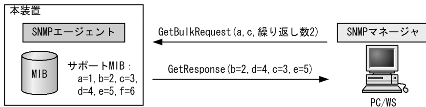
図 22-11 GetBulkRequest オペレーション
