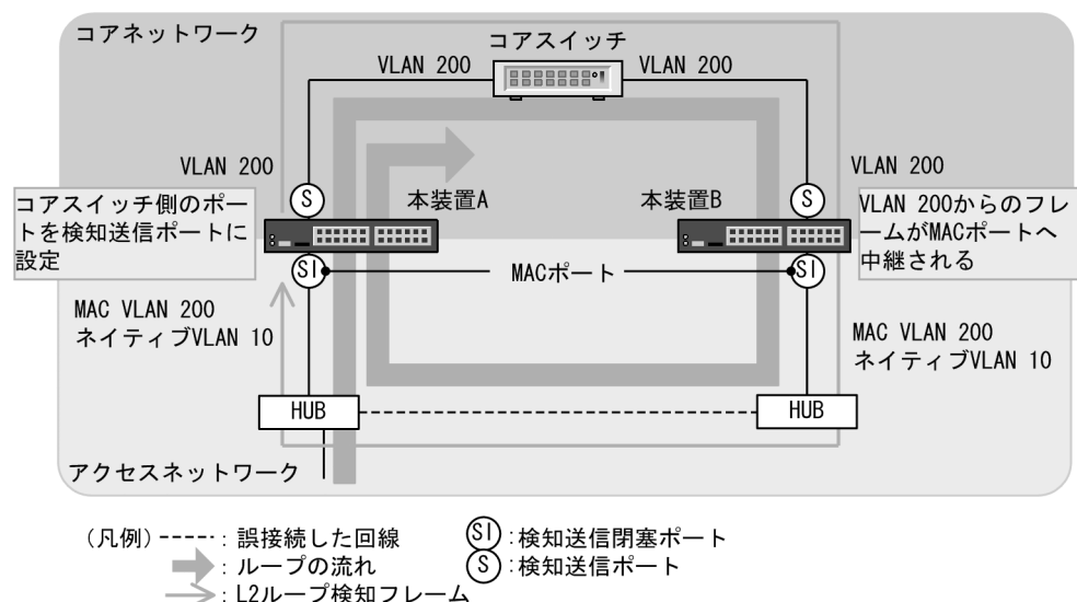
図 20-4 ループ検知可能な構成
