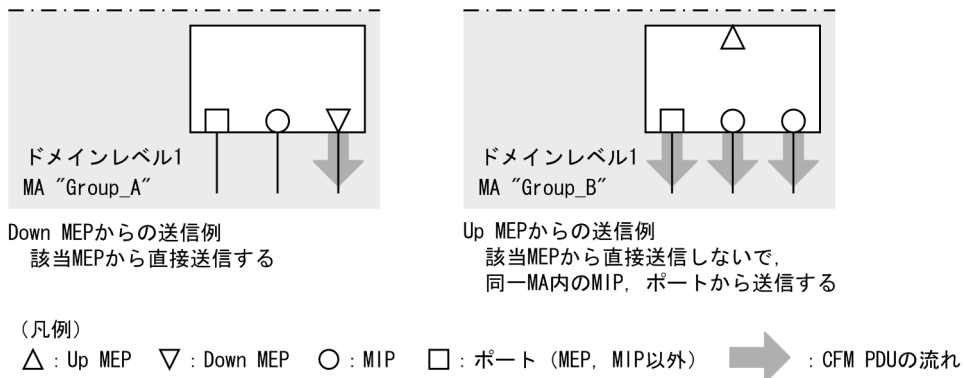
図 21-6 Down MEP, Up MEP からの送信
