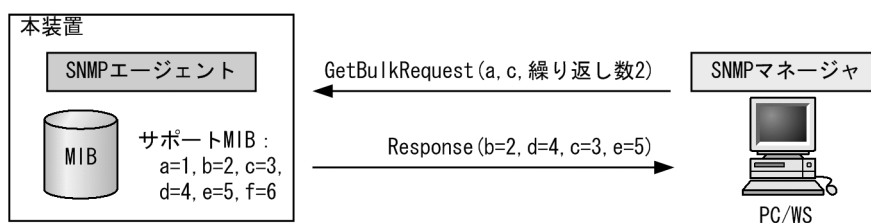
図 22-19 GetBulkRequest オペレーション
