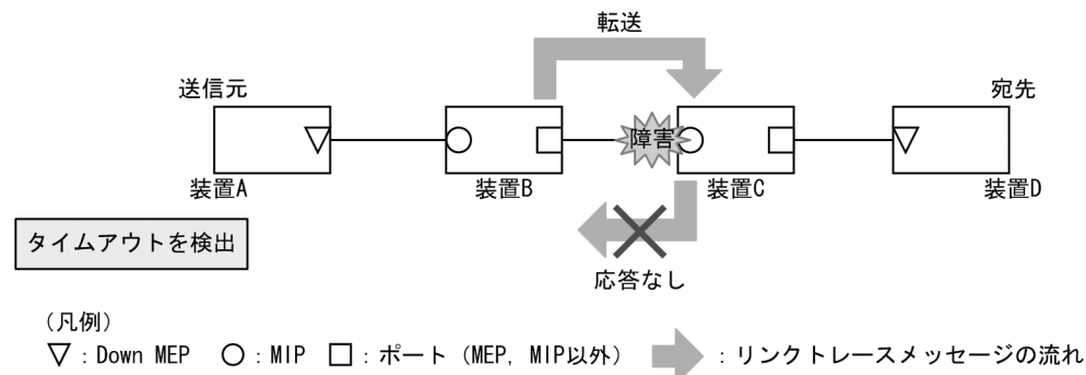
図 21-25 Linktrace でタイムアウトを検出した例
