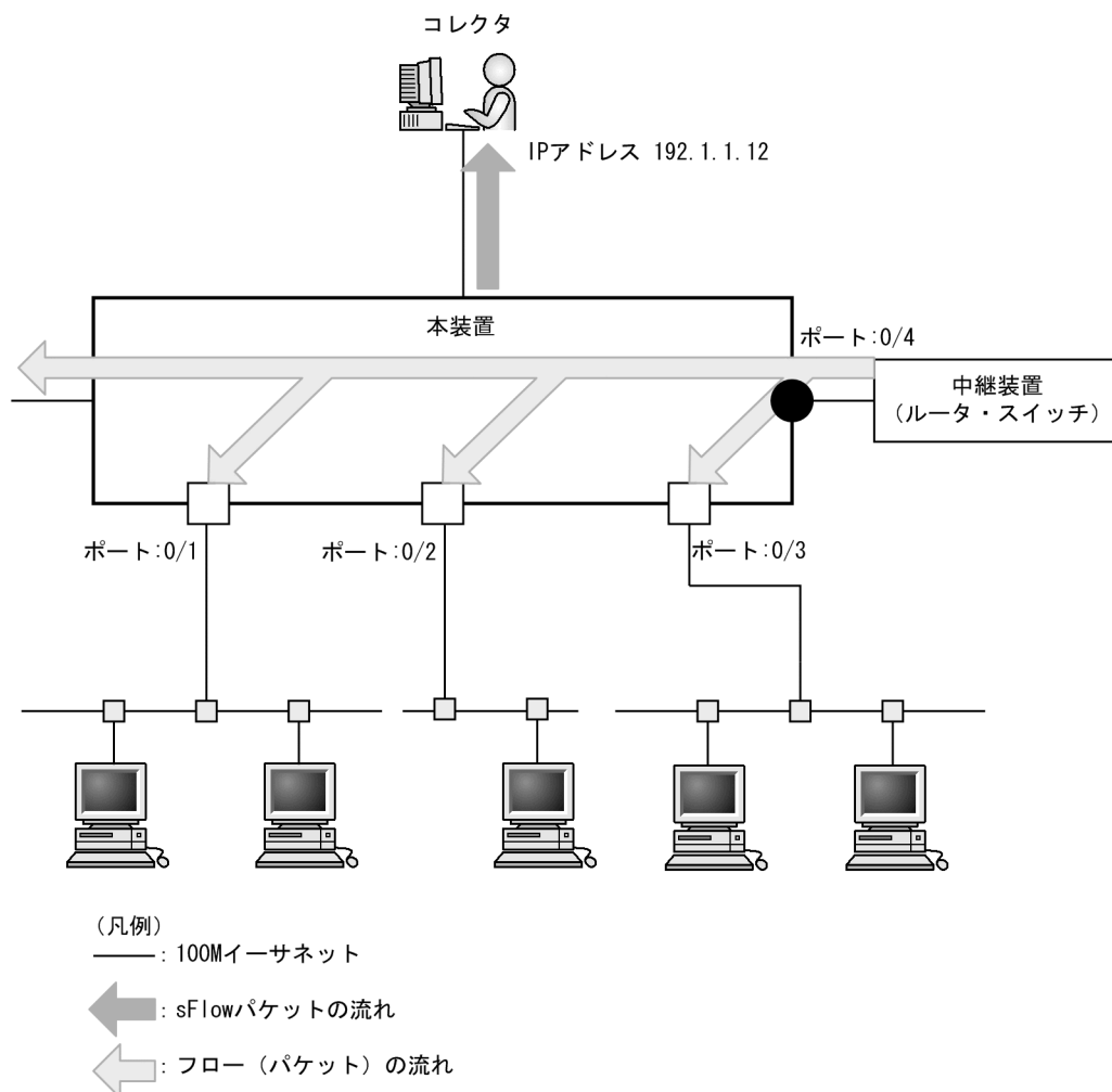
図 24-7 ポート 0/4 の受信パケットをモニタする設定例
