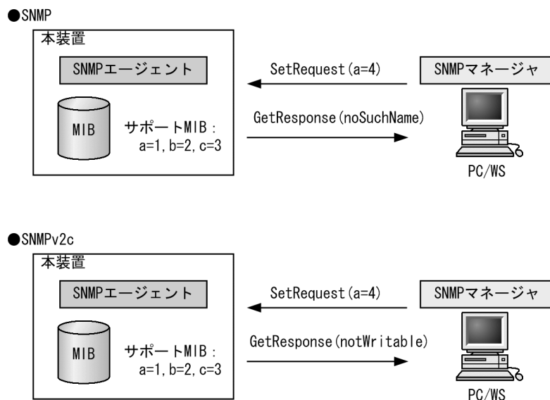
図 22-13 MIB 変数が読み出し専用の場合の SetRequest オペレーション
