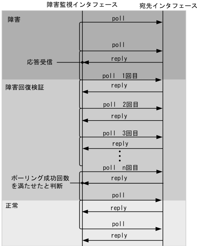
図 16-10 障害回復検証動作シーケンス
