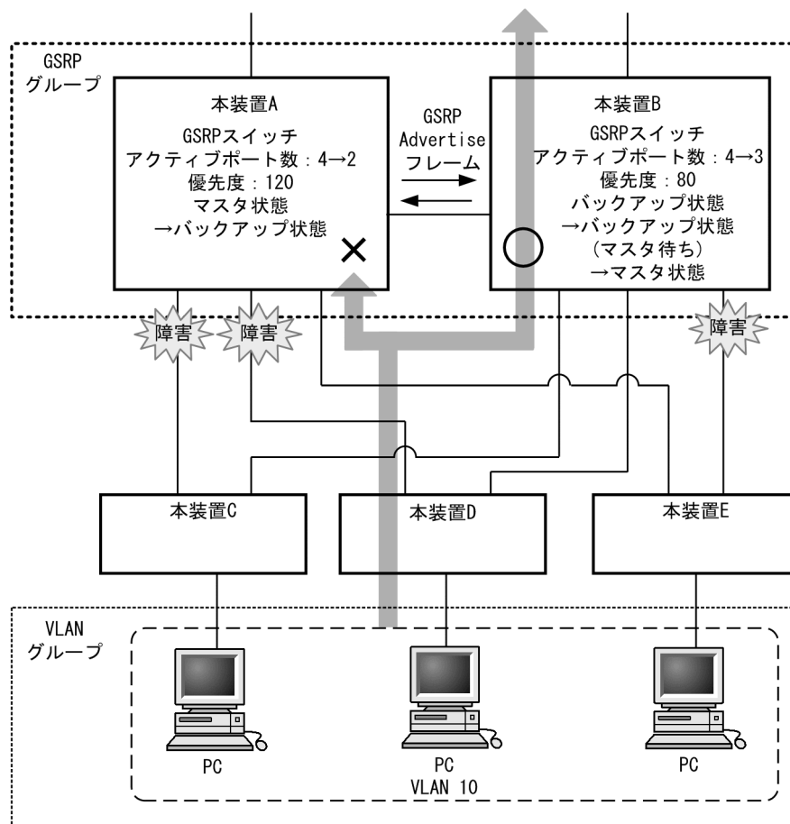
図 14-7 リンク障害時の動作例
