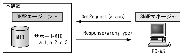
図 22-22 設定値のタイプが正しくない場合の SetRequest オペレーション例
