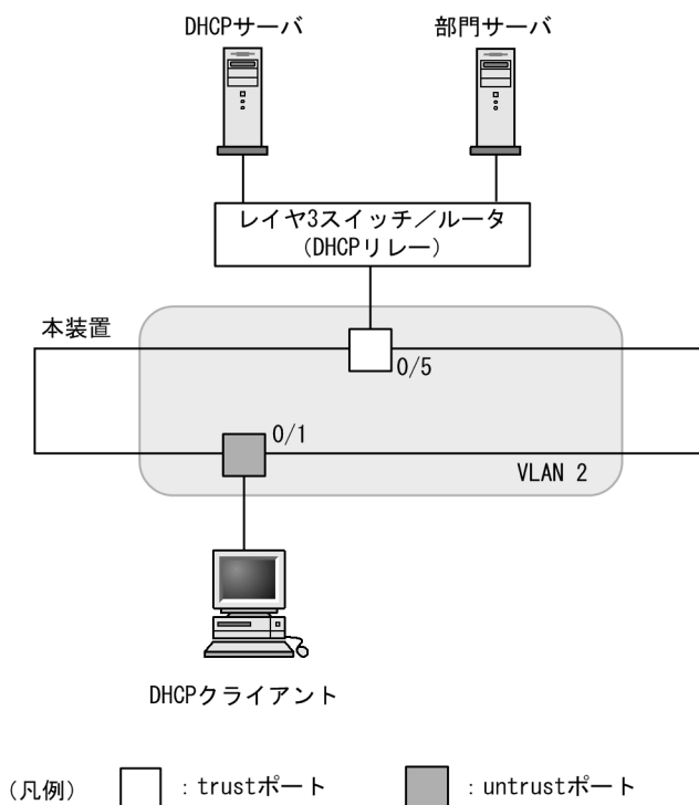
図 13-10 DHCP snooping の基本的な構成例
