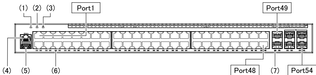
図1-7 正面パネルレイアウト
