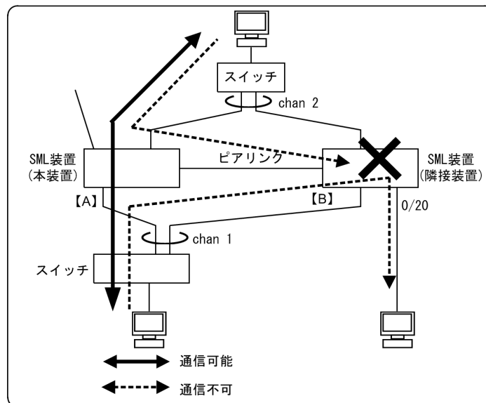
図 20-10 装置障害時の動作
