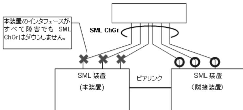
図 20-12 SML ChGr 内インタフェースの障害
