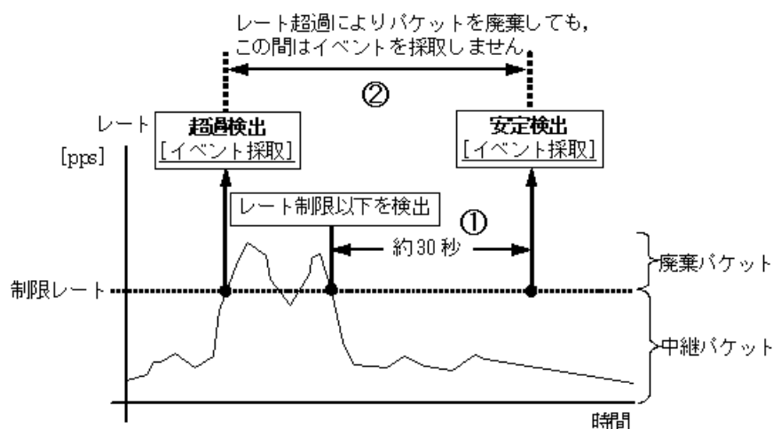
図 15-12 DHCP パケット受信レートの運用ログ情報採取契機
