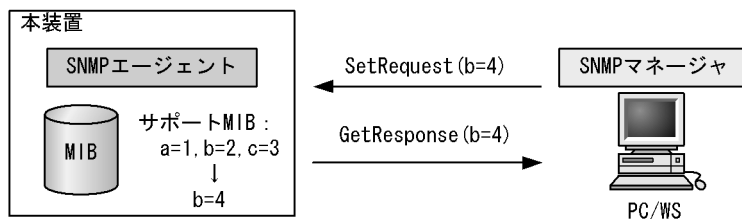
図 25-11 SetRequest オペレーション
