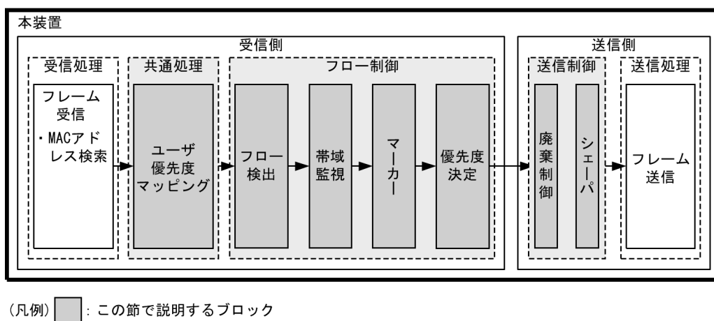
図 2-1 本装置の QoS 制御の機能ブロック
