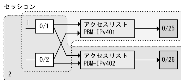
図 30-5 複数モニターポート対複数ミラーポートの設定例
