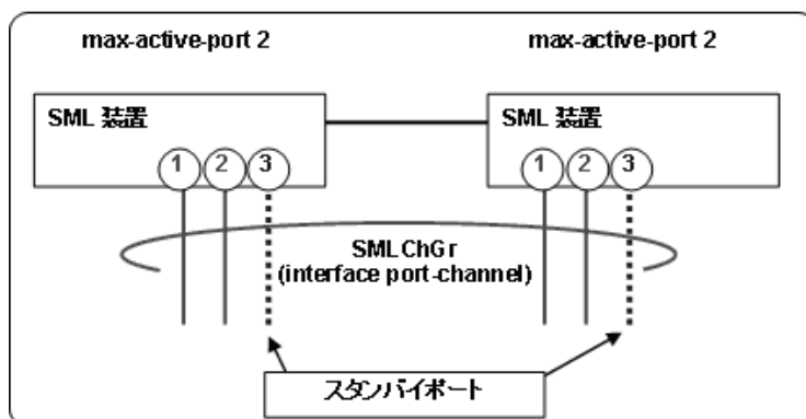
図 20-15 スタンバイリンクの制限
