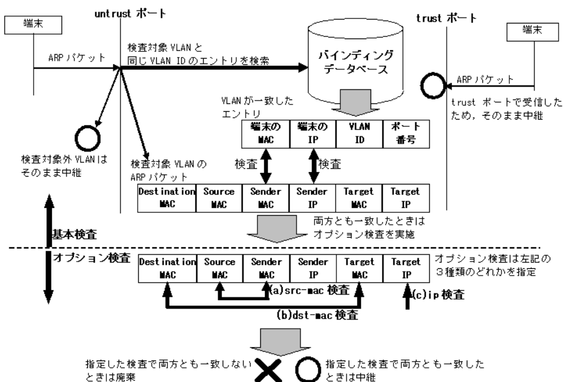
図 15-14 ダイナミック ARP 検査の基本検査とオプション検査の関係
