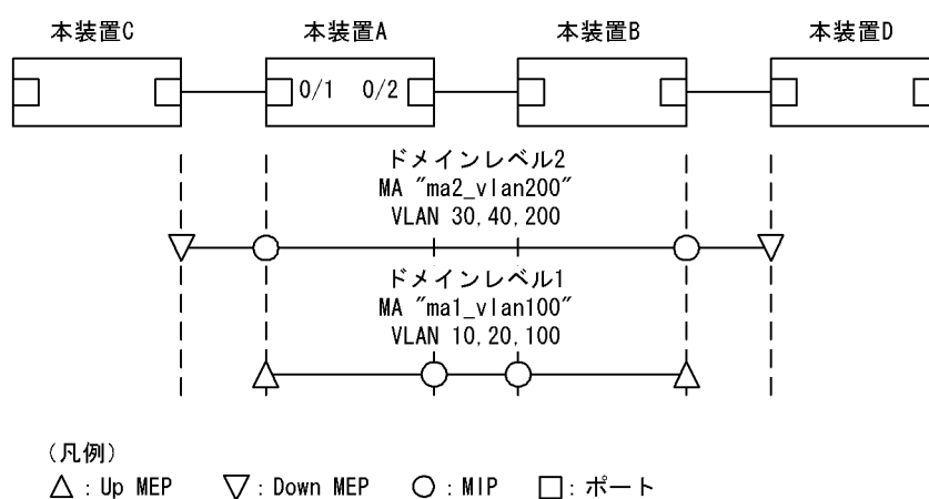
図 24-31 CFM の設定例（複数ドメイン）
