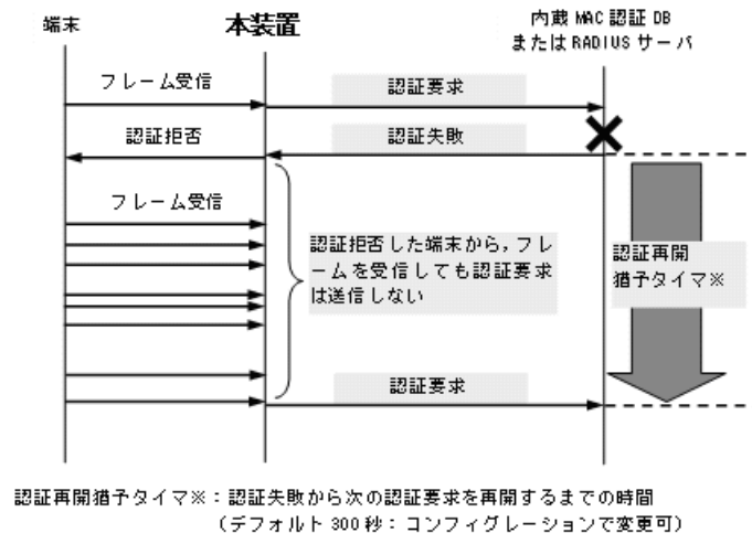
図 10-3 認証再開猶予タイマ概要
