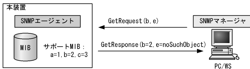
図 25-7 GetRequest オペレーション (SNMPv2C)
