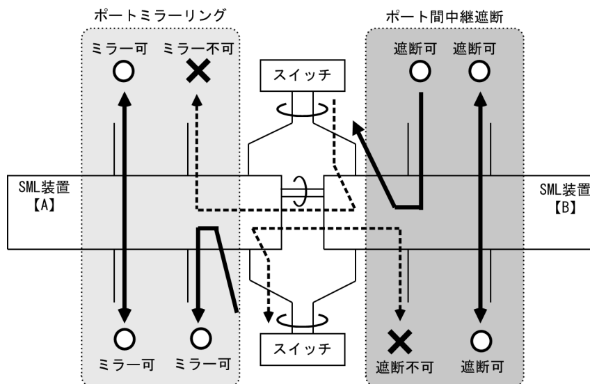
図 20-19 ポートミラーリング・ポート間中継遮断機能の使用可否
