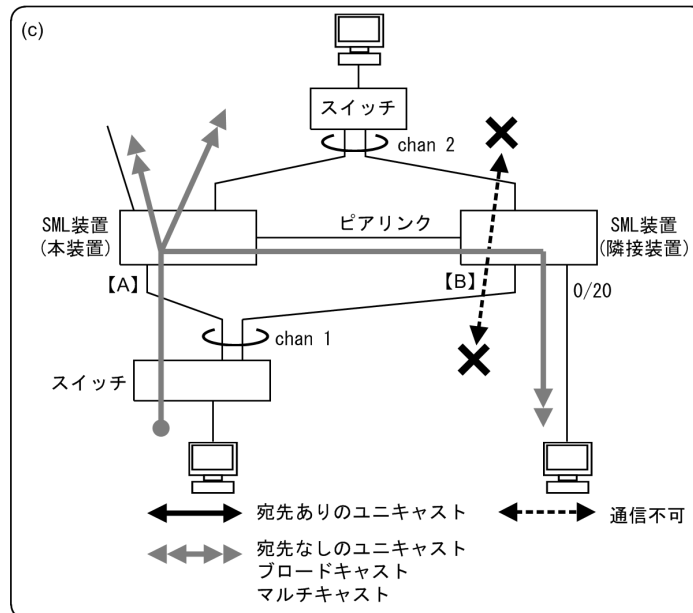
図 20-6 MAC アドレステーブルのエントリに一致しないフレームの中継
