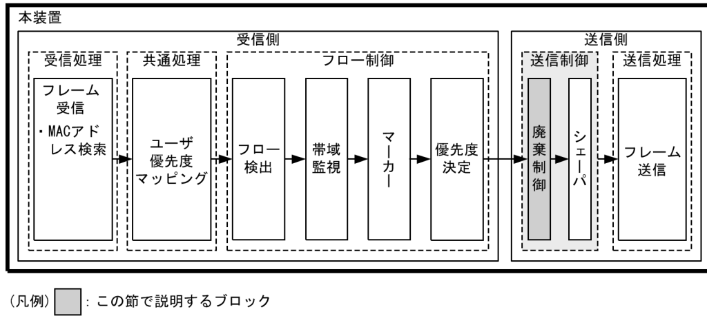
図 4-6 廃棄制御の位置づけ
