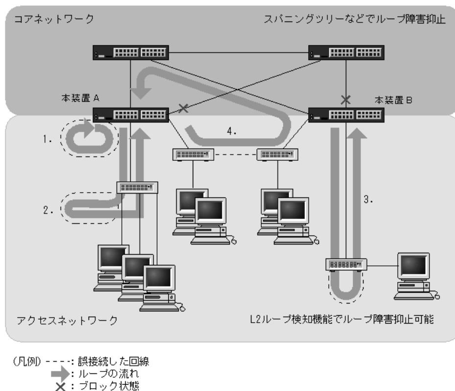
図 23-1 ループ障害の発生例
