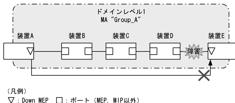
図 24-10 ドメイン内に MIP が設定されていない構成の例
