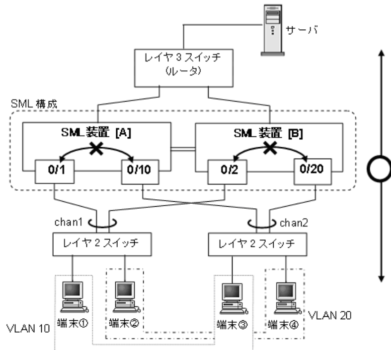
図 20-23 SML 構成でポート間中継遮断機能を使用する場合の構成例
