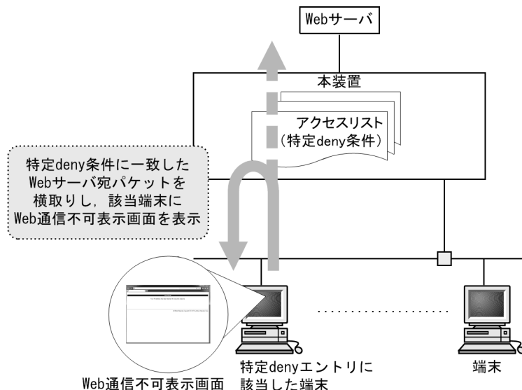
図 17-1 特定端末への Web 通信不可表示機能概要図
