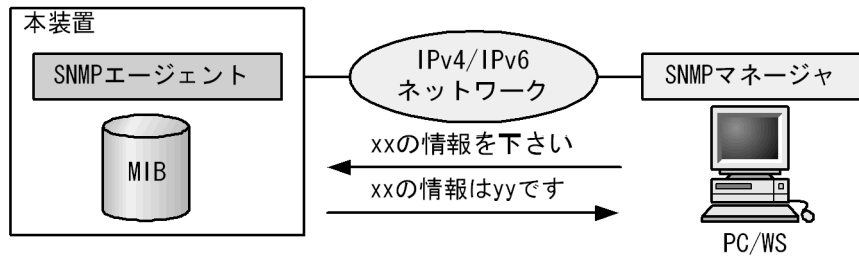
図 25-2 MIB 取得の例
