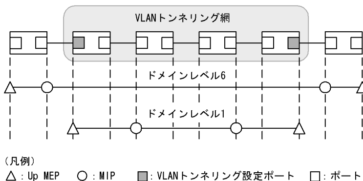
図 24-27 VLAN トンネリング網内と VLAN トンネリング網外で CFM を使用する例
