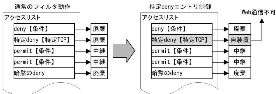
図 17-2 特定 deny エントリ制御
