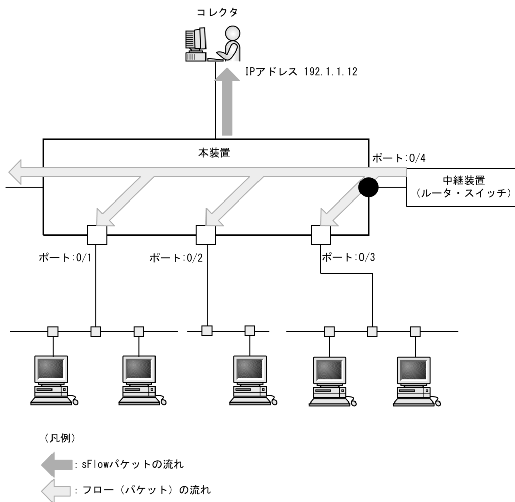
図 27-7 ポート 0/4 の受信パケットをモニタする設定例
