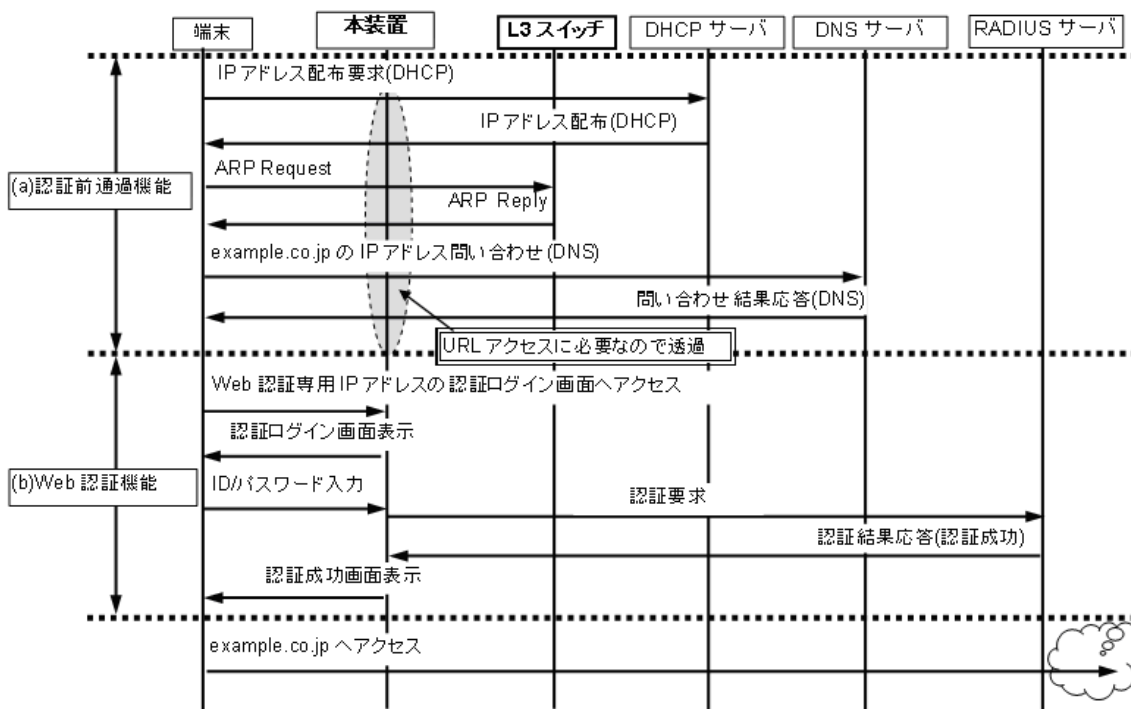
図 8-7 認証動作（Web 認証専用 IP アドレス使用時）
