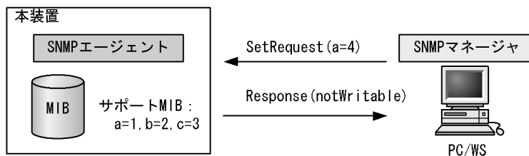
図 25-20 MIB 変数が読み出し専用の場合の SetRequest オペレーション
