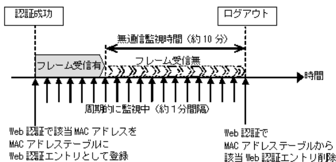
図 8-4 認証済み端末の無通信監視概要
