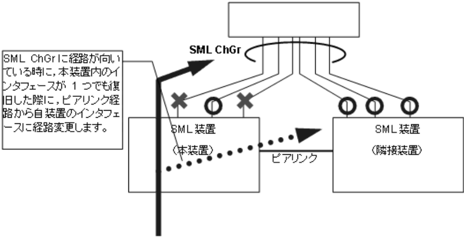
図 20-14 SML ChGr インタフェースへの経路復旧
