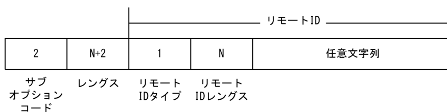
図 15-11 リモート ID タイプ 1 の形式
