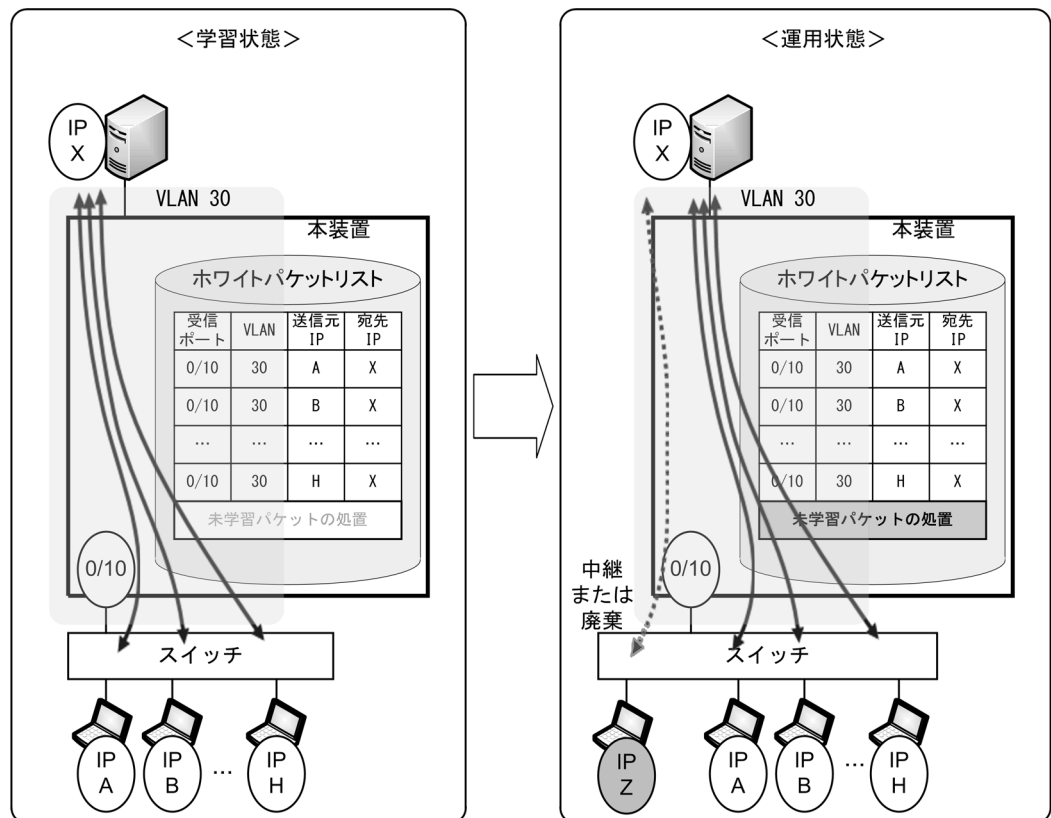
図 16-5 ホワイトパケットリスト機能の概要
