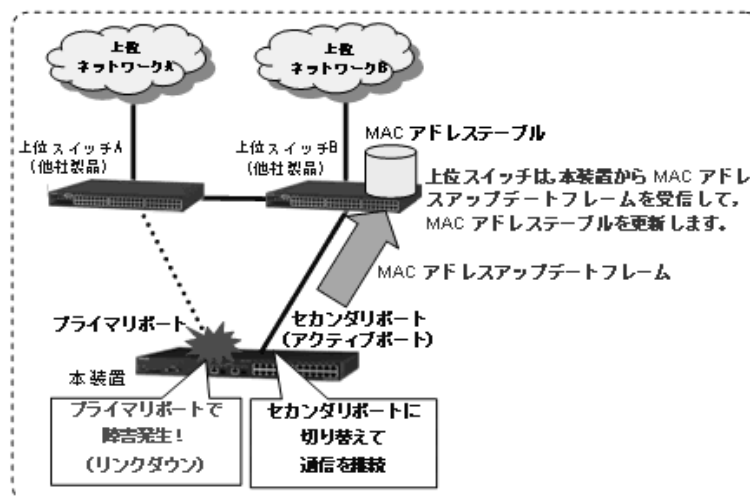
図 19-5 MAC アドレスアップデート機能概要
