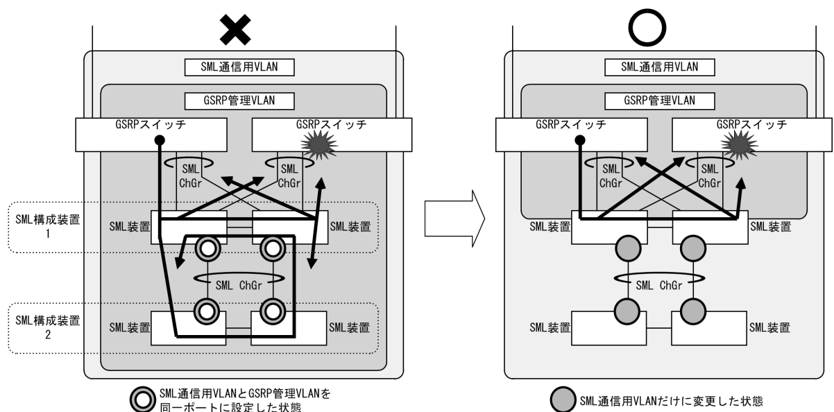
図 20-22 GSRP 管理 VLAN と SML 通信用 VLAN の混在
