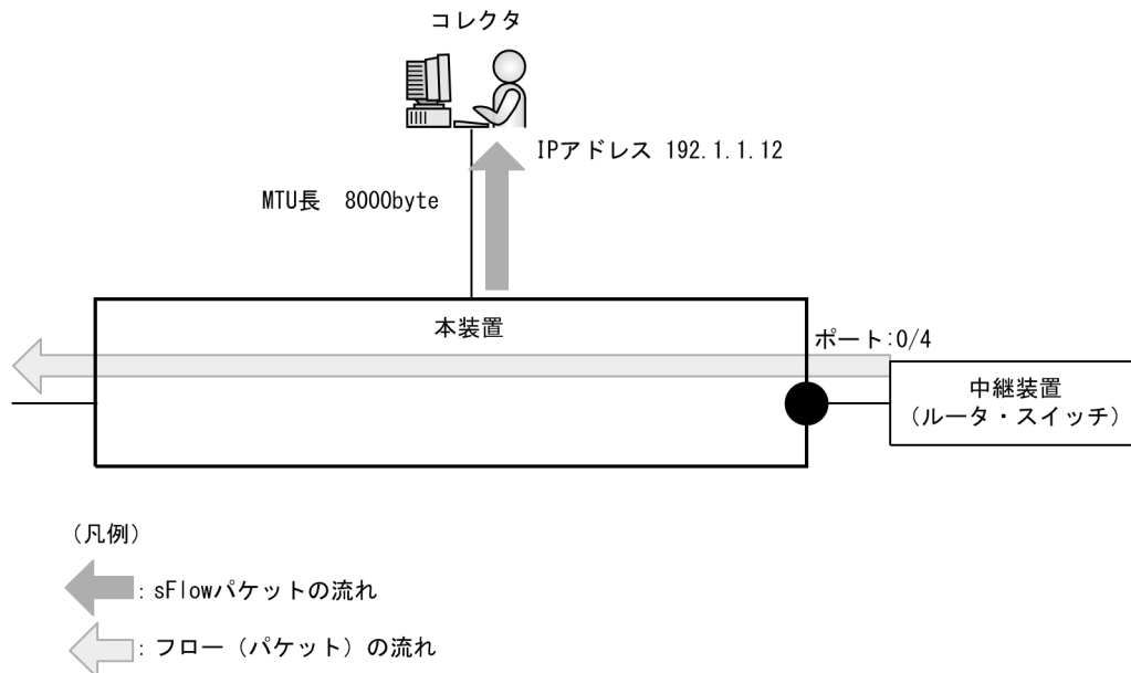
図 27-9 コレクタへの送信を MTU=8000byte に設定する例
