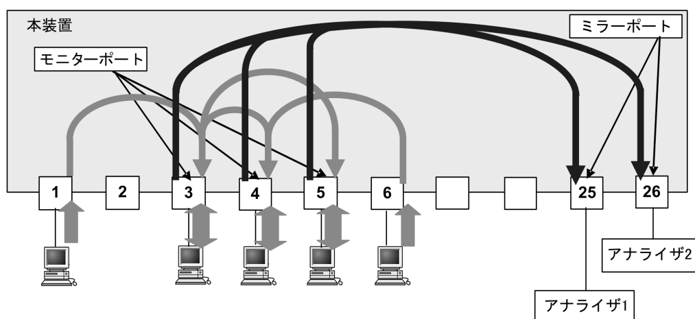
図 29-5 多対 2 のミラーリング
