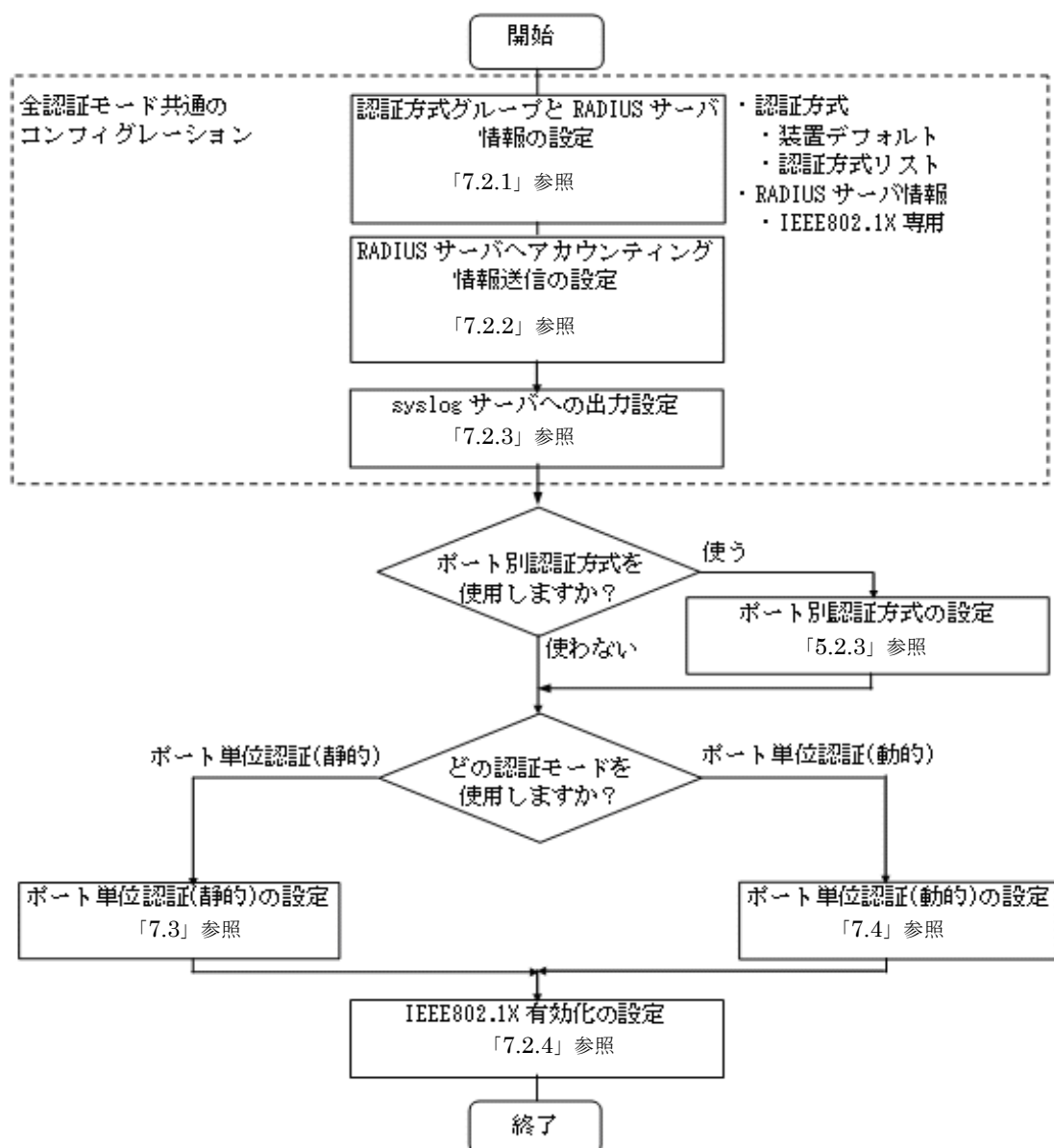
図 7-1 IEEE802.1X の設定手順
