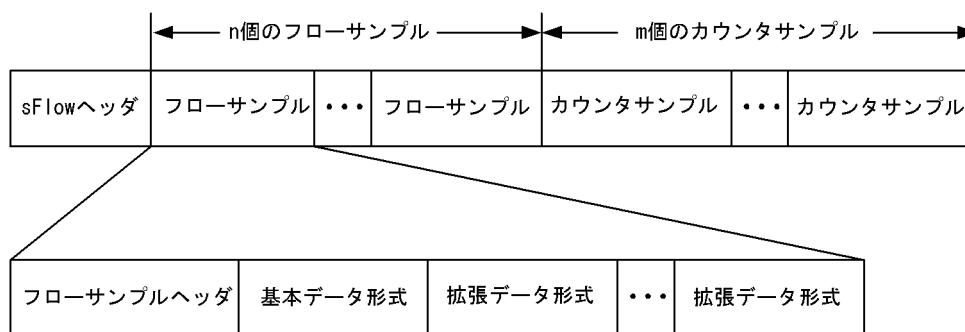
図 27-5 フローサンプルのフォーマット
