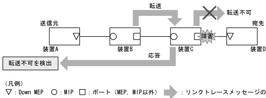
図 24-26 Linktrace で通信不可を検出した例
