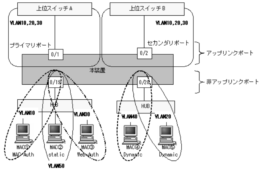
図 19-6 MAC アドレス送信対象例
