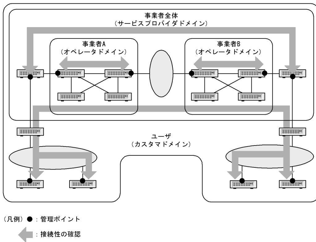
図 24-1 CFM の構成例
