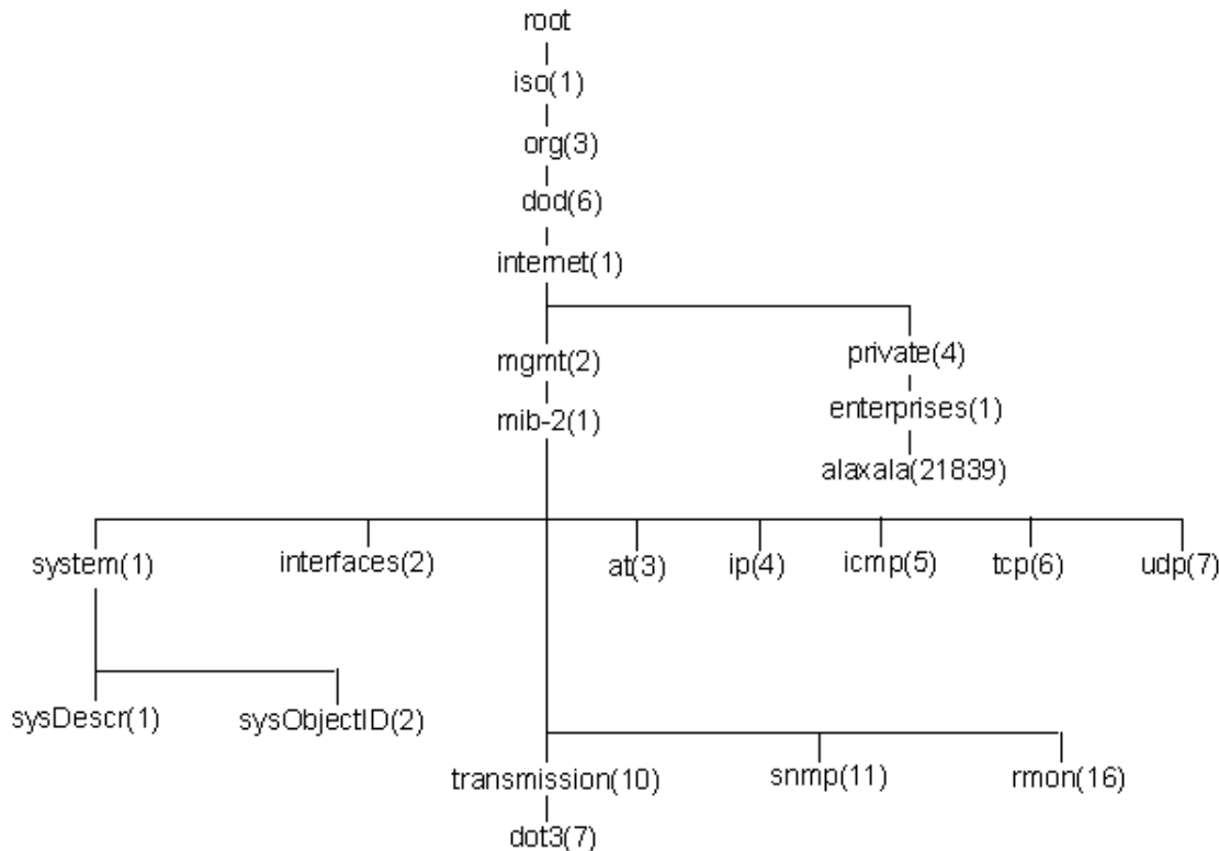
図 25-5 MIB ツリーの構造例
