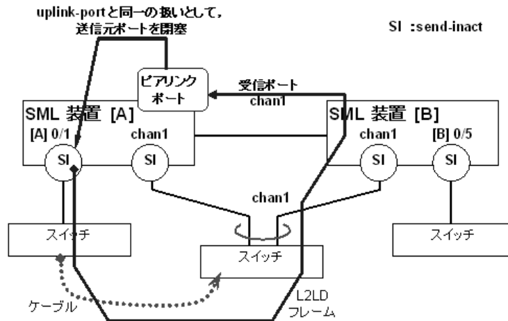
図 20-18 SML ChGr でのループ検知
