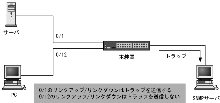
図 25-25 リンクトラップの構成図
