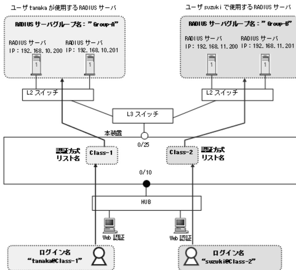
図 5-8 ユーザ ID 別認証方式構成図例
