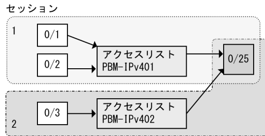
図 30-4 複数モニターポート対 1 ミラーポートの設定例
