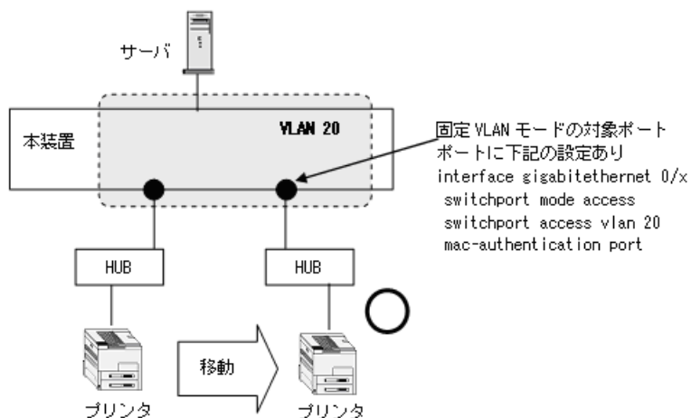
図 10-6 固定 VLAN モード ローミング概要図
