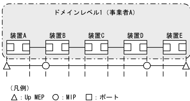
図 24-17 MIP 設定後の構成例
