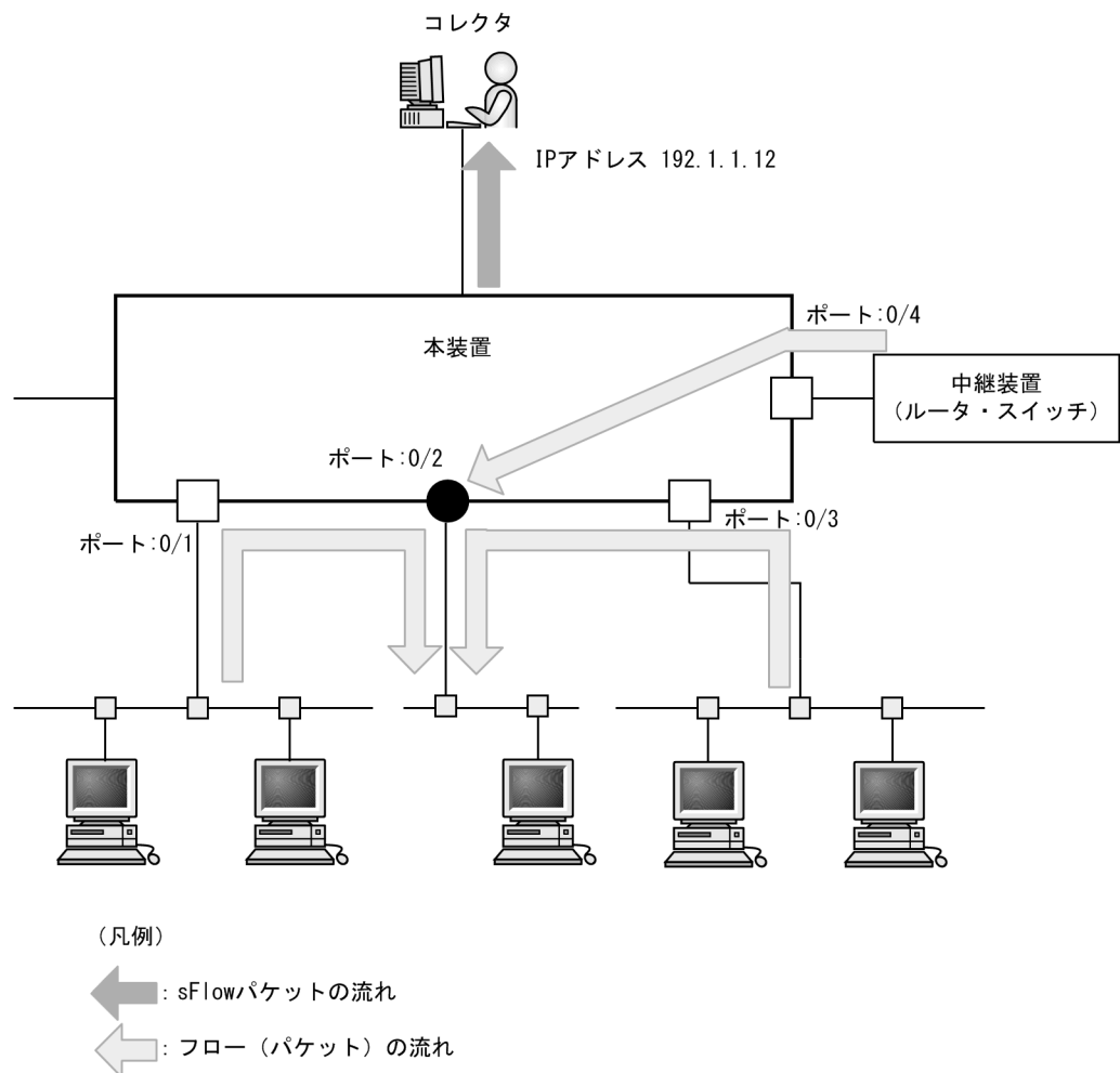
図 27-8 ポート 0/2 の送信パケットをモニタする設定例
