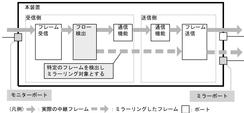
図 30-1 受信フレームに対するポリシーベースミラーリングの動作
