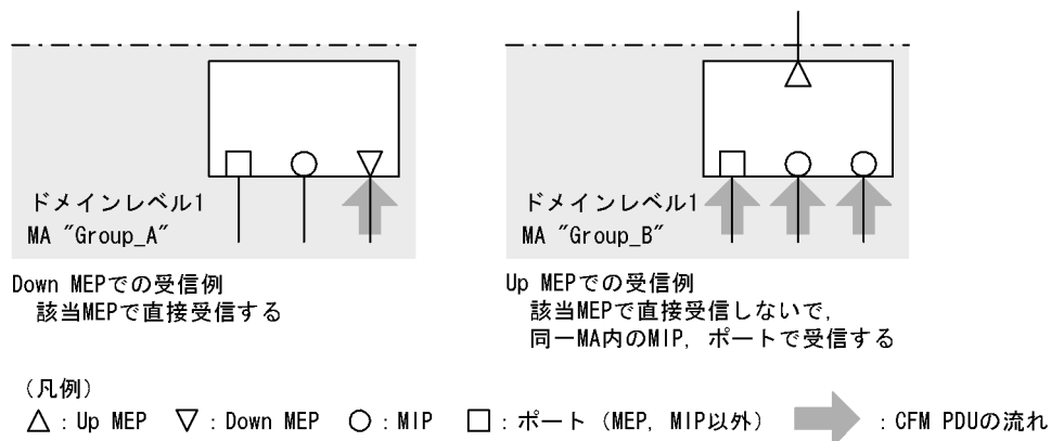
図 24-7 Down MEP, Up MEP での受信
