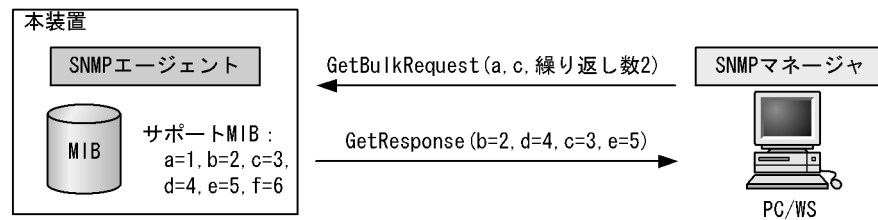
図 25-10 GetBulkRequest オペレーション
