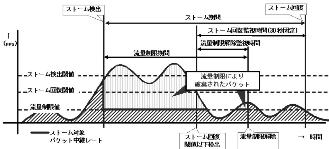
図 21-1 流量制限動作
