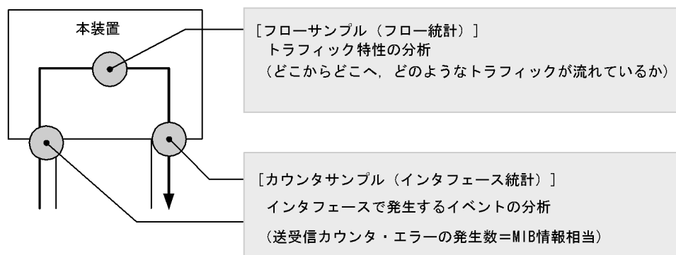
図 27-3 フローサンプルとカウンタサンプル
