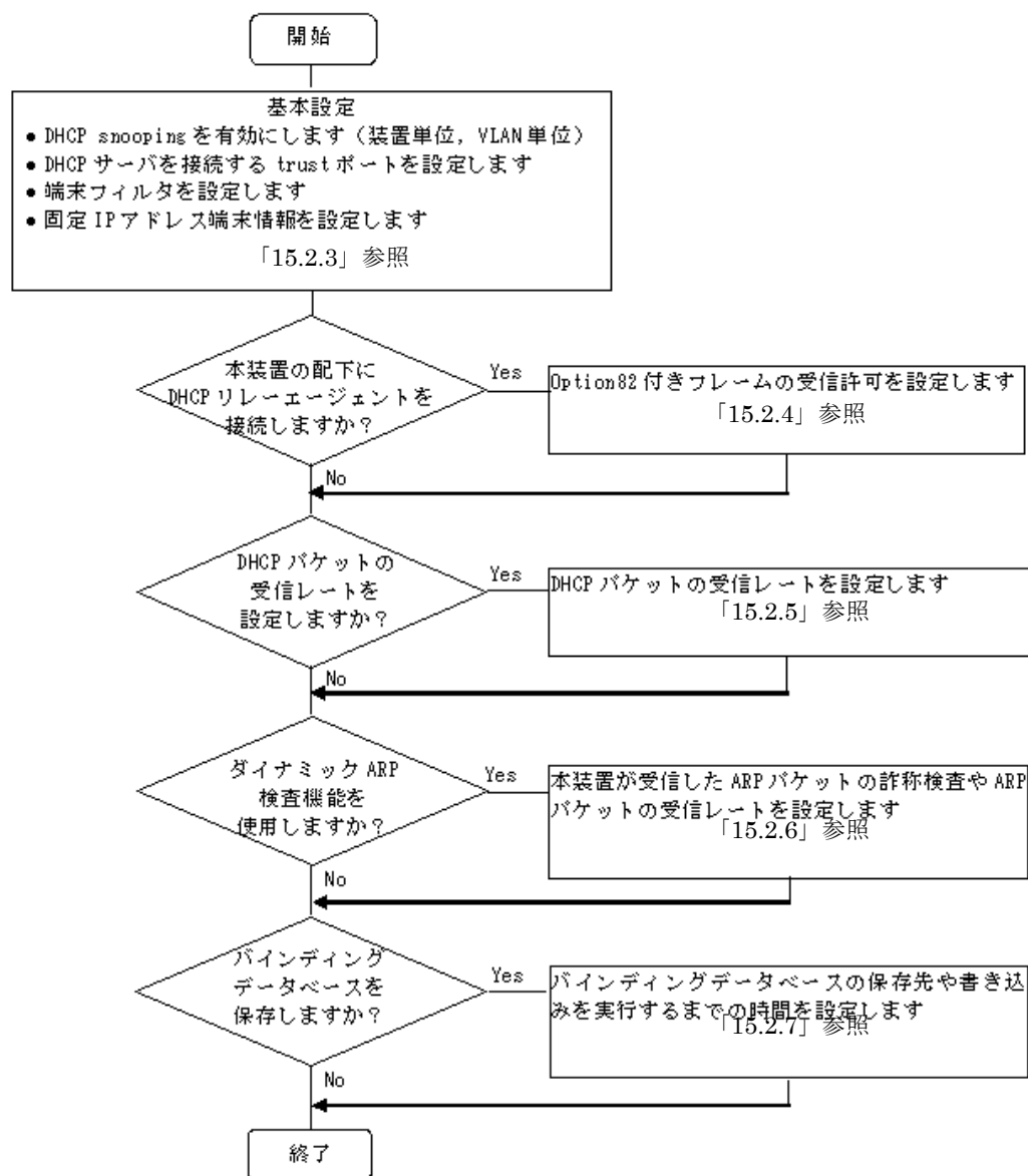
図 15-16 DHCP snooping の設定手順
