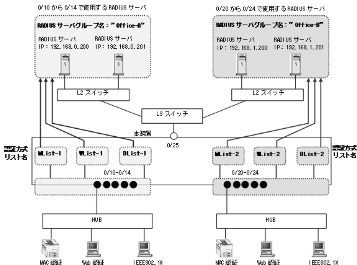
図 5-7 ポート別認証方式構成図例
