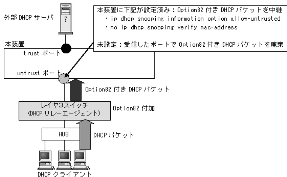
図 15-6 Option82 付きパケットが付加される構成例
