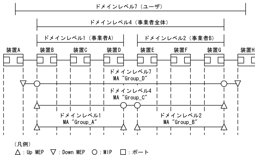
図 24-15 ドメインレベル7の設定
