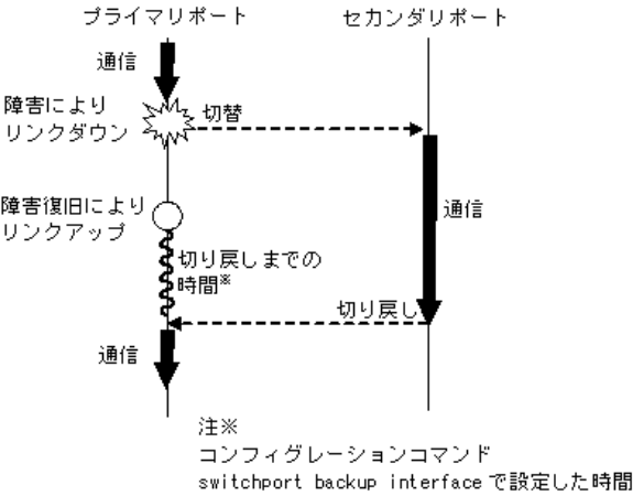
図 19-4 タイマ切り戻し概要
