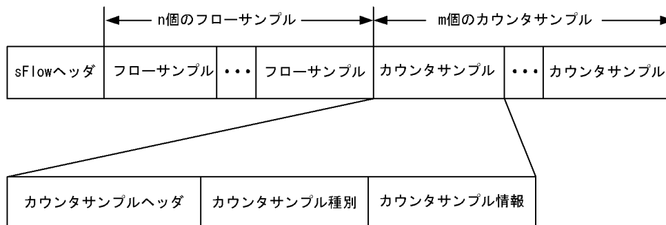
図 27-6 カウンタサンプルのフォーマット
