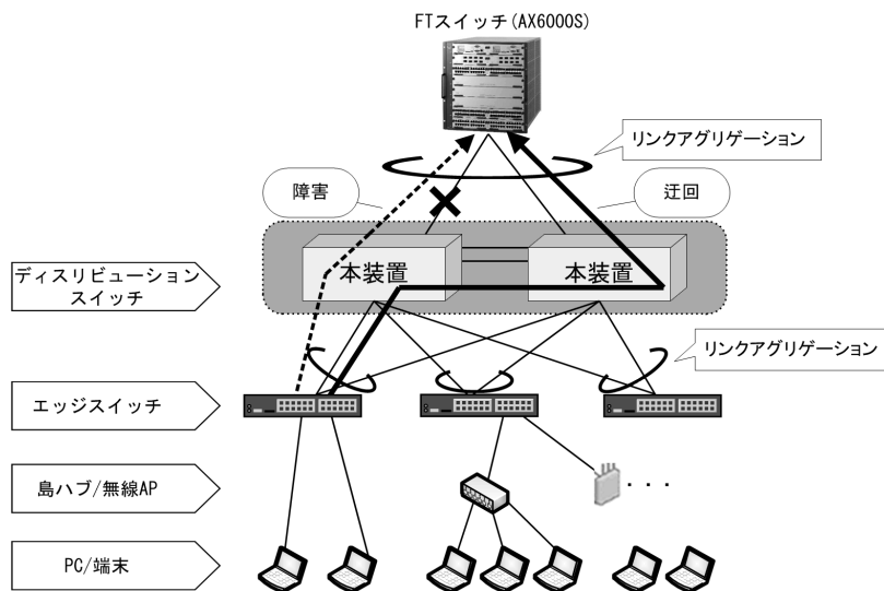
図 20-1 SML 機能による回線障害の迂回
