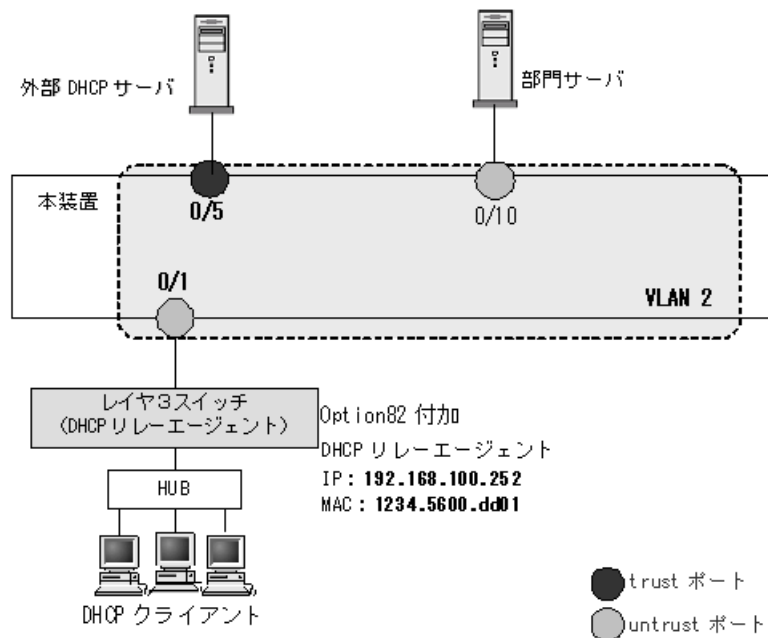
図 15-19 本装置の配下に DHCP リレーエージェントを接続した場合の構成例
