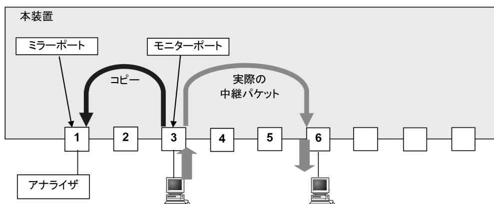
図 29-1 受信フレームのミラーリング
