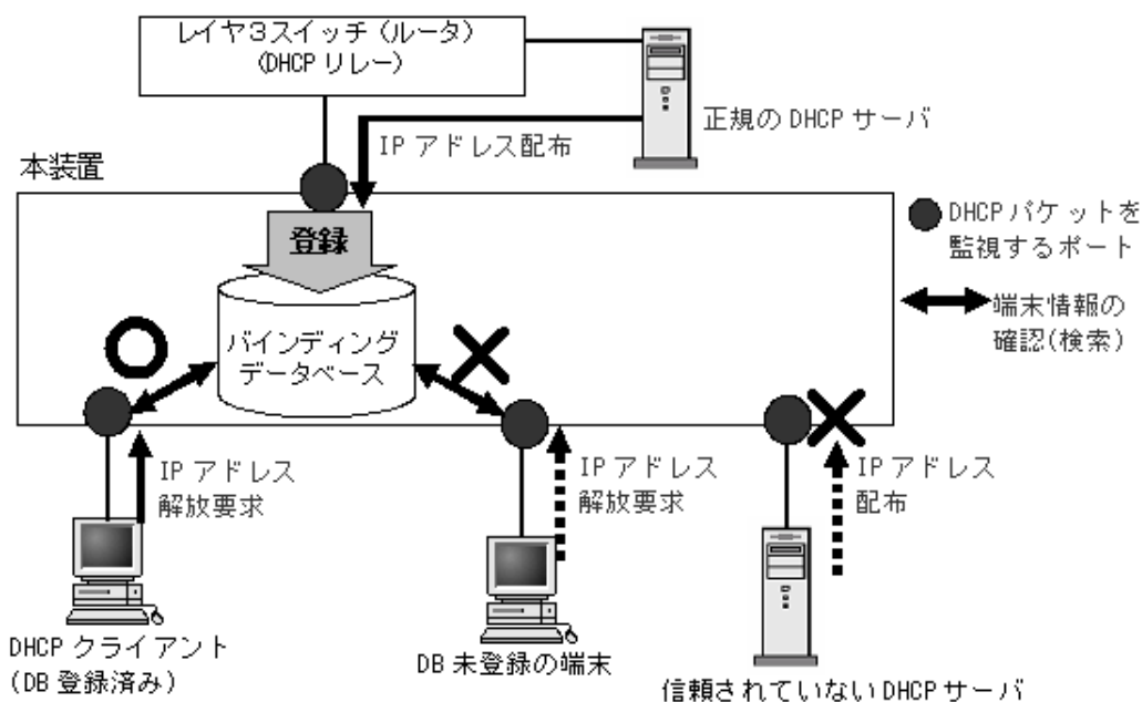
図 15-1 DHCP snooping 概要
