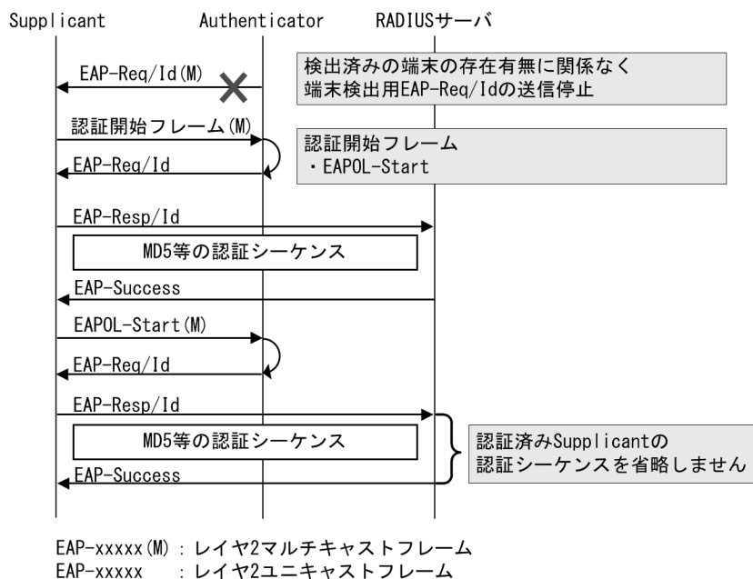
図 6-8 passive の EAP-Request/Identity のシーケンス
