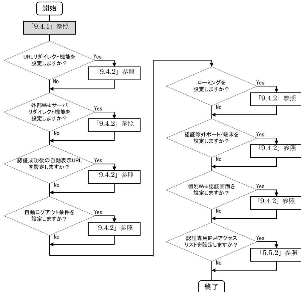
図 9-6 ダイナミック VLAN モードの設定手順
