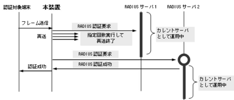
図 5-10 RADIUS サーバ選択のシーケンス
