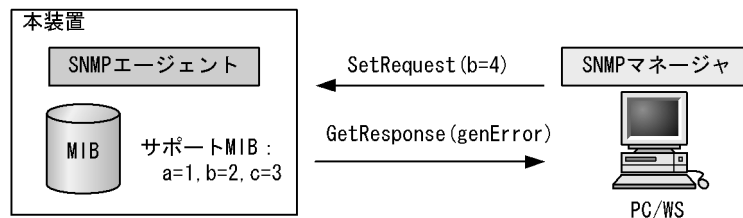
図 25-14 装置の状態によって設定できない場合の SetRequest オペレーション
