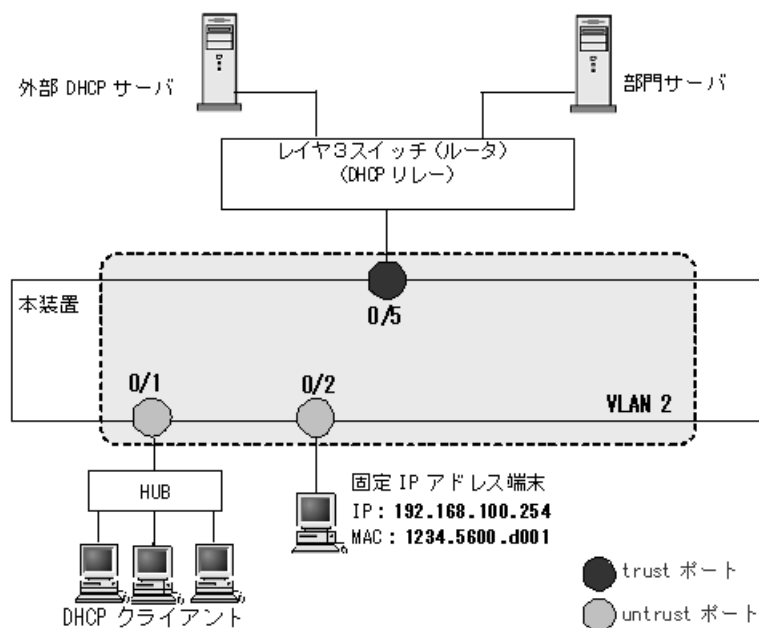
図 15-18 固定 IP アドレス端末を接続した場合の構成例
