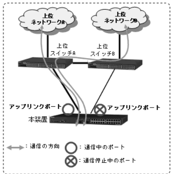
図 19-1 アップリンク・リダンダント概要
