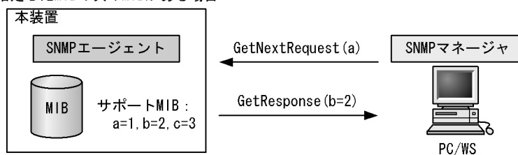
図 25-8 GetNextRequest オペレーション
