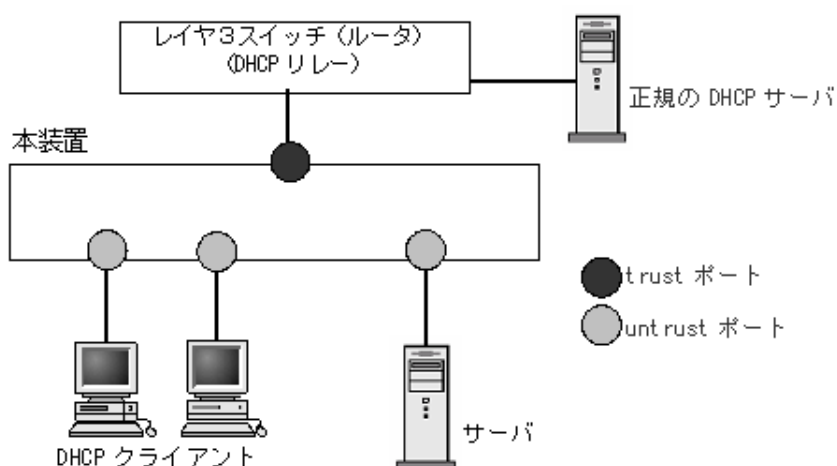
図 15-3 DHCP snooping のポート種別
