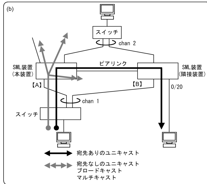
図 20-5 MAC アドレステーブルに登録されているピアリンク向け中継
