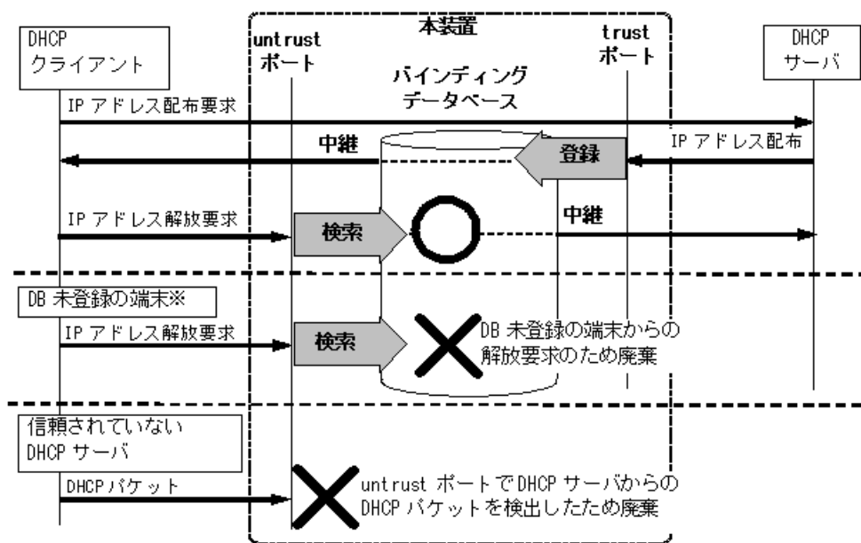
図 15-4 DHCP パケット監視の動作概要
