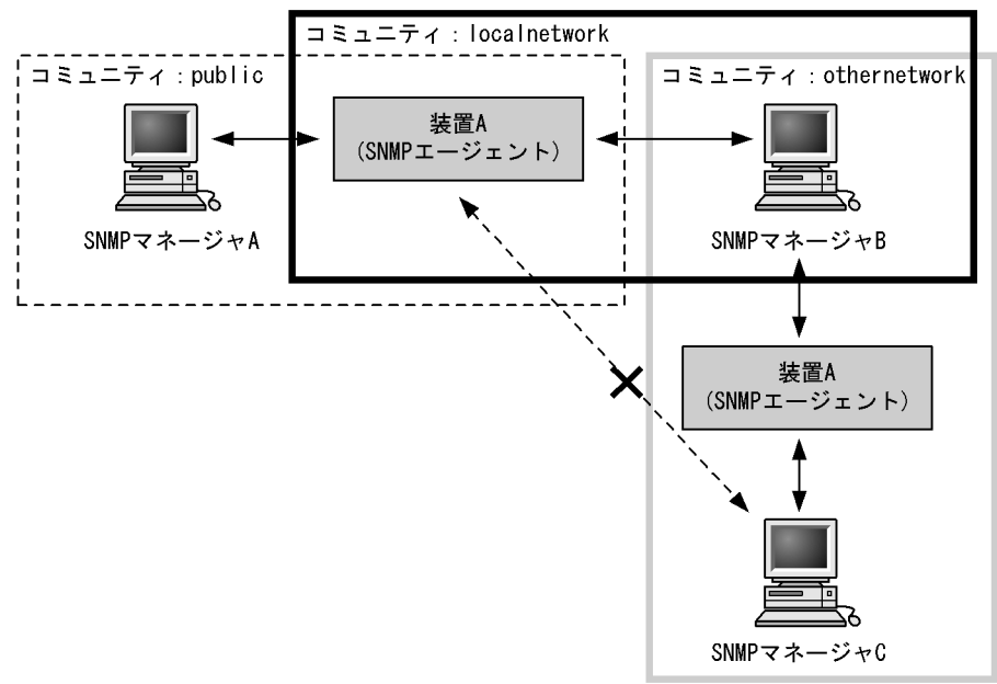
図 25-15 コミュニティによるオペレーション
