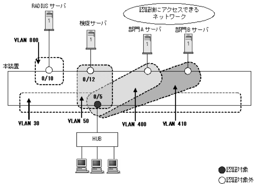
図 5-22 ダイナミック VLAN モードの VLAN 名称指定の使用例
