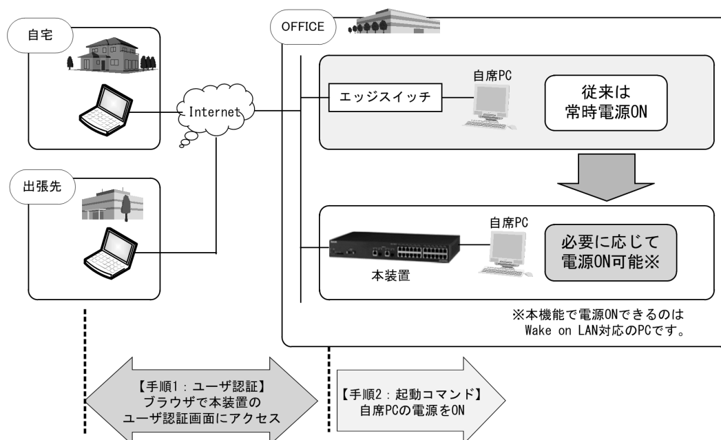
図 13-1 セキュア Wake on LAN 概要図
