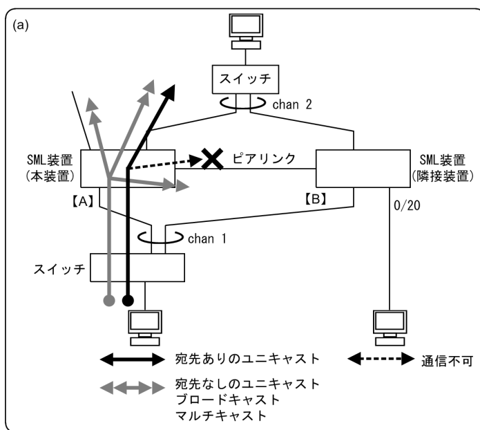
図 20-4 MAC アドレステーブルのエントリに登録されている SML ChGr 向け中継
