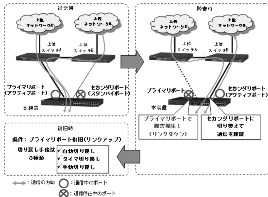
図 19-2 アップリンク・リダンダント動作概要
