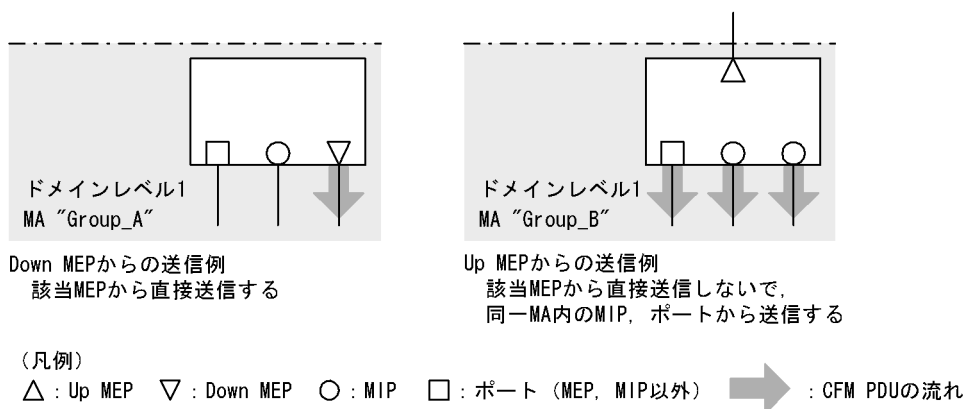
図 24-6 Down MEP, Up MEP からの送信
