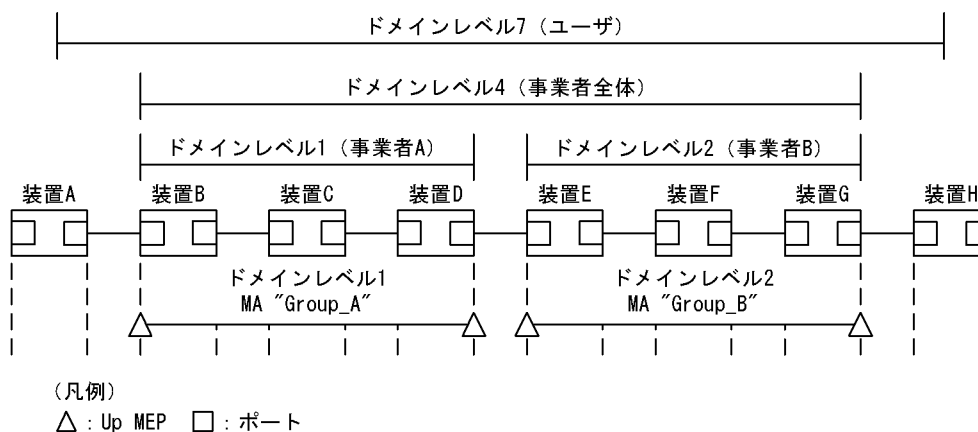
図 24-13 ドメインレベル 1, 2 の設定
