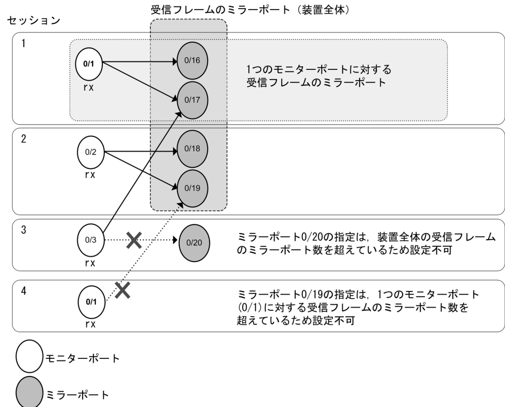
図 29-7 受信フレームのミラーポート数（ホワイトリスト機能、ICMP 限定ミラーリング機能のミラー設定無）
