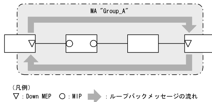
図 24-22 MEP に対して Loopback を実行
