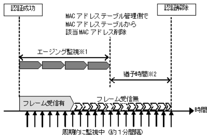
図 6-12 MAC アドレステーブルエージング監視による解除概要
