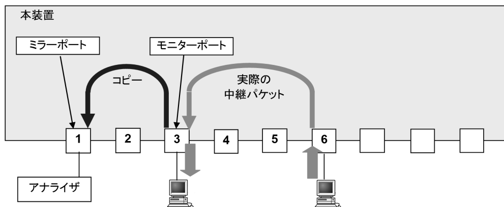
図 29-2 送信フレームのミラーリング
