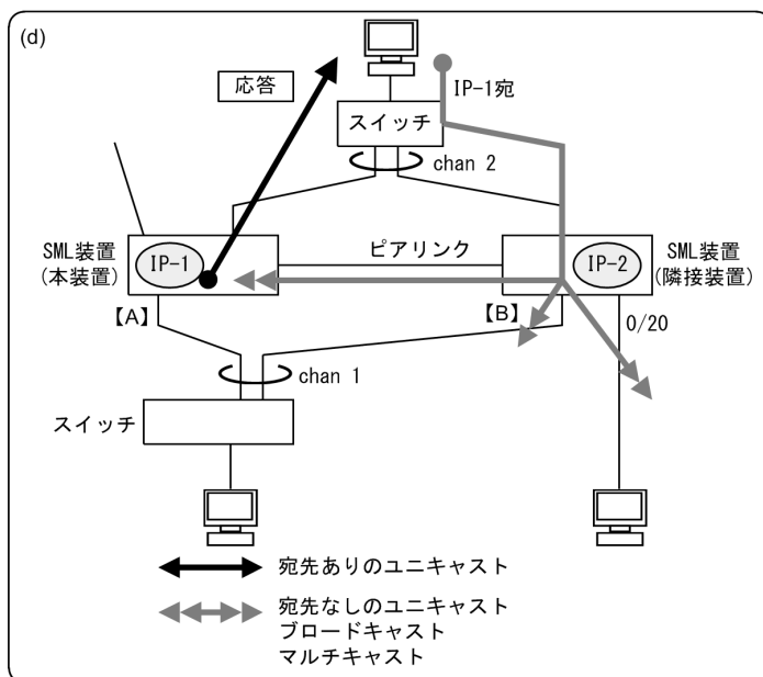
図 20-7 本装置宛のフレーム
