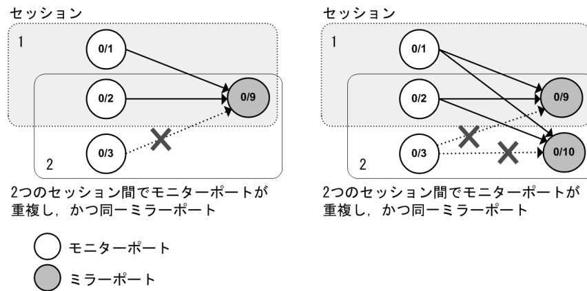
図 30-2 設定不可の組み合わせ
