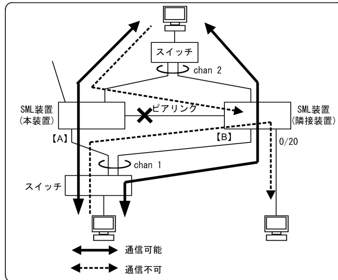
図 20-9 ピアリンク障害時の動作
