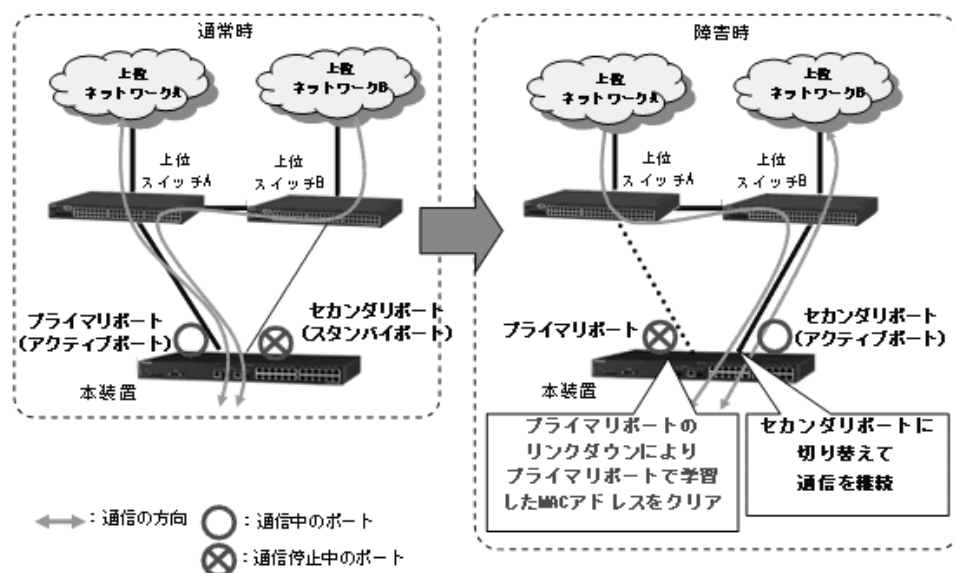
図 19-3 プライマリ・セカンダリ切り替え概要
