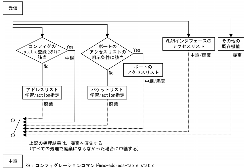
図 16-9 機能併用時の判定イメージと廃棄優先
