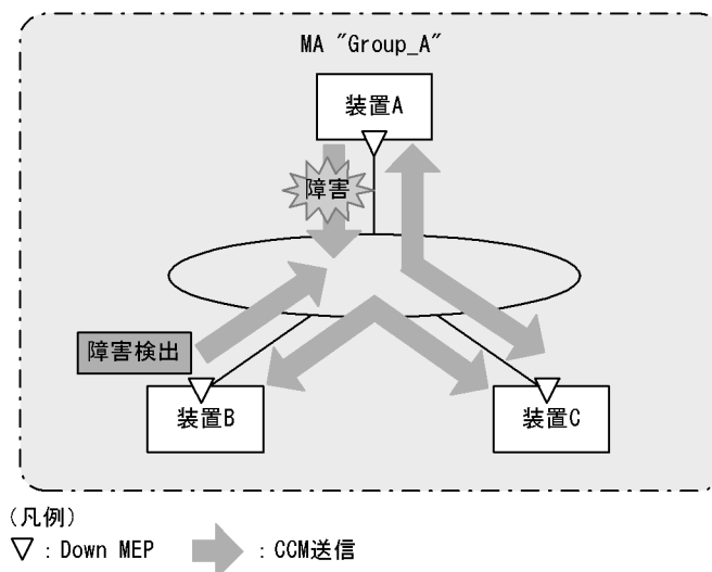
図 24-19 CC で障害を検出
