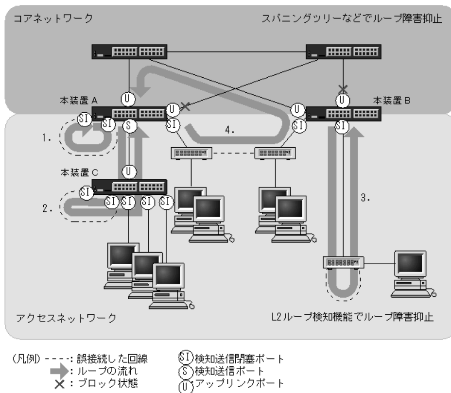
図 23-2 L2 ループ検知機能を適用したネットワーク構成例
