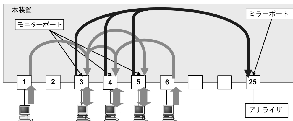
図 29-3 複数ポートのフレームのミラーリング（多対 1）
