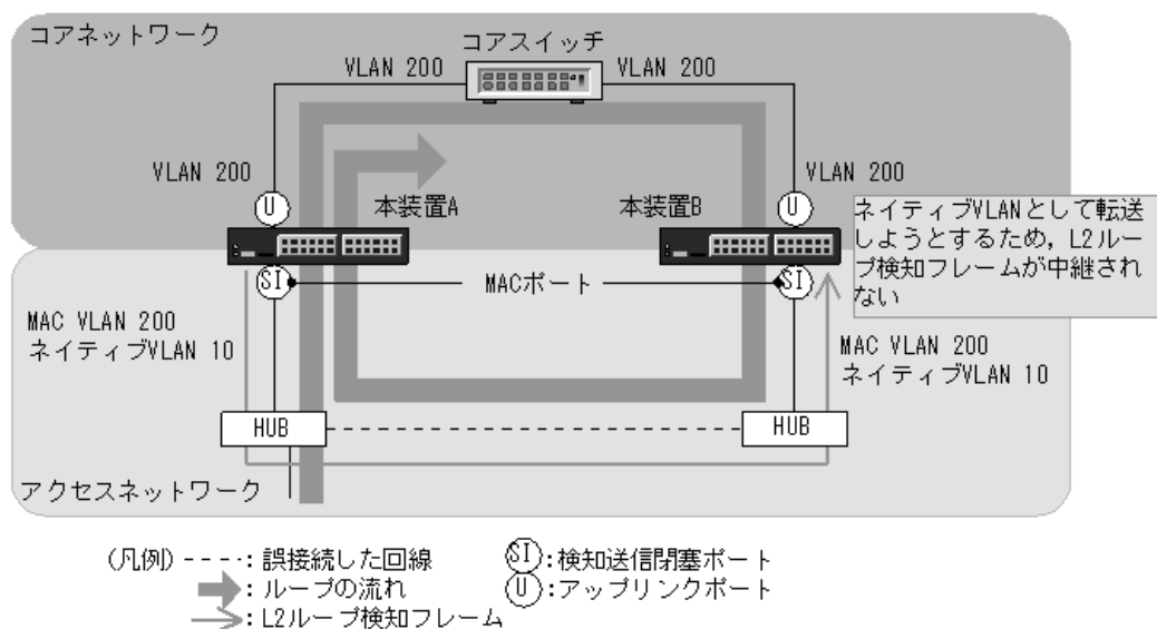
図 23-3 ループ検知の制限となる構成
