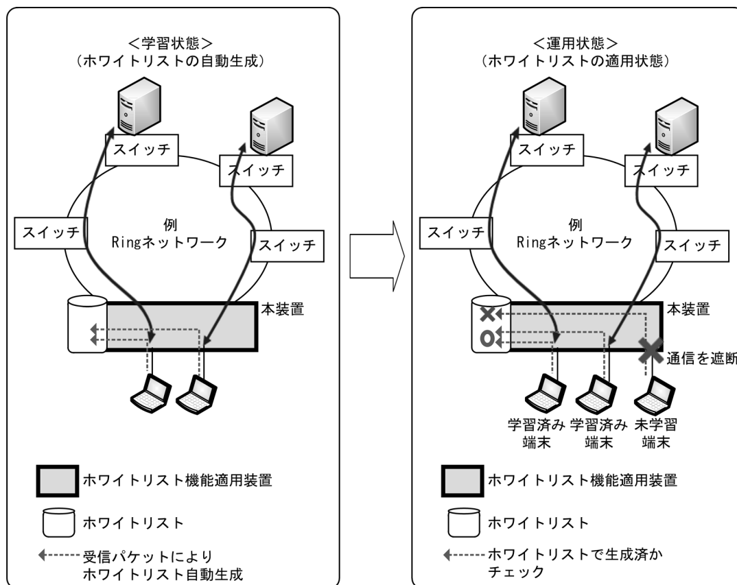
図 16-1 ホワイトリスト機能の概要
