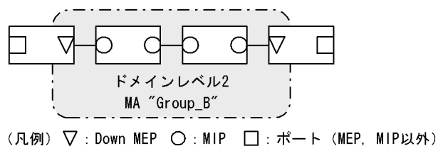
図 24-5 Down MEP の設定例
