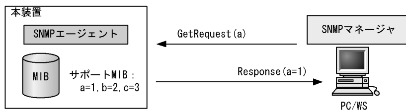
図 25-16 GetRequest オペレーション
