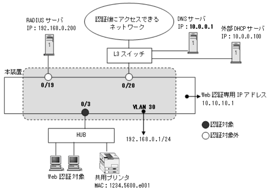
図 5-21 認証専用 IPv4 アクセスリストの使用例
