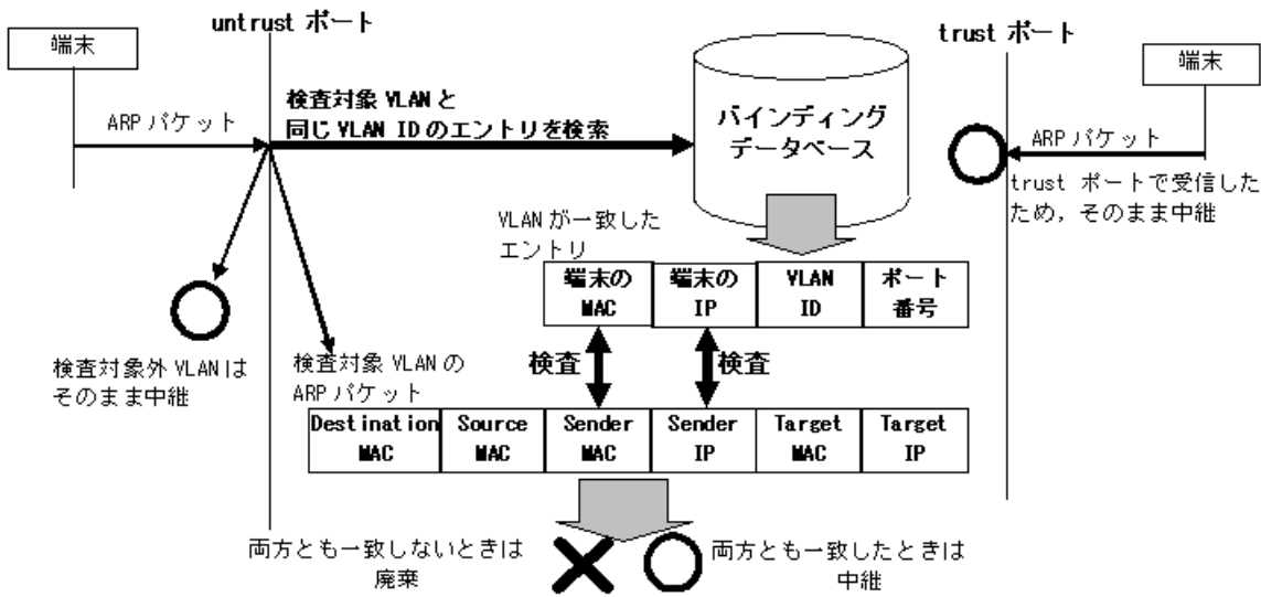
図 15-13 ダイナミック ARP 検査の基本検査概要
