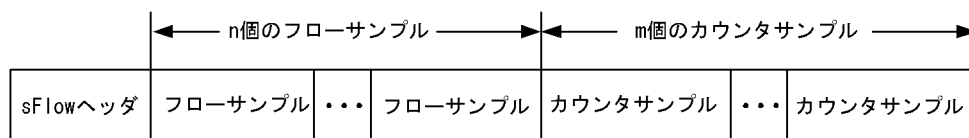
図 27-4 sFlow パケットフォーマット
