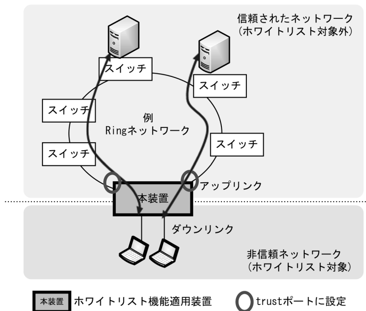
図 16-8 ホワイトリスト機能と Ring ネットワークの併用例
