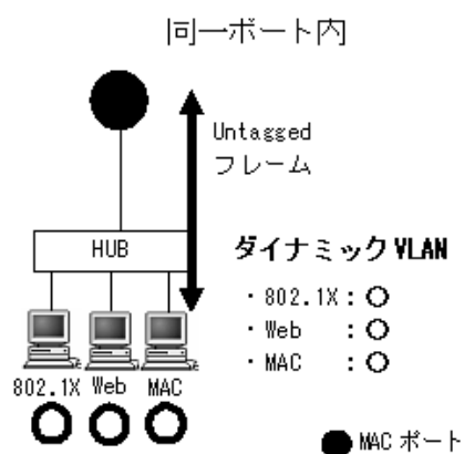
図 5-27 同一ポート内ダイナミック VLAN モードの共存例
