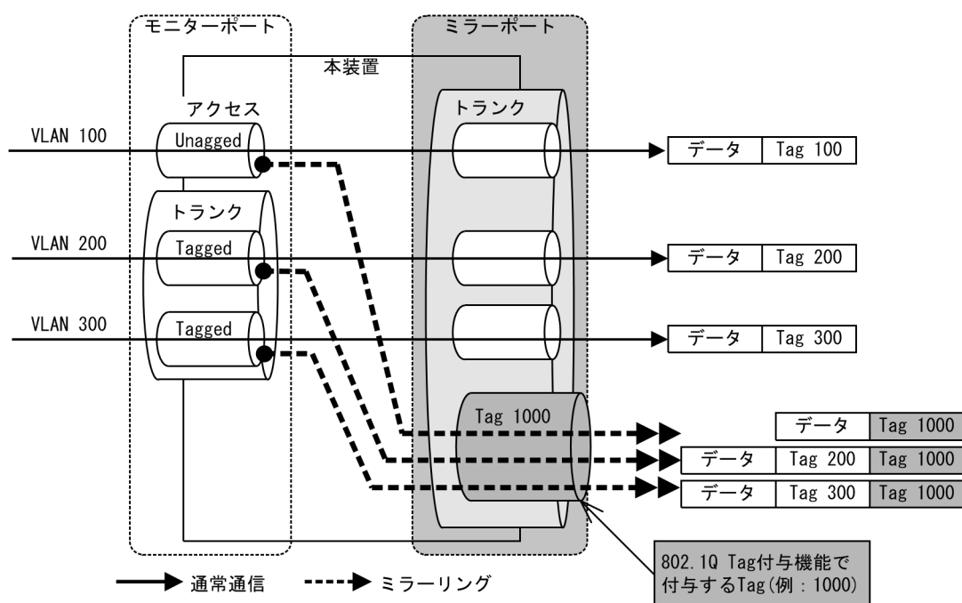
図 29-6 802.1Q Tag 付与機能の概要
