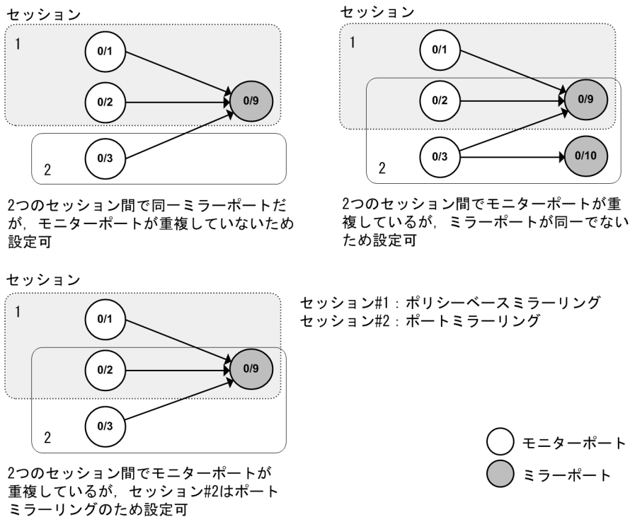
図 30-3 設定可能な組み合わせ
