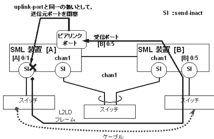
図 20-17 隣接装置の単独ポートで受信した L2 ループ検知フレームの動作
