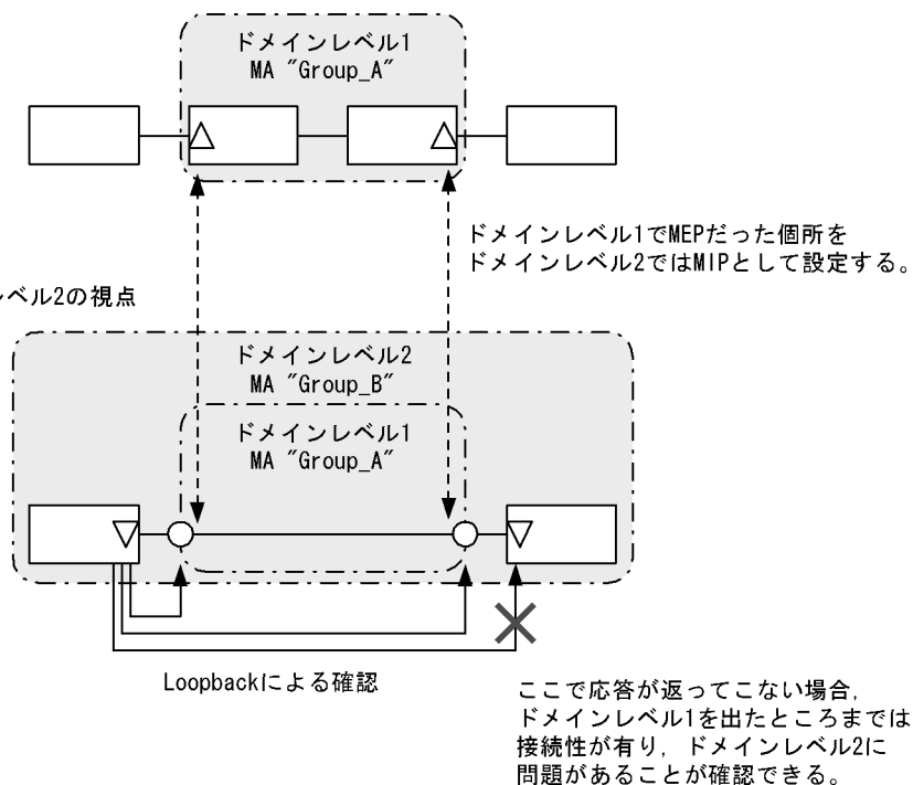
図 24-9 ドメインレベル1とドメインレベル2の階層構造の例
