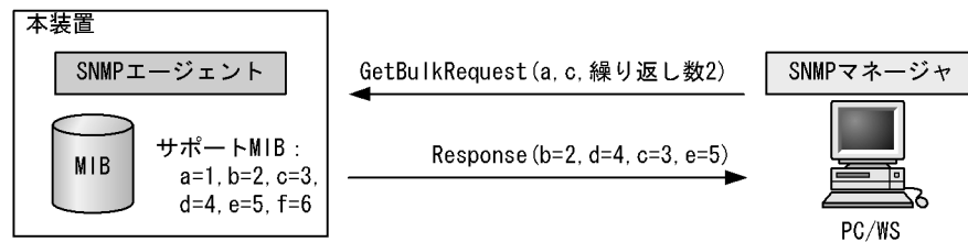
図 25-18 GetBulkRequest オペレーション
