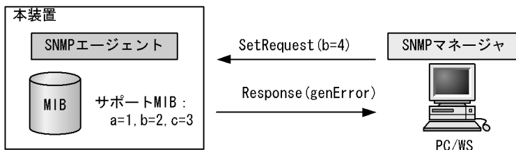
図 25-22 装置の状態によって設定できない場合の SetRequest オペレーション
