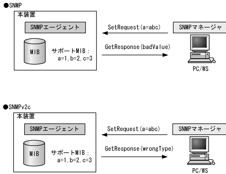
図 25-13 設定値のタイプが正しくない場合の SetRequest オペレーション例
