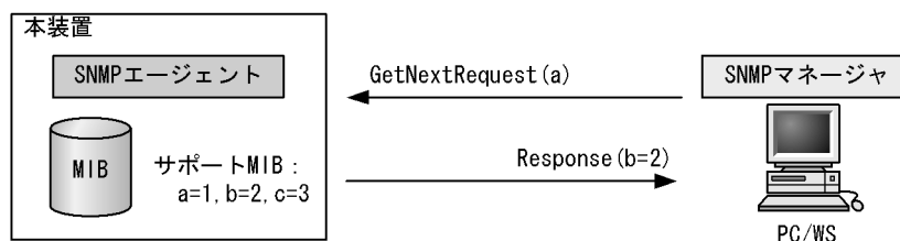
図 25-17 GetNextRequest オペレーション
