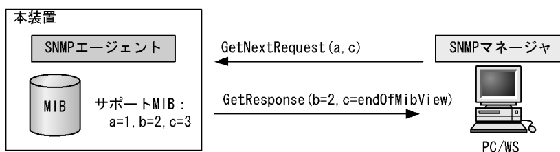
図 25-9 GetNextRequest オペレーション (SNMPv2C)
