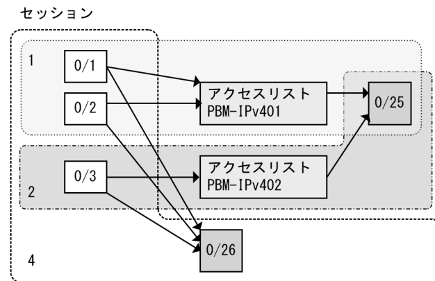
図 30-6 ポートミラーリングと併用
