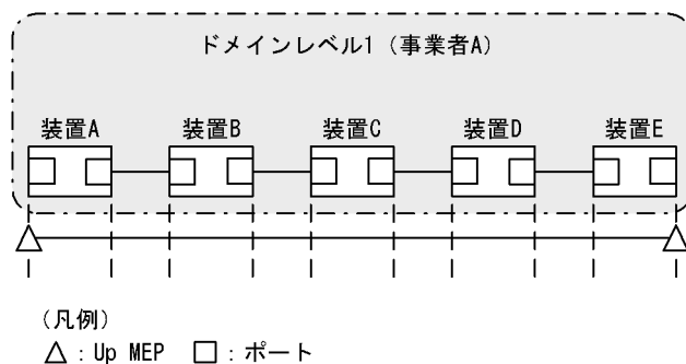
図 24-16 MIP 設定前の構成例
