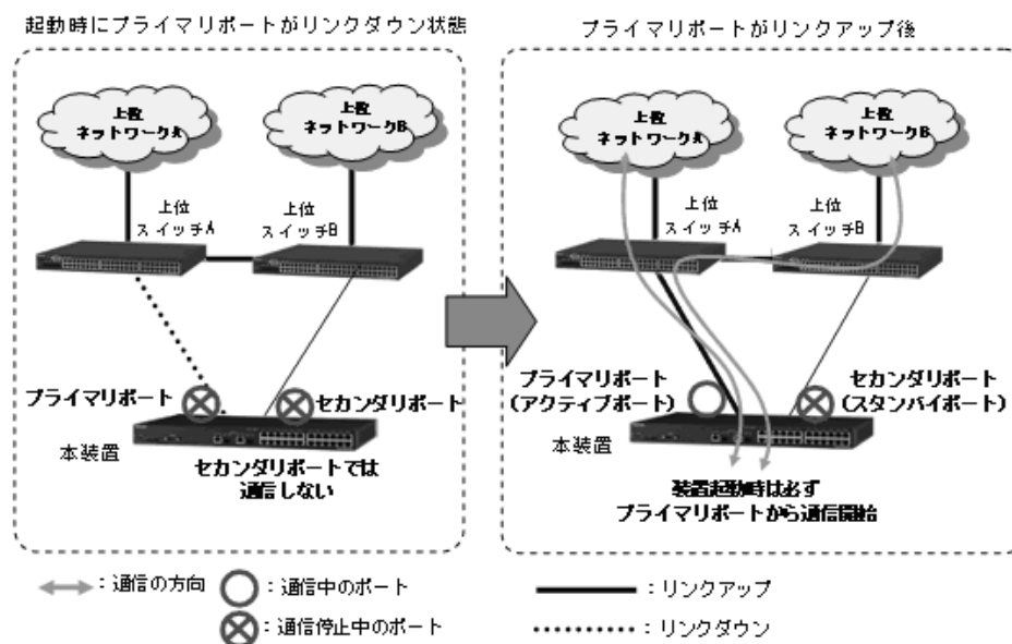
図 19-7 装置起動時のアクティブポート固定機能有効時の動作
