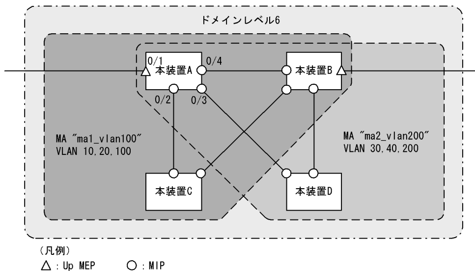
図 24-32 CFM の設定例（同ドメイン、複数 MA）
