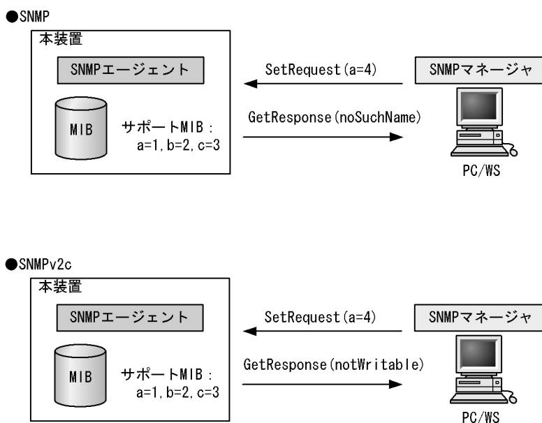
図 25-12 MIB 変数が読み出し専用の場合の SetRequest オペレーション
