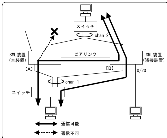
図 20-8 SML ChGr 障害時の動作
