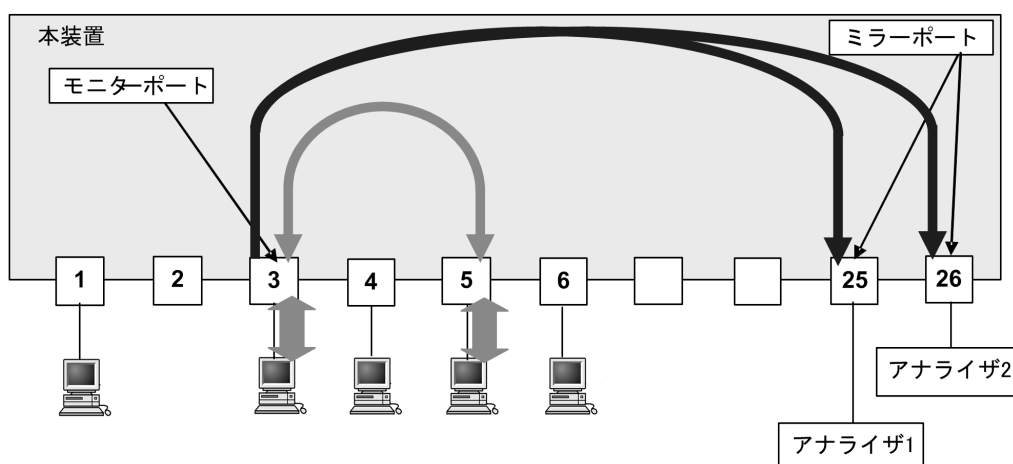
図 29-4 1 対 2 のミラーリング
