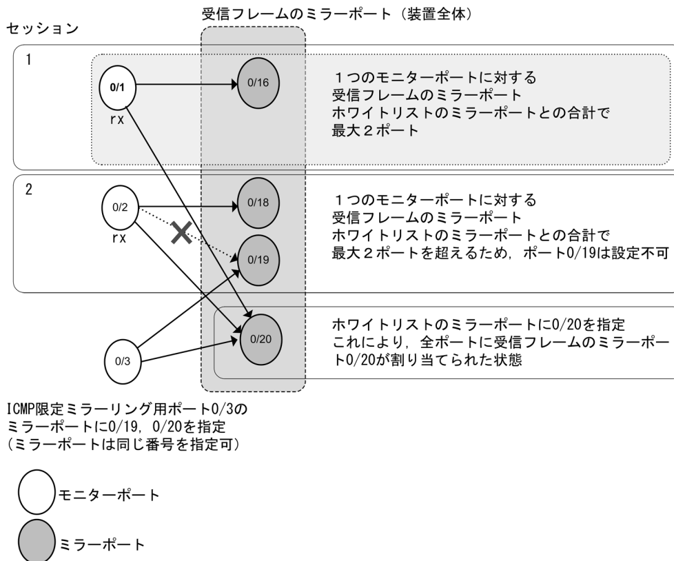
図 29-8 受信フレームのミラーポート数（ホワイトリスト機能、ICMP 限定ミラーリング機能のミラー設定有）
