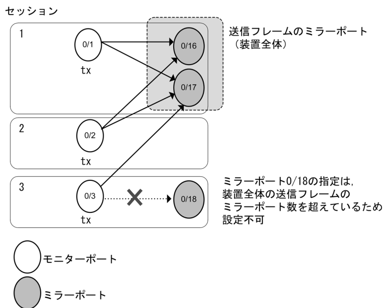
図 29-9 送信フレームのミラーポート数
