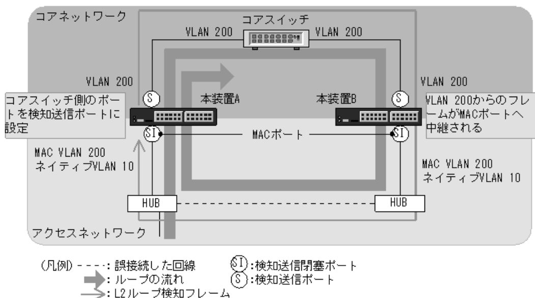
図 23-4 ループ検知可能な構成
