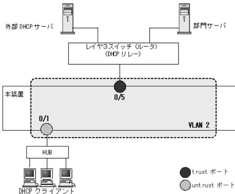
図 15-17 レイヤ3スイッチ経由の構成例
