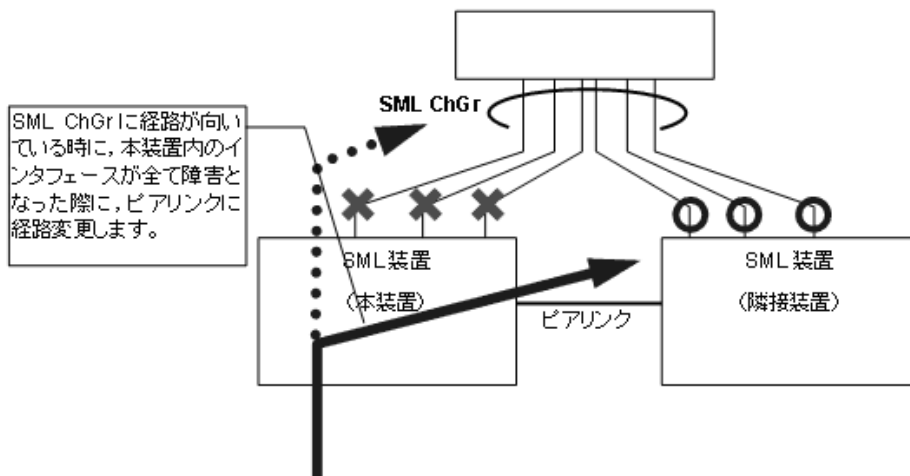
図 20-13 ピアリンクへの経路切り替え
