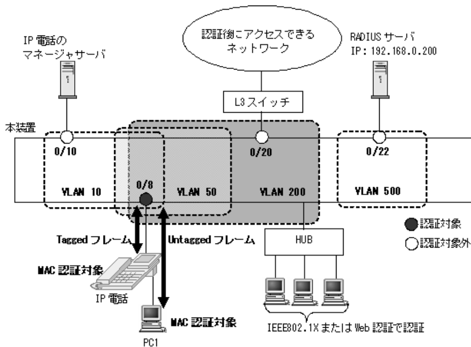
図 5-29 MAC ポートで Tagged フレームを認証する構成例
