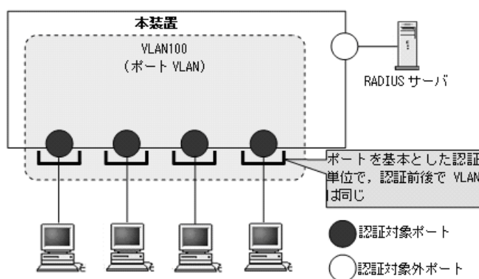
図 6-3 ポート単位認証（静的）の構成例
