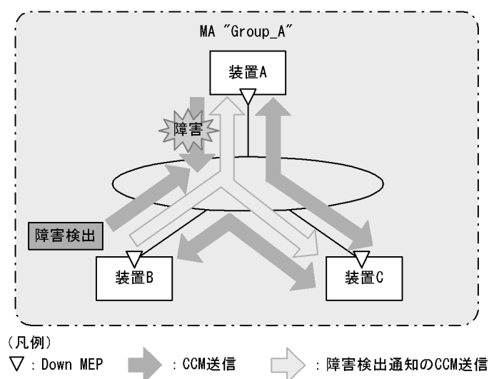
図 24-20 障害を全 MEP に通知
