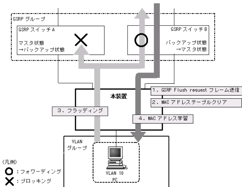
図 18-2 GSRP Flush request フレームによる切り替え制御の概要
