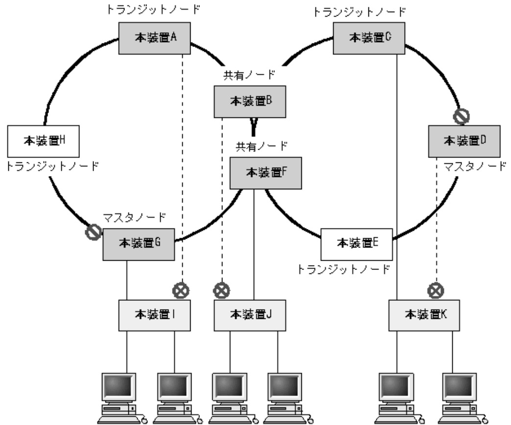
図 26-2 Ring Protocol とスパニングツリーの併用例（マルチリング構成）
