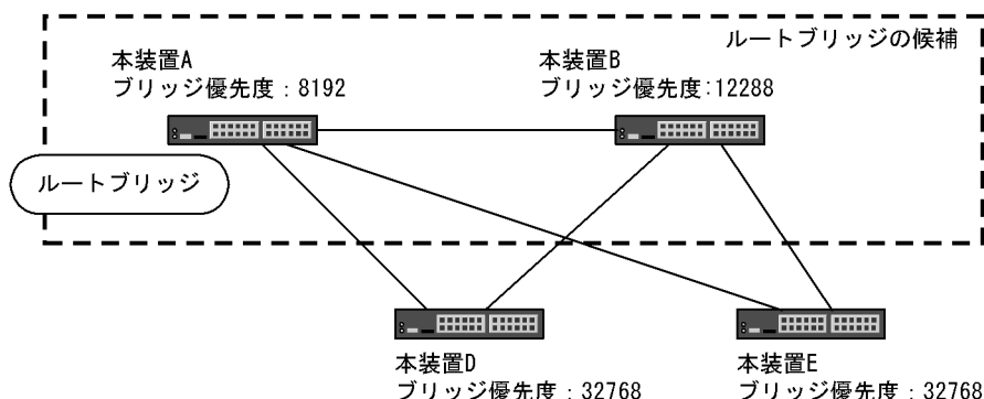
図 23-18 本装置 A、本装置 B をルートブリッジの候補として運用
