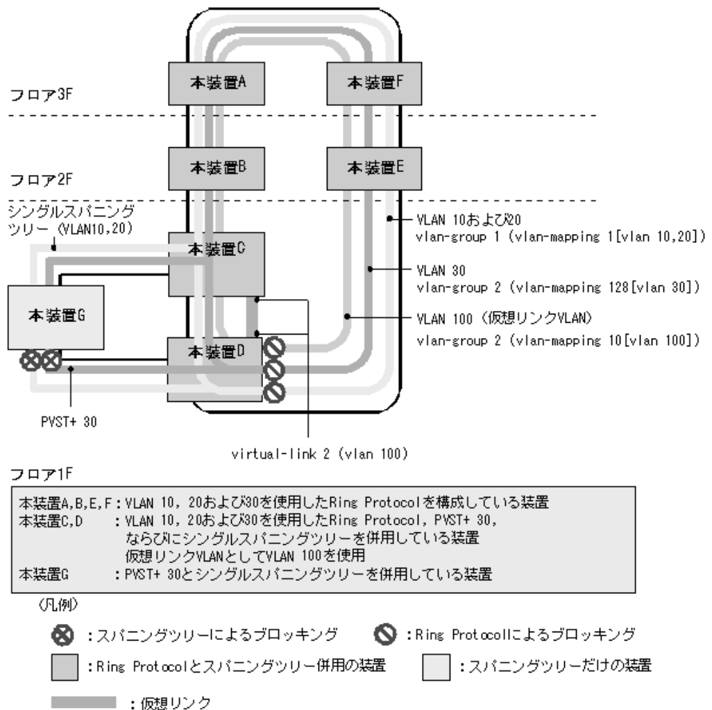
図 26-6 シングルスパニングツリー, PVST+, および Ring Protocol の共存構成
