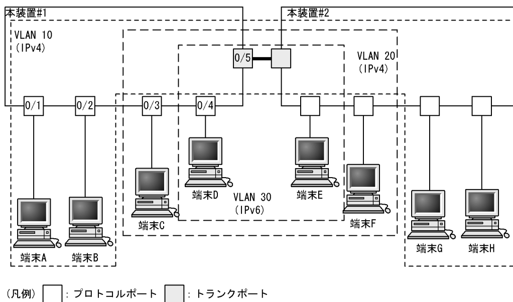
図 21-7 プロトコル VLAN の設定例
