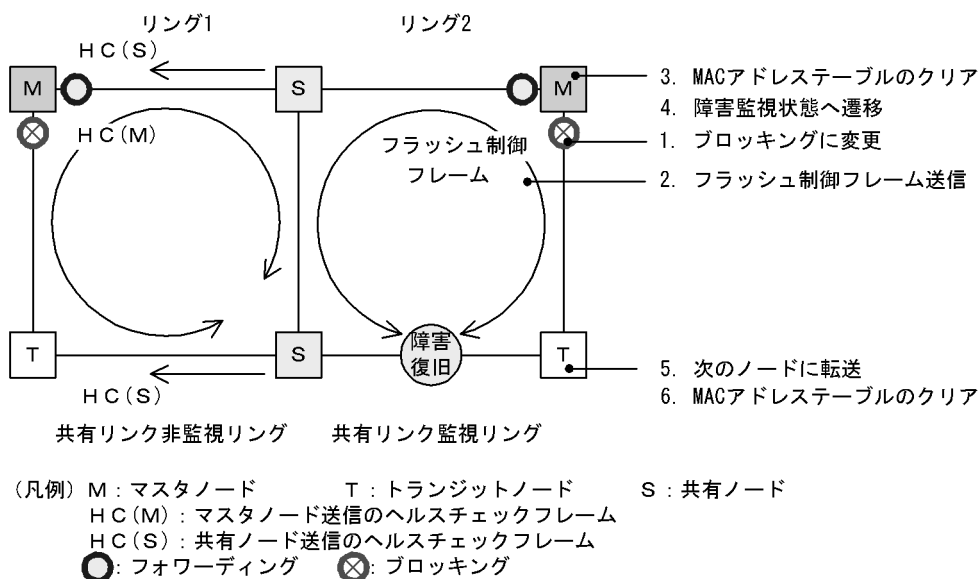
図 24-20 共有リンク監視リングでの共有リンク以外のリング障害復旧時の動作
