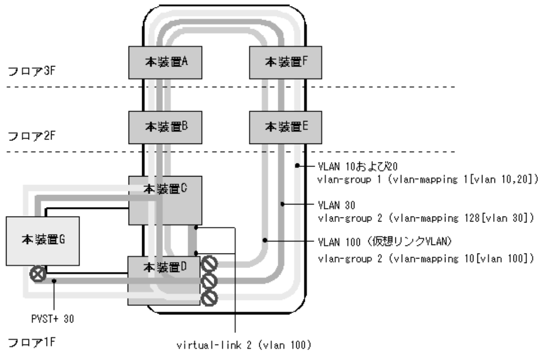
図 26-4 PVST+ と Ring Protocol の共存構成
