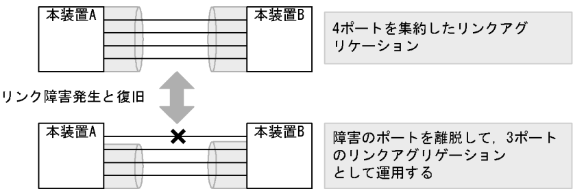
図 18-1 リンクアグリゲーションの構成例
