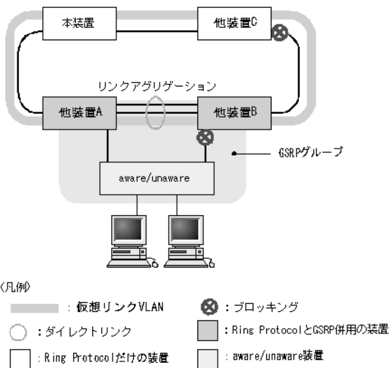
図 26-9 Ring Protocol と GSRP の併用例と本装置の位置づけ (ダイレクトリンクをリングネットワークで使用する場合)
