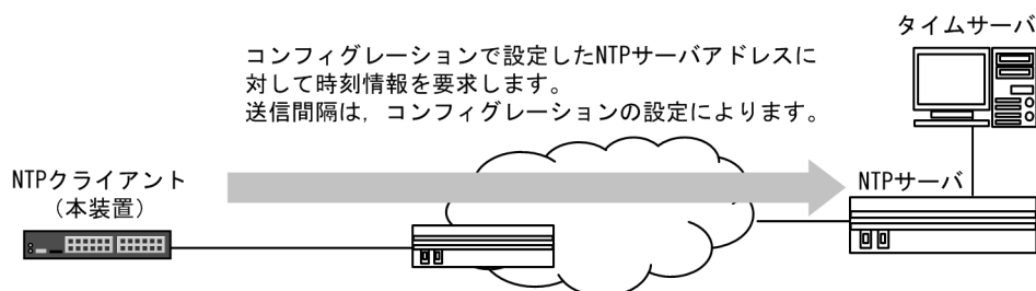
図 11-1 Unicast モードによる時刻情報取得図 (プライマリ設定時)
