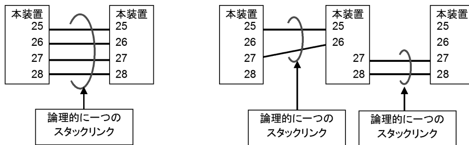
図 7-4 24 ポートモデルのスタックポート接続
