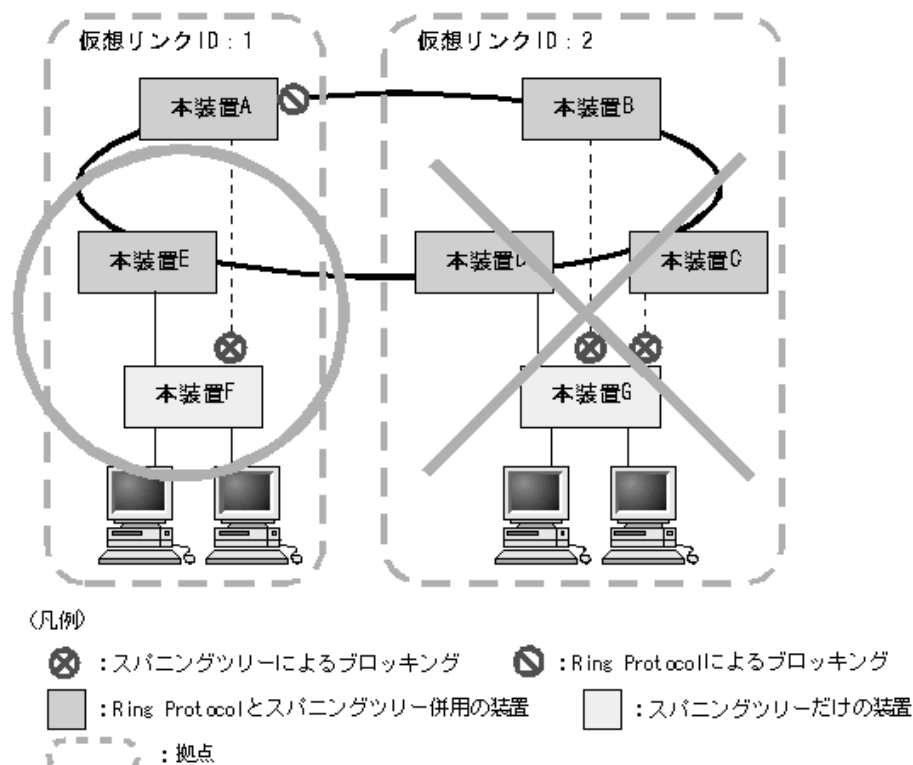
図 26-8 仮想リンクの禁止構成
