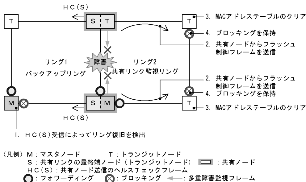
図 24-28 バックアップリングからの切り戻し動作
