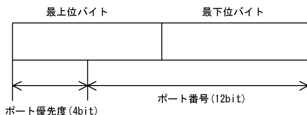
図 23-3 ポート識別子
