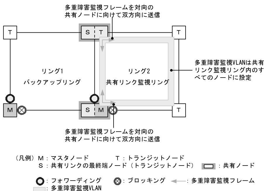
図 24-23 多重障害監視の動作概要
