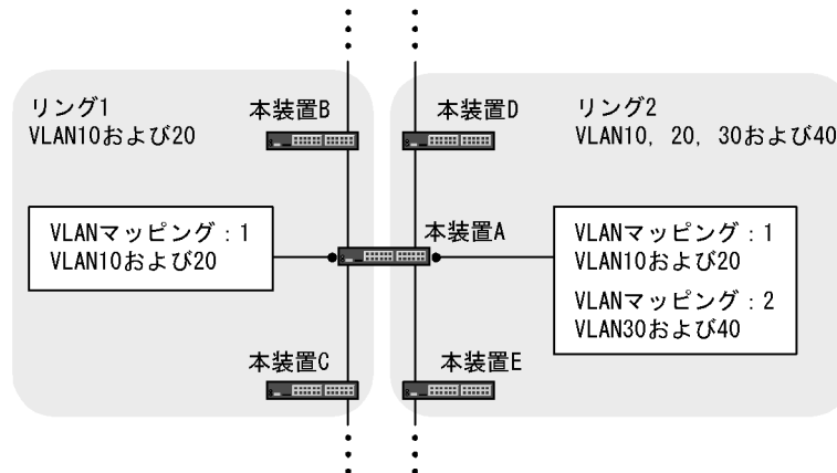
図 24-30 リングごとの VLAN マッピングの割り当て例
