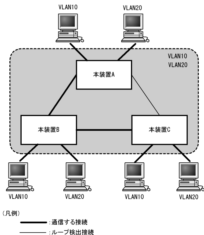
図 23-10 シングルスパニングツリーによるネットワーク構成
