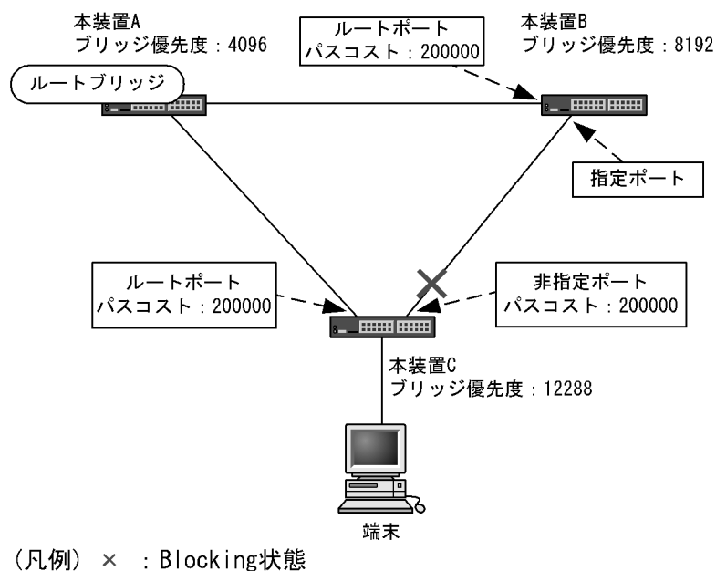
図 23-4 スパニングツリーのトポロジー設計
