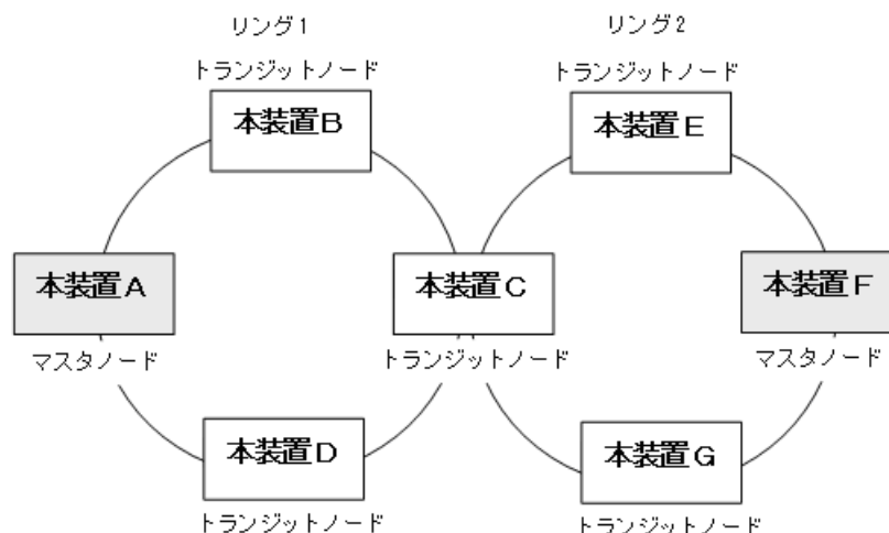
図 24-5 マルチリング構成
