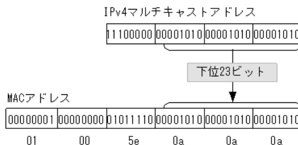
図 27-3 IPv4 マルチキャストアドレスと MAC アドレスの対応
