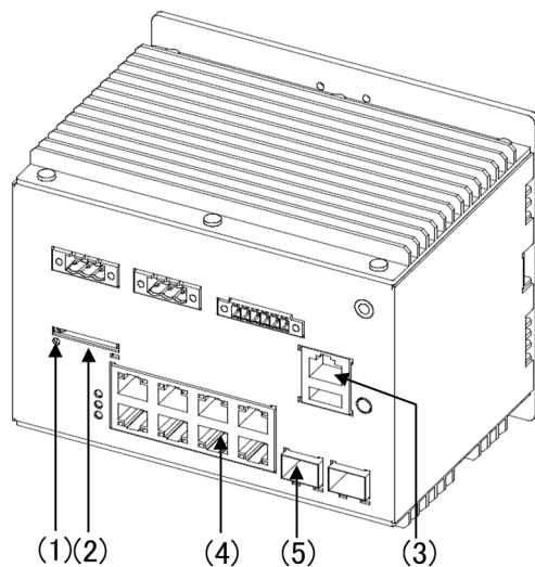
図 2-8 外観図 (08TC1)
