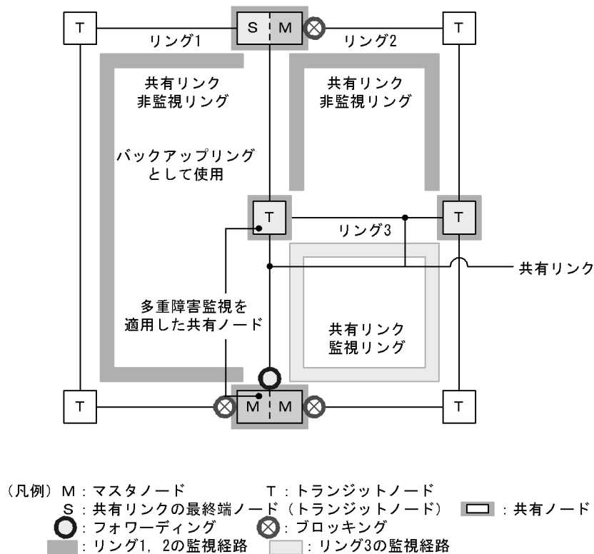
図 24-38 共有リンク内の共有ノードで多重障害を監視する構成
