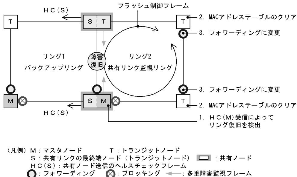
図 24-29 共有リンク障害復旧時の動作
