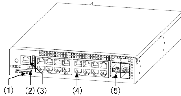
図 2-9 外観図 (16P4X)
