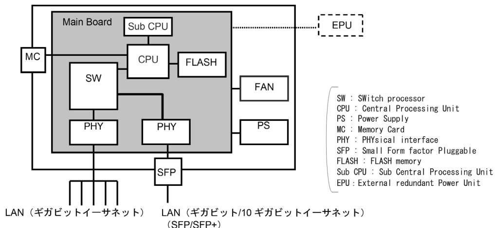
図 2-12 ハードウェアの構成 (24T4X, 48T2X)
