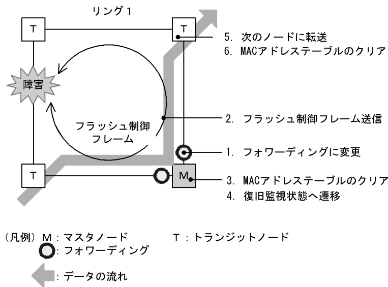
図 24-9 リング障害時の動作
