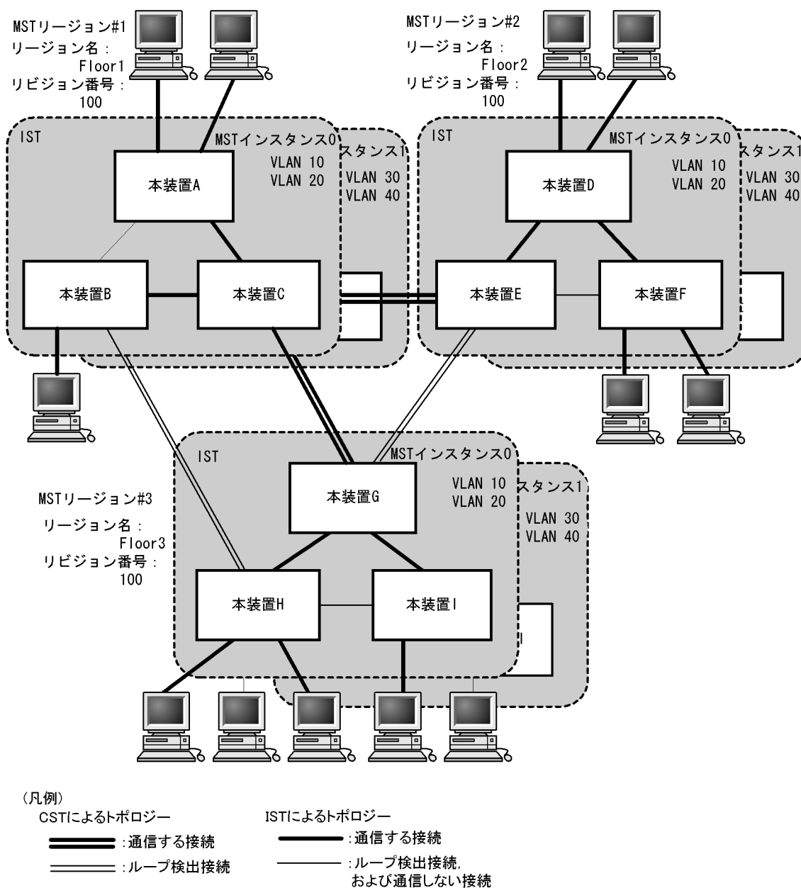
図 23-15 MST リージョンによるネットワーク構成
