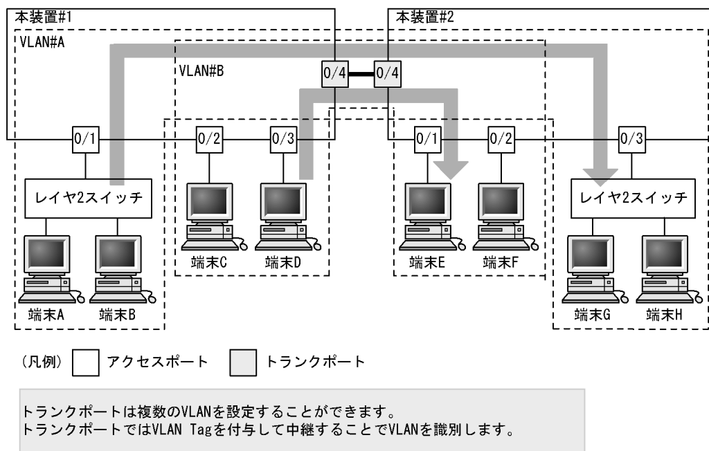
図 21-3 ポート VLAN の構成例
