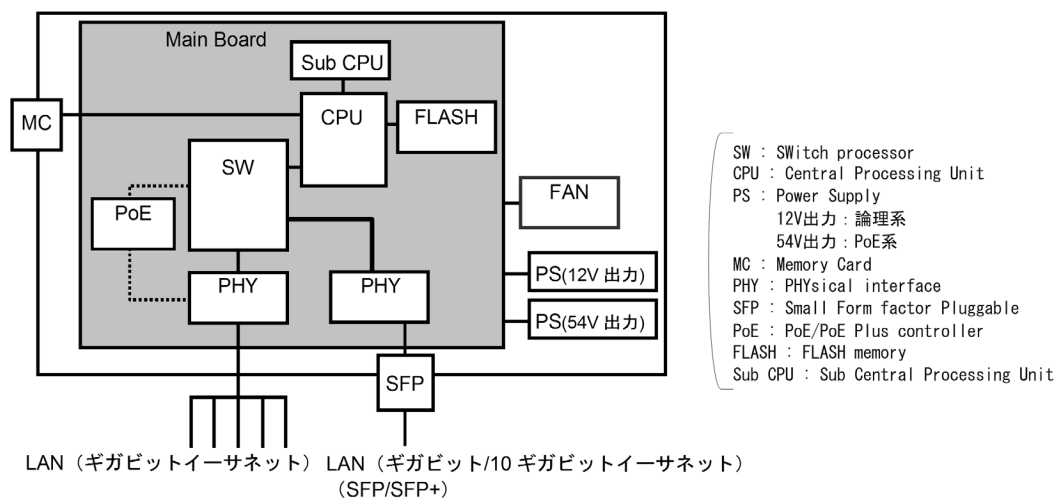
図 2-14 ハードウェアの構成 (48P2X)
