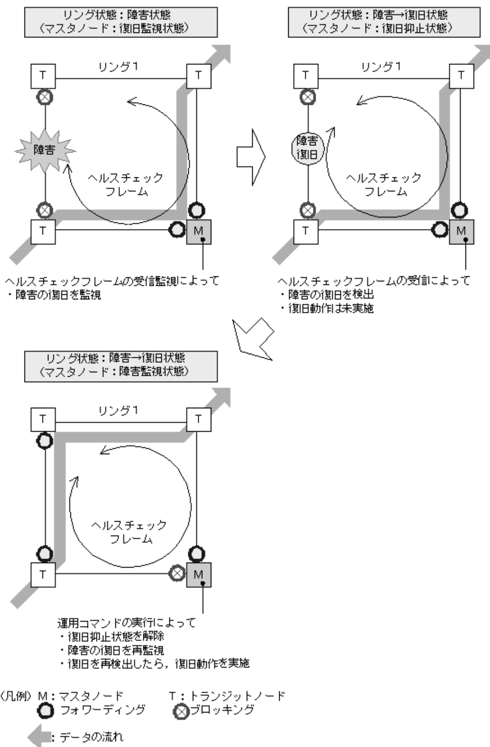
図 24-11 運用コマンドの実行によって経路切り戻し抑止を解除した場合の動作
