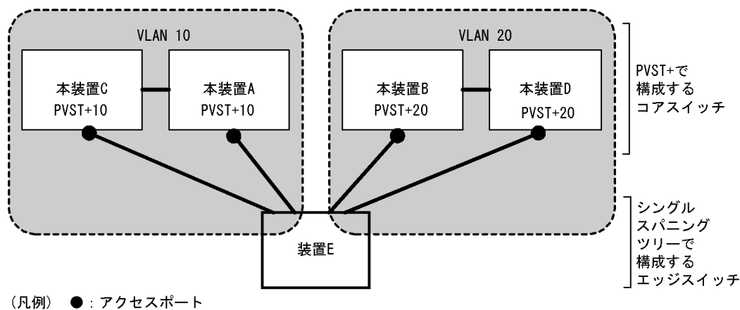
図 23-8 シングルスパニングツリーとの禁止構成例
