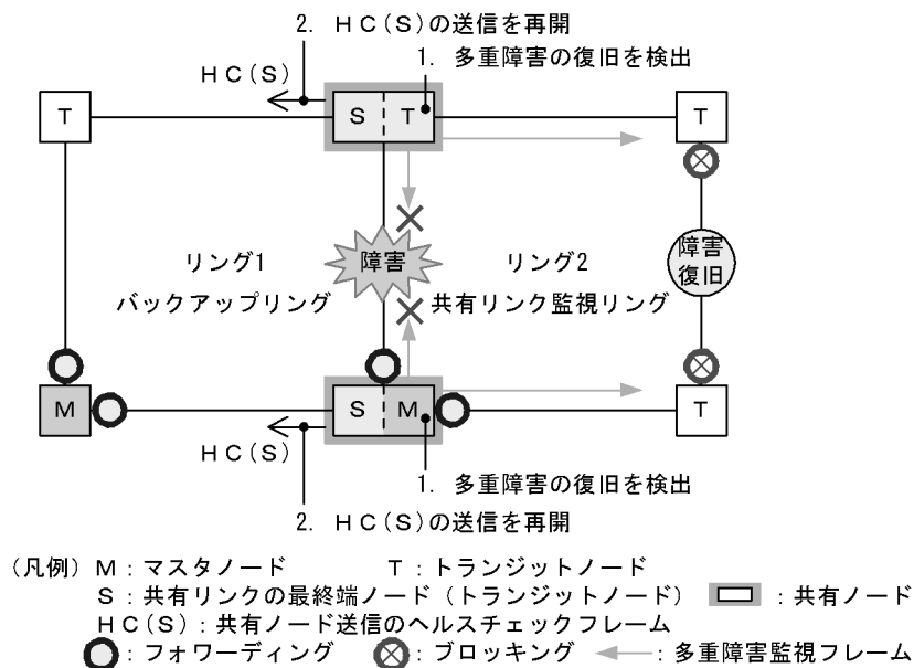
図 24-27 多重障害からの一部復旧時の動作
