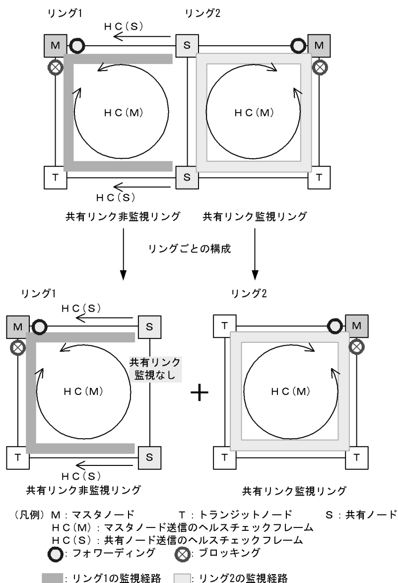
図 24-12 リング正常時の状態
