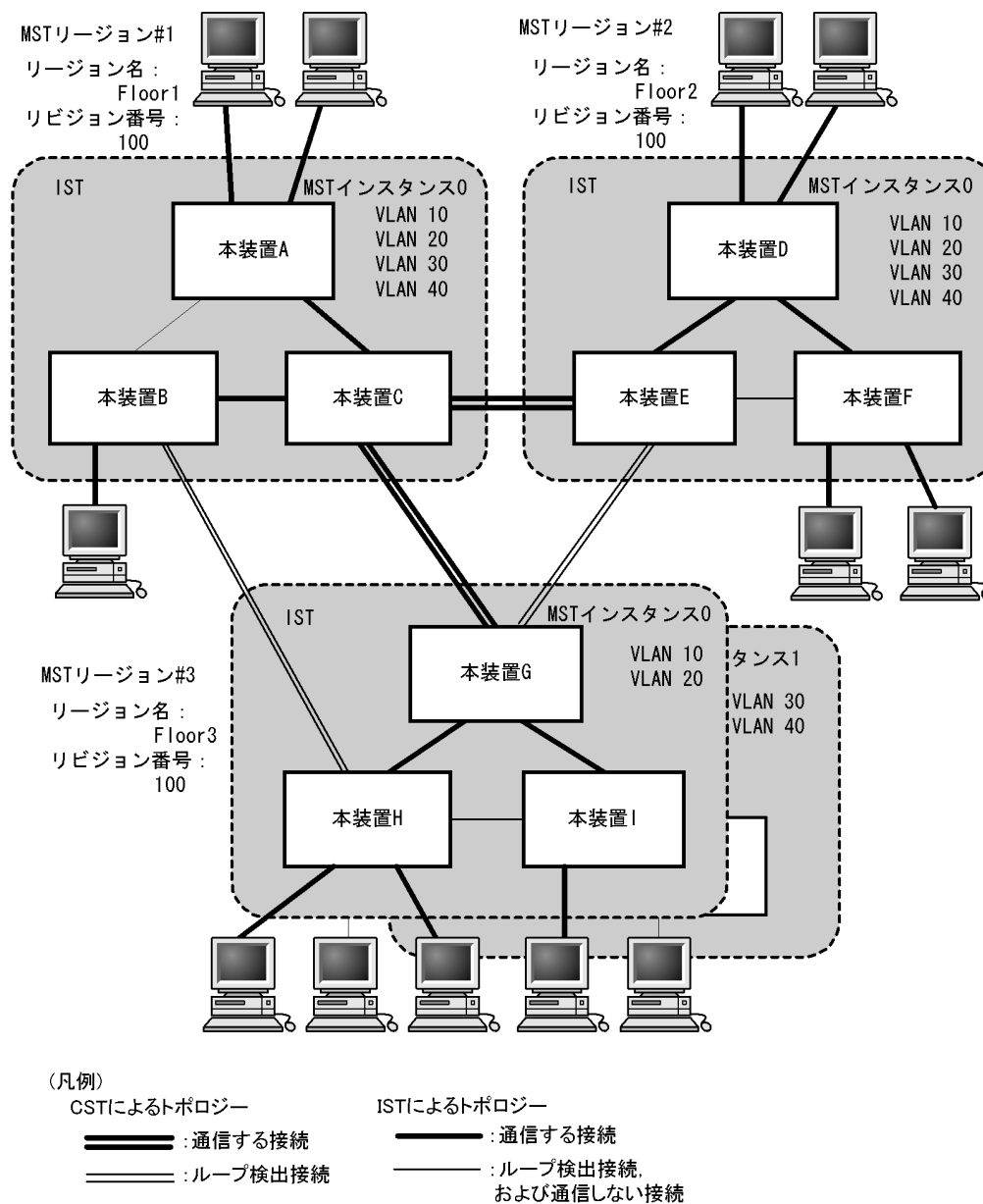
図 23-13 マルチプルスパニングツリー概要
