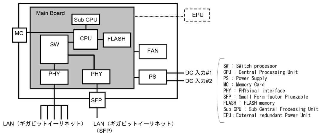
図 2-15 ハードウェアの構成 (48TD)
