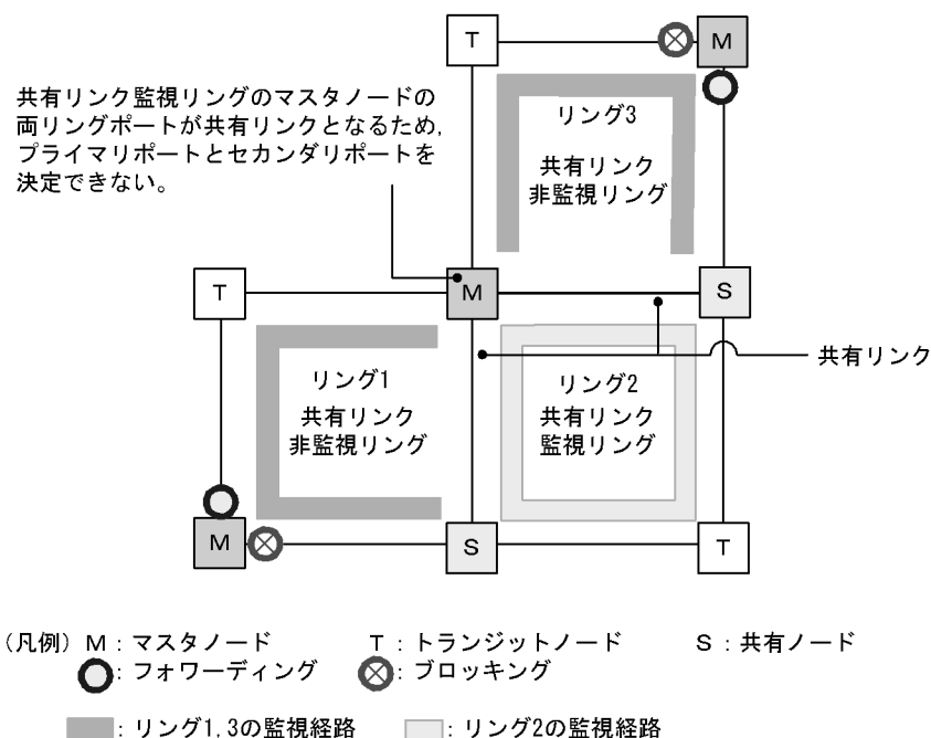
図 24-36 マスタノードのプライマリポートが決定できない構成
