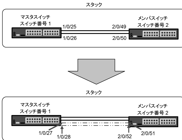
図 8-5 スタックリンクの追加
