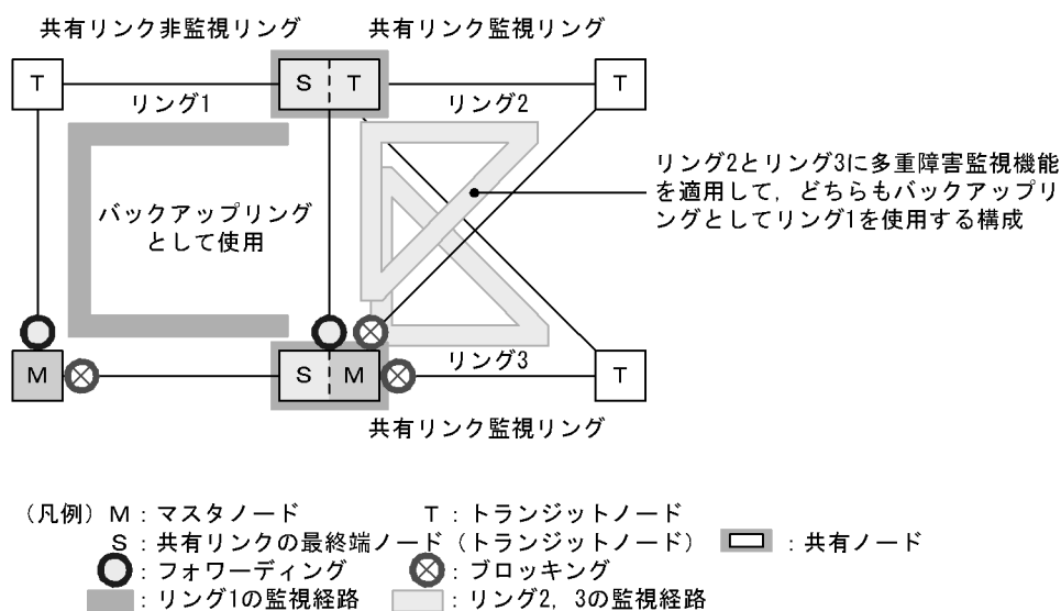
図 24-37 複数の共有リンク監視リングが同じバックアップリングを使用する構成
