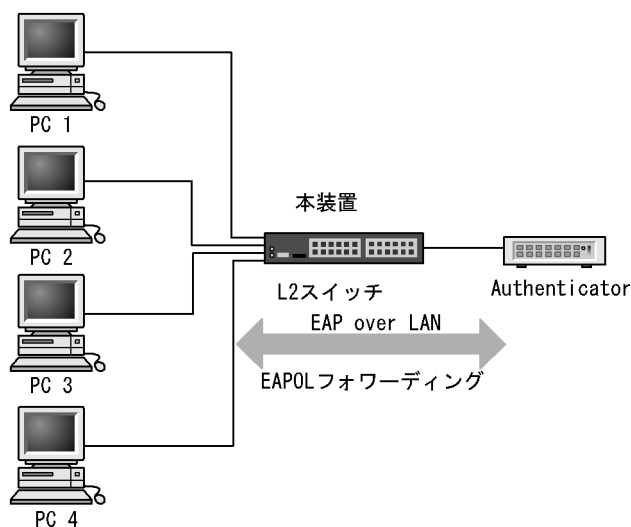
図 22-4 EAPOL フォワーディング機能の適用例
