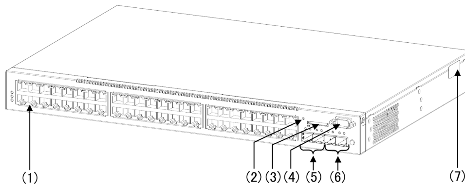
図 2-4 外観図 (48T2X)
