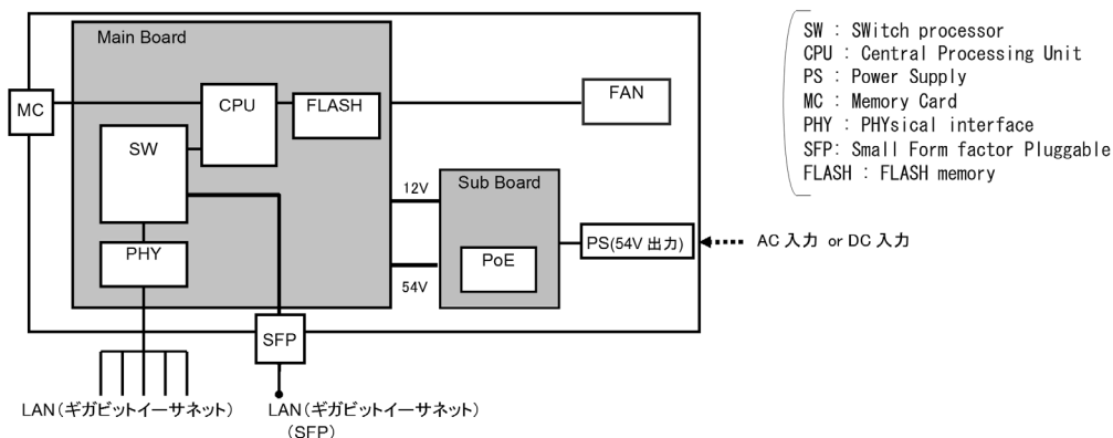
図 2-18 ハードウェアの構成 (08P, 08PD1, 08PD2)
