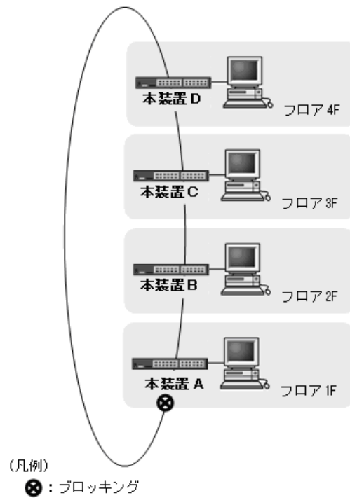
図 24-2 Ring Protocol の適用例（その 1）
