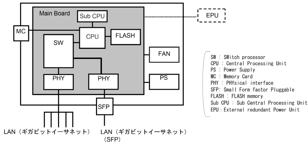
図 2-13 ハードウェアの構成 (48T)
