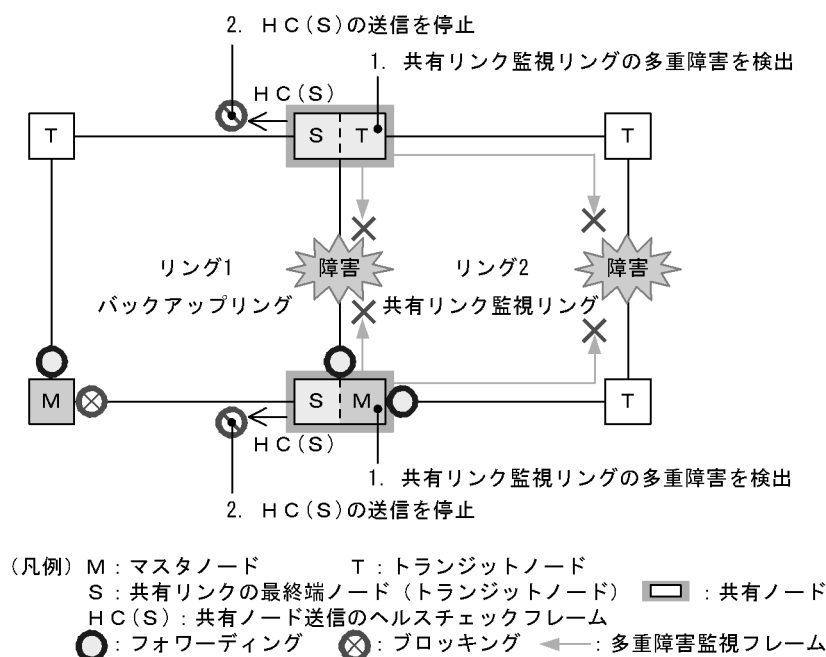
図 24-25 多重障害発生時の動作
