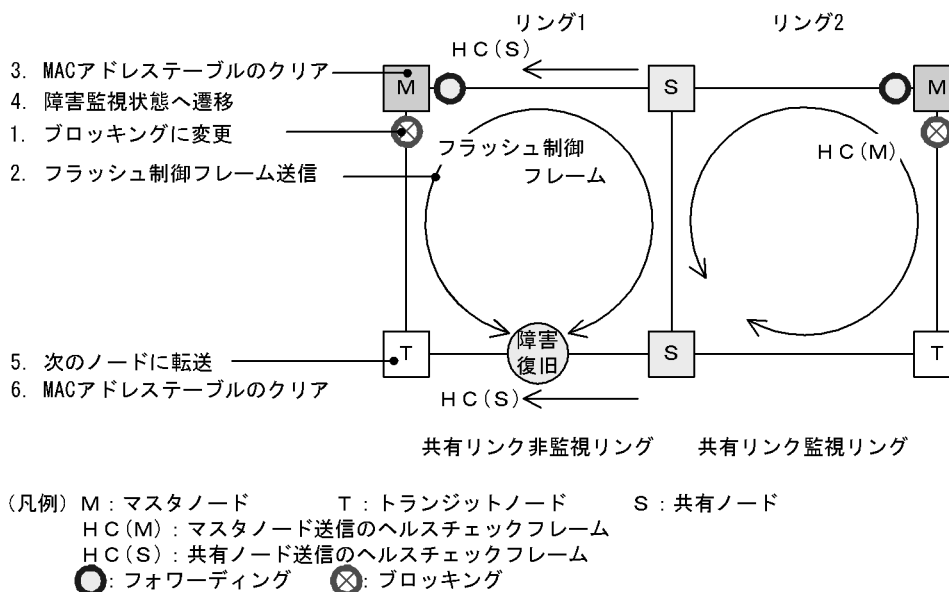
図 24-18 共有リンク非監視リングでの共有リンク以外のリング障害復旧時の動作
