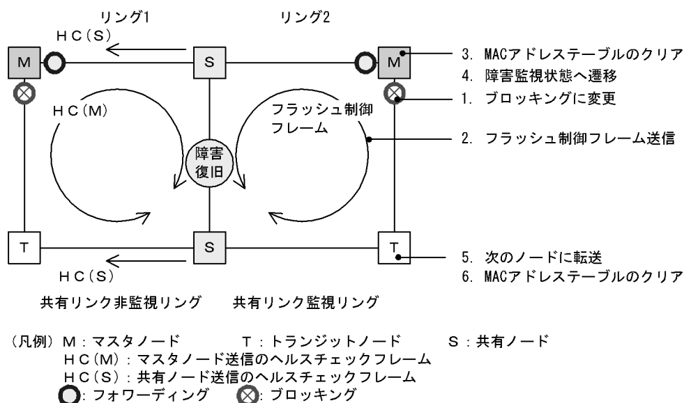
図 24-16 共有リンク復旧時の動作
