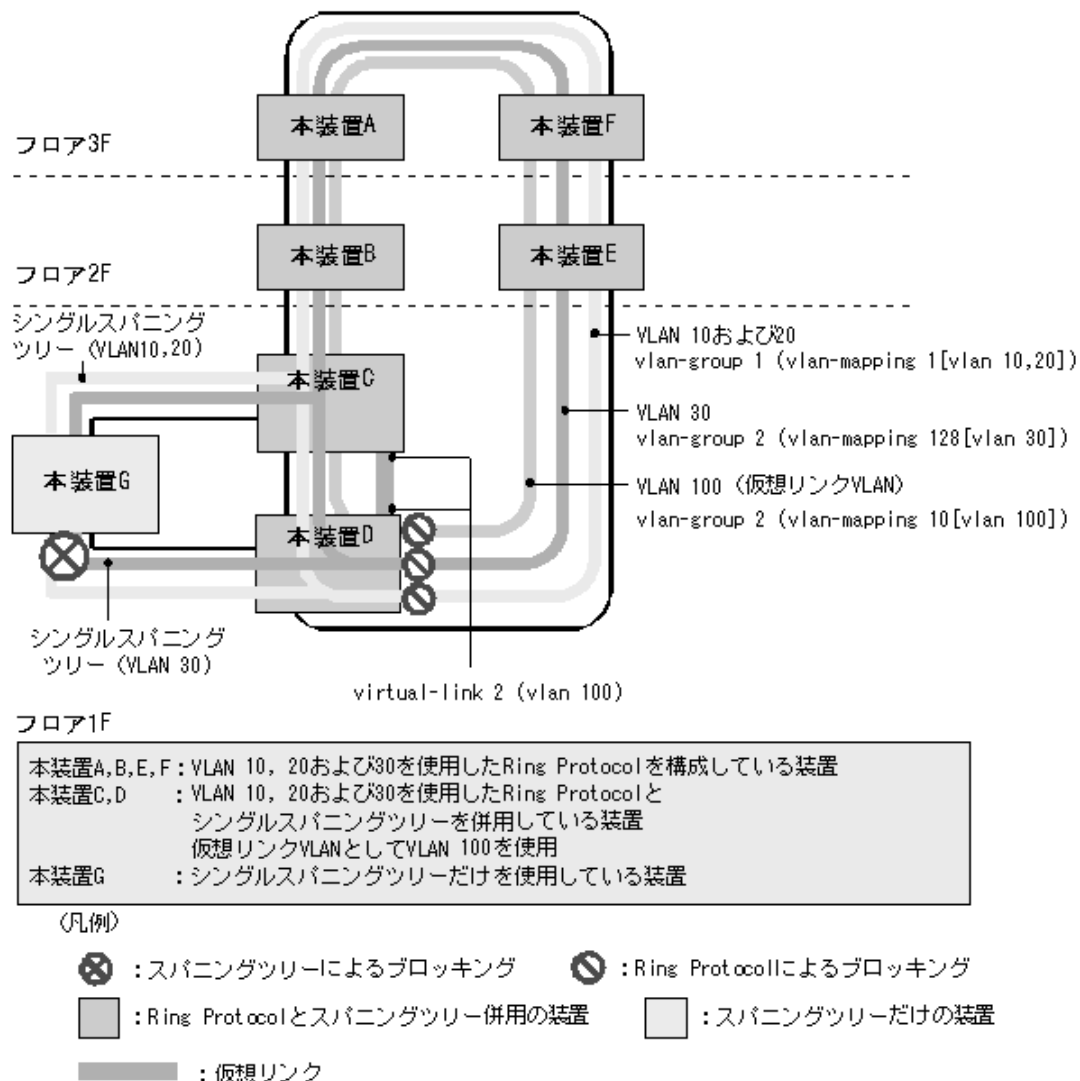
図 26-5 シングルスパニングツリーと Ring Protocol の共存構成
