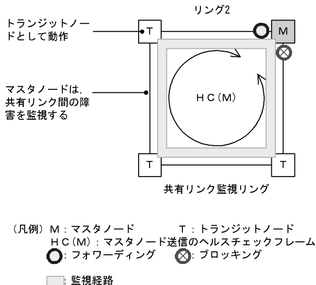
図 24-14 共有リンク監視リングでの正常時の動作
