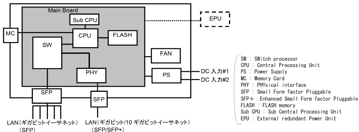
図 2-17 ハードウェアの構成 (24S4XD)
