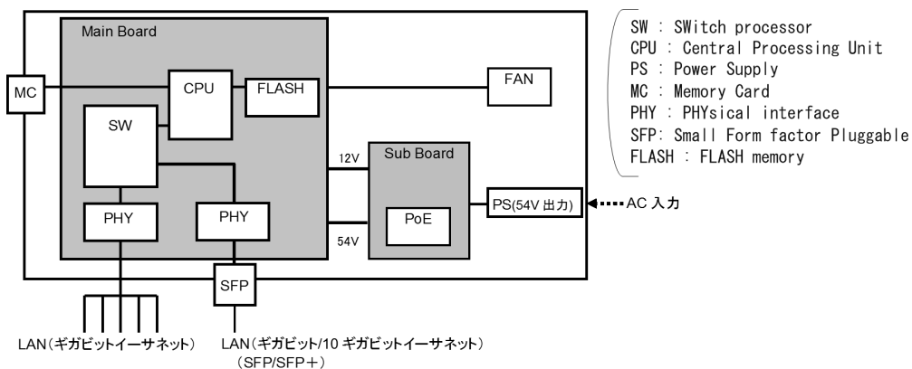
図 2-20 ハードウェアの構成 (16P4X)
