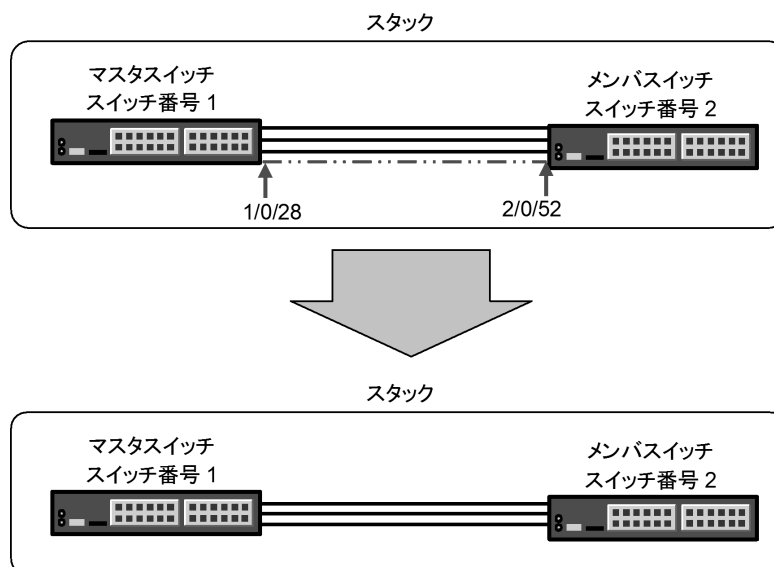
図 8-6 スタックリンクの削除
