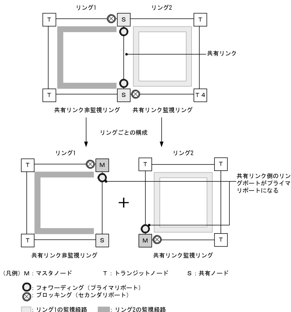
図 24-31 共有リンクをマスタノードとした場合のポート状態
