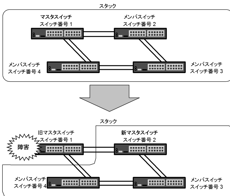
図 7-11 マスタスイッチ障害時
