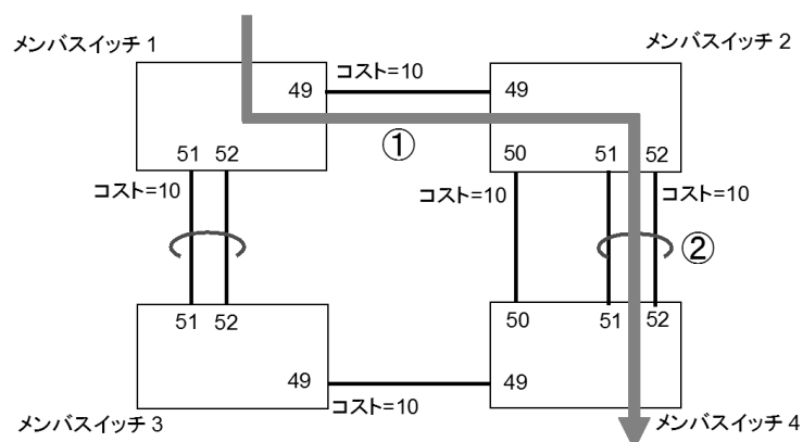
図 7-8 全経路が同一コストの場合
