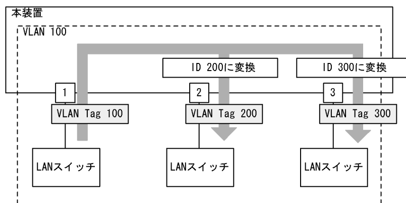
図 22-2 Tag 変換の構成例
