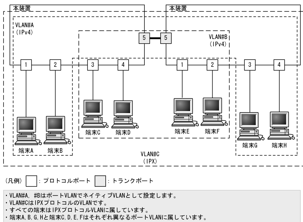
図 21-6 プロトコルポートでネイティブ VLAN を使用する構成例
