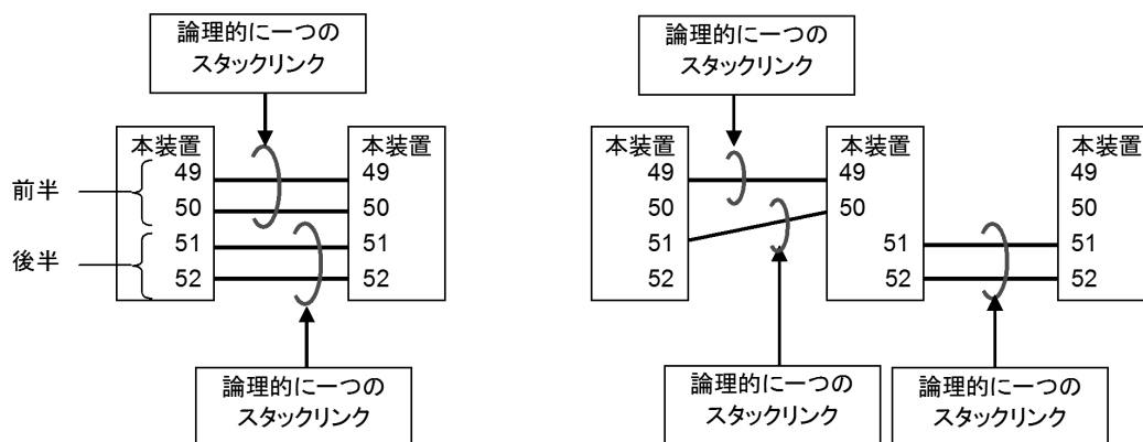
図 7-5 48 ポートモデルのスタックポート接続
