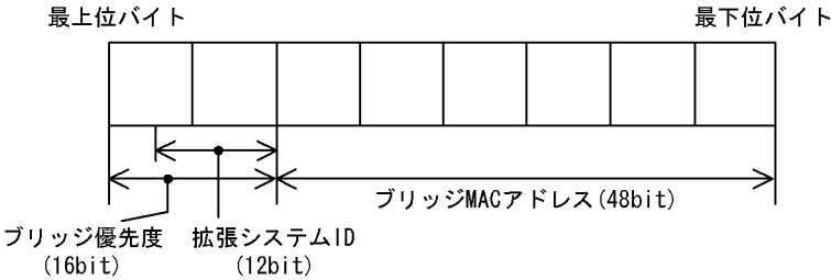
図 23-2 ブリッジ識別子
