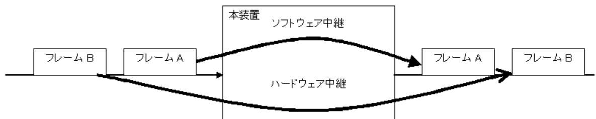
図 17-3 ソフトウェア中継によるフレームの入れ替わり
