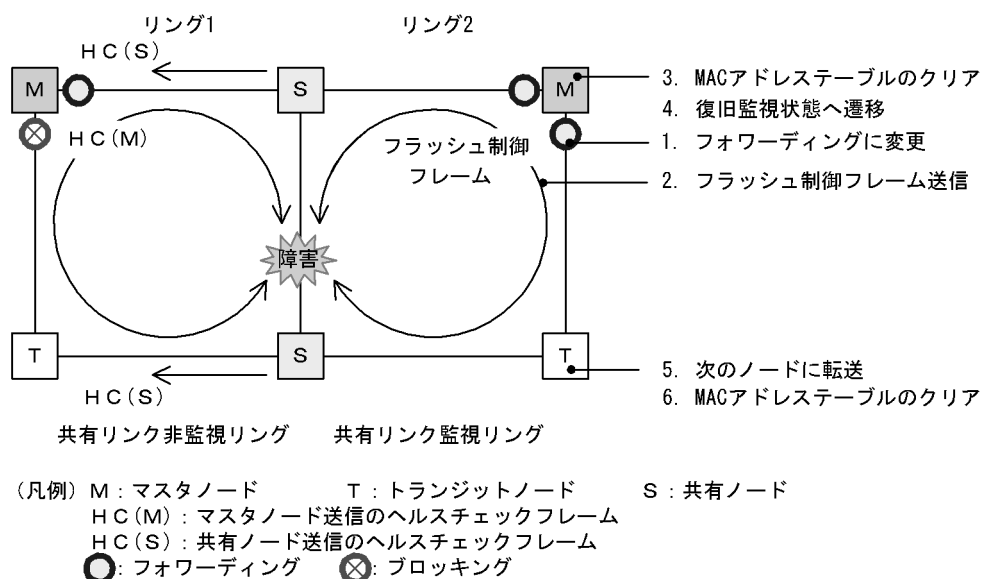
図 24-15 共有リンク障害時の動作
