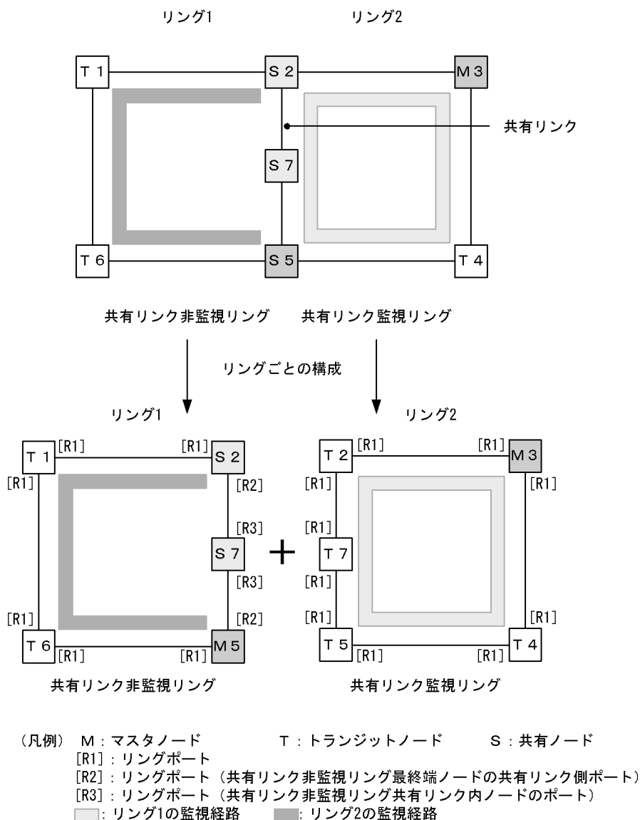
図 25-4 共有リンクありのマルチリング構成（拡張構成）
