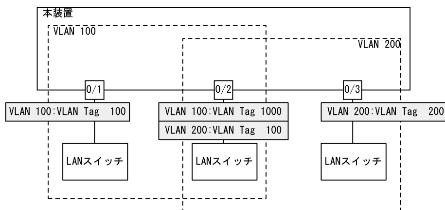
図 22-3 Tag 変換の設定例
