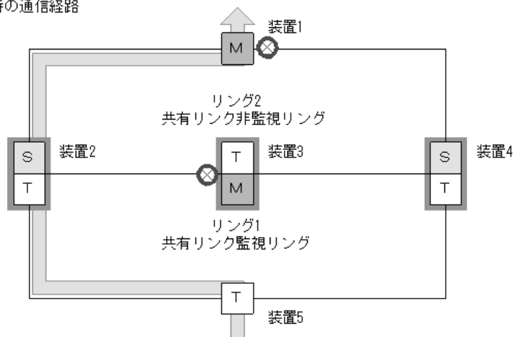
図 24-39 マスタノードの両リングポートが共有リンクとなる構成例
