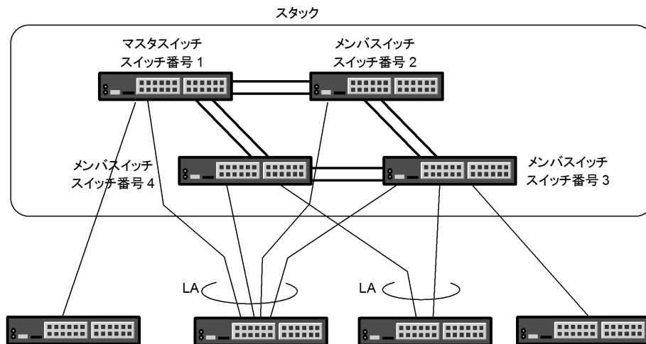
図 7-3 メンバスイッチ 4 台でのスタック構成例
