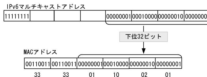
図 27-4 IPv6 マルチキャストアドレスと MAC アドレスの対応
