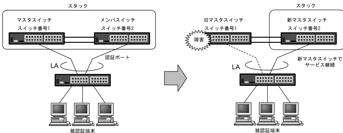
図 7-2 スタック動作時の認証機能
