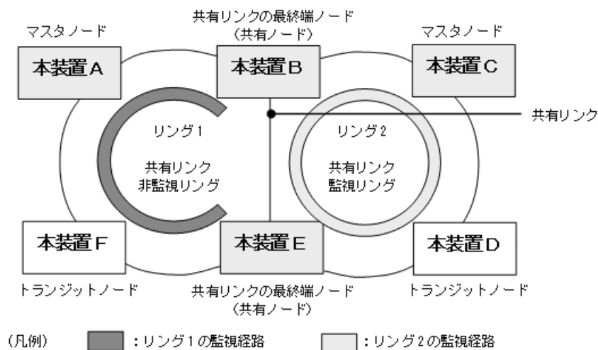
図 24-6 共有リンクありのマルチリング構成
