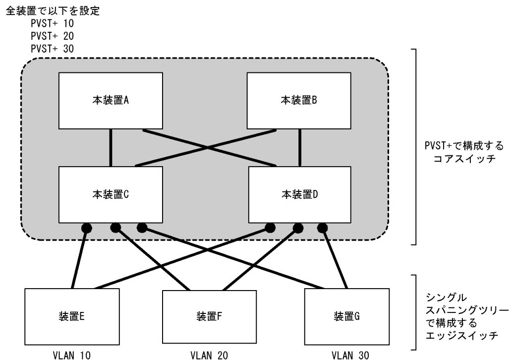
図 23-7 シングルスパニングツリーとの接続
