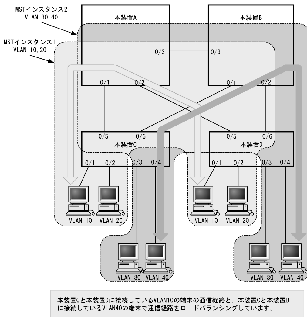
図 23-14 マルチプルスパニングツリーのロードバランシング構成
