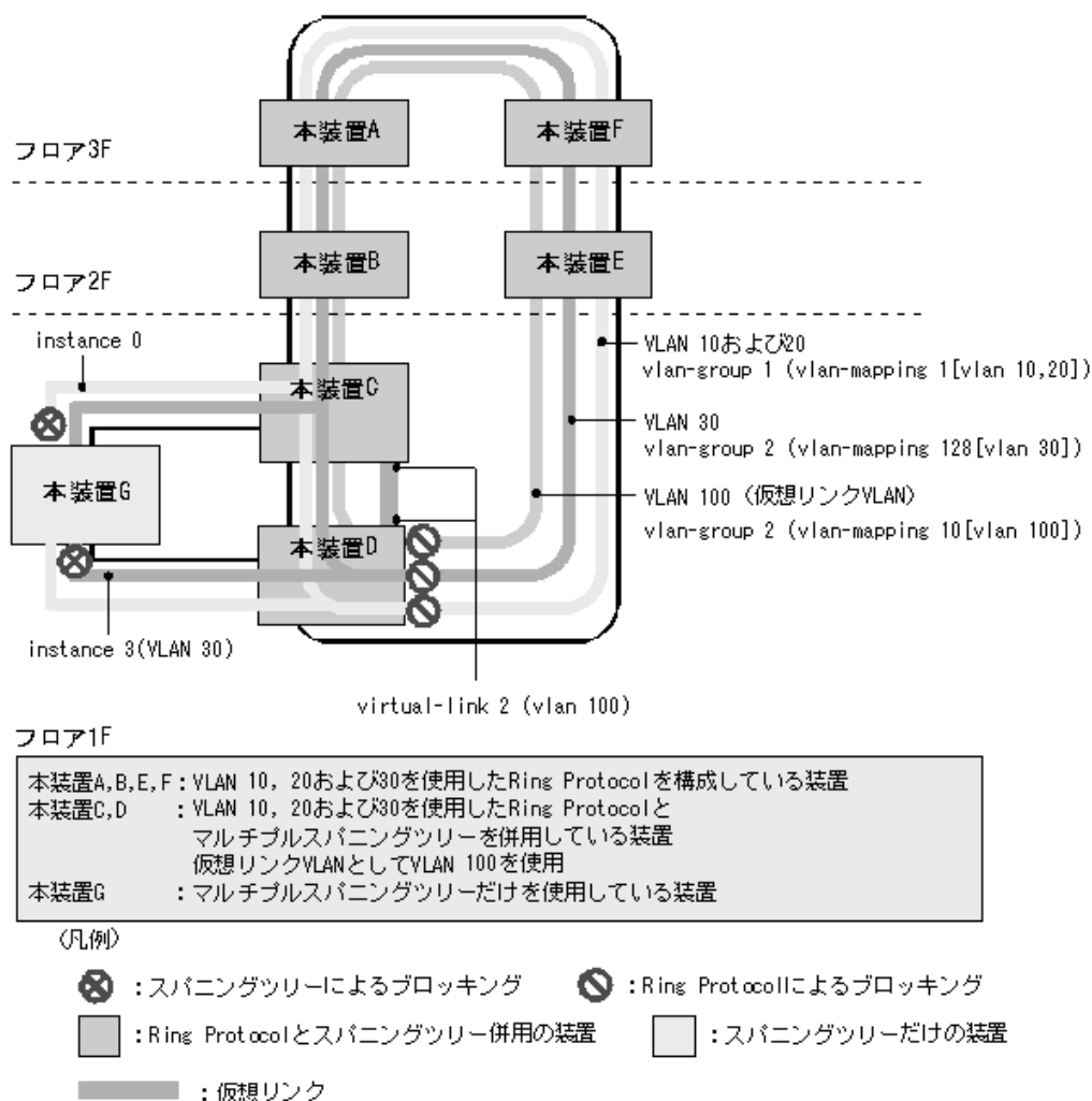
図 26-7 マルチプルスパニングツリーと Ring Protocol の共存構成
