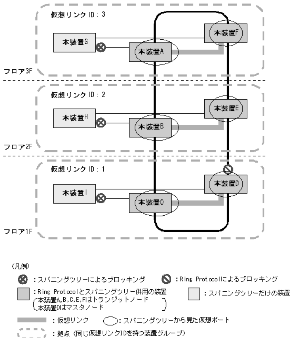
図 26-3 仮想リンクの概要
