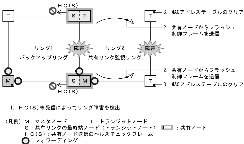
図 24-26 バックアップリングへの切り替え動作
