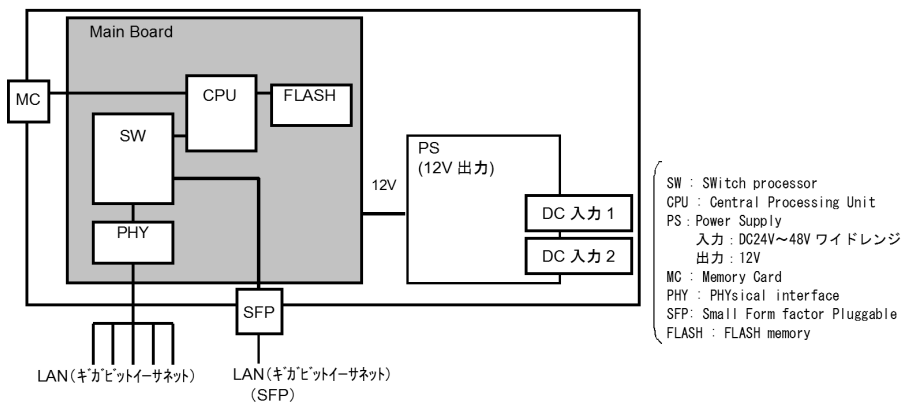
図 2-19 ハードウェアの構成 (08TC1)
