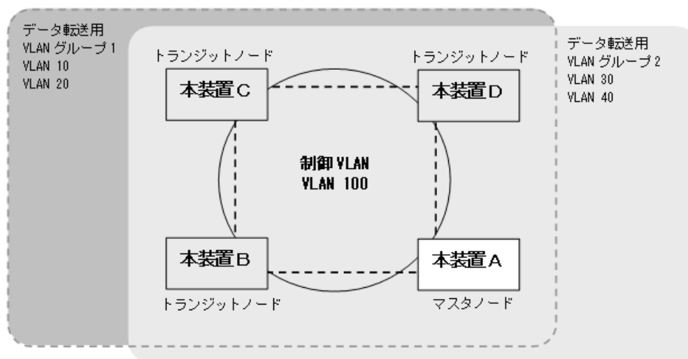
図 24-4 シングルリング構成
