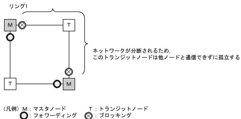
図 24-33 同一リング内に複数のマスタノードを設定
