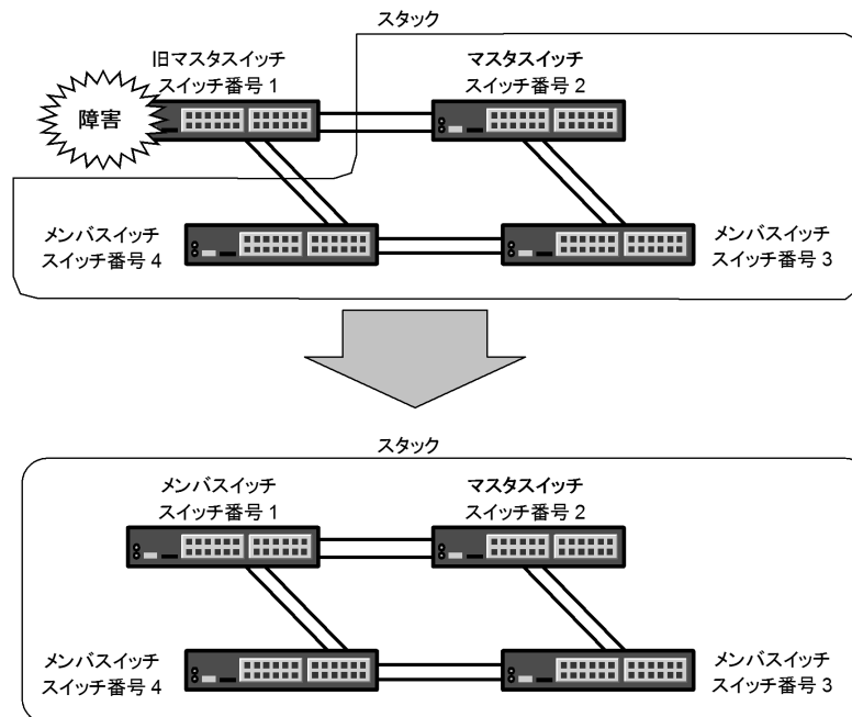
図 7-12 旧マスタスイッチ復旧時
