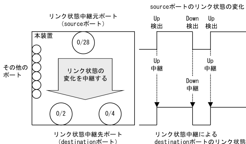
図 17-8 リンク状態中継機能の概要
