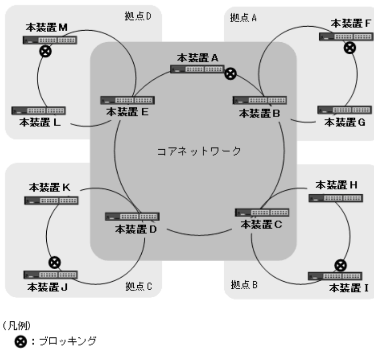
図 24-3 Ring Protocol の適用例（その 2）
