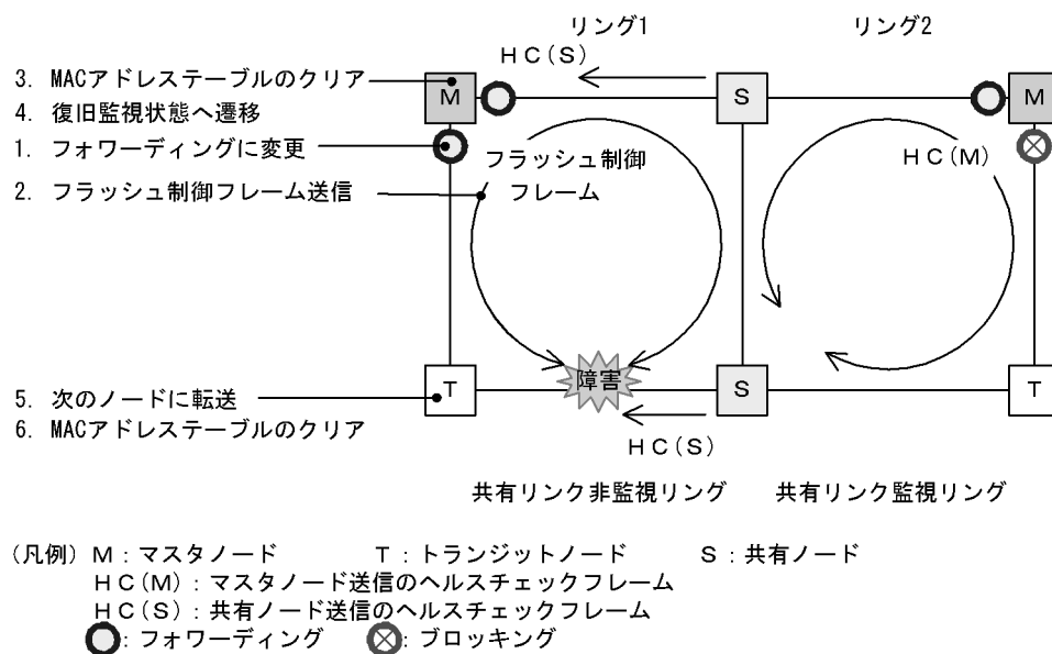
図 24-17 共有リンク非監視リングにおける共有リンク以外のリング障害時の動作
