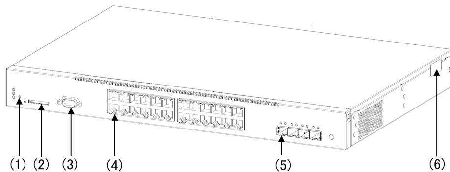
図 2-2 外観図 (24T4X)
