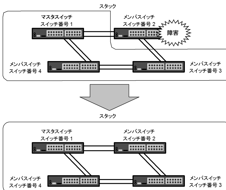
図 7-14 マスタ以外のメンバスイッチ復旧時
