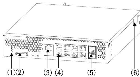
図 2-7 外観図 (08P, 08PD1, 08PD2)
