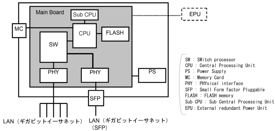
図 2-10 ハードウェアの構成（24T）
