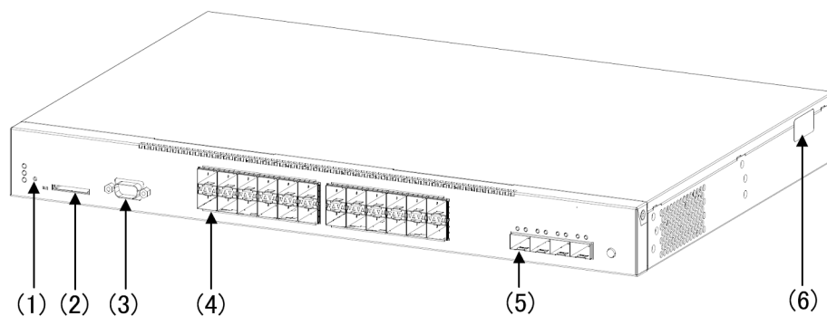
図 2-6 外観図 (24S4X, 24S4XD)
