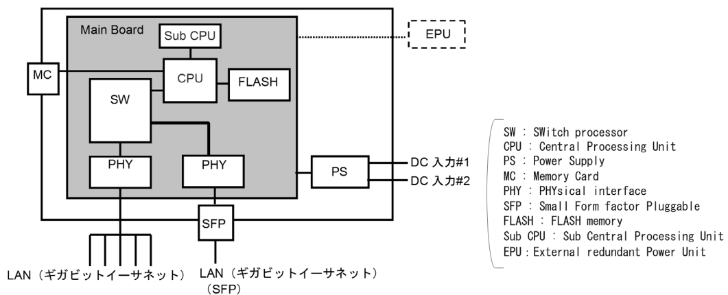
図 2-11 ハードウェアの構成（24TD）
