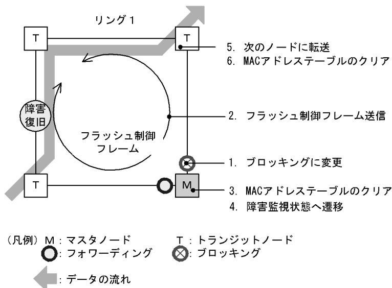
図 24-10 障害復旧時の動作
