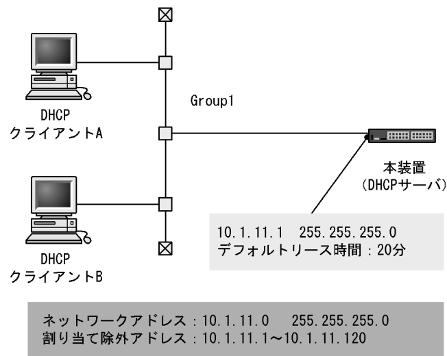
図 31-1 クライアントーサーバ構成（動的 IP アドレス配布時）
