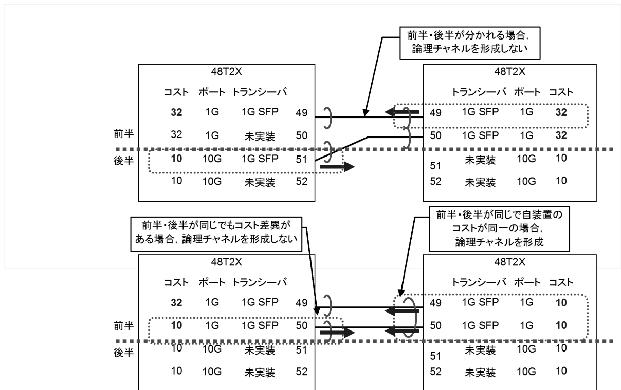
図 7-7 48ポートモデルの論理チャンネルグループ形成例
