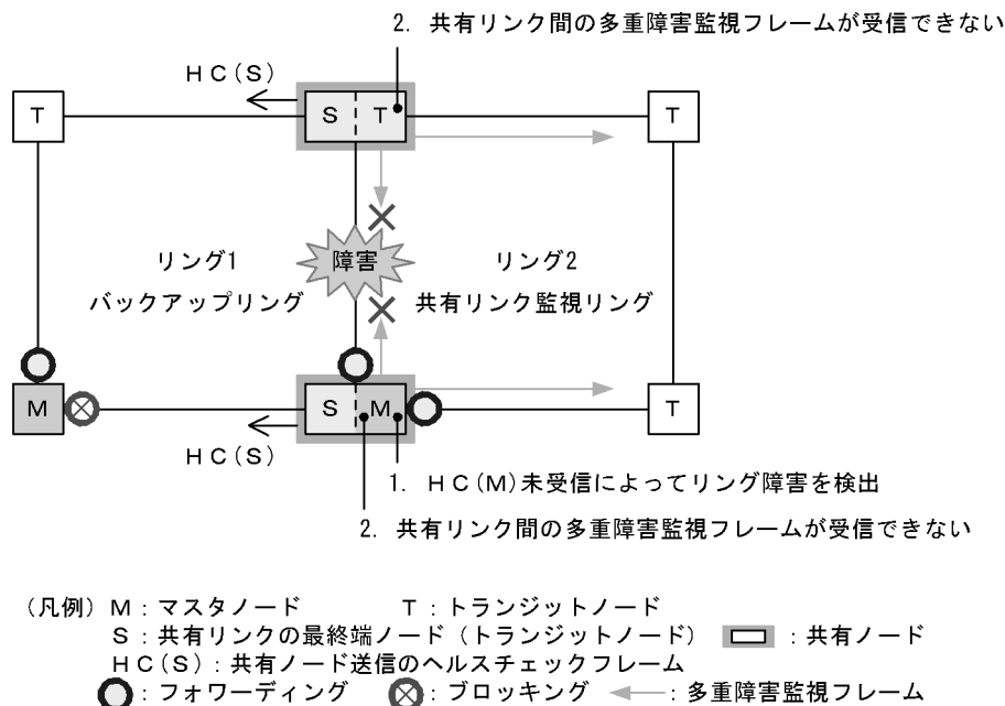
図 24-24 共有リンク障害時の動作
