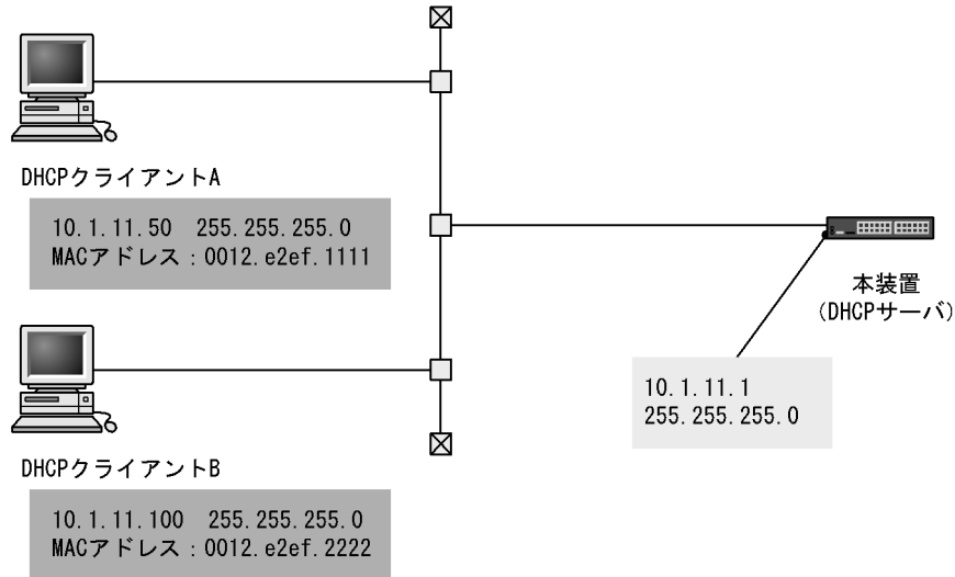
図 31-2 クライアントーサーバ構成（固定 IP アドレス配布時）
