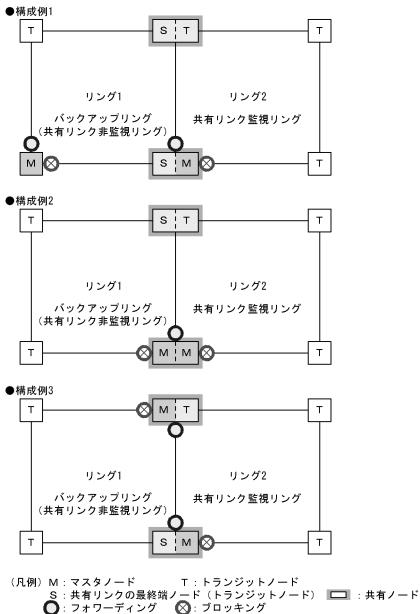
図 24-22 多重障害監視機能の基本構成例
