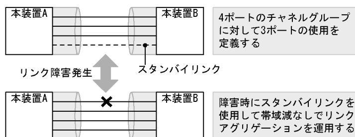
図 18-3 スタンバイリンク機能の構成例
