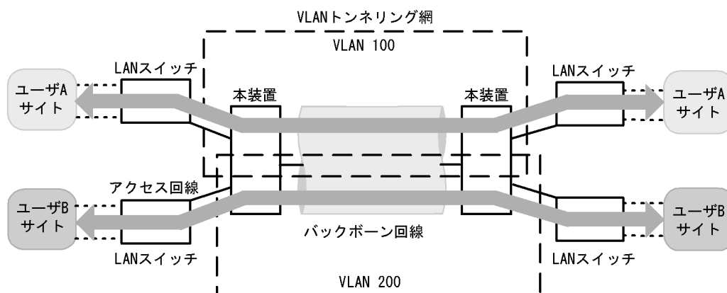
図 22-1 VLAN トンネリング概要（広域イーサネットサービス適用例）
