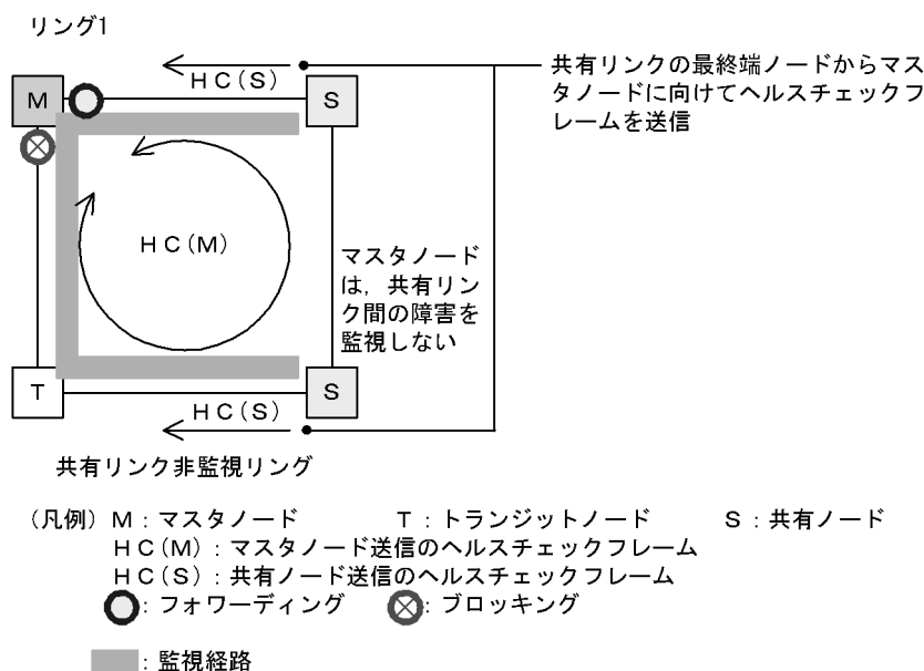
図 24-13 共有リンク非監視リングでの正常時の動作
