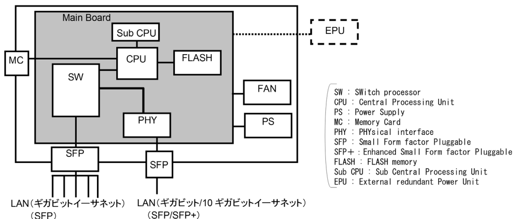
図 2-16 ハードウェアの構成 (24S4X)
