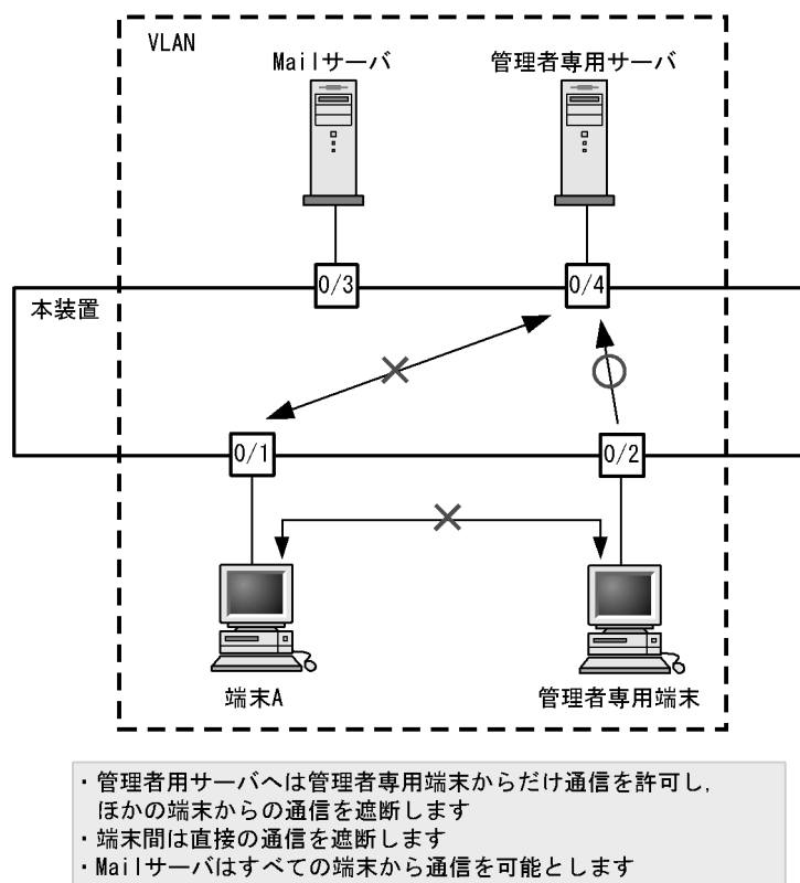
図 22-6 ポート間中継遮断機能の設定例
