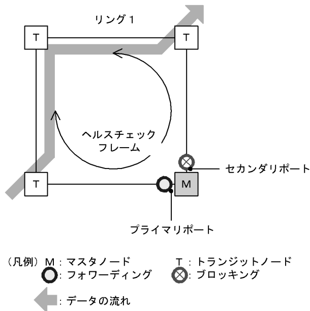
図 24-8 リング正常時の動作
