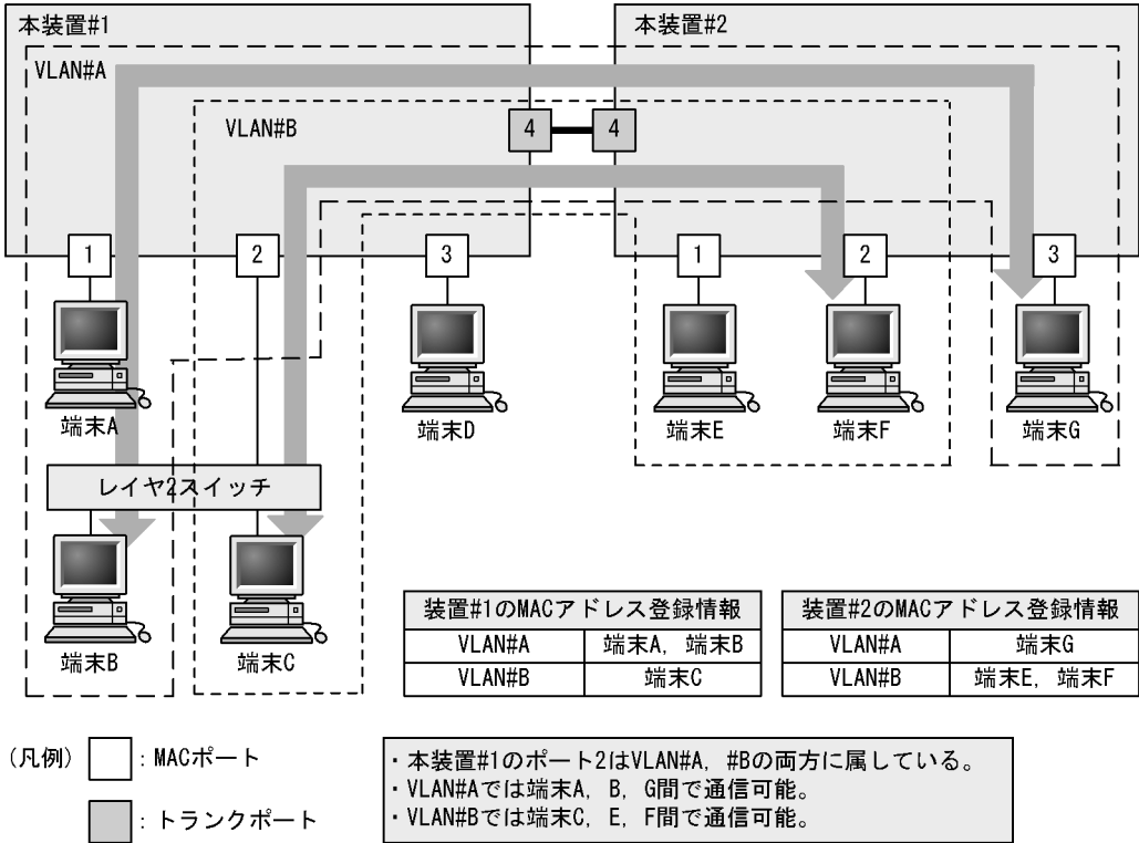
図 21-8 MAC VLAN の構成例
