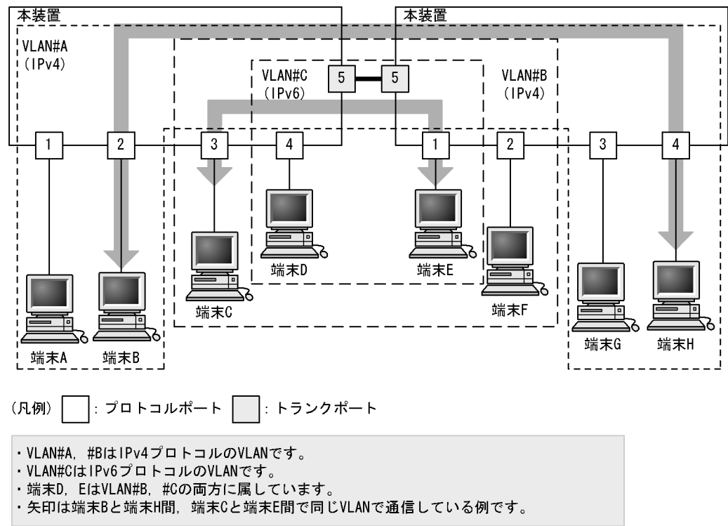
図 21-5 プロトコル VLAN の構成例
