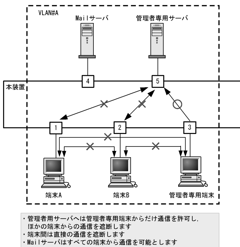
図 22-5 ポート間中継遮断機能の適用例
