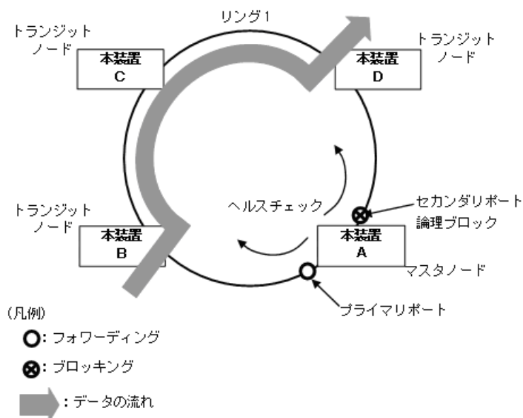
図 24-1 Ring Protocol の概要
