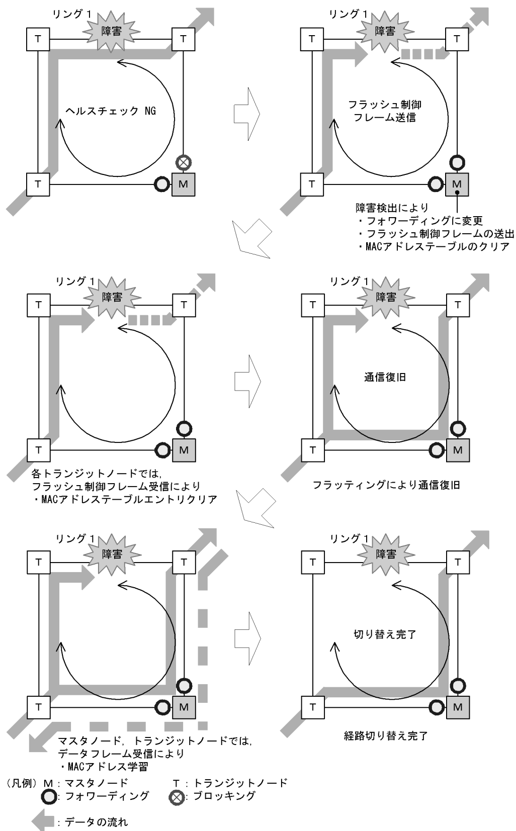
図 24-7 Ring Protocol の経路切り替え動作概要
