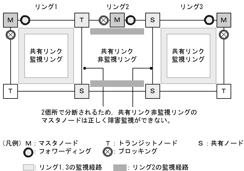
図 24-34 共有リンク監視リングが複数ある構成
