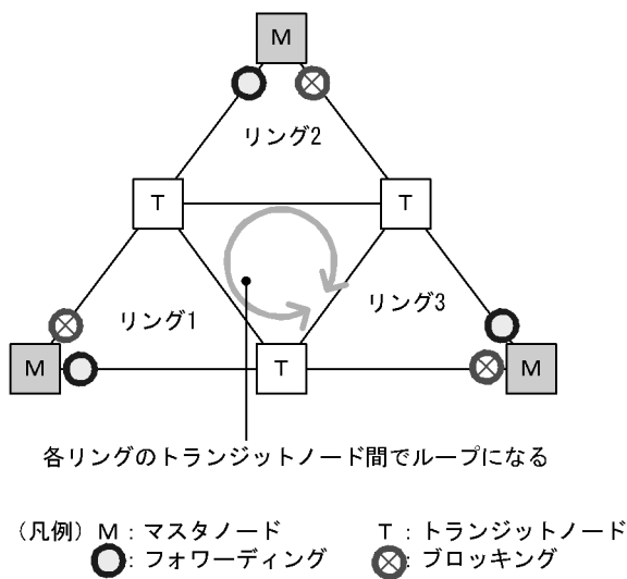
図 24-35 ループになるマルチリング構成
