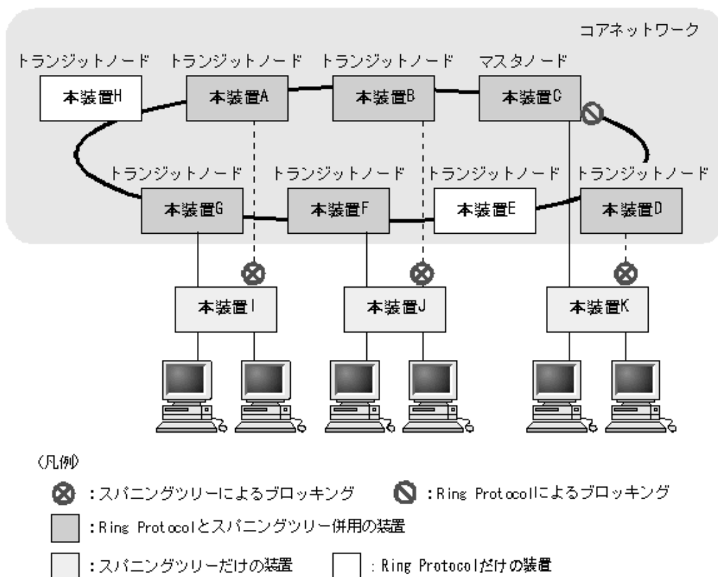
図 26-1 Ring Protocol とスパニングツリーの併用例（シングルリング構成）
