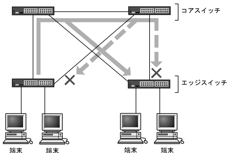
図 23-1 スパニングツリーを適用したネットワークの概要
