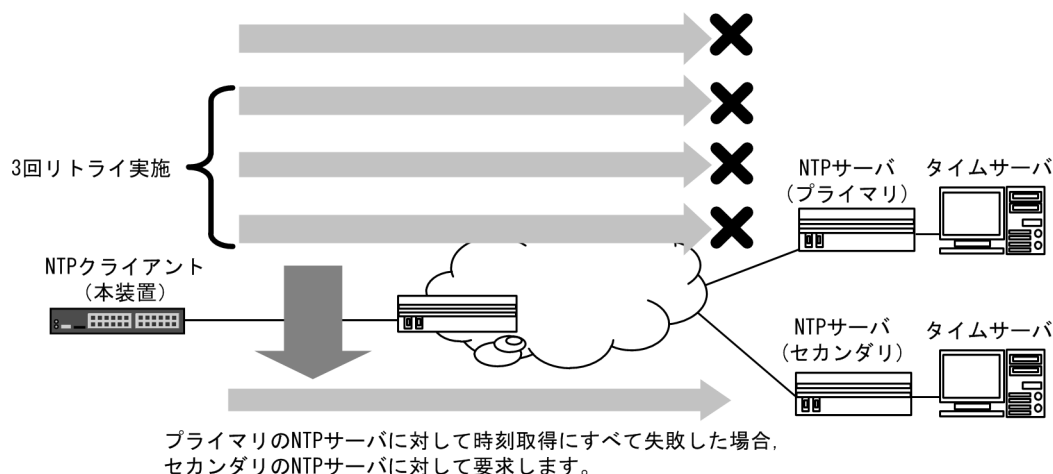
図 11-2 Unicast モードによる時刻情報取得図 (プライマリ/セカンダリ設定時)
