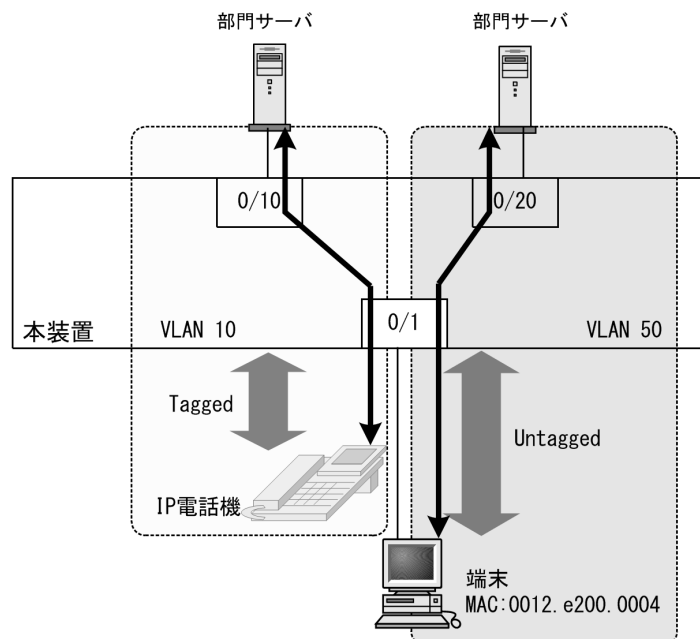
図 21-11 MAC ポートでの Tagged フレーム中継の設定例
