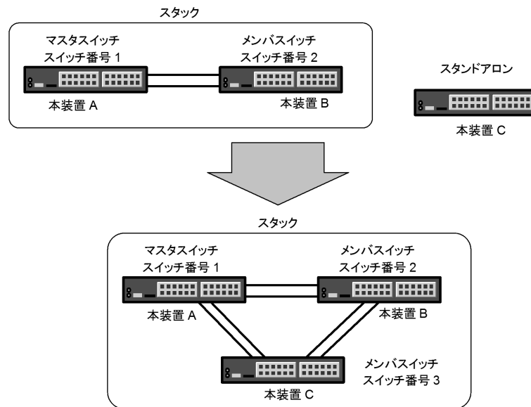
図 8-3 メンバスイッチの追加
