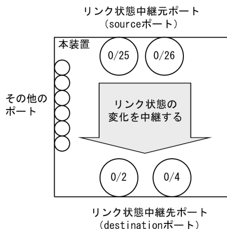
図 17-9 リンク状態中継機能の設定例
