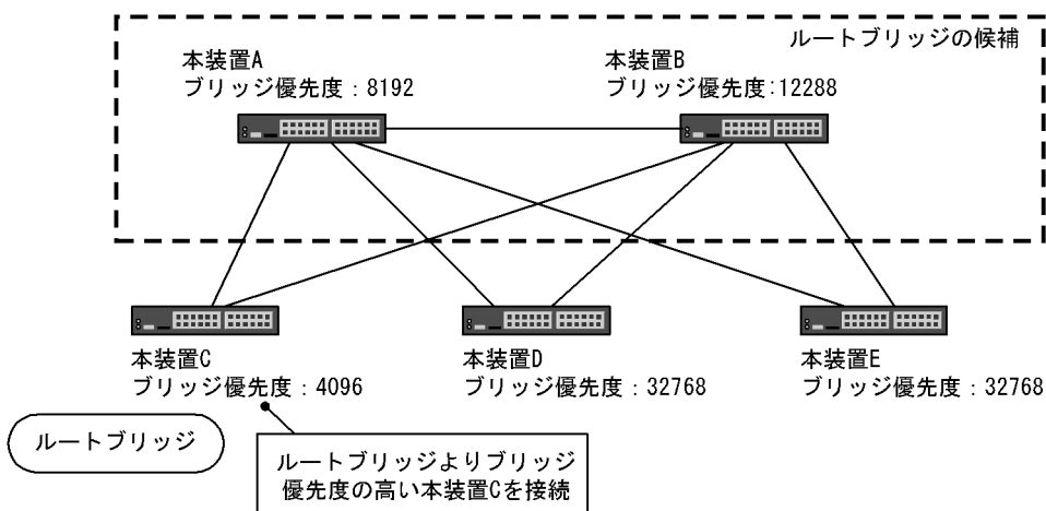
図 23-19 本装置 A、本装置 B よりブリッジ優先度の高い本装置 C を接続
