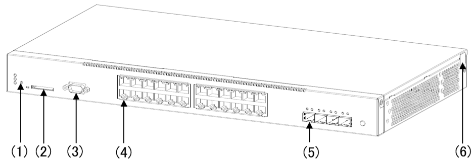
図 2-1 外観図 (24T, 24TD)
