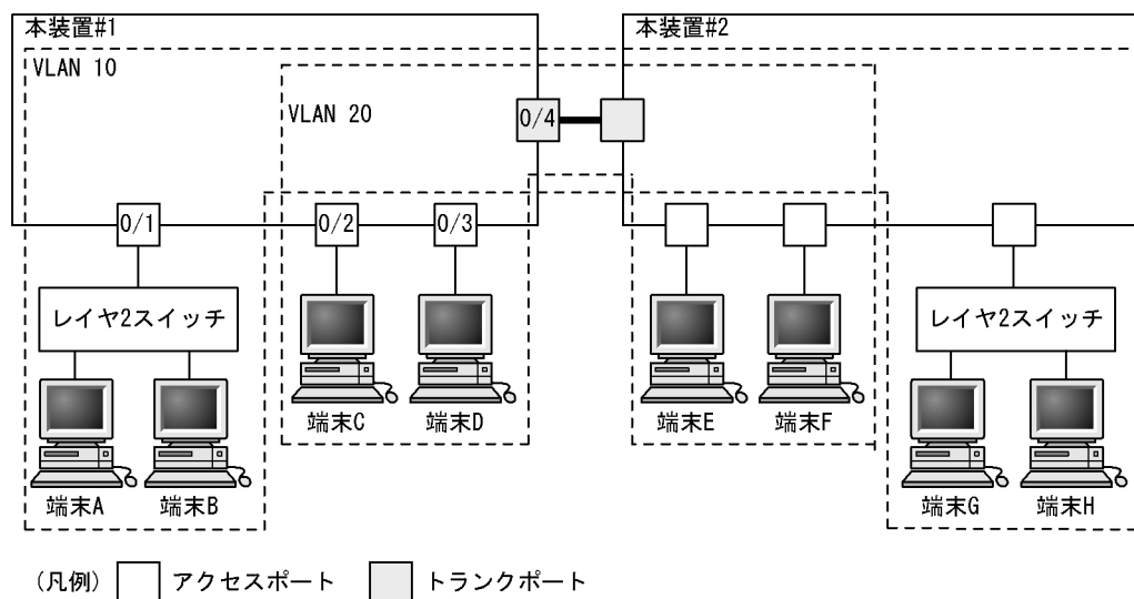
図 21-4 ポート VLAN の設定例
