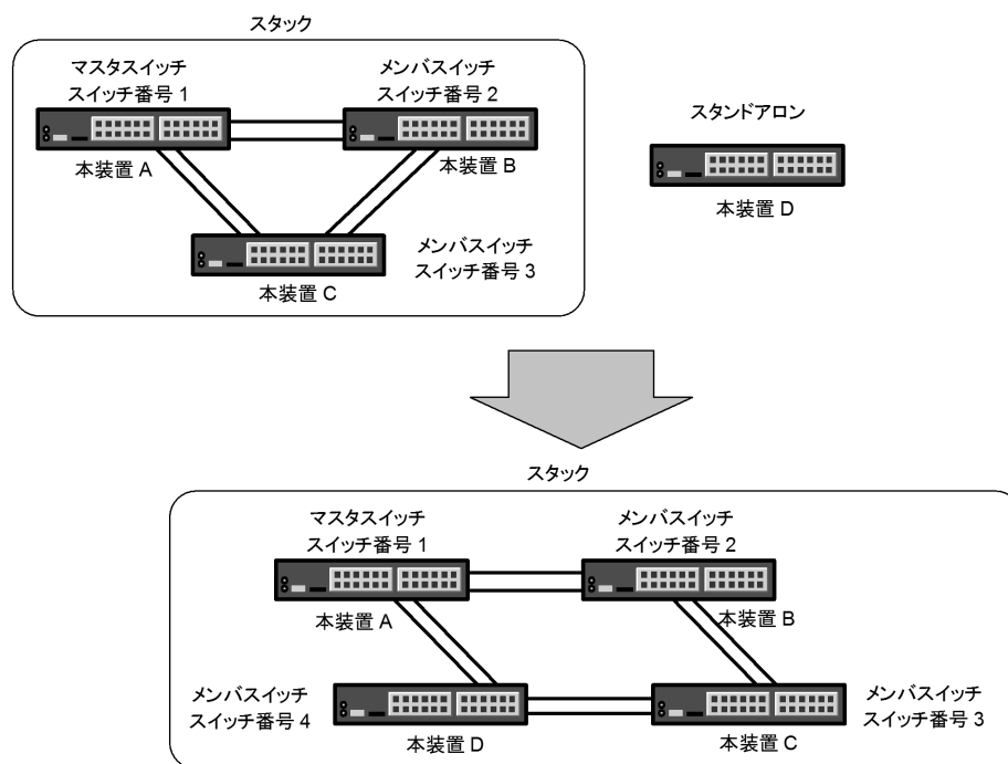
図 8-4 メンバスイッチの追加
