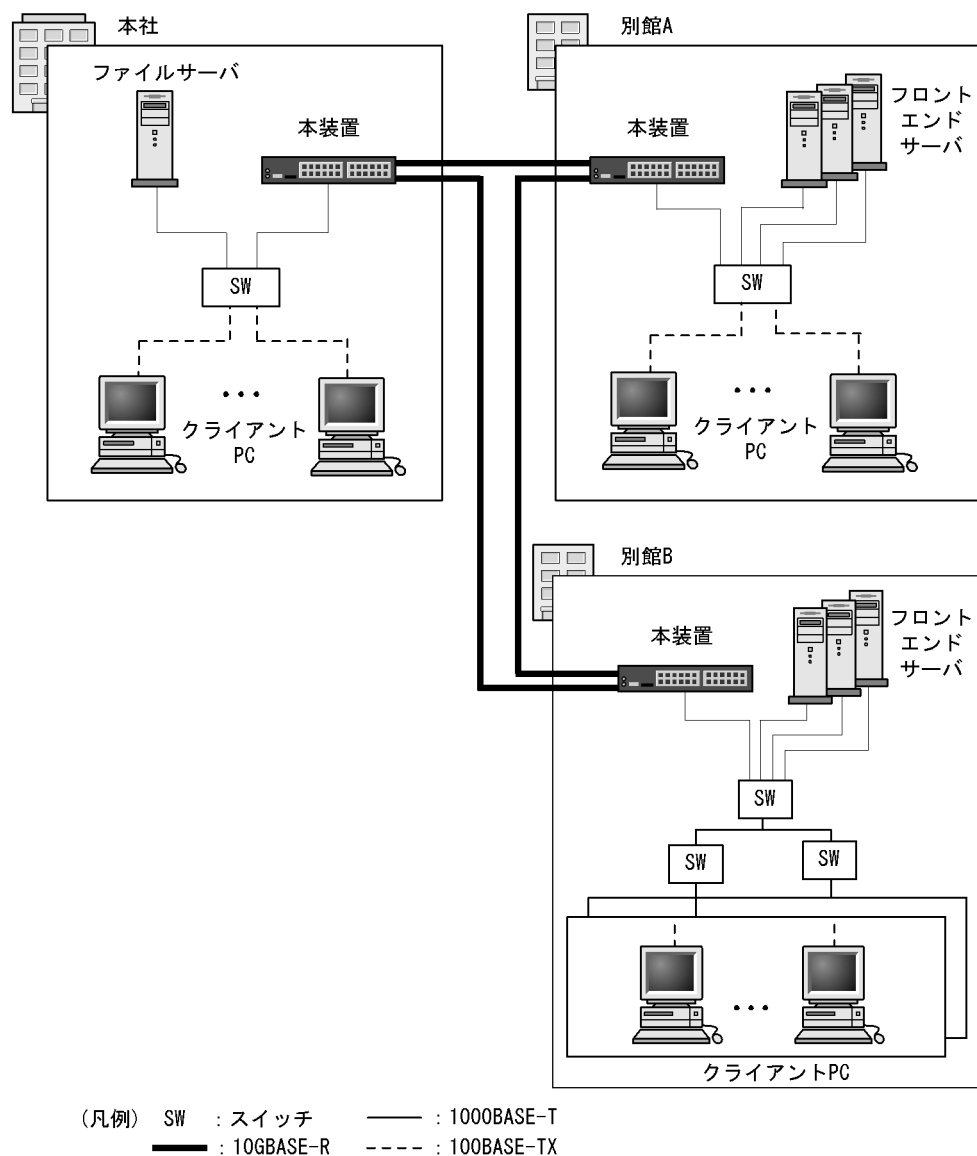
図 17-1 イーサネットの構成例
