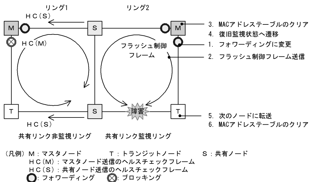
図 24-19 共有リンク監視リングでの共有リンク以外のリング障害時の動作
