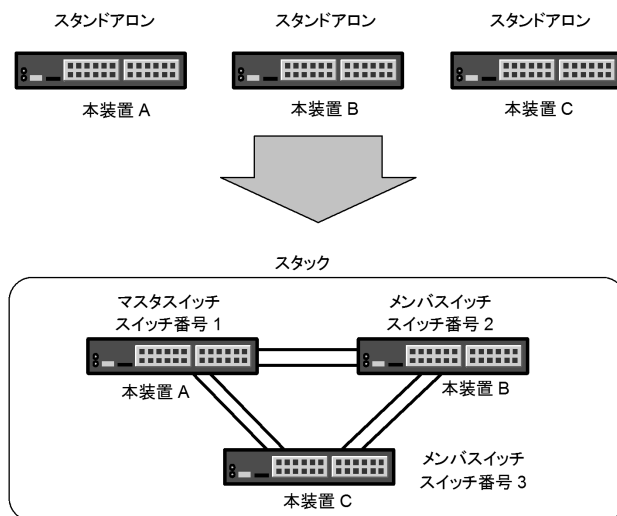
図 8-2 スタンドアロンからの構築
