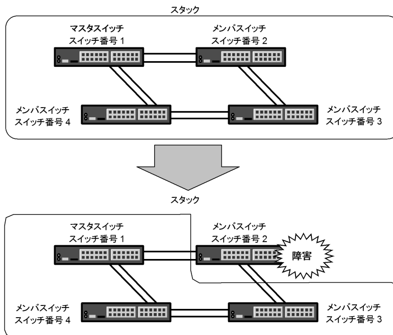
図 7-13 マスタ以外のメンバスイッチ障害時
