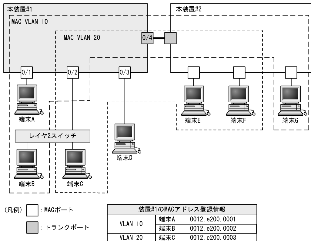
図 21-10 MAC VLAN の設定例
