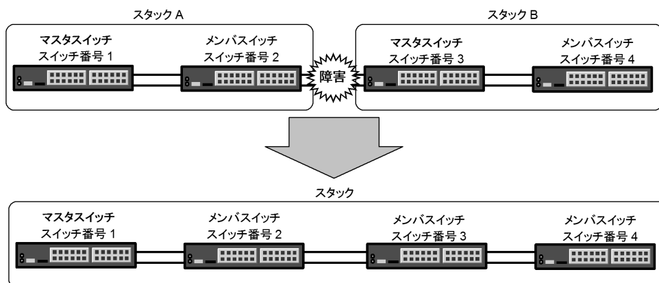
図 7-16 スタックリンク復旧時
