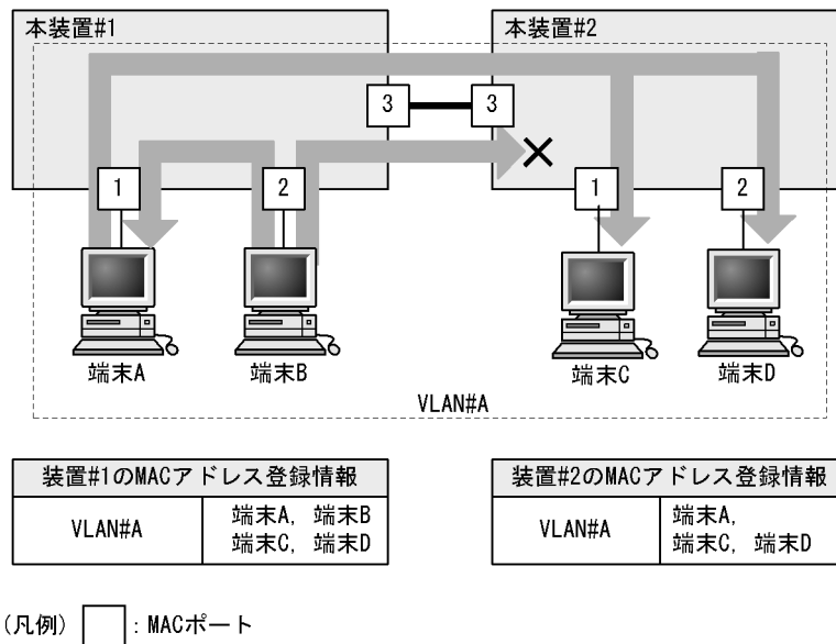
図 21-9 装置間を MAC ポートで接続した場合
