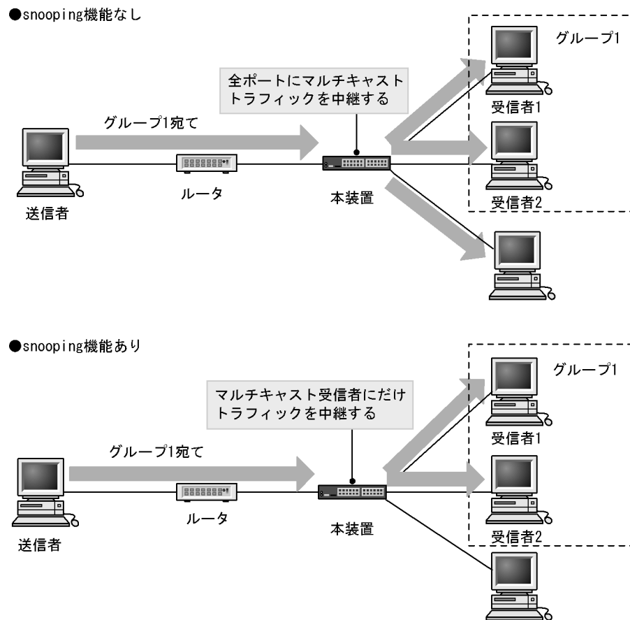
図 27-2 IGMP snooping/MLD snooping 概要
