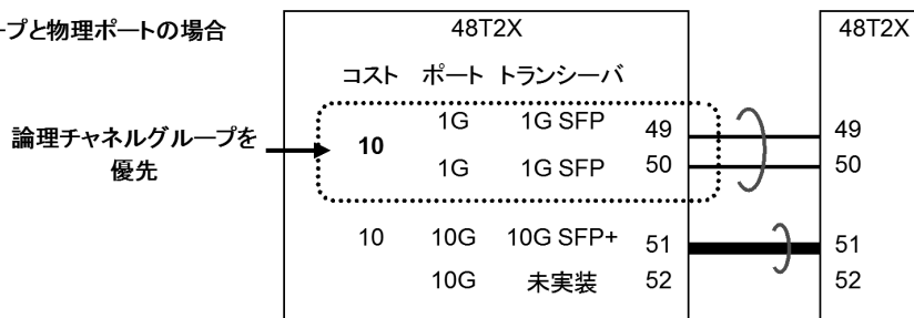
図 7-6 同一コスト設定時の経路選択例
