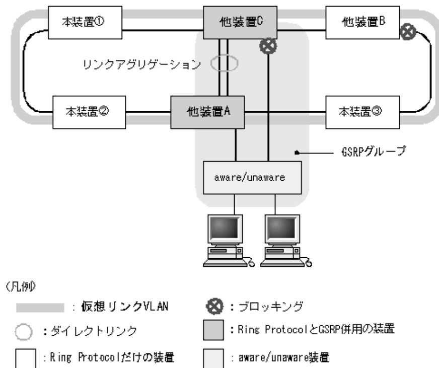
図 26-10 Ring Protocol と GSRP の併用例と本装置の位置づけ（ダイレクトリンクをリングネットワークで使用しない場合）
