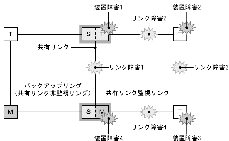
図 24-21 共有リンク監視リングでの障害発生例
