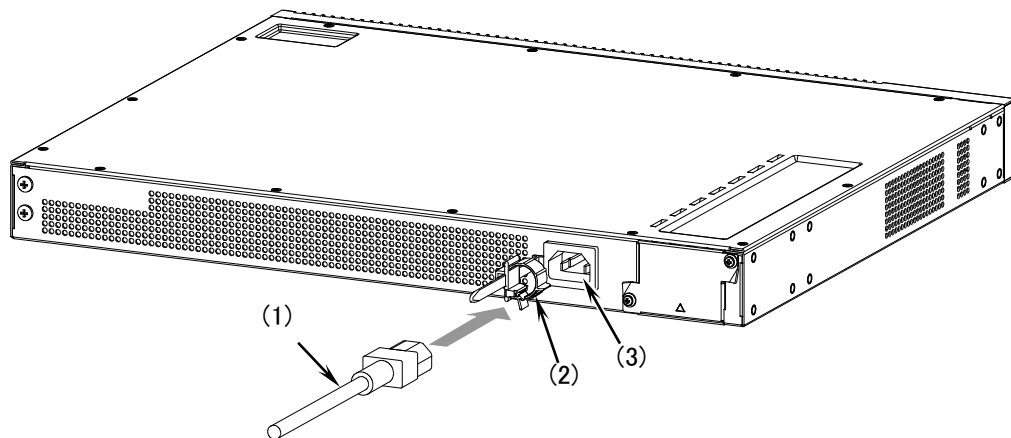
図4-16 電源の投入
