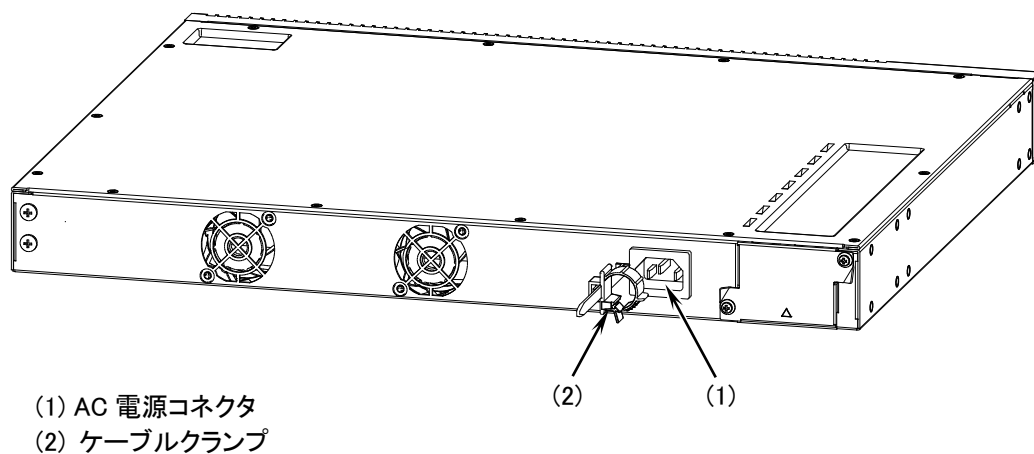
図1-10 背面外観
