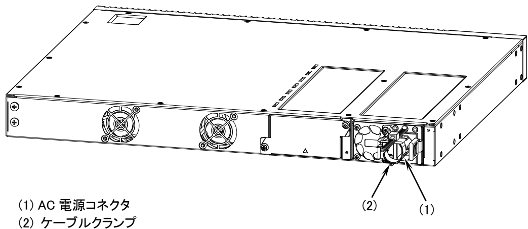
図1-18 背面外観
