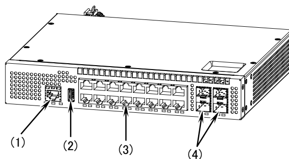
図1-1 正面外観
