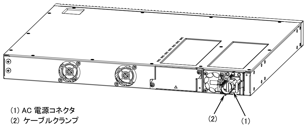
図1-22 背面外観
