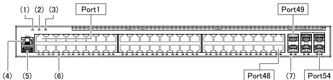
図1-11 正面パネルレイアウト
