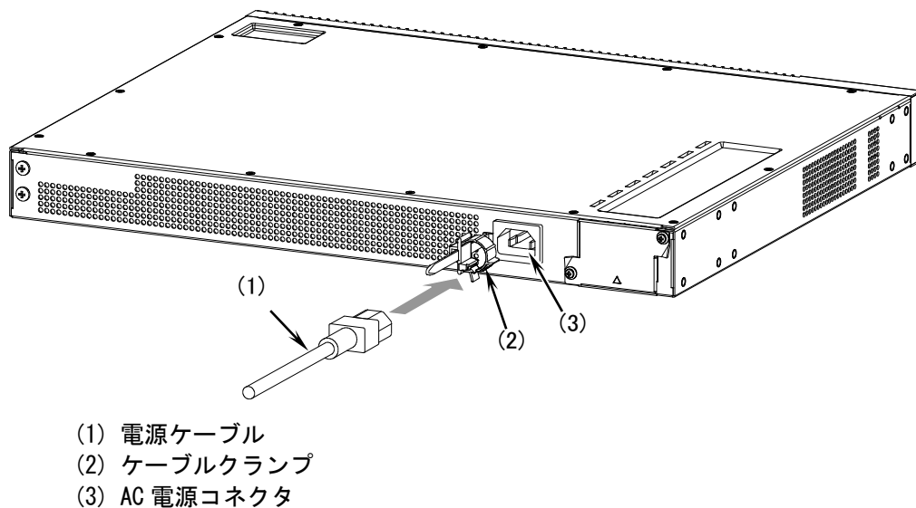
図4-7 電源ケーブルの取り付け
