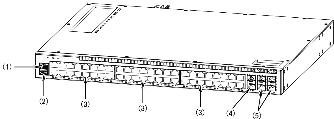
図1-9 正面外観
