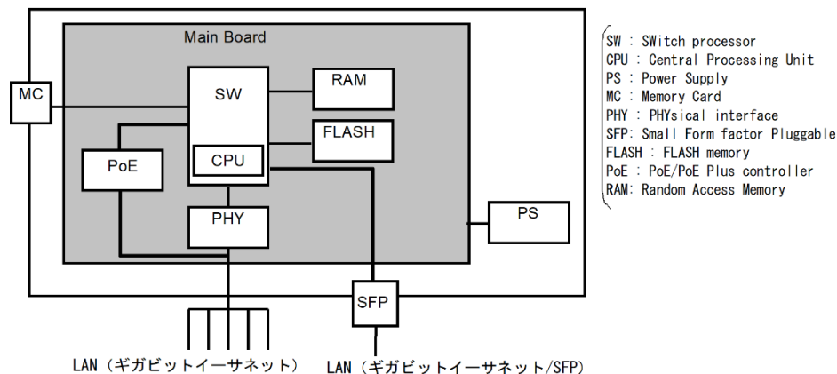
図 2-15a ハードウェアの構成 (AX2130S-24PH モデル)
