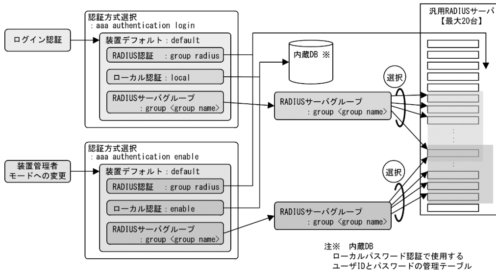
図 8-7 認証方式設定の相関図
