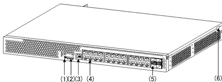
図 2-7a AX2130S-24PH モデル
