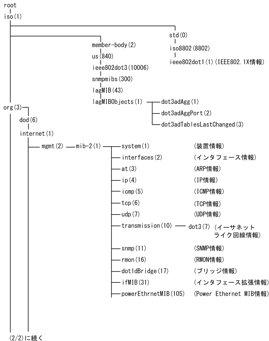
図 1-1 MIB 体系図 (1/2)
