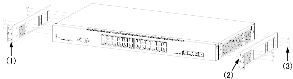
図 4-10 ラック固定金具の取り付け【50mm 奥に調整する場合】 (AX2200S, AX2130S-24PH)
