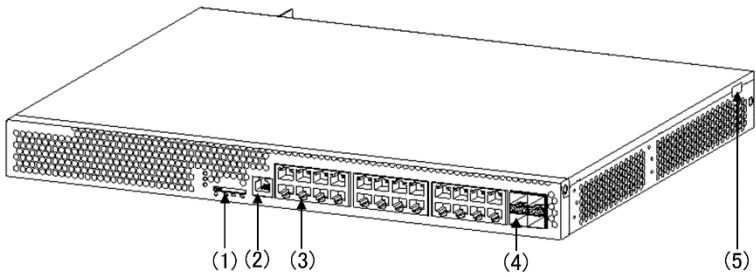
図 1-21a 正面外観
