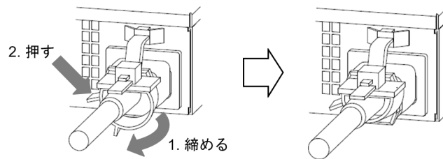
図 4-16 電源ケーブルのクランプ (AX2130S-16T, AX2130S-16P)
