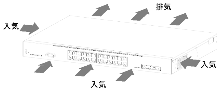
図 2-7 AX2230S-24P のエアフロー
