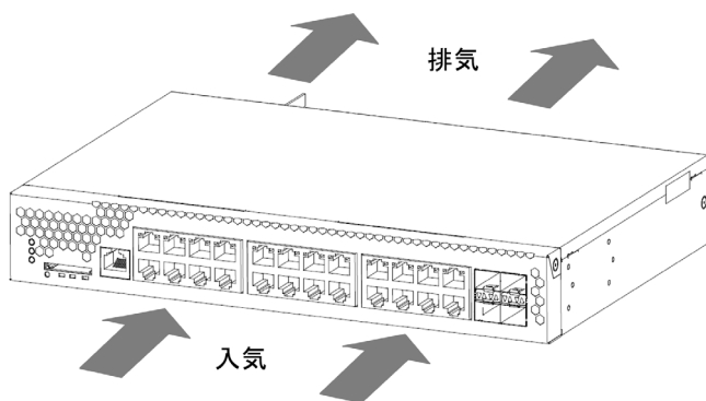
図 2-8 AX2130S-24P/AX2130S-16P のエアフロー
