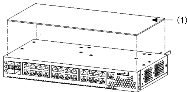
図 4-3 マグネットシートの貼り付け (AX2130S-24T, AX2130S-24TH, AX2130S-24P)
