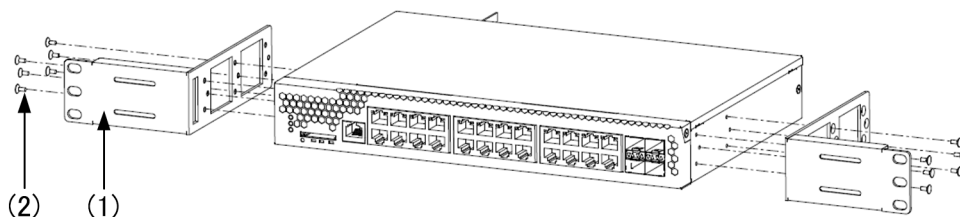
図 4-7 ラック固定金具の取り付け (AX2130S-24T, AX2130S-24TH, AX2130S-24P)
