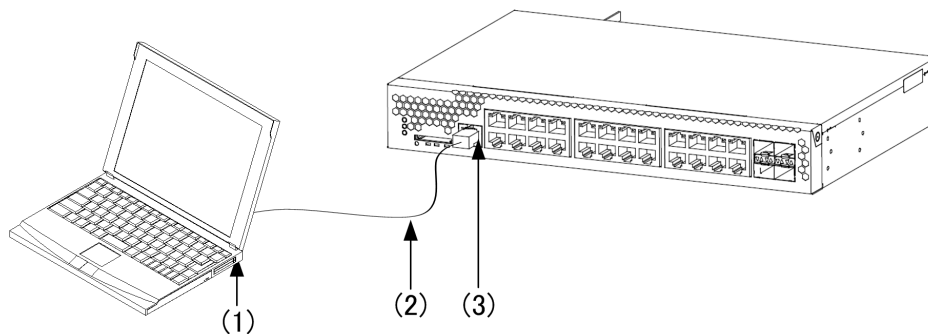
図 4-27 運用端末の接続図 (AX2100S)
