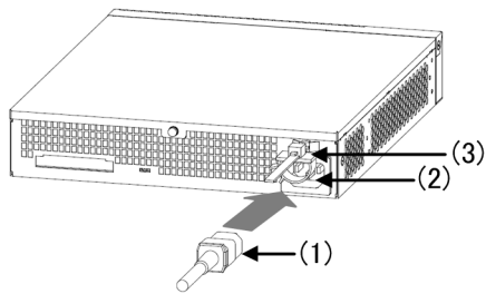
図 4-14 電源ケーブルの取り付け (AX2130S-16T, AX2130S-16P)
