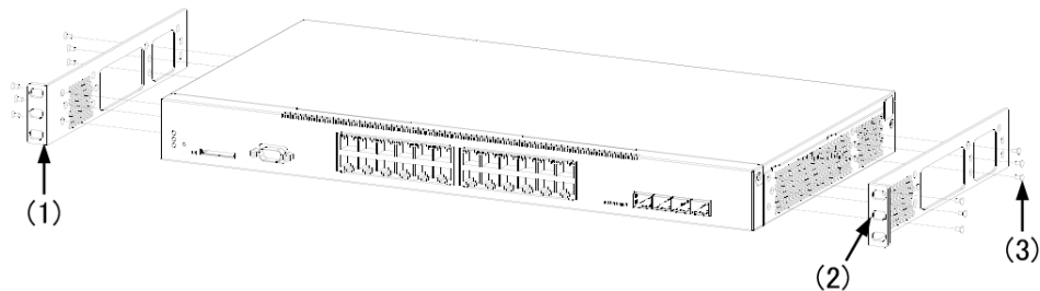
図 4-6 ラック固定金具の取り付け (AX2200S)
