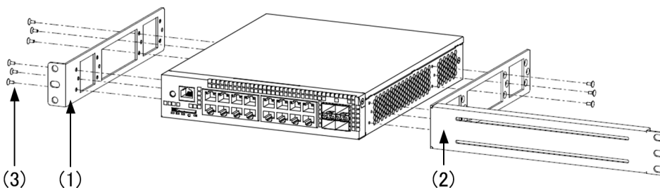
図 4-8 ラック固定金具の取り付け（AX2130S-16T, AX2130S-16P）
