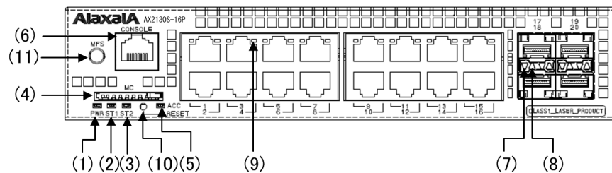
図 1-12 正面パネルレイアウト
