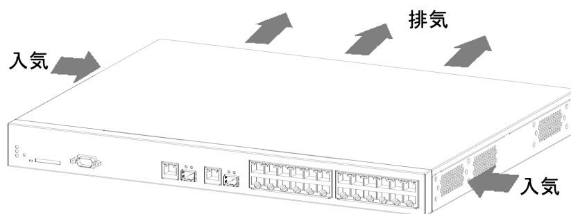
図 2-10 AX1240S-24P2C, AX1240S-48T2C のエアフロー
