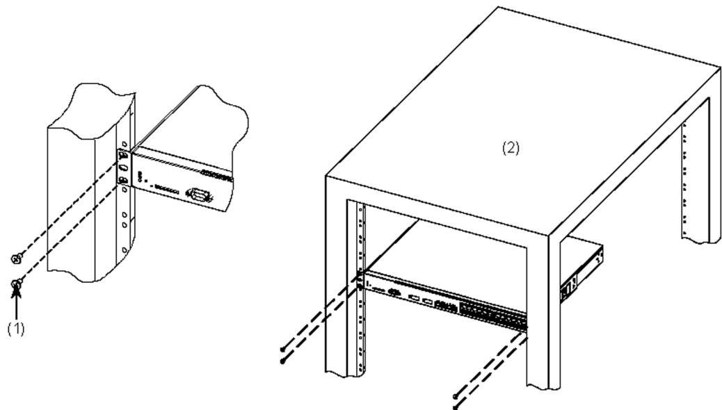
図 4-11 ラックへの搭載 (AX2130S-16T, AX2130S-16P 以外)
