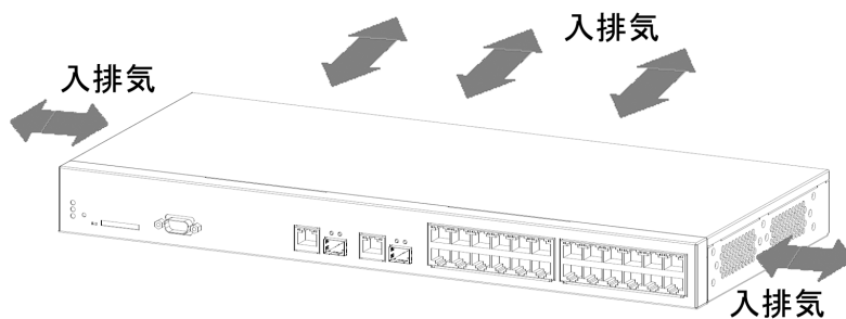
図 2-9 AX1250S-24T2C, AX1240S-24T2C のエアフロー
