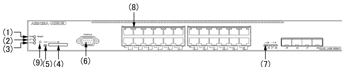
図 1-6 正面パネルレイアウト
