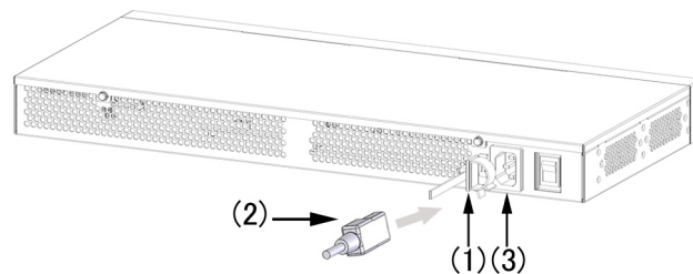
図 4-13 電源ケーブルの取り付け (AX2130S-16T, AX2130S-16P 以外)
