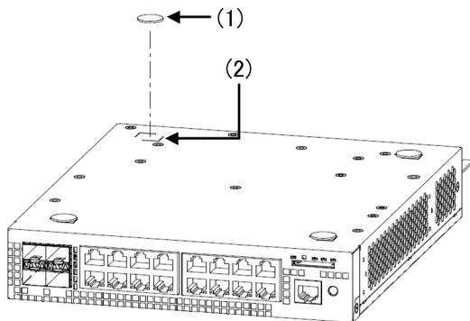
図 4-2 ゴム足の取り付け（AX2130S-16T, AX2130S-16P）
