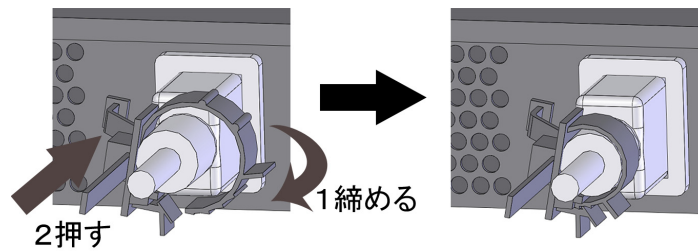
図 4-15 電源ケーブルのクランプ (AX2130S-16T, AX2130S-16P 以外)
