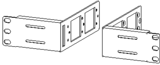
図 1-37 ラック固定金具（AX2100S 19 インチラック搭載モデル用）
