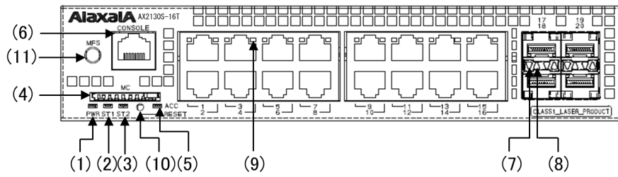
図 1-9 正面パネルレイアウト
