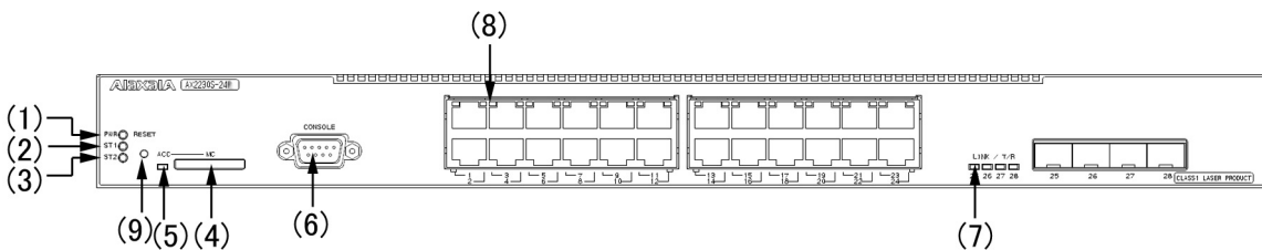
図 1-3 正面パネルレイアウト
