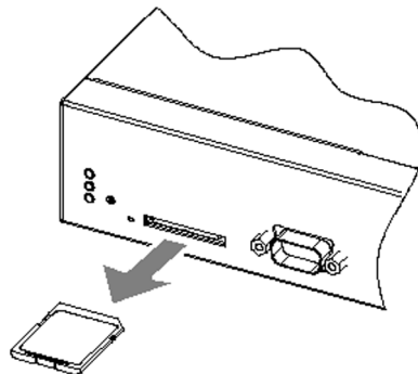
図 4-19 メモ리카ードの取り出し
