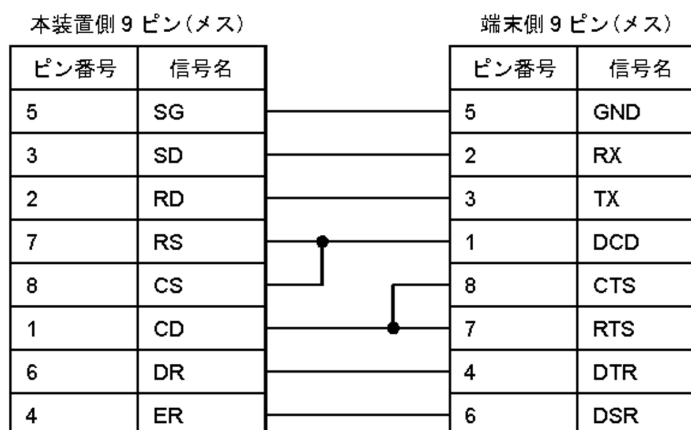
図 C-1 運用端末接続ケーブル・ピン配置 (両端 D-sub 9 ピン)
