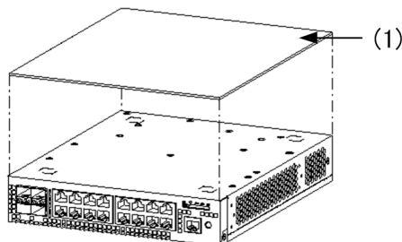
図 4-4 マグネットシートの貼り付け (AX2130S-16T, AX2130S-16P)
