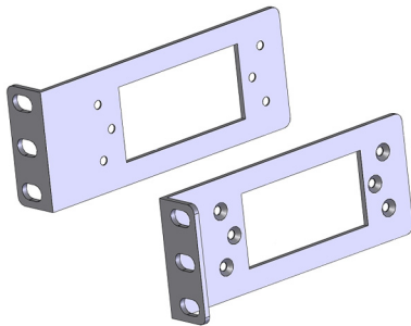
図 1-38 ラック固定金具（AX1250S, AX1240S 用）
