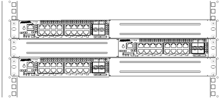
図 4-12 ラックへの搭載 (AX2130S-16T, AX2130S-16P)
