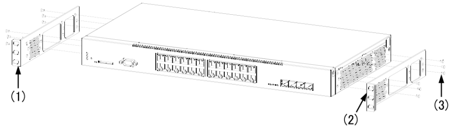
図 4-10 ラック固定金具の取り付け【50mm 奥に調整する場合】(AX2200S)
