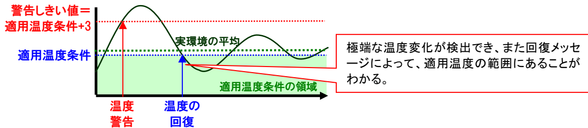
図 3.1-3 温度警告メッセージしきい値=+マージンの場合
