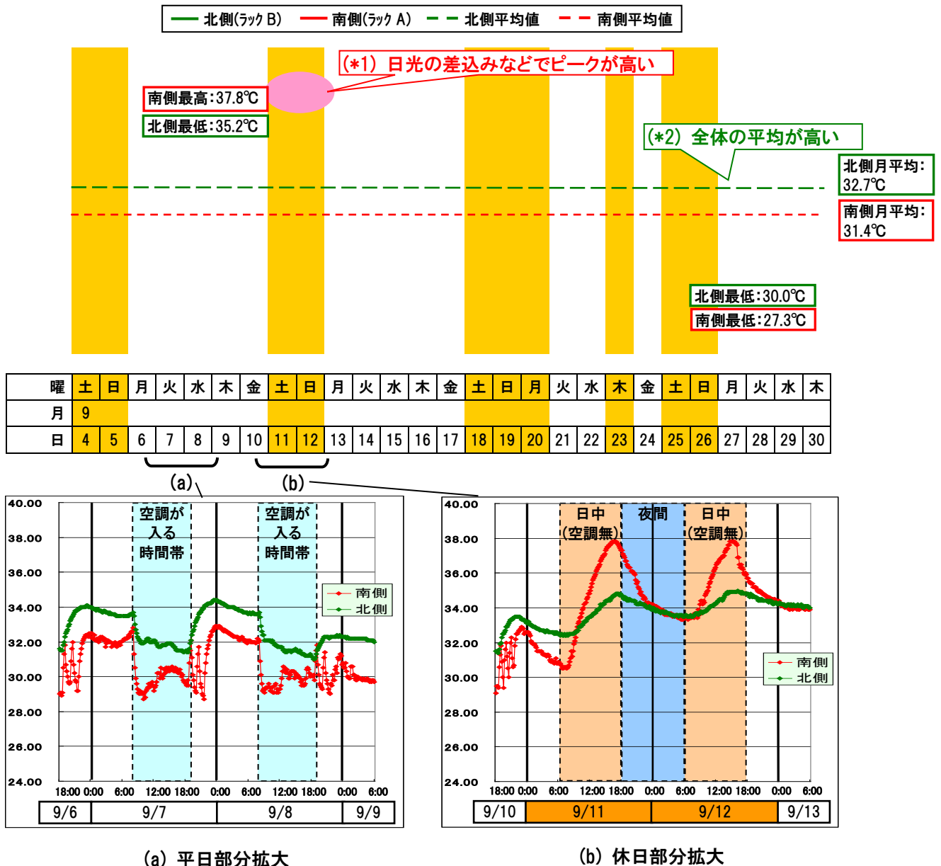
図 4.1-3 フロア設置のラック内温度観測例
