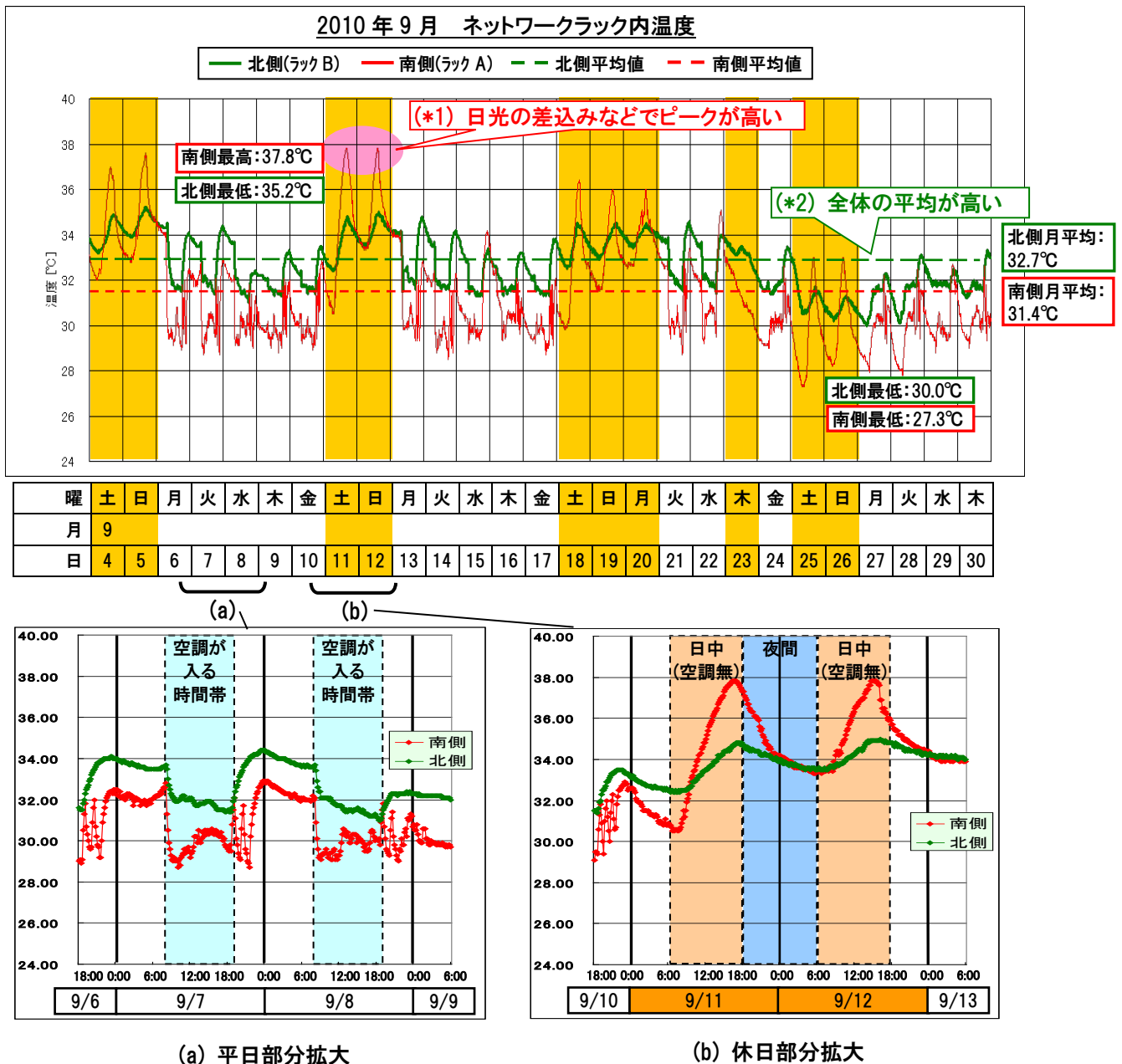
図 4.1-3 フロア設置のラック内温度観測例
