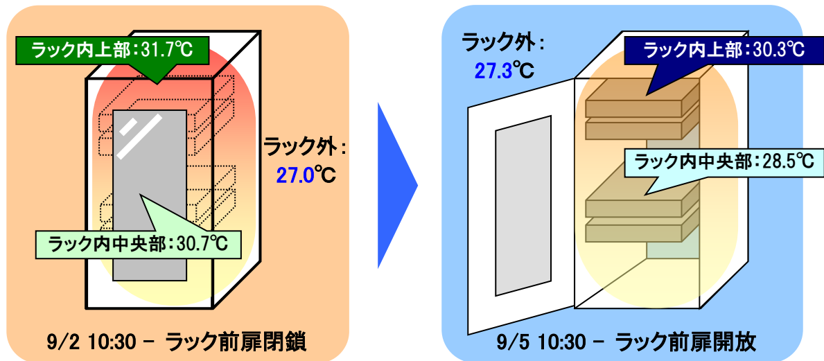
図 4.3-3 (A)点(10:30 時点)でのラックの温度分布のようす
