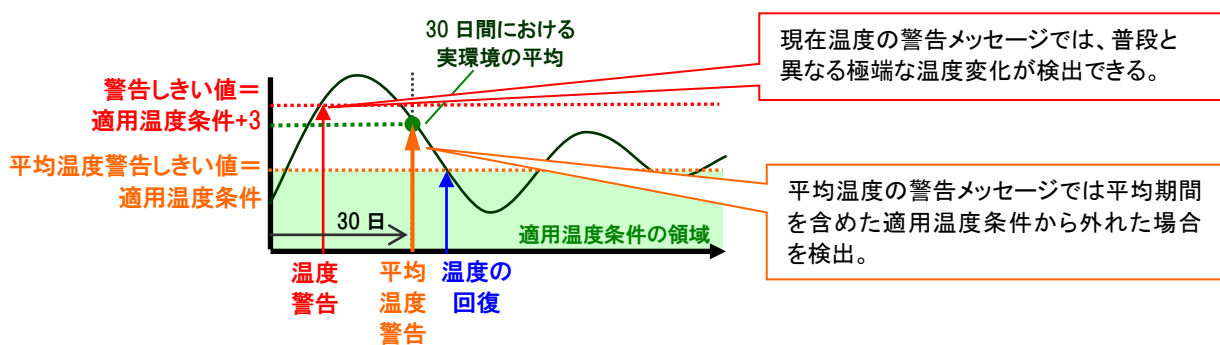
図 3.1-1 平均温度警告メッセージと現在温度警告メッセージの併用
