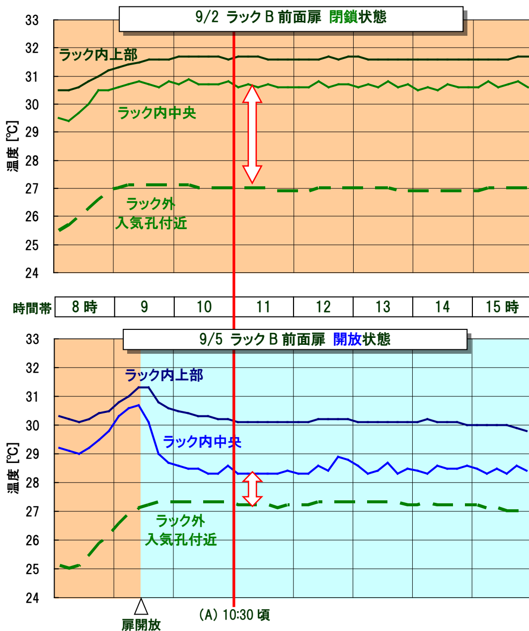
図 4.3-2 ラック前扉の状態による温度差の比較
