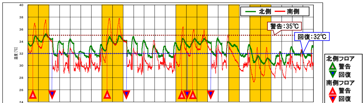
図 4.2-1 しきい値設定が 35℃の場合の温度警告メッセージ出力予想
