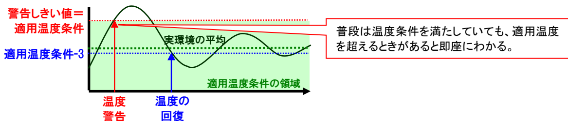
図 3.1-2 温度警告メッセージしきい値＝適用温度条件の場合
