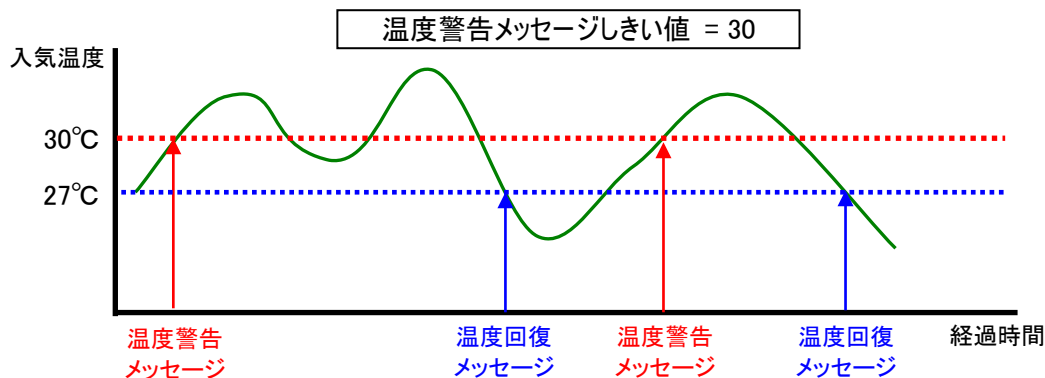
図 2.2-3 温度警告のしきい値設定を 30(℃) に設定した場合の動作
