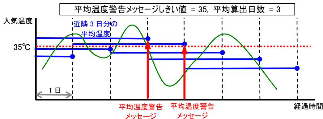
図 2.2-4 平均温度警告のしきい値設定を 35(℃)に設定した場合の動作
