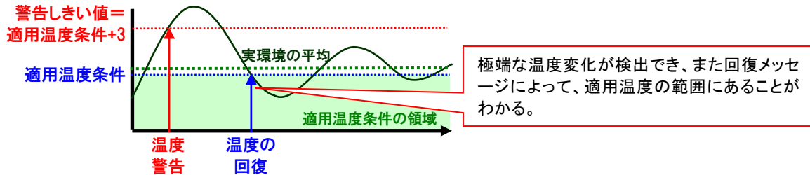
図 3.1-3 温度警告メッセージしきい値=+マージンの場合
