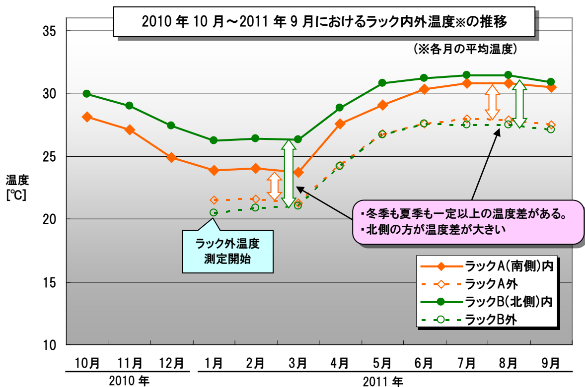
図 4.3-1 ラック内および周辺の月平均温度
