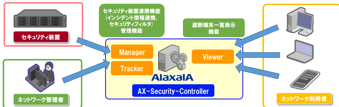
図 2-1 AX-Security-Controller の構成
