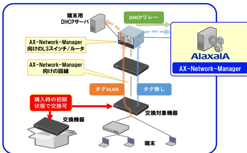
図 5-2 購入時の初期状態のままの交換機を使用できるネットワーク例
