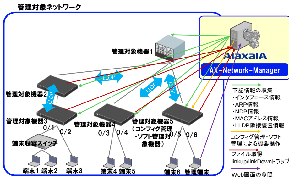
図 5-1 前提とするネットワーク構成例
