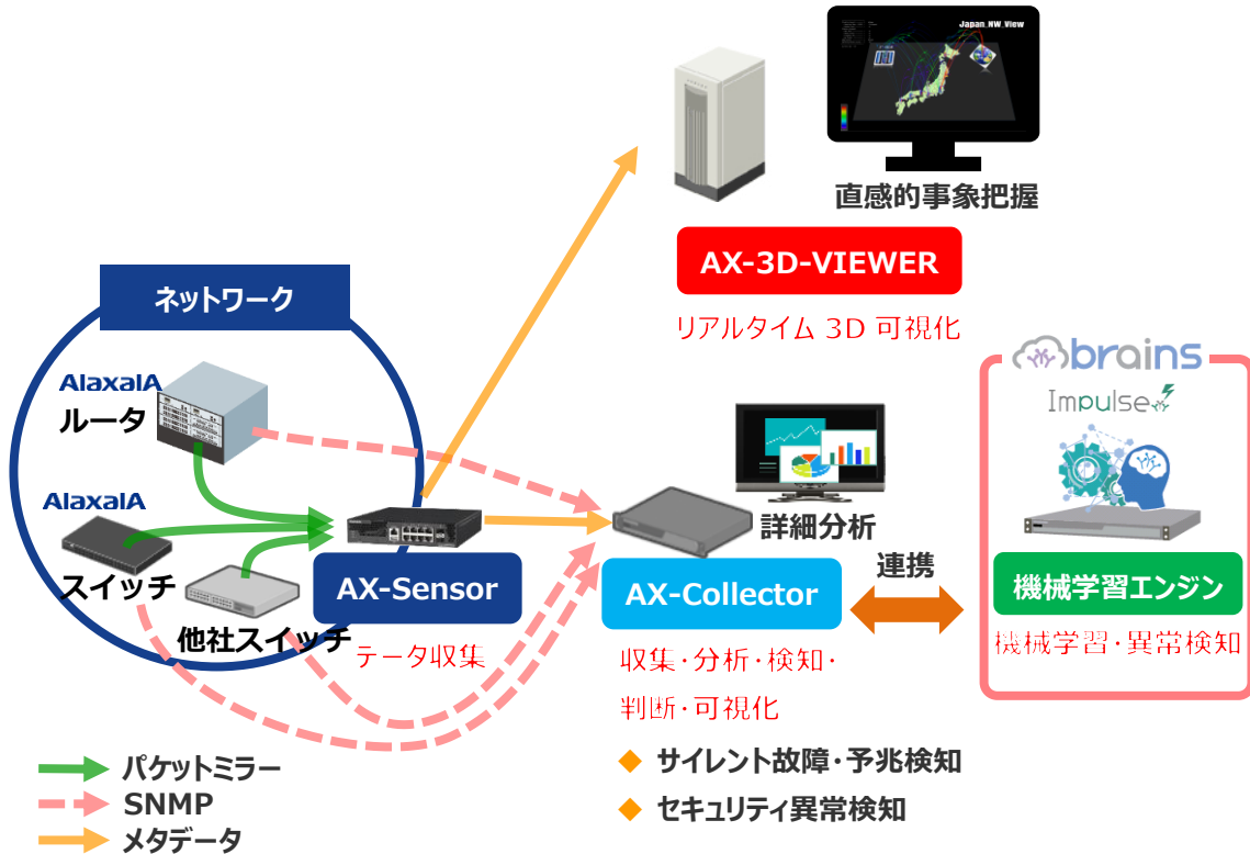
図 1-1 ネットワーク可視化・異常検知ソリューション概要
