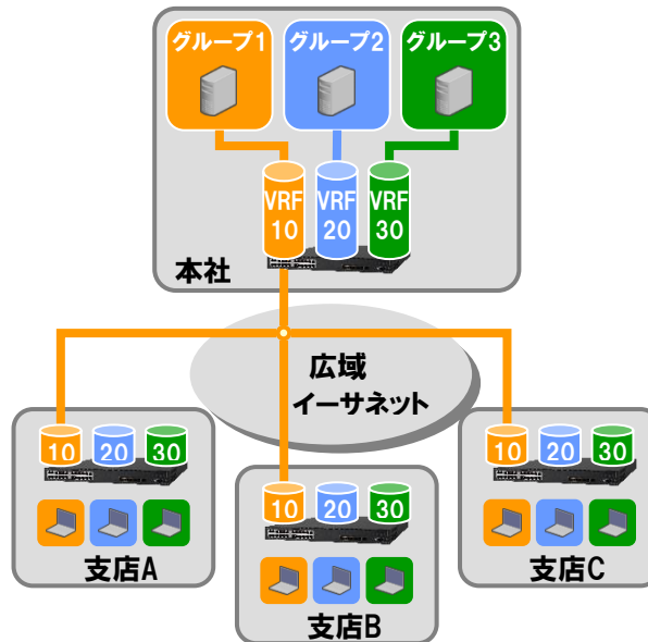
図 7 ネットワーク・パーティション
