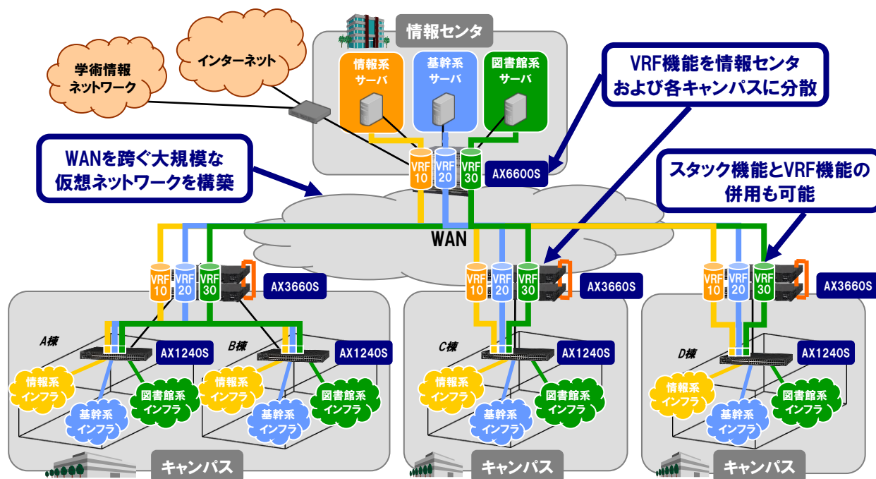
図 6 キャンパスネットワークへの適用例
