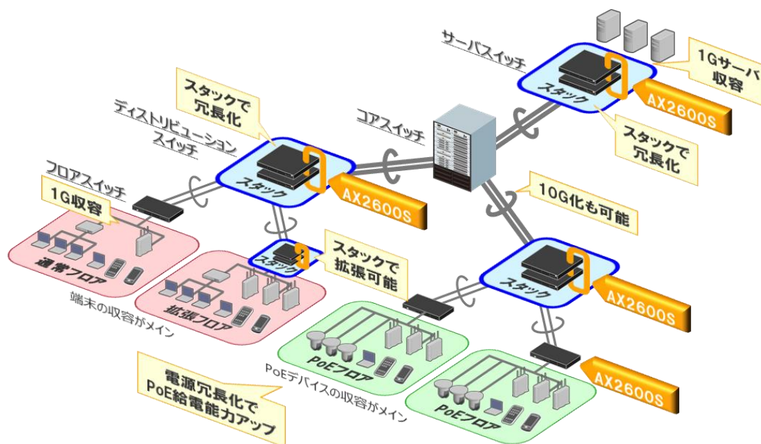
図 5 デISTRIBUTIONスイッチ、フロアスイッチとしての構成例
