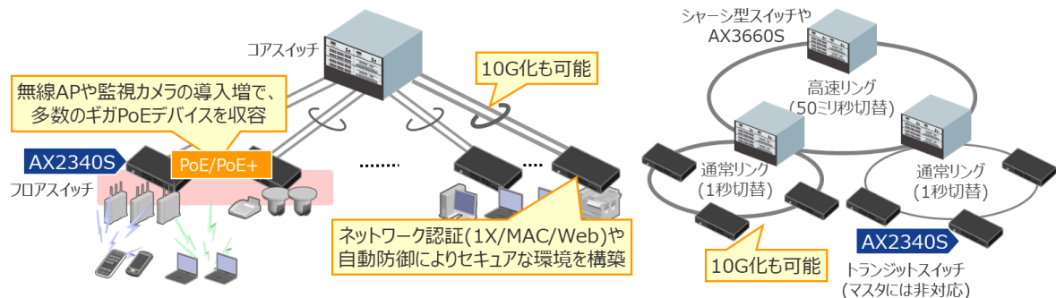
図 6 AX2340S を用いたネットワーク構成例
