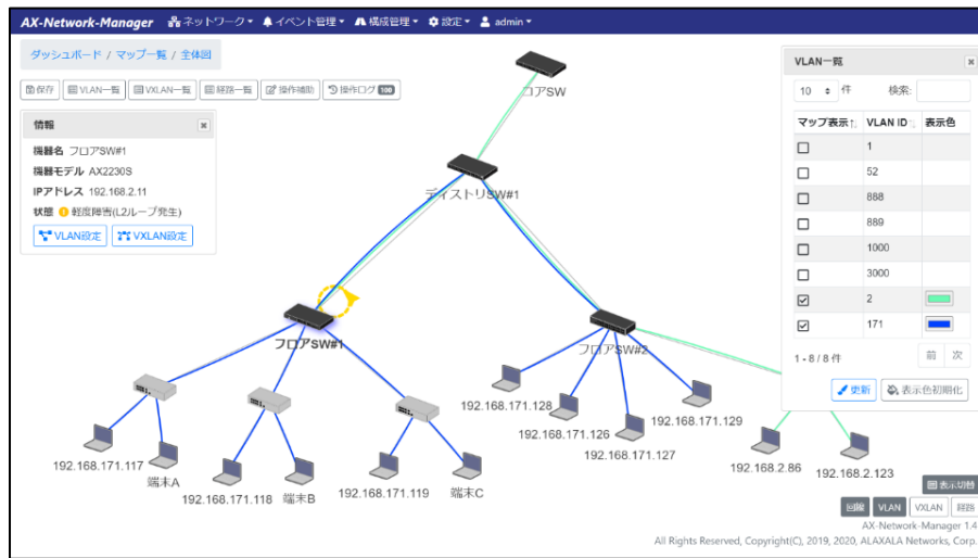
本サービスのGUI管理画面例
