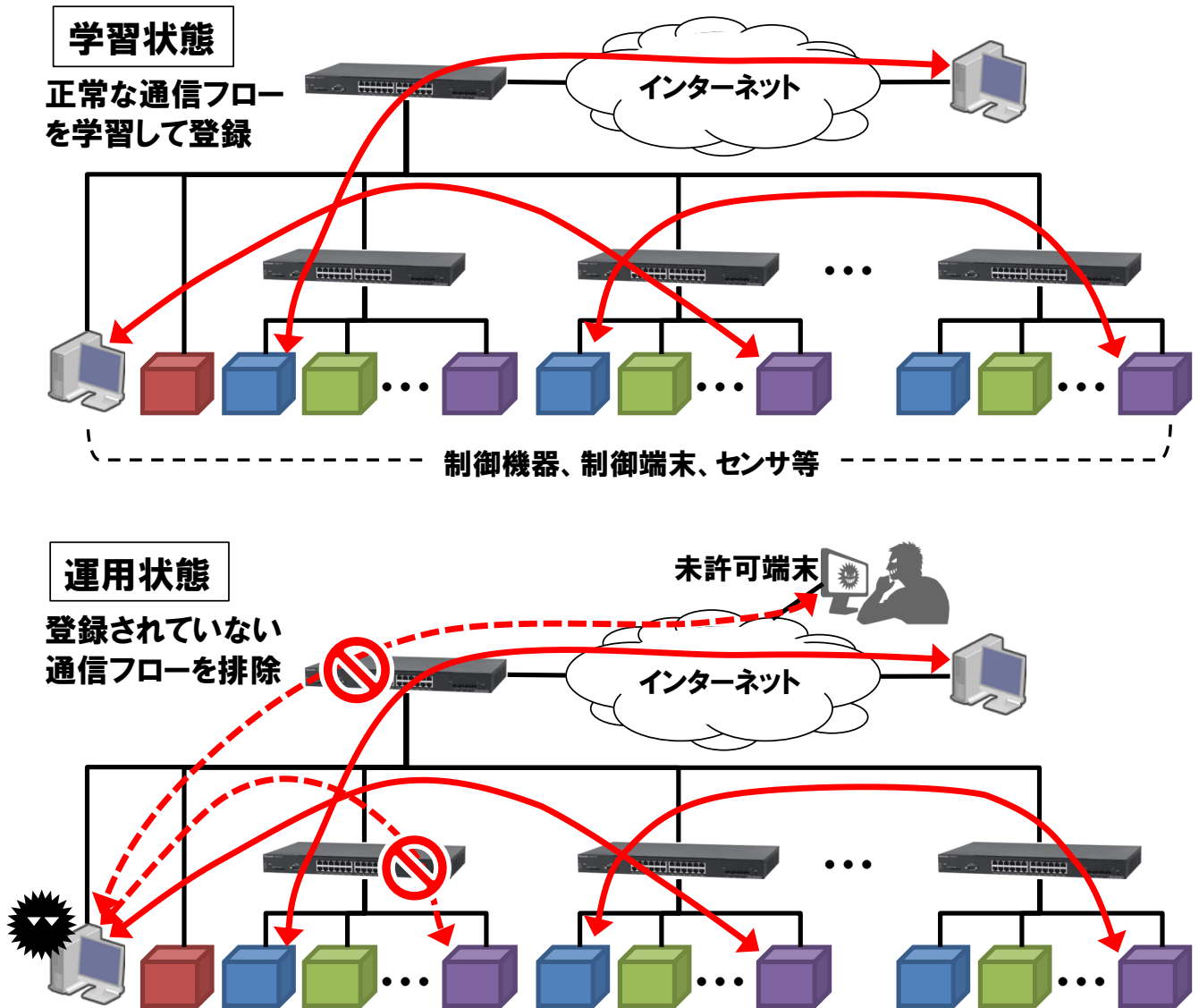
図 ホワイトリスト機能の動作
