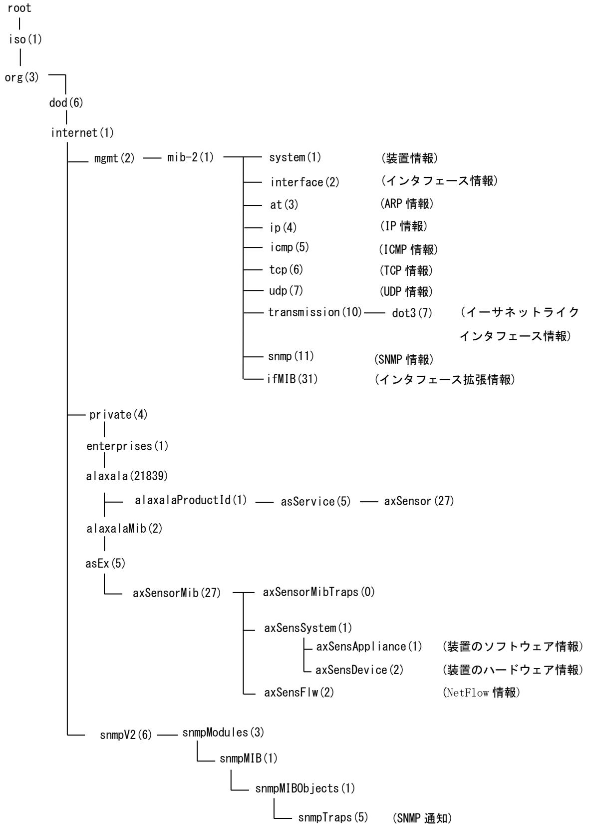
図 1.1-1 MIB 体系図
