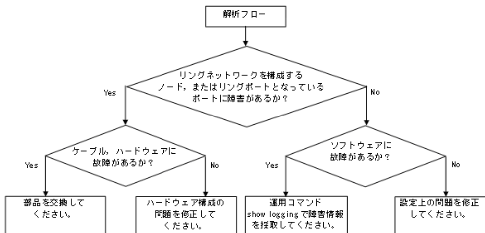
図 3-2 解析フロー
