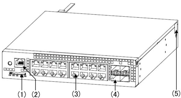
図 2-2b AX2130S-16P モデル
