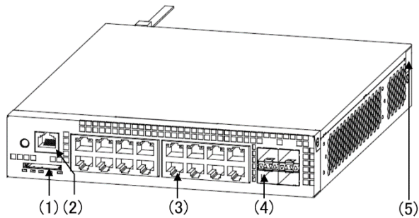
図 2-2a AX2130S-16T モデル
