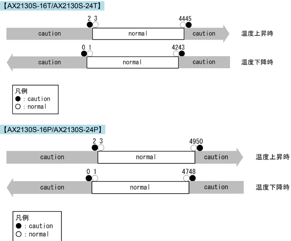
図 7-5 運用環境レベルと温度値【AX2100S】
