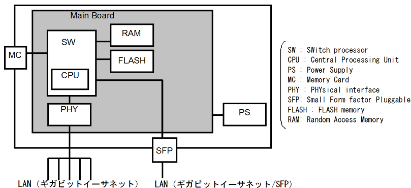
図 2-10a ハードウェアの構成 (AX2130S-16T モデル)
