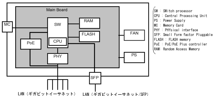
図 2-10b ハードウェアの構成 (AX2130S-16P モデル)
