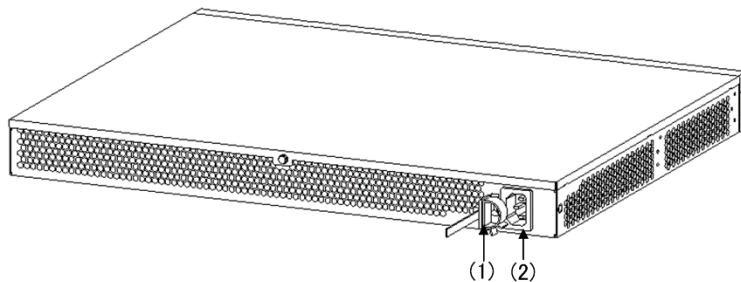
図 1-21b 背面外観
