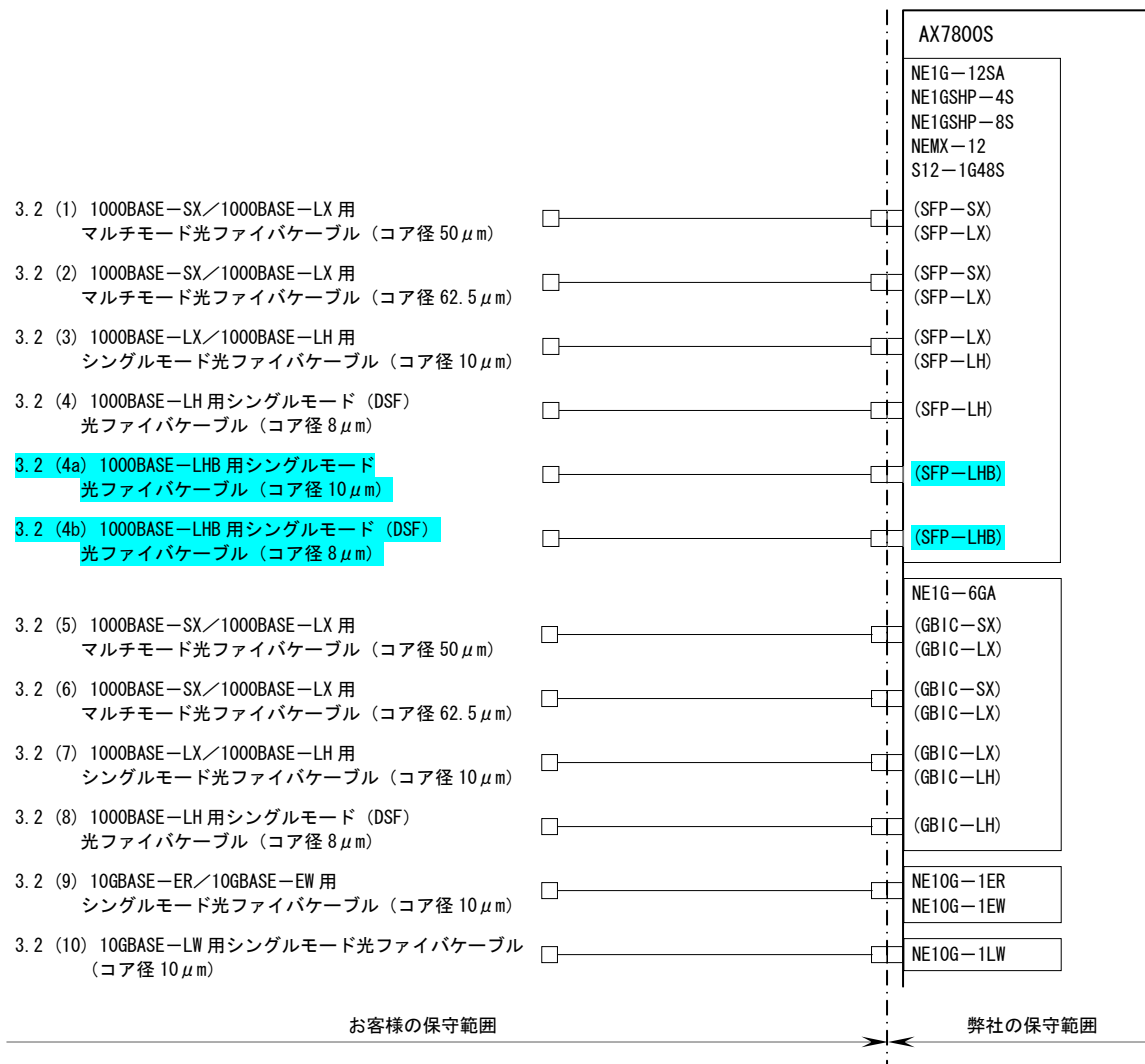
図 3-1 AX7800S シリーズ接続ケーブル系統図
