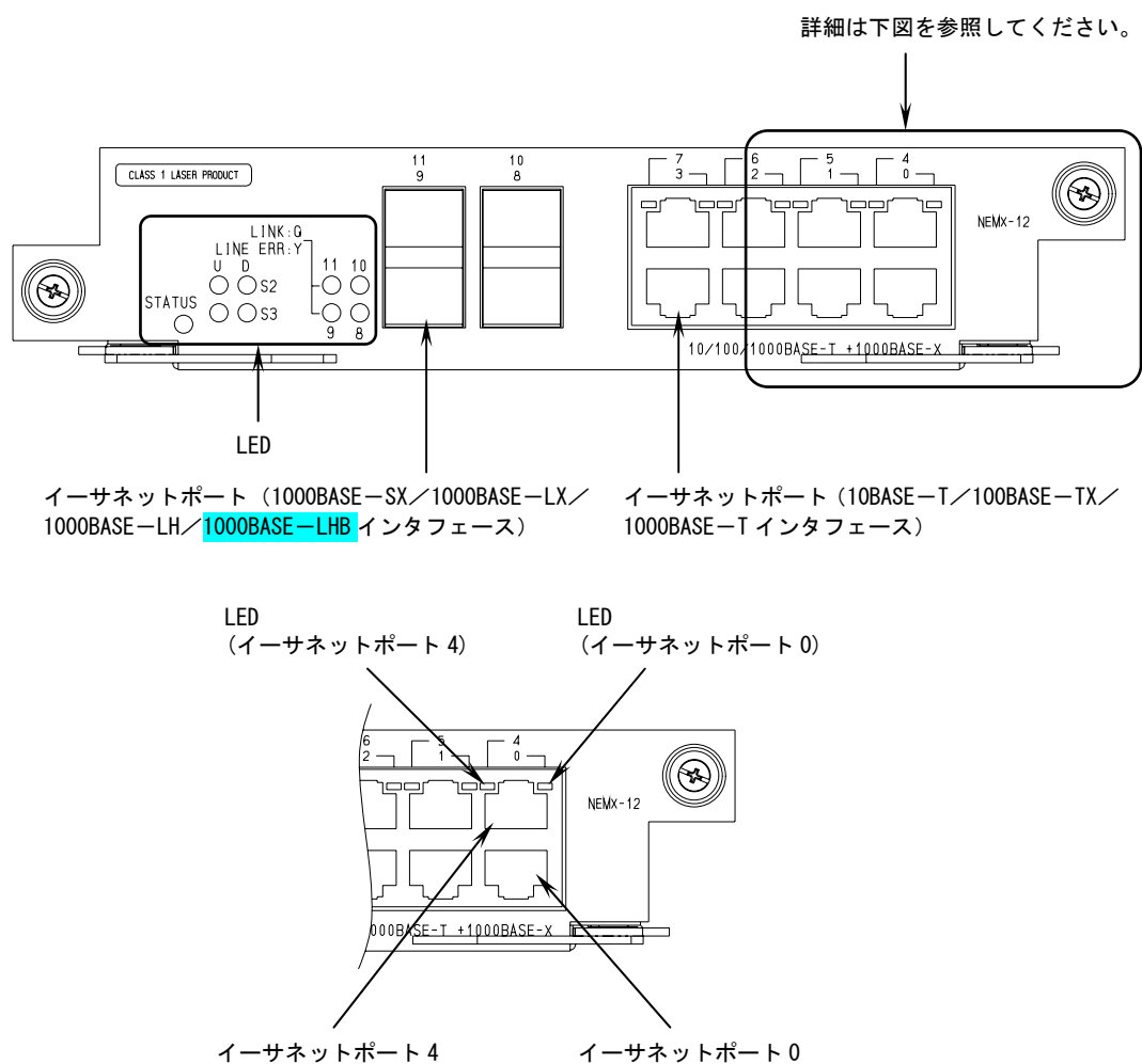
図 1-69 NEMX-12 の正面外観
