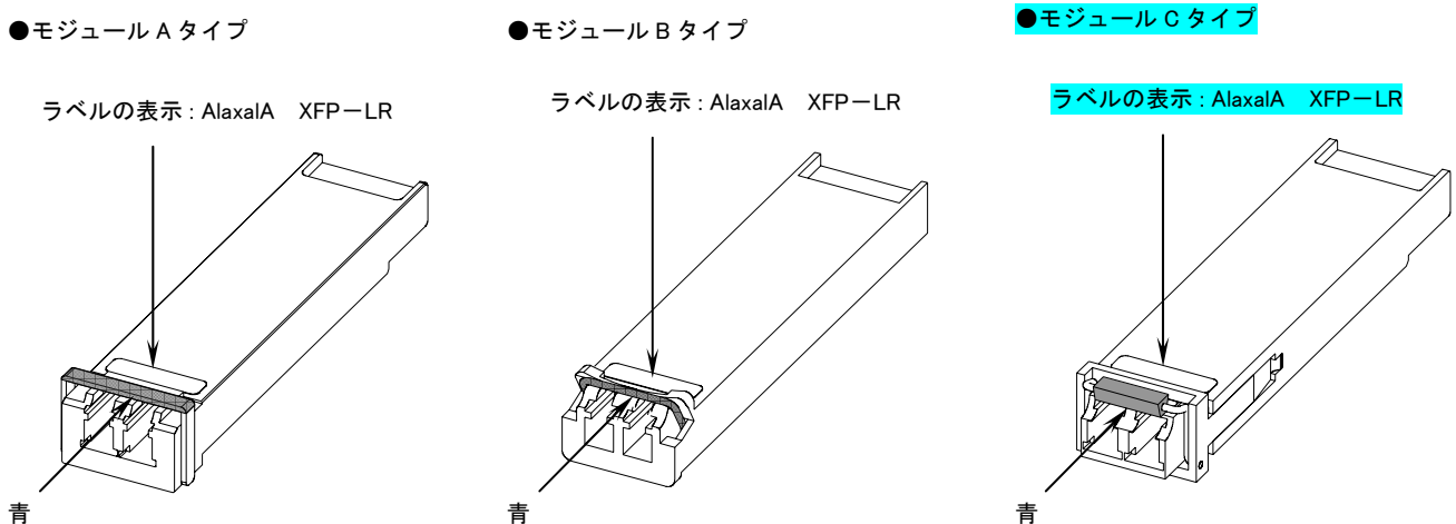
図 1-99 XFP-LRの外観
