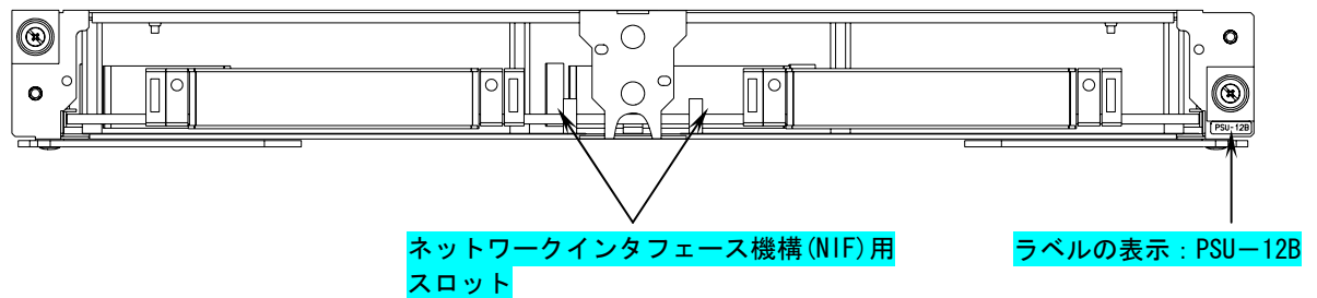
図 1-57a PSU-12B の正面外観
