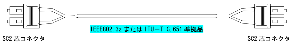
図 3-6 1000BASE-SX/1000BASE-LX 用マルチモード光ファイバケーブル (コア径 50 \mu m) の概略図
