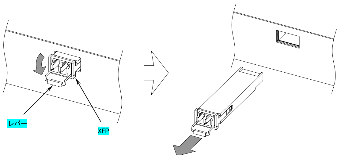
図 4-72b モジュール C タイプの取り外し
