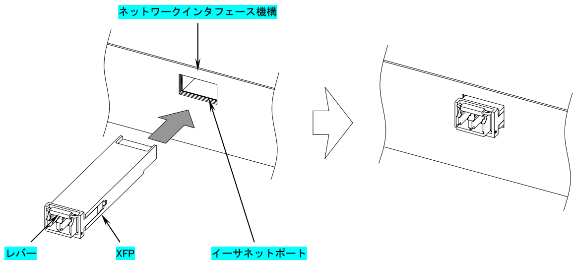
図 4-72a モジュール C タイプの取り付け
