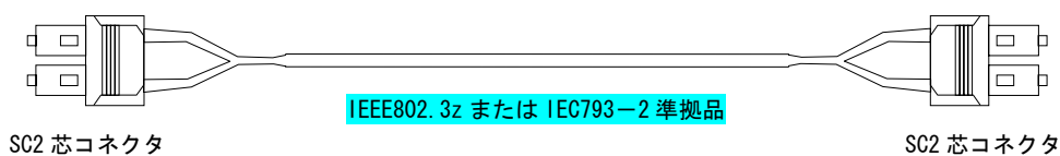
図 3-7 1000BASE-SX/1000BASE-LX 用マルチモード光ファイバケーブル (コア径 62.5 \mu m) の概略図
