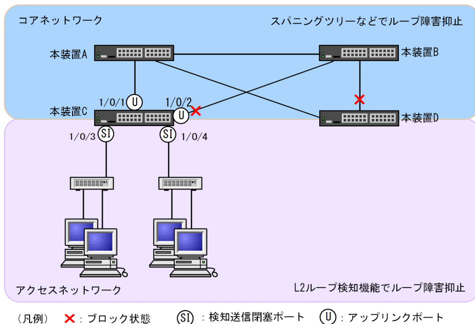
図 16-6 L2 ループ検知の設定例
