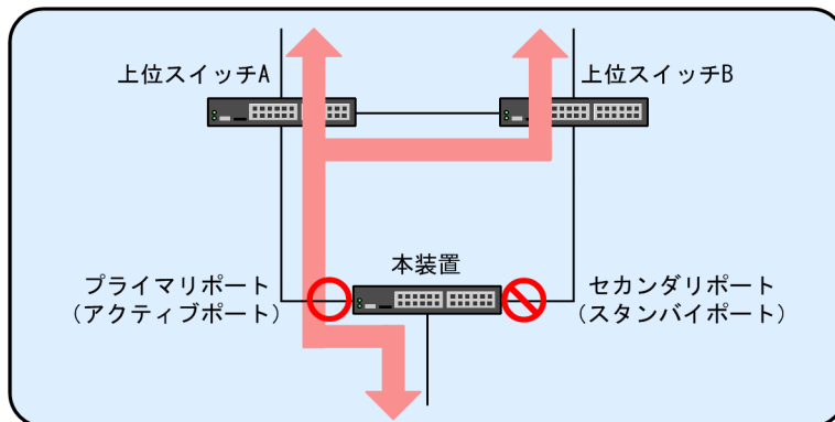
図 15-2 アップリンク・リダンダントの動作概要
