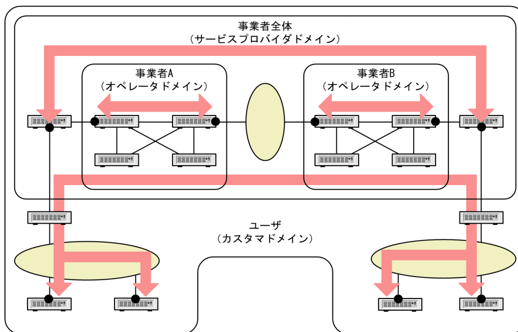
図 22-1 CFM の構成例
