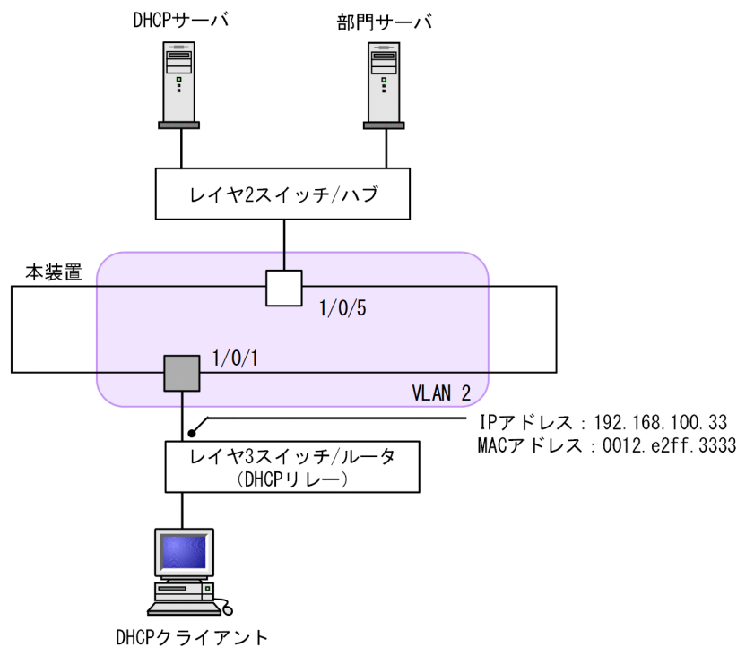
図 13-12 本装置の配下に DHCP リレーを接続した場合の構成例
