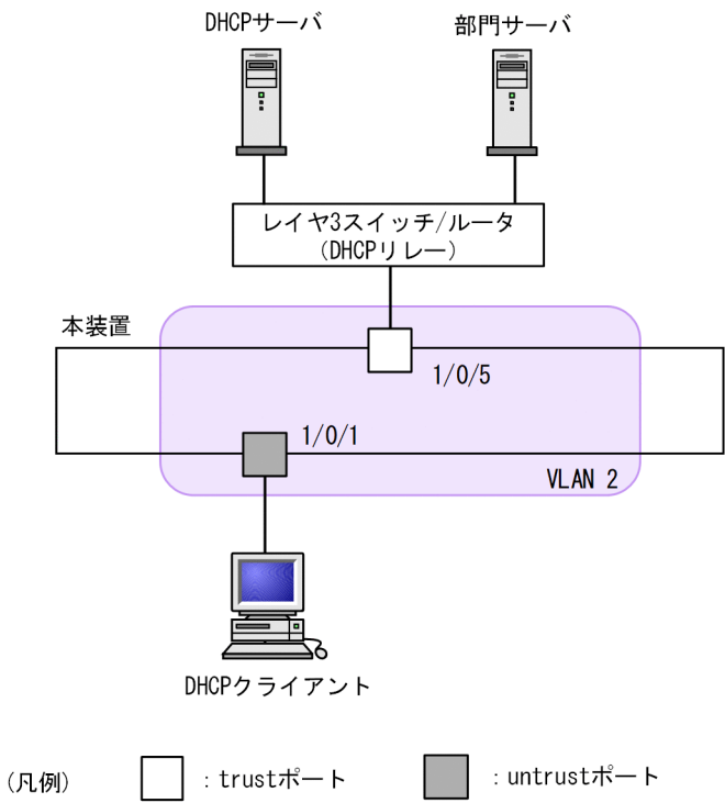
図 13-10 DHCP snooping の基本的な構成例
