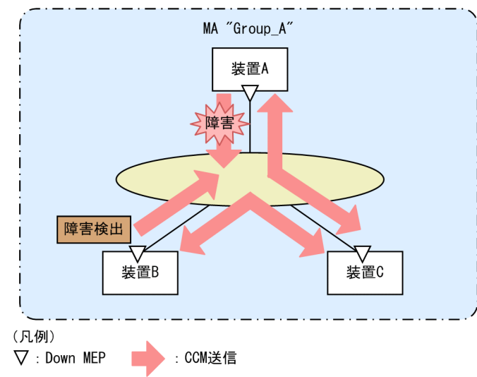
図 22-19 CC で障害を検出
