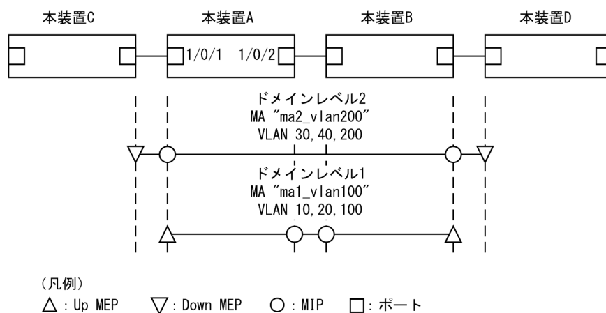
図 22-31 CFM の設定例 (複数ドメイン)
