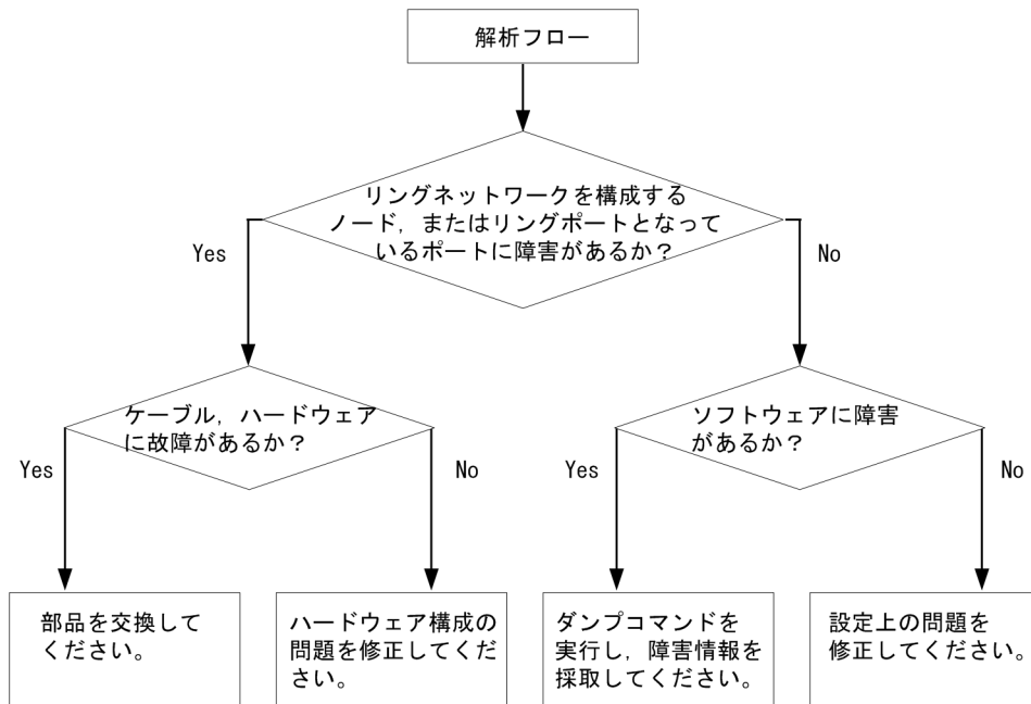
図 4-1 解析フロー
